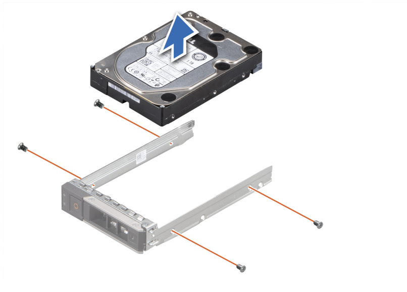
Abbildung 36. Laufwerk aus Laufwerksträger entfernen
