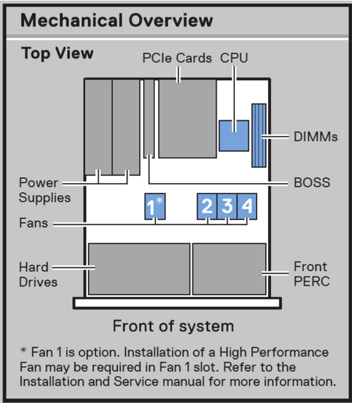
Abbildung 10. Mechanische Übersicht
