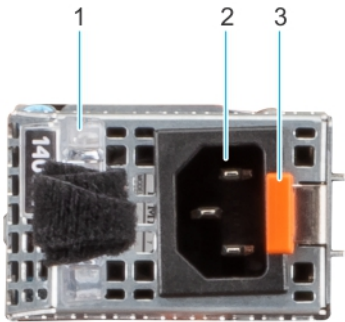
Figure 11. Configuration de l'accès par l'arrière : Voyant d'état du bloc d'alimentation secteur
