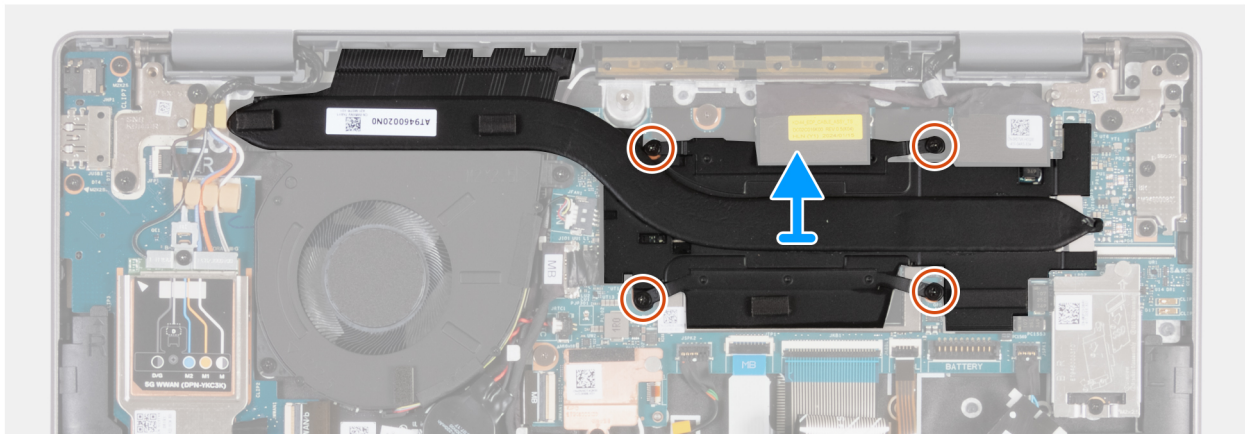
Afbeelding 44. De koelplaat verwijderen
