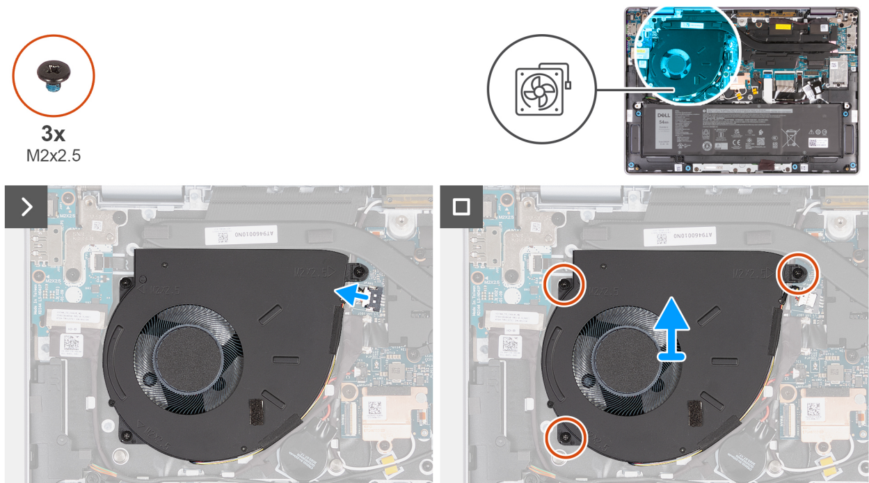
Afbeelding 35. De ventilator verwijderen (voor computers die worden geleverd met alleen WLAN-ondersteuning)
