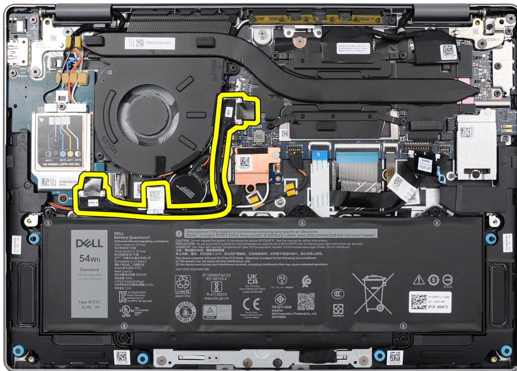
Afbeelding 52. Locatie van de kabel van de I/O-kaart
