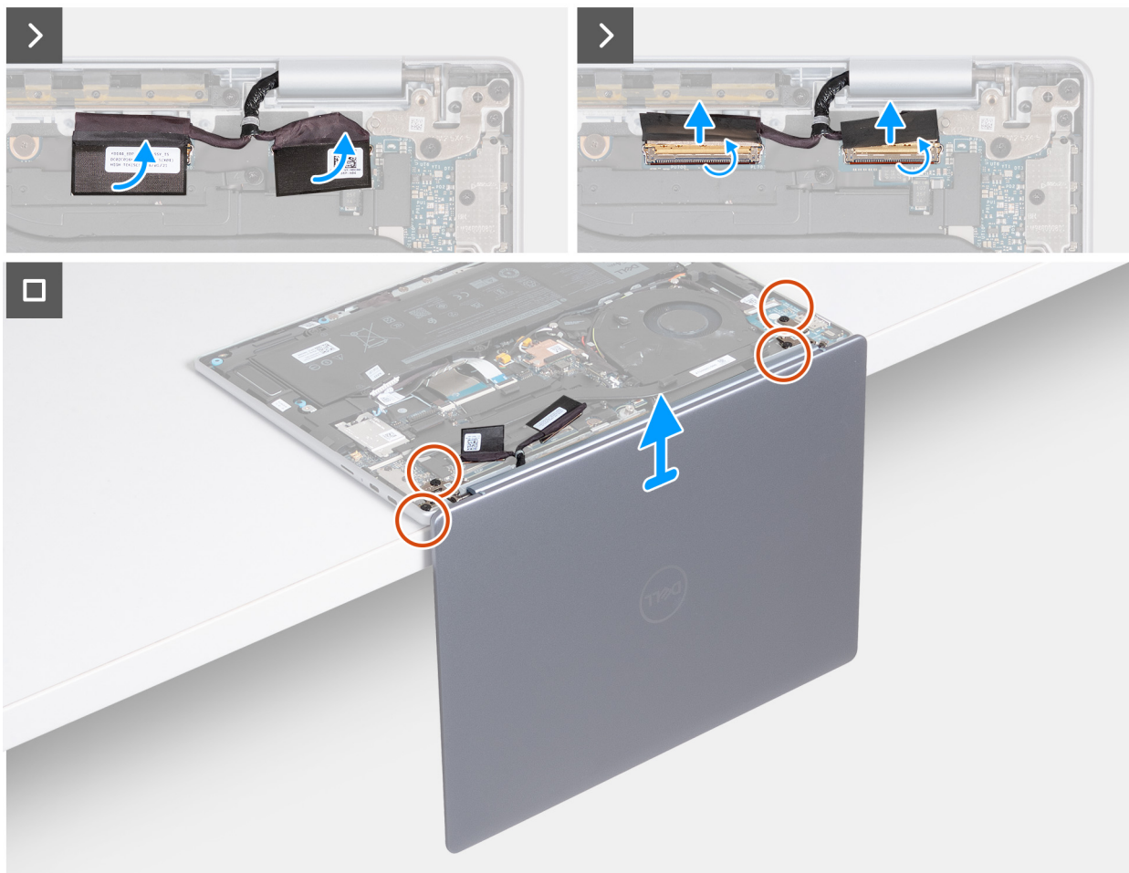
Afbeelding 74. De beeldschermeenheid verwijderen (voor computers die worden geleverd met alleen WLAN-ondersteuning)
