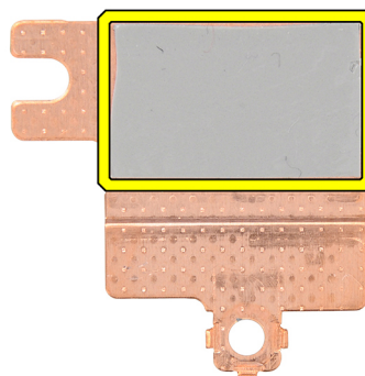
Afbeelding 67. Thermische pad onder het thermische schild van de WLAN-kaart
