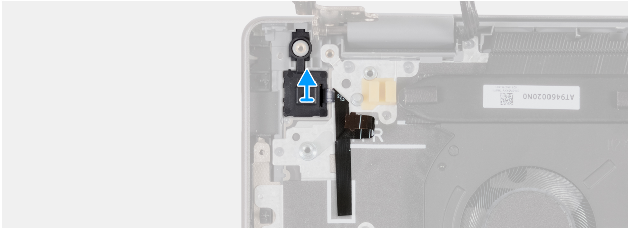
Afbeelding 89. De aan-uitknop met vingerafdrukkezer verwijderen
