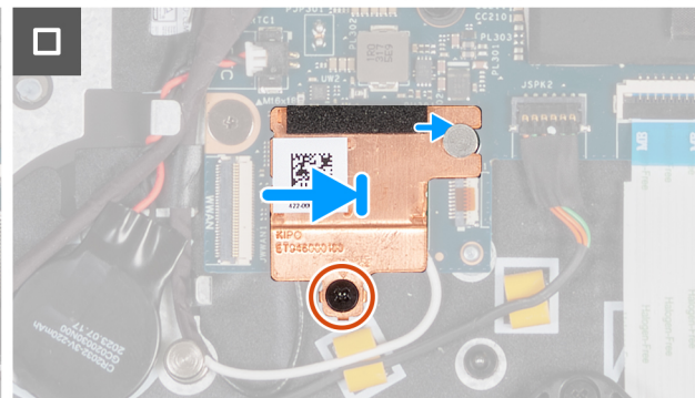
Afbeelding 61. De WLAN-antennemodule plaatsen (voor computers die worden geleverd met alleen WLAN-ondersteuning)
