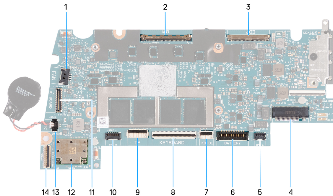
Afbeelding 96. Systemkaartconnectoren
