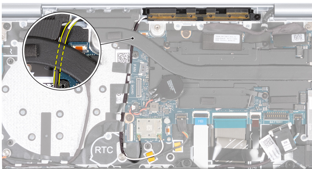
Afbeelding 60. WLAN-antennekabels verwijderen
