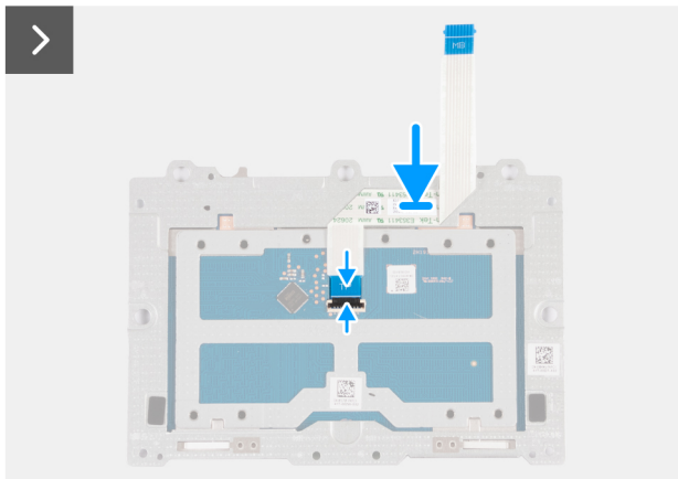
Afbeelding 87. De touchpadeenheid plaatsen
