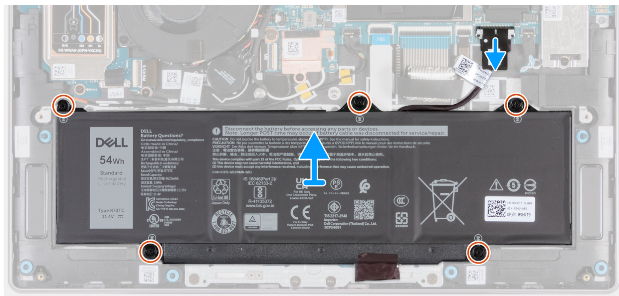
Afbeelding 39. De batterij verwijderen
