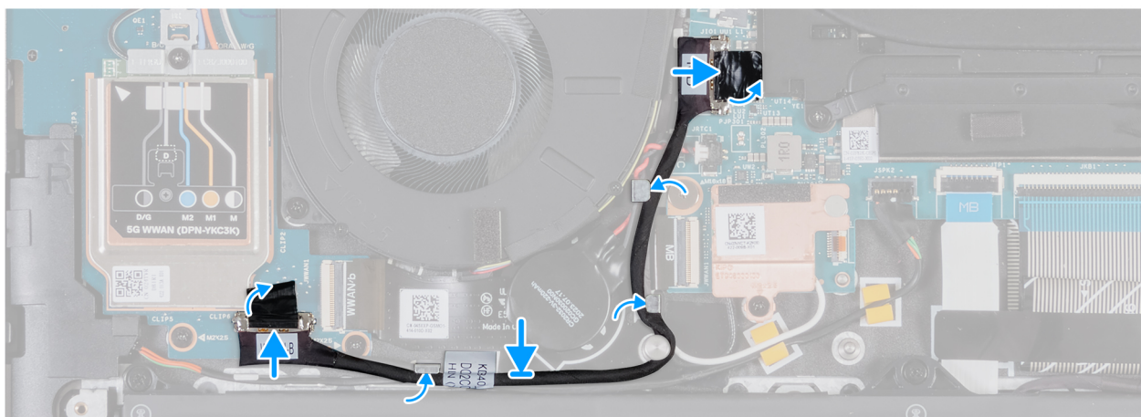
Afbeelding 55. De kabel van de I/O-kaart plaatsen (voor computers die worden geleverd met WWAN-ondersteuning)
