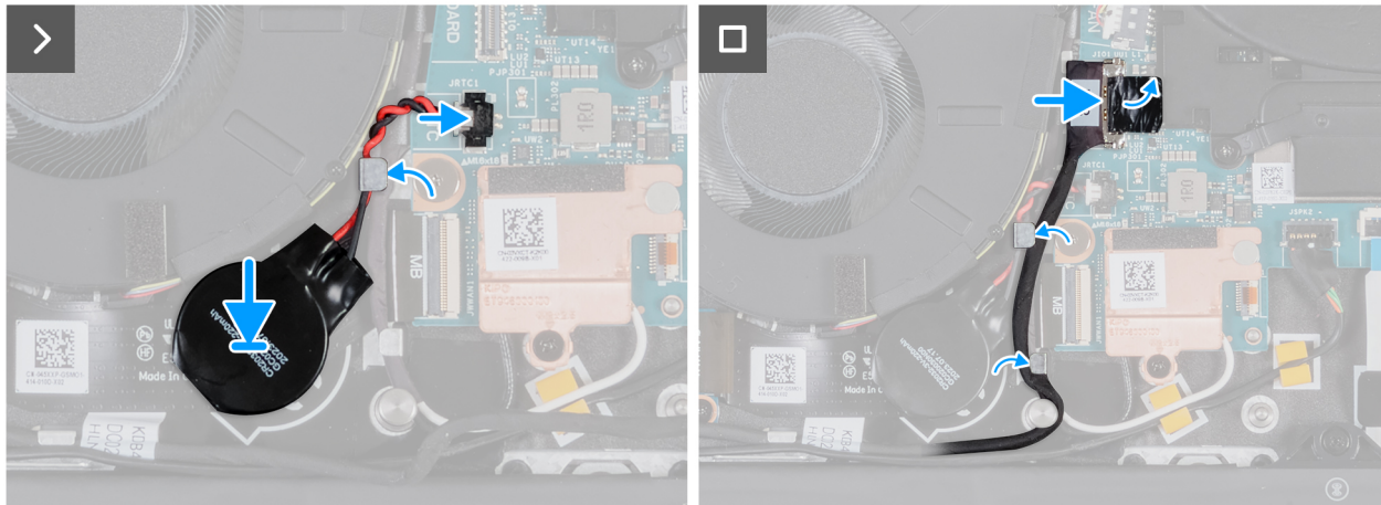
Afbeelding 47. De knoopcelbatterij plaatsen
