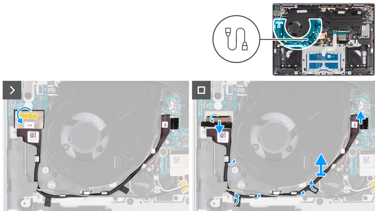
Afbeelding 49. De kabel van de I/O-kaart verwijderen (voor computers die worden geleverd met alleen WLAN-ondersteuning)
