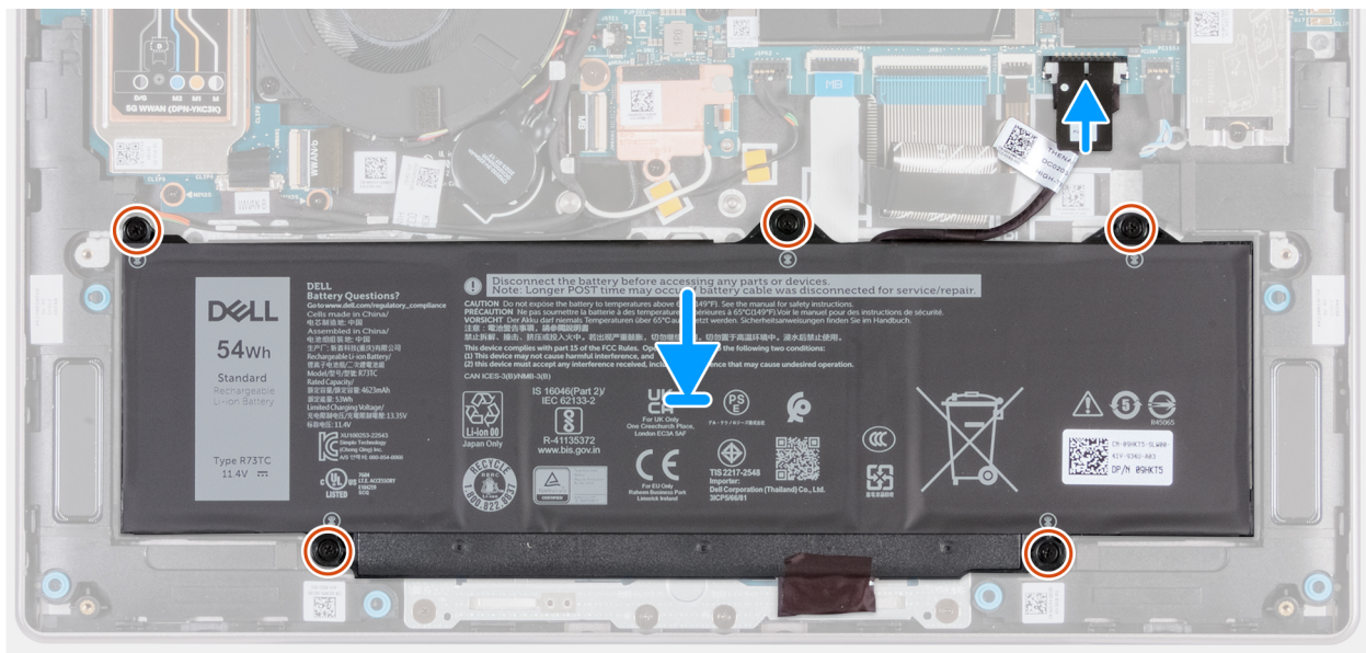
Afbeelding 40. De batterij plaatsen
