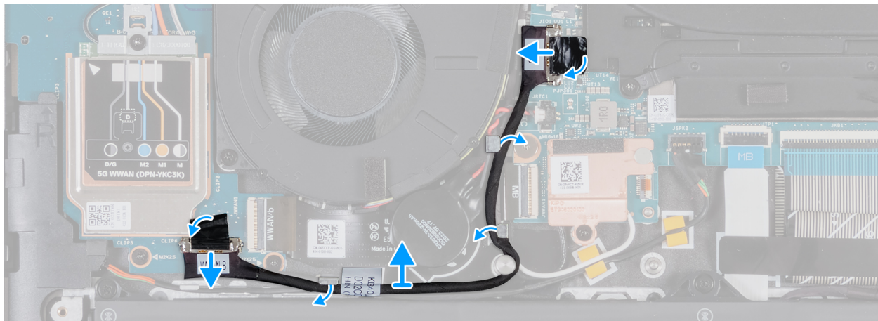
Afbeelding 53. De kabel van de I/O-kaart verwijderen (voor computers die worden geleverd met WWAN-ondersteuning)
