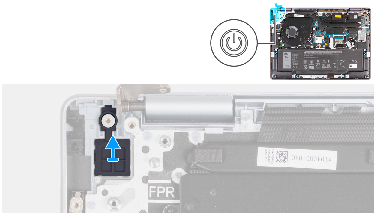
Afbeelding 88. De aan-uitknop verwijderen
