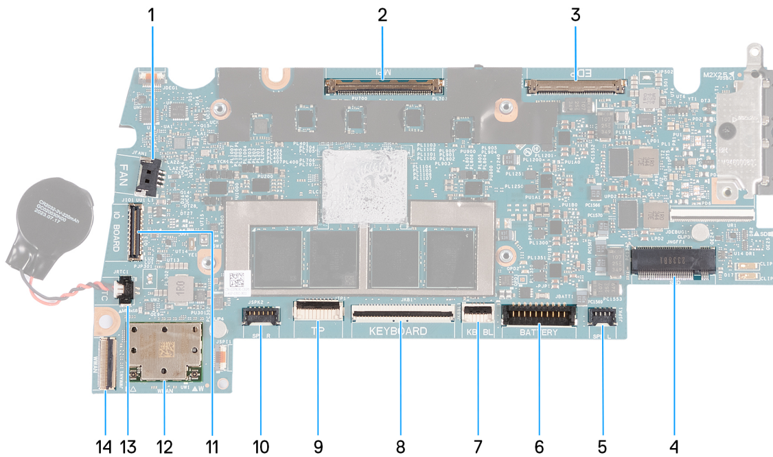
Afbeelding 93. Systemkaartconnectoren
