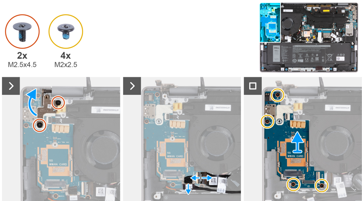
Afbeelding 84. De I/O-kaart verwijderen (voor computers die worden geleverd met WWAN-ondersteuning)
