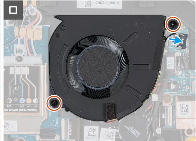
Afbeelding 38. De ventilator plaatsen (voor computers die worden geleverd met WWAN-ondersteuning)
