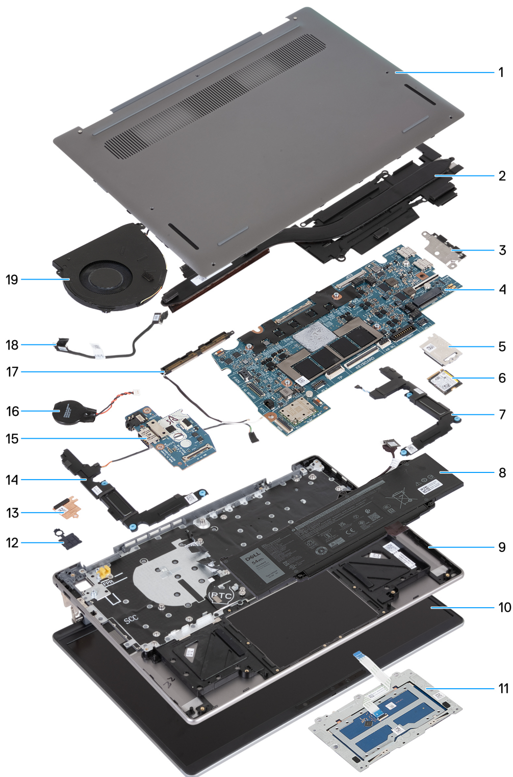
Afbeelding 9. Belangrijkste onderdelen van de Latitude 7455 (computers die worden geleverd met alleen WLAN-ondersteuning)
