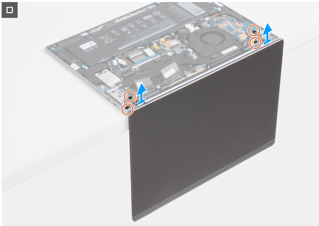
Afbeelding 78. De beeldschermeenheid verwijderen (voor computers die worden geleverd met WWAN-ondersteuning)
