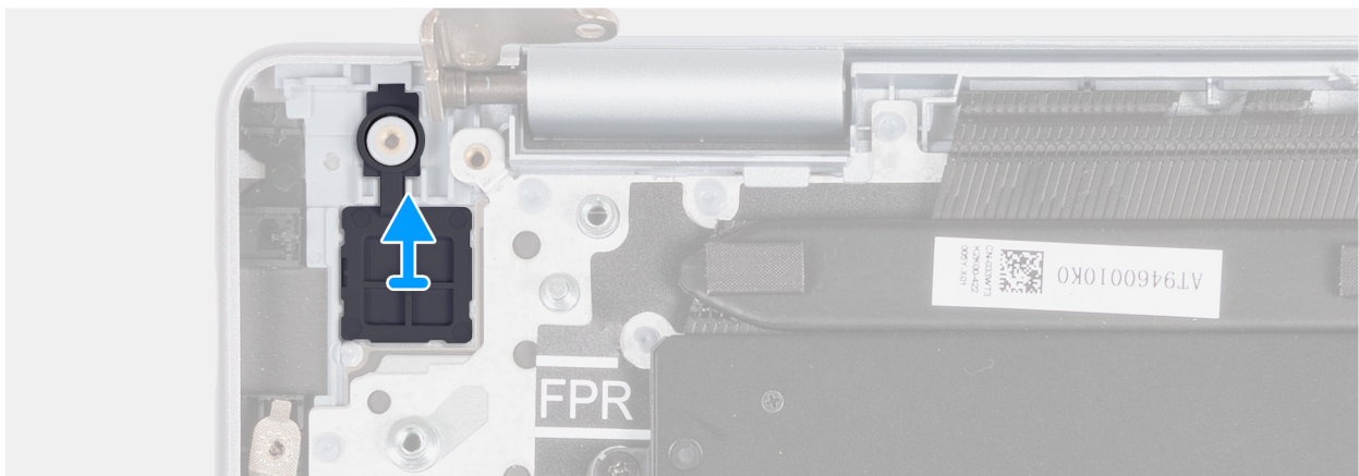
Afbeelding 88. De aan-uitknop verwijderen
