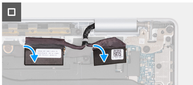
Afbeelding 76. De beeldscherm eenheid plaatsen (voor computers die worden geleverd met alleen WLAN-ondersteuning)
