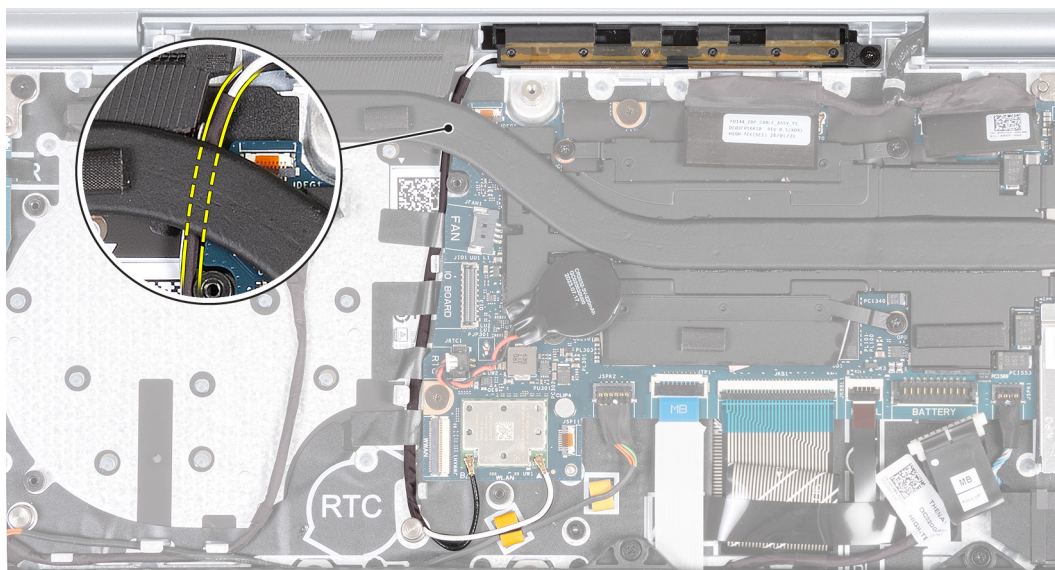
Afbeelding 60. WLAN-antennekabels verwijderen
