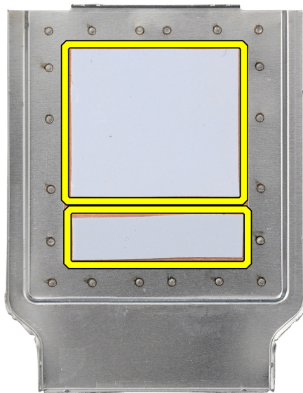
Afbeelding 27. Thermische pads aan de onderkant van het thermische schild van de WWAN-kaart
