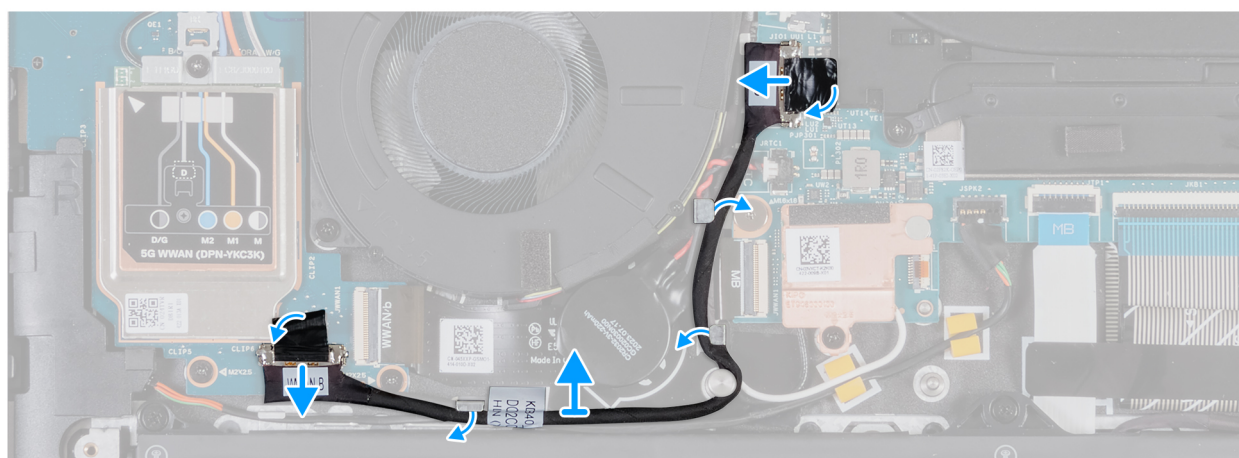
Afbeelding 53. De kabel van de I/O-kart verwijderen (voor computers die worden geleverd met WWAN-ondersteuning)
