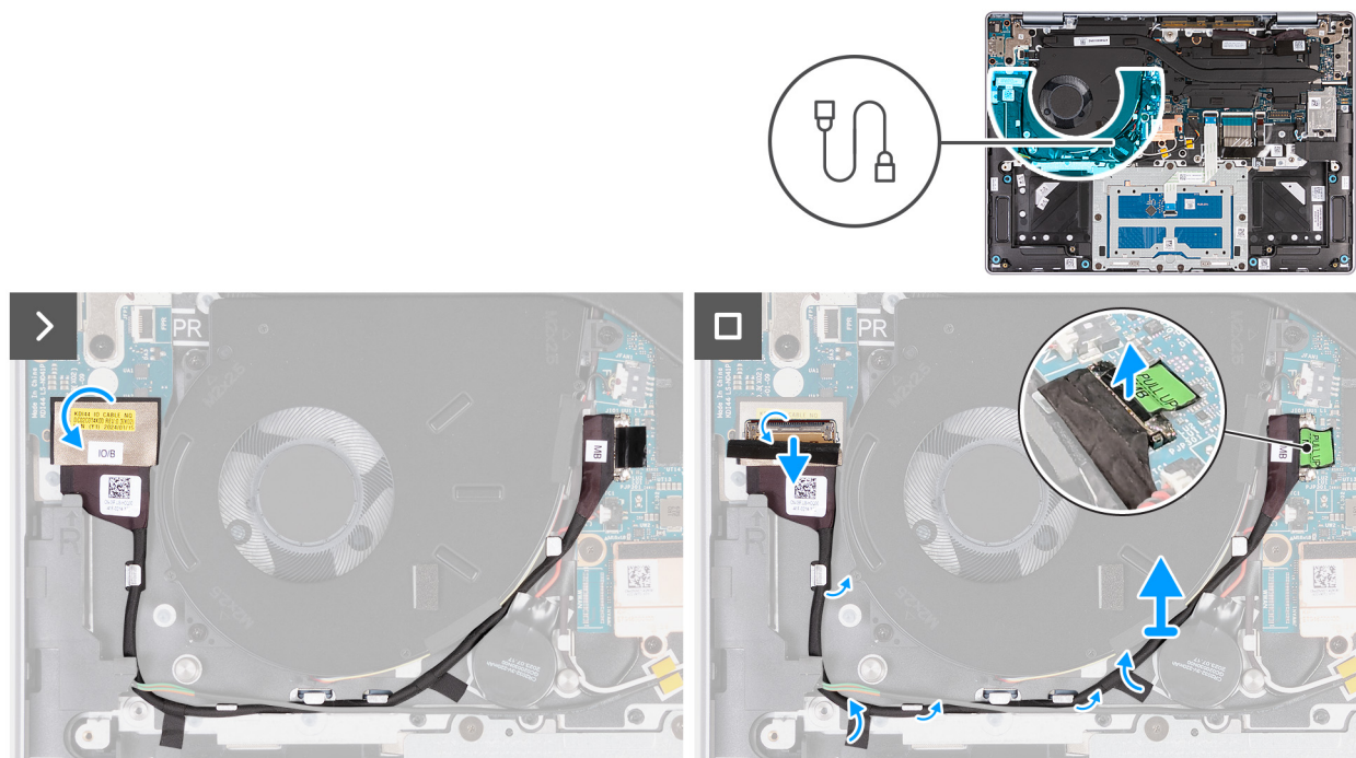
Afbeelding 49. De kabel van de I/O-kaart verwijderen (voor computers die worden geleverd met alleen WLAN-ondersteuning)
