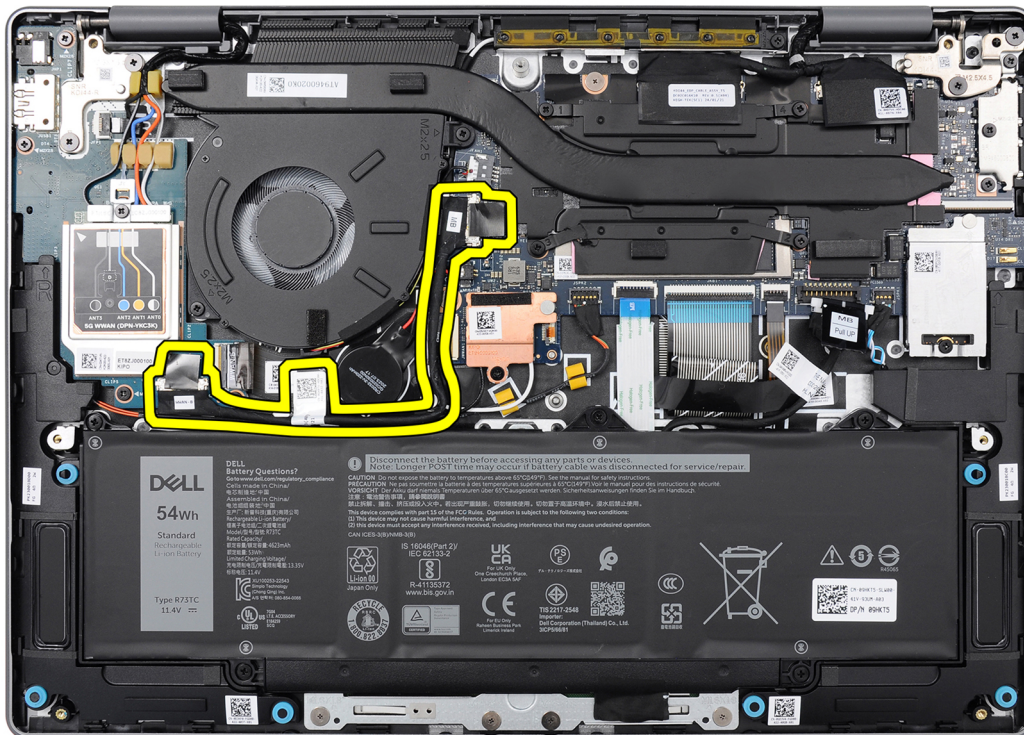
Afbeelding 52. Locatie van de kabel van de I/O-kart
