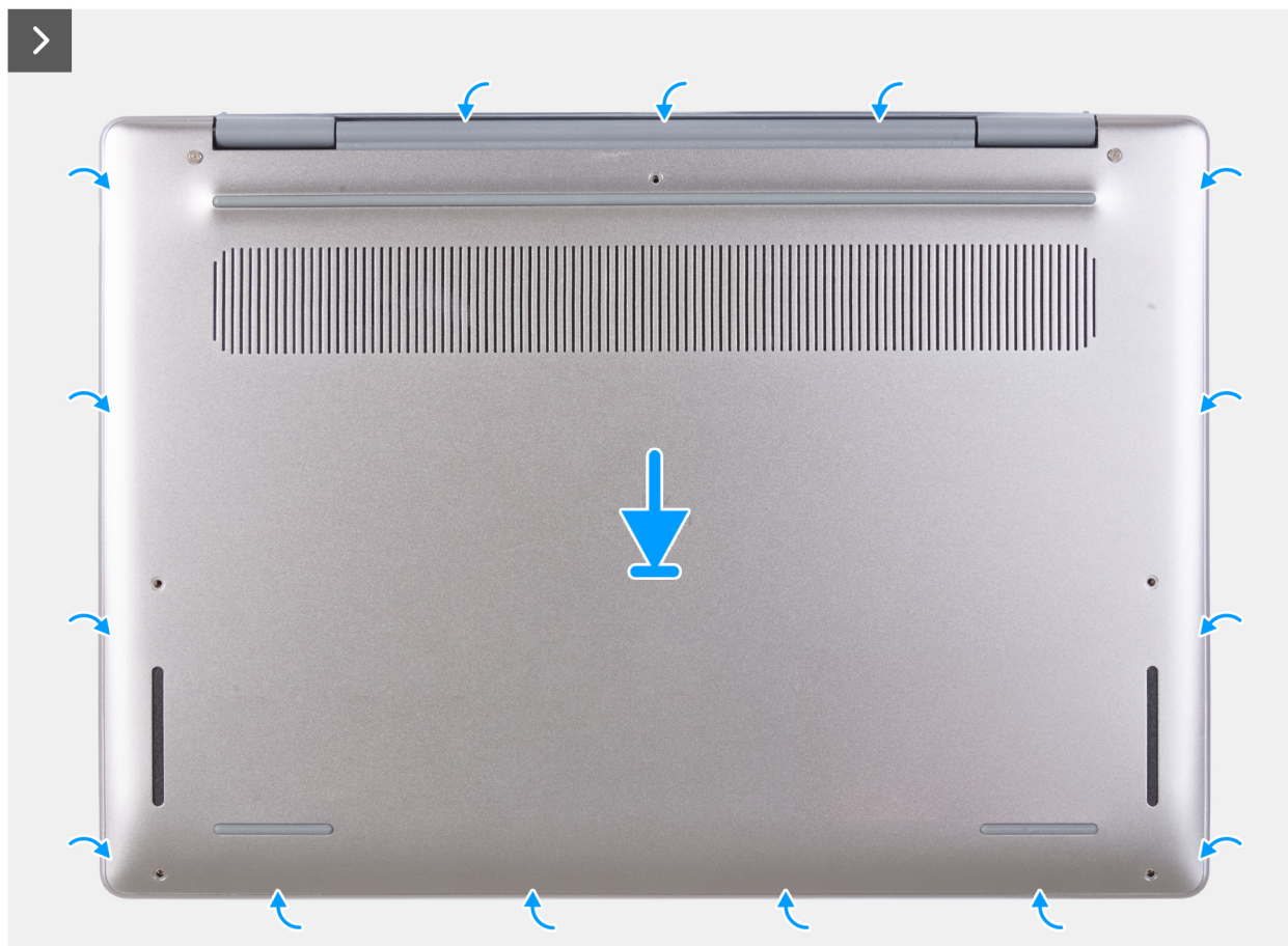
Afbeelding 19. De onderplaat plaatsen
