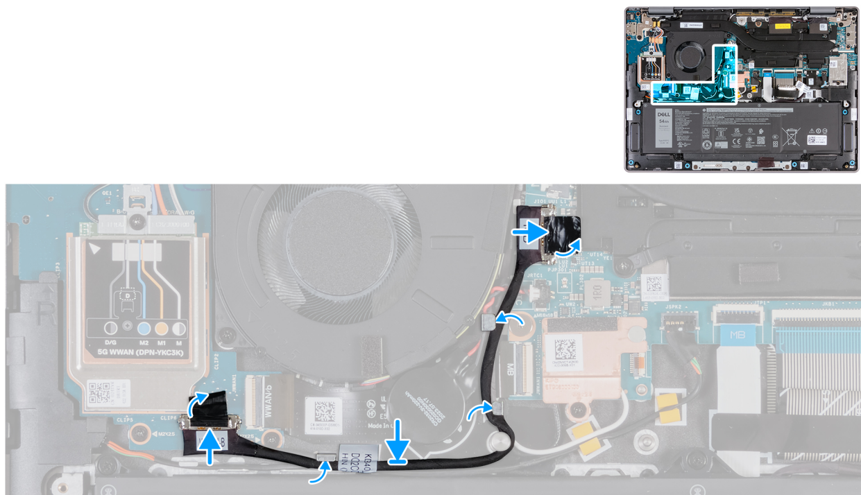
Afbeelding 55. De kabel van de I/O-kaart plaatsen (voor computers die worden geleverd met WWAN-ondersteuning)
