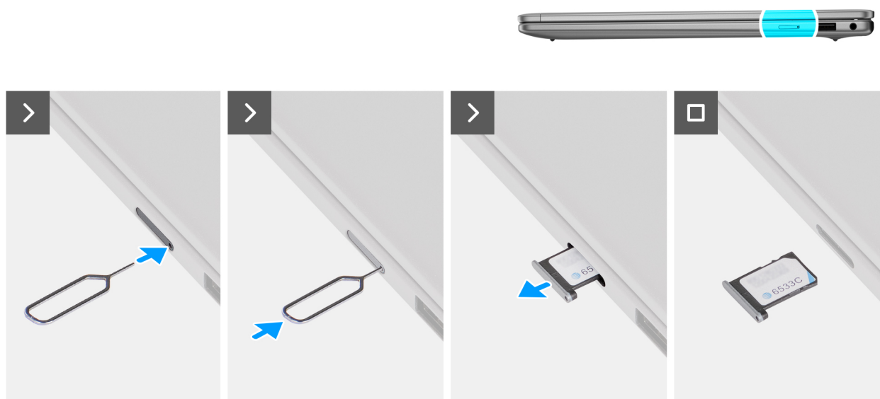
Afbeelding 13. Het simkaartvak verwijderen
