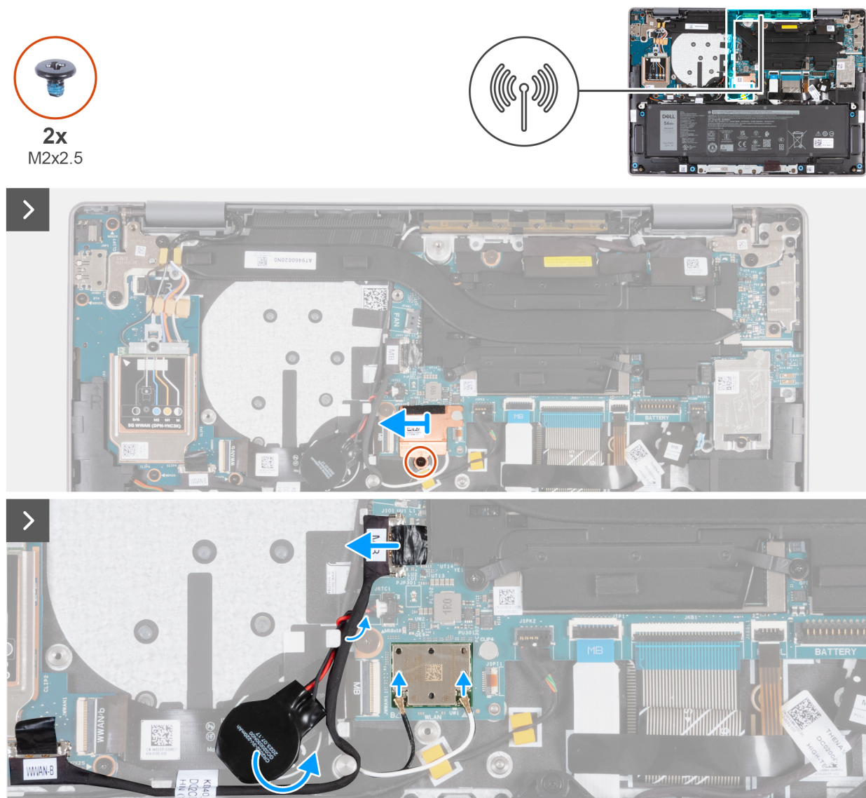
Afbeelding 65. De WLAN-antennemodule verwijderen
