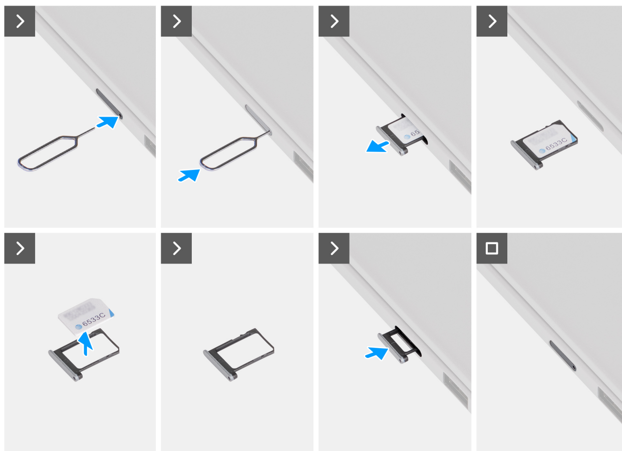
Afbeelding 11. De simkaart verwijderen
