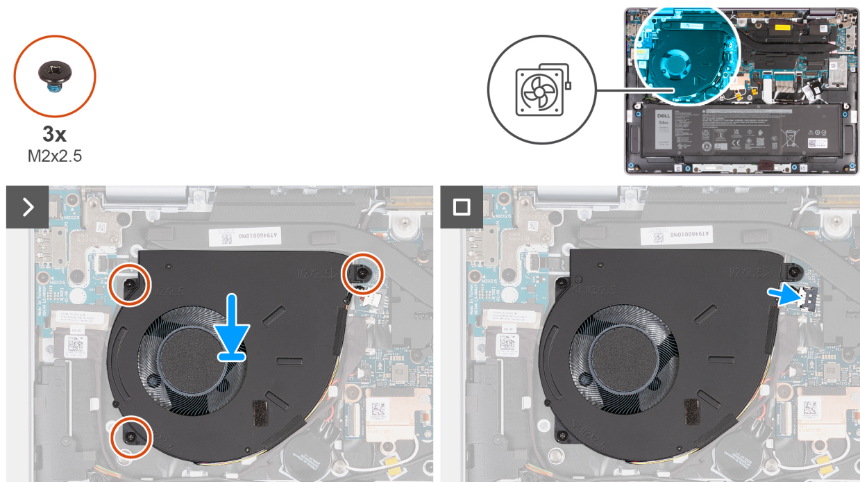
Afbeelding 36. De ventilator plaatsen (voor computers die worden geleverd met alleen WLAN-ondersteuning)
