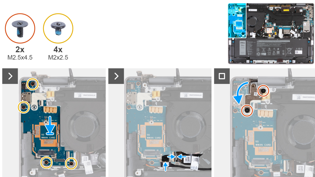
Afbeelding 85. De I/O-kaart plaatsen De I/O-kaart verwijderen (voor computers die worden geleverd met WWAN-ondersteuning)
