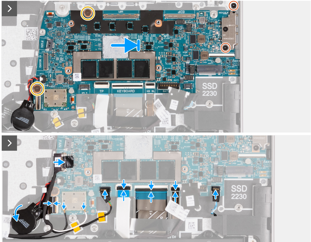
Afbeelding 98. De systeemkaart plaatsen
