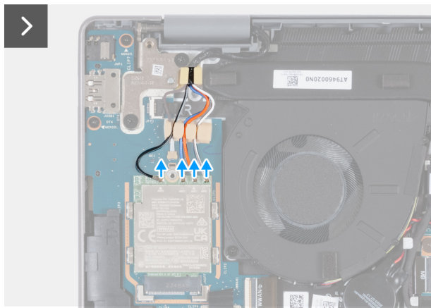
Afbeelding 26. De 5G WWAN-kaart verwijderen
