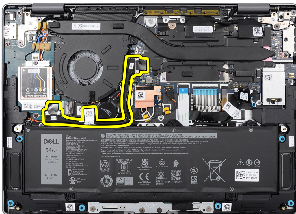
Afbeelding 54. Locatie van de kabel van de I/O-kaart
