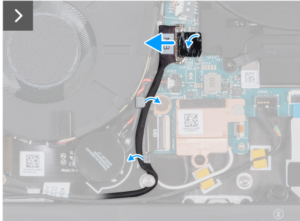
Afbeelding 46. De knoopcelbatterij verwijderen
