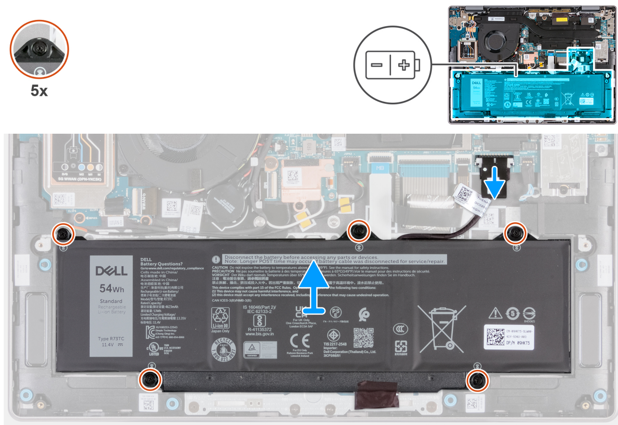
Afbeelding 39. De batterij verwijderen
