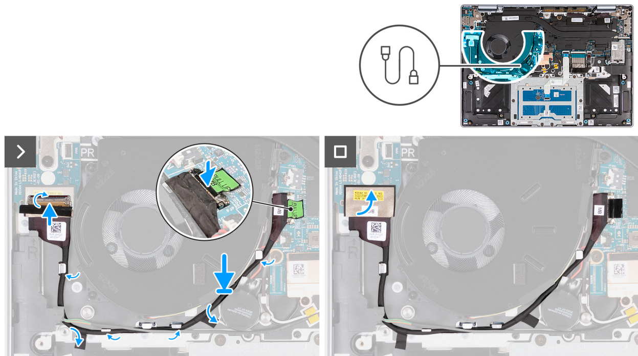
Afbeelding 51. De kabel van de I/O-kaart plaatsen (voor computers die worden geleverd met alleen WLAN-ondersteuning)
