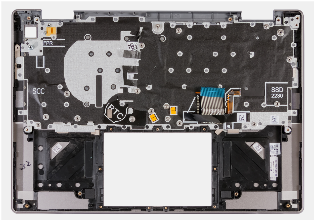
Afbeelding 101. Palmsteun- en toetsenbordeenheid
