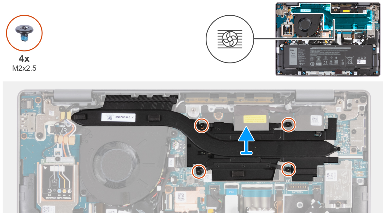
Afbeelding 44. De koelplaat verwijderen
