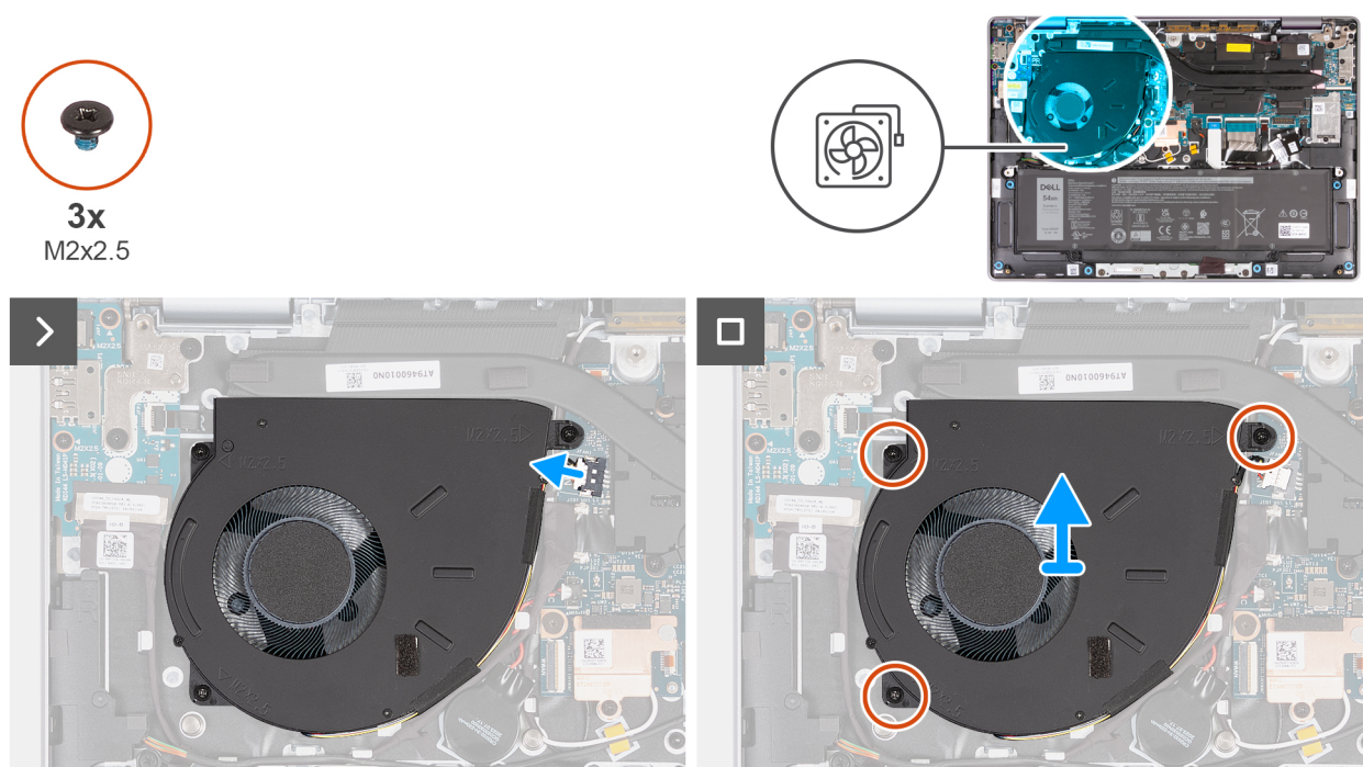
Afbeelding 35. De ventilator verwijderen (voor computers die worden geleverd met alleen WLAN-ondersteuning)
