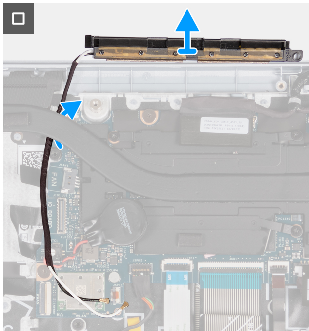
Afbeelding 58. De WLAN-antennemodule verwijderen (voor computers die worden geleverd met alleen WLAN-ondersteuning)
