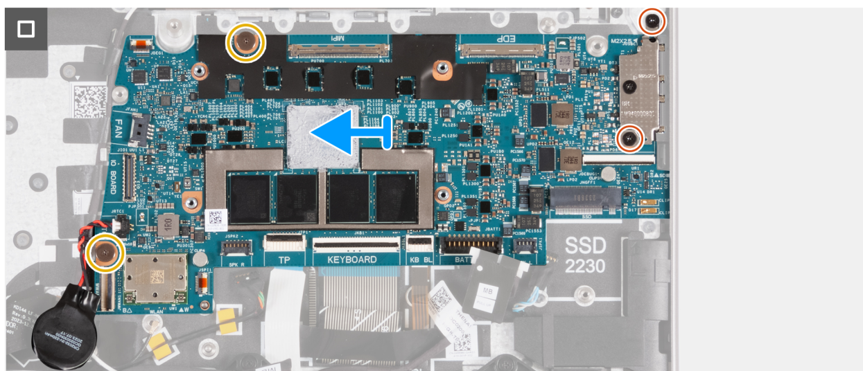
Afbeelding 95. De systeemkaart verwijderen
