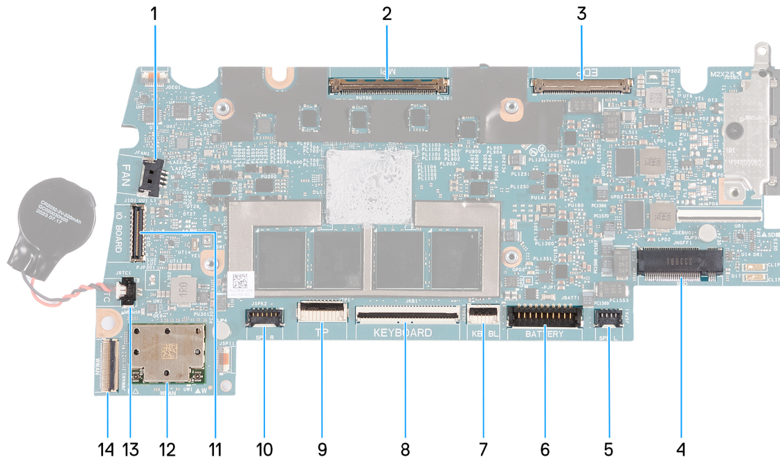
Afbeelding 97. Systeemkaartconnectoren
