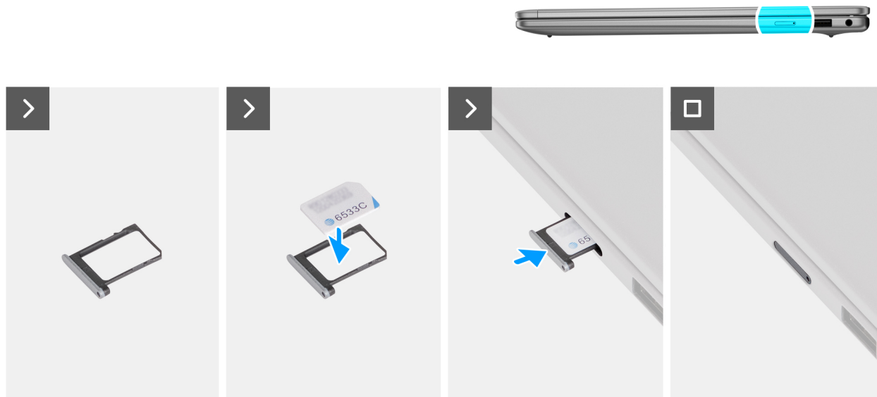
Afbeelding 14. Het simkaartvak plaatsen
