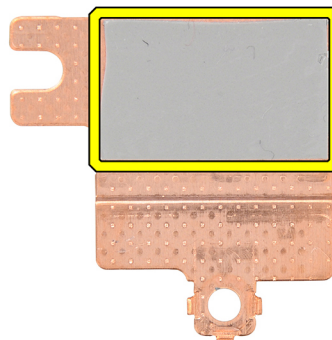
Afbeelding 67. Thermische pad onder het thermische schild van de WLAN-kaart
