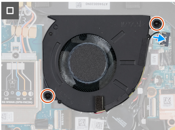
Afbeelding 38. De ventilator plaatsen (voor computers die worden geleverd met WWAN-ondersteuning)
