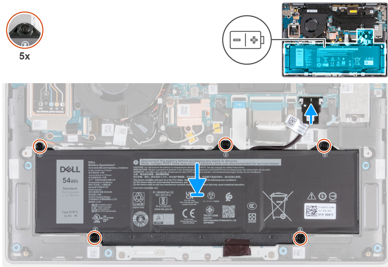
Afbeelding 40. De batterij plaatsen
