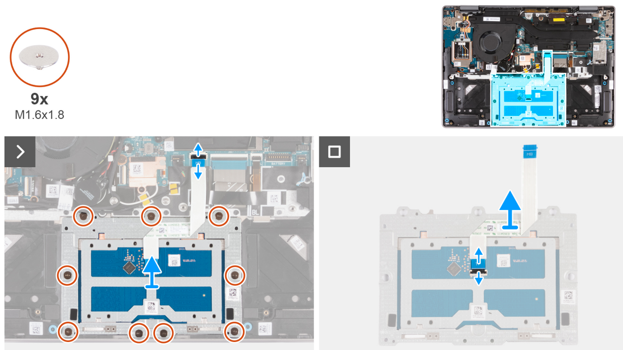
Afbeelding 86. De touchpadeenheid verwijderen
