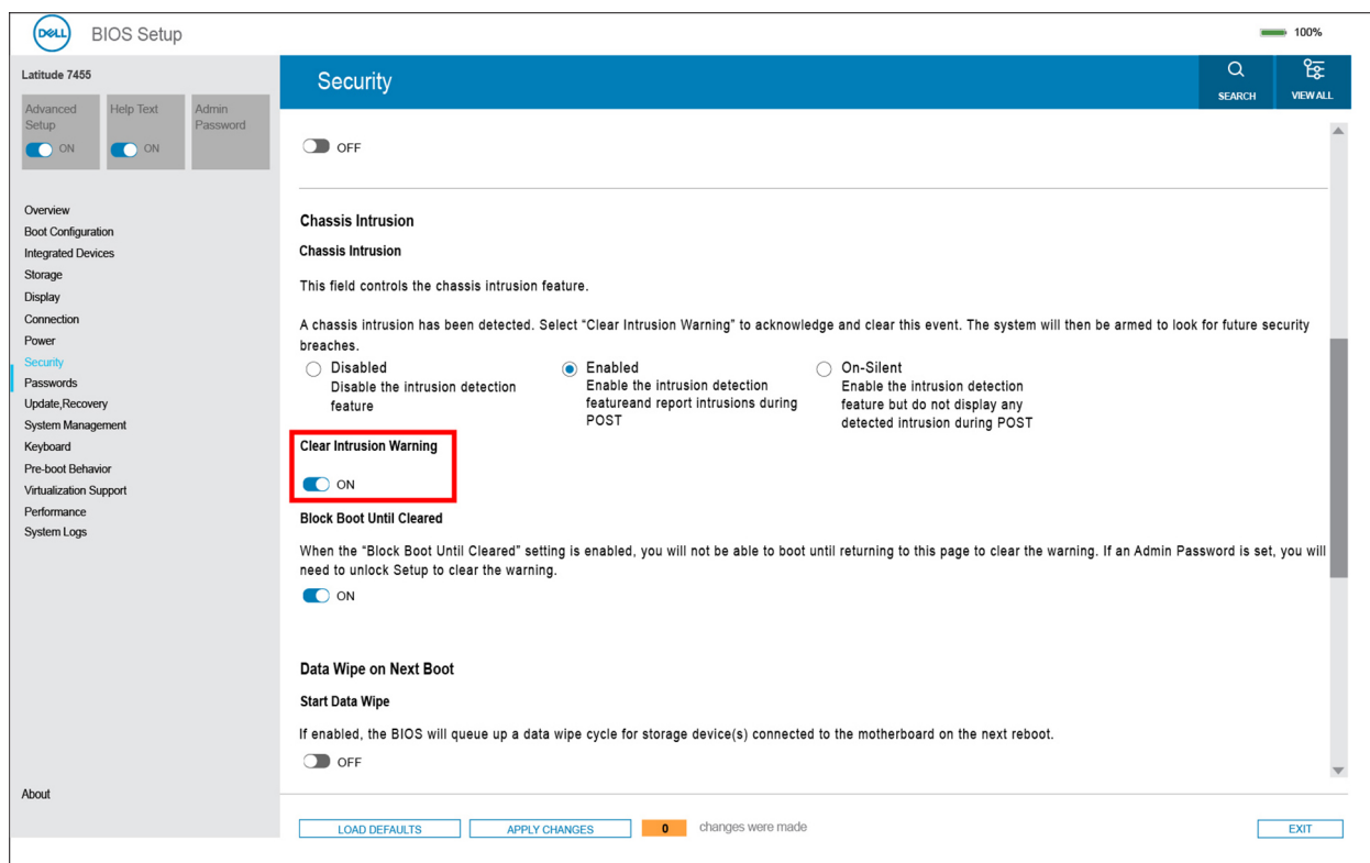
Afbeelding 105. Intrusiewaarschuwing wissen
