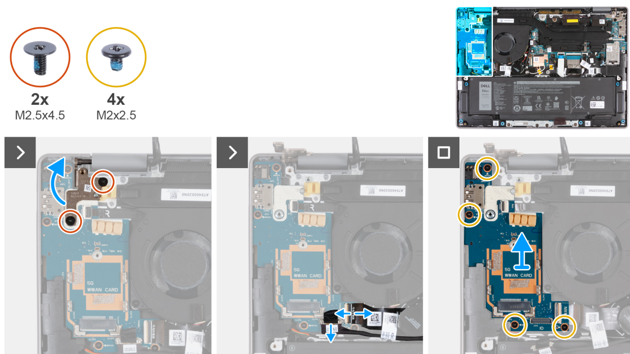
Afbeelding 84. De I/O-kaart verwijderen (voor computers die worden geleverd met WWAN-ondersteuning)
