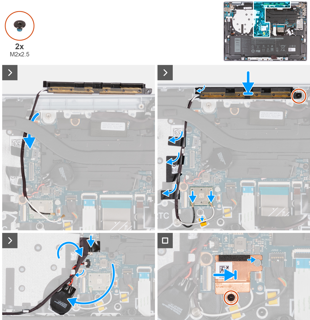
Afbeelding 61. De WLAN-antennemodule plaatsen (voor computers die worden geleverd met alleen WLAN-ondersteuning)
