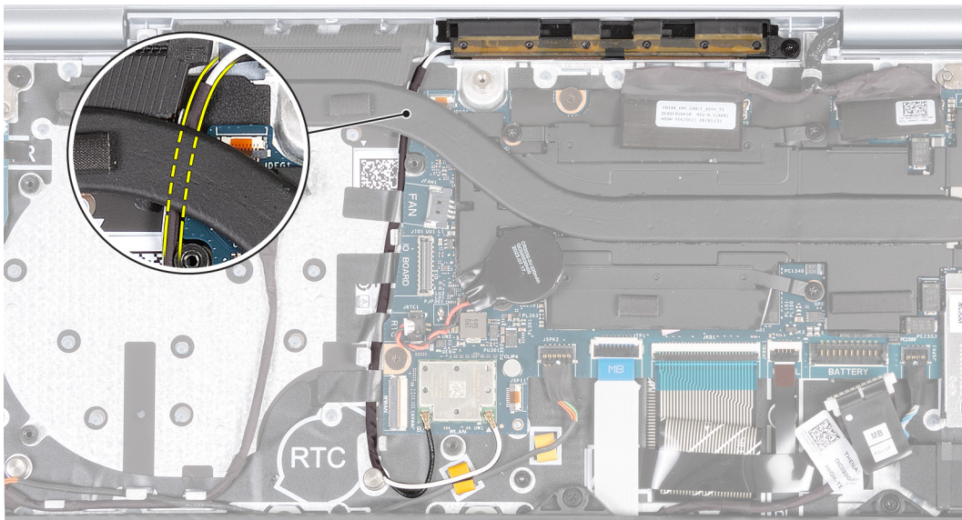
Afbeelding 68. WLAN-antennekabels verwijderen
