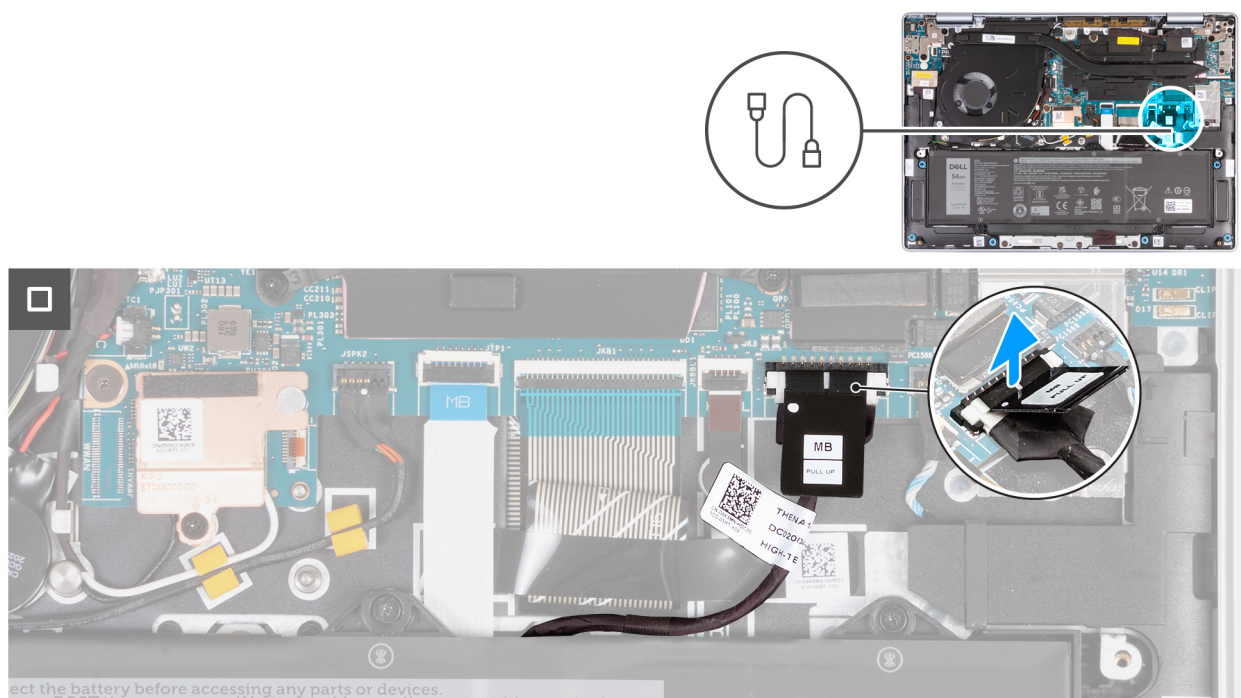
Afbeelding 17. De batterijkabel loskoppelen
