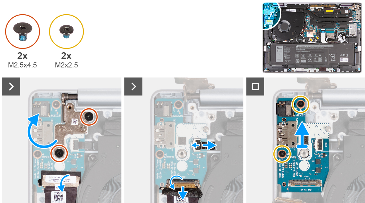
Afbeelding 82. De I/O-kaart verwijderen (voor computers die worden geleverd met alleen WLAN-ondersteuning)
