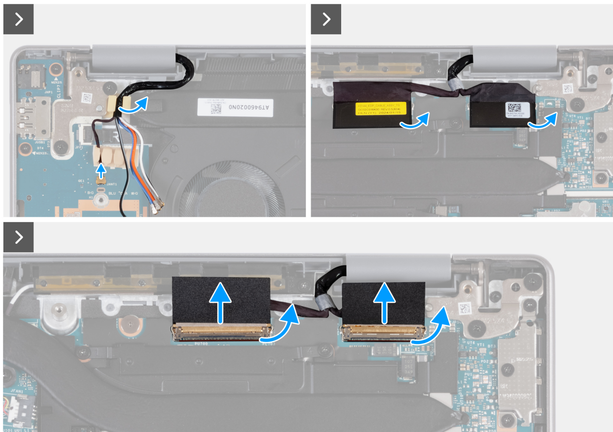
Afbeelding 77. De beeldschermeenheid verwijderen (voor computers die worden geleverd met WWAN-ondersteuning)
