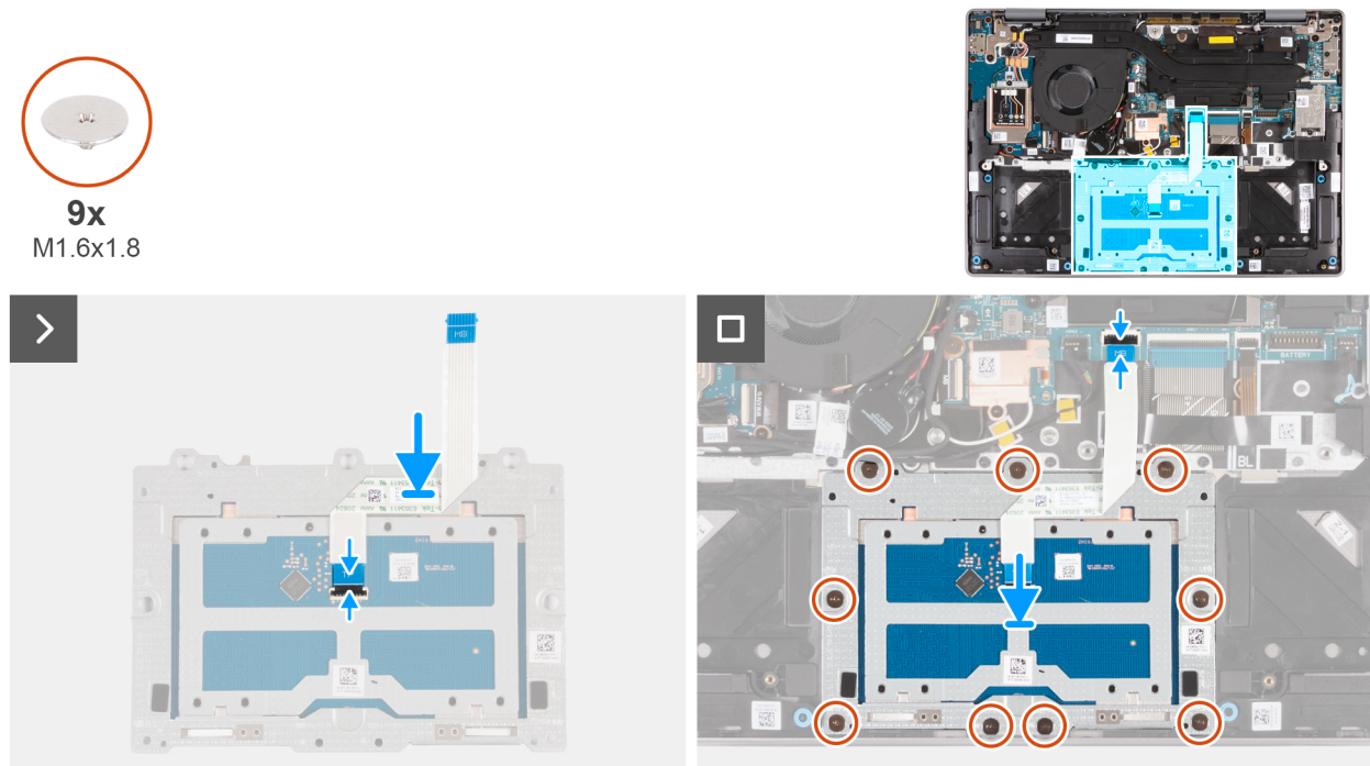
Afbeelding 87. De touchpadeenheid plaatsen
