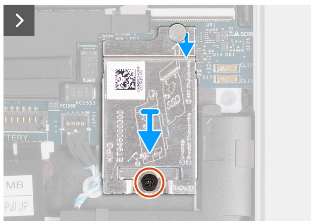
Afbeelding 21. De SSD verwijderen
