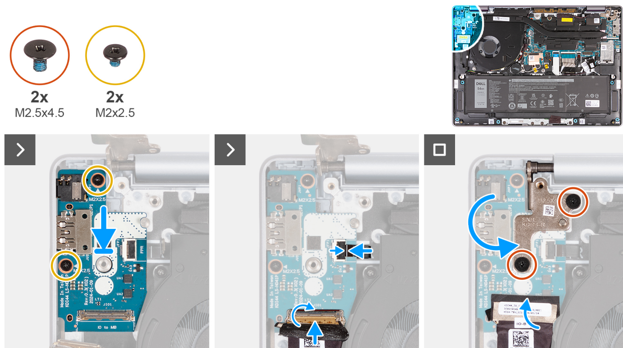
Afbeelding 83. De I/O-kaart plaatsen (voor computers die worden geleverd met alleen WLAN-ondersteuning)
