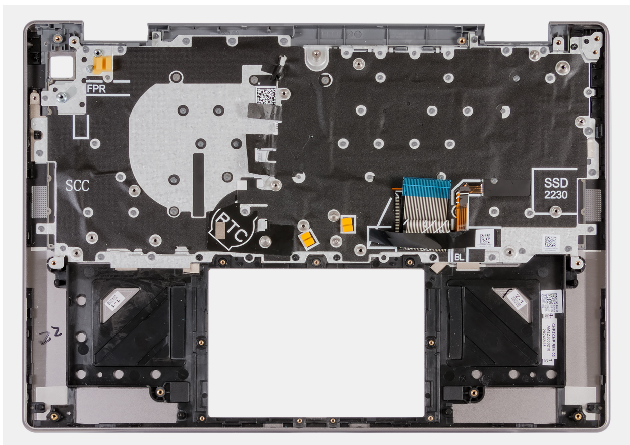
Afbeelding 100. Palmsteun- en toetsenbordeenheid
