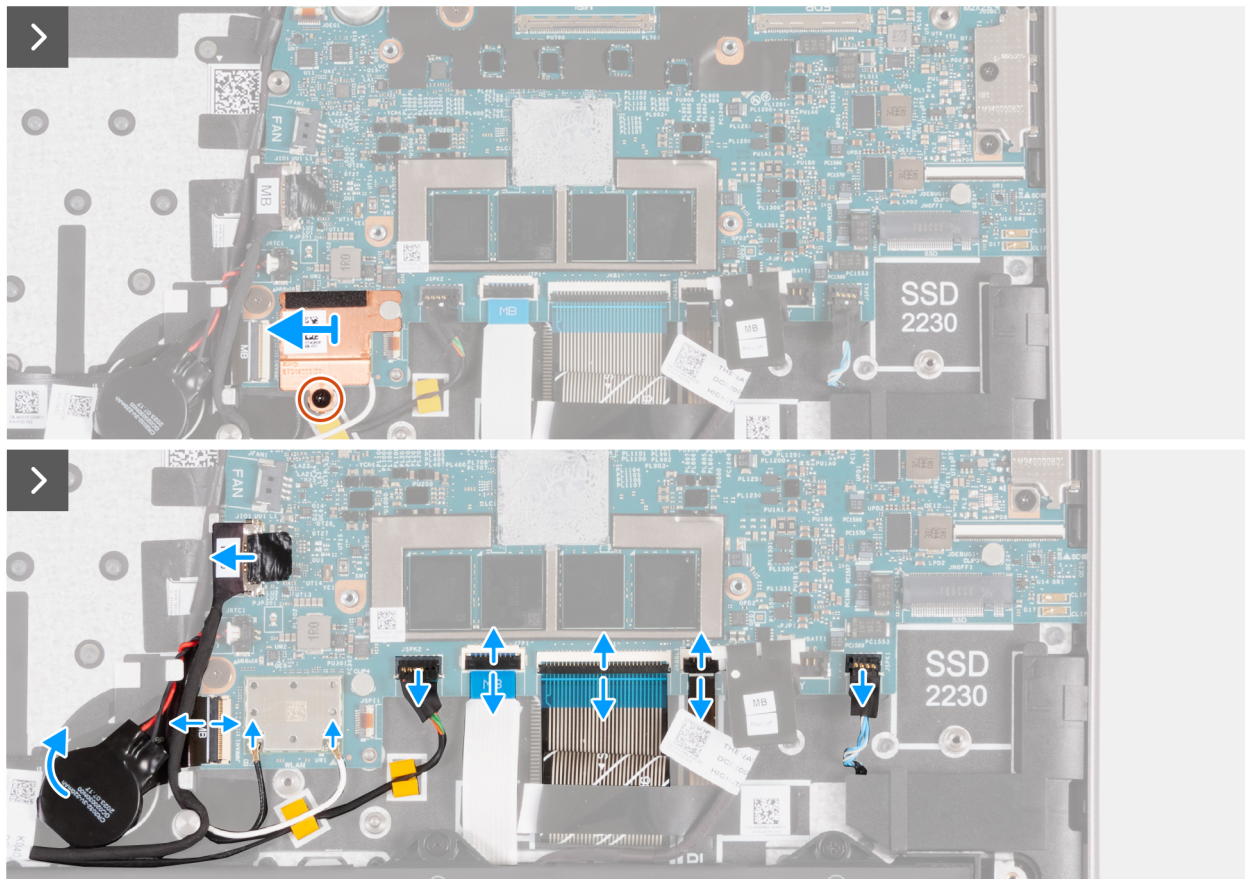
Afbeelding 94. De systeemkaart verwijderen
