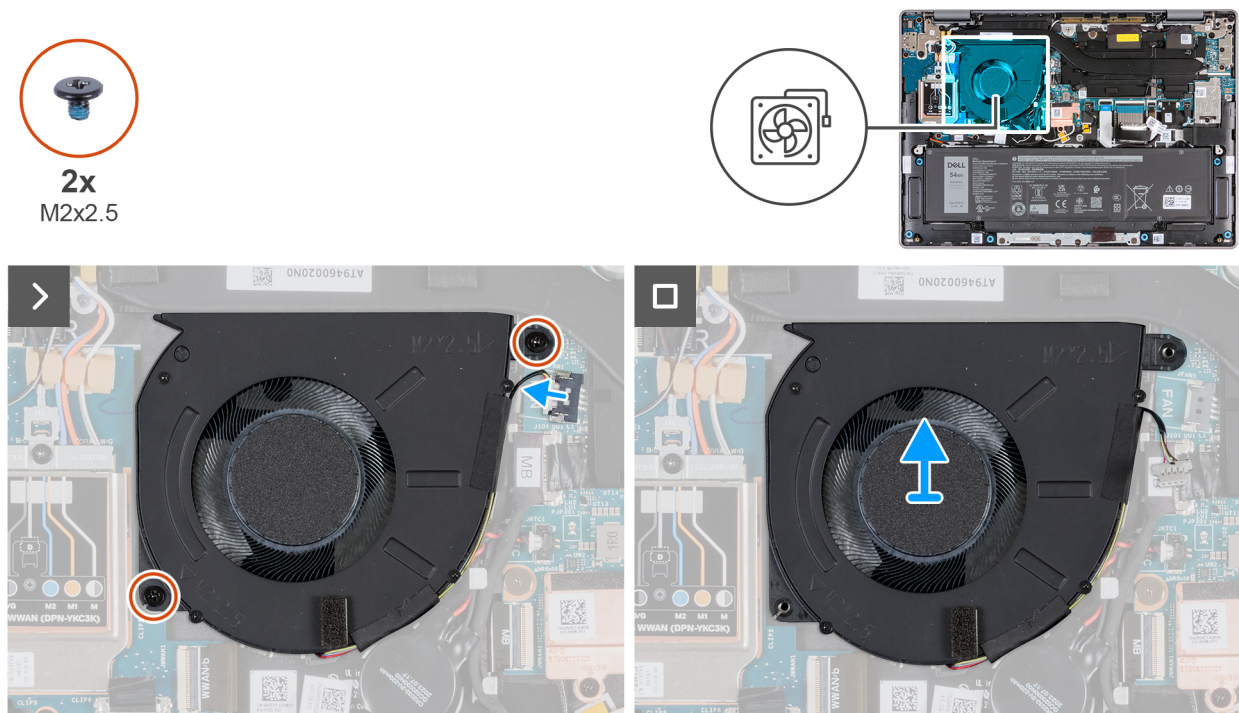
Afbeelding 37. De ventilator verwijderen (voor computers die worden geleverd met WWAN-ondersteuning)
