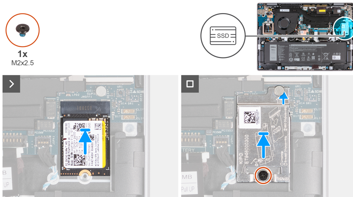
Afbeelding 23. De SSD plaatsen
