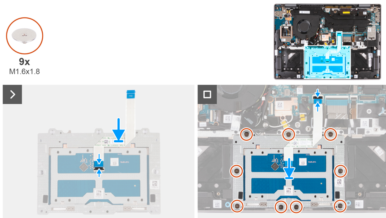
Figure 87. Installation de l'assemblage du pavé tactile
