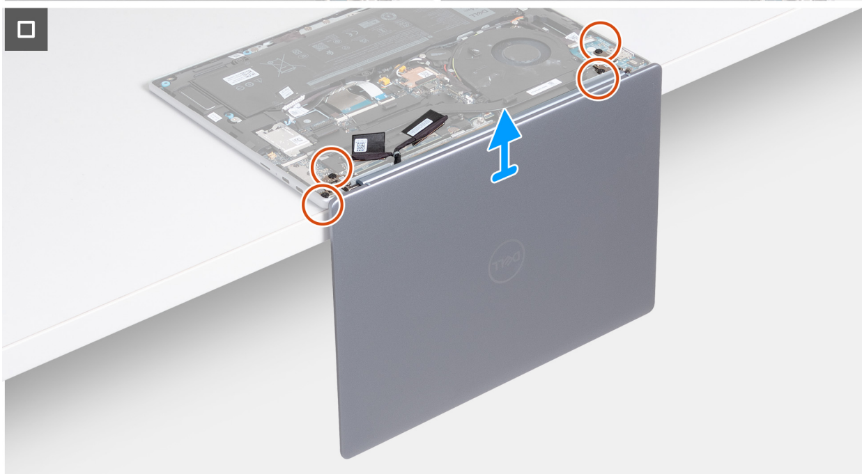
Figure 74. Retrait de l'assemblage d'écran (pour les ordinateurs expédiés avec une prise en charge WLAN uniquement)
