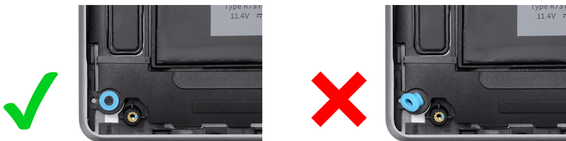
Figure 34. Installation des passe-câbles en caoutchouc
