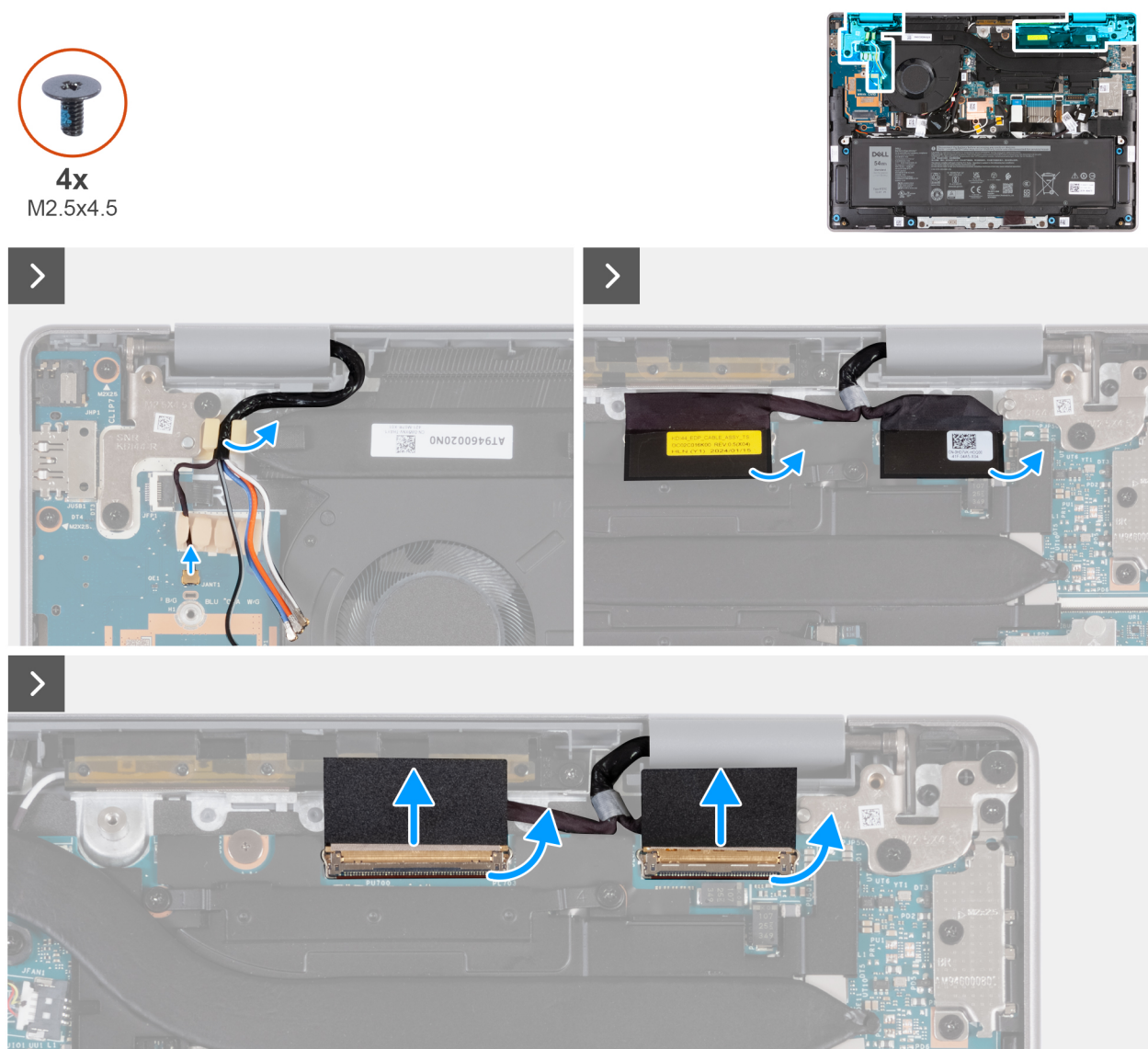
Figure 77. Retrait de l'assemblage d'écran (pour les ordinateurs expédiés avec une prise en charge WWAN)
