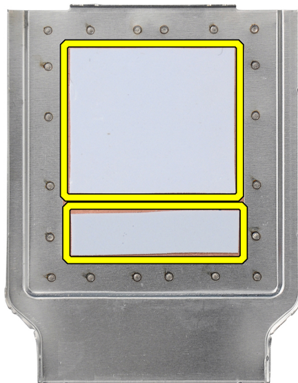
Figure 27. Tampons thermiques sur la partie inférieure de la protection thermique WWAN
