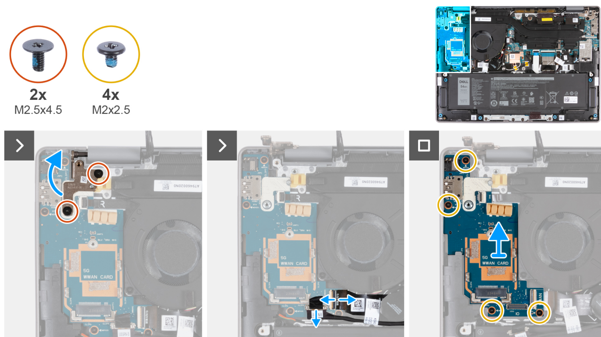
Figure 84. Retrait de la carte d'E/S (pour les ordinateurs expédiés avec une prise en charge WWAN)
