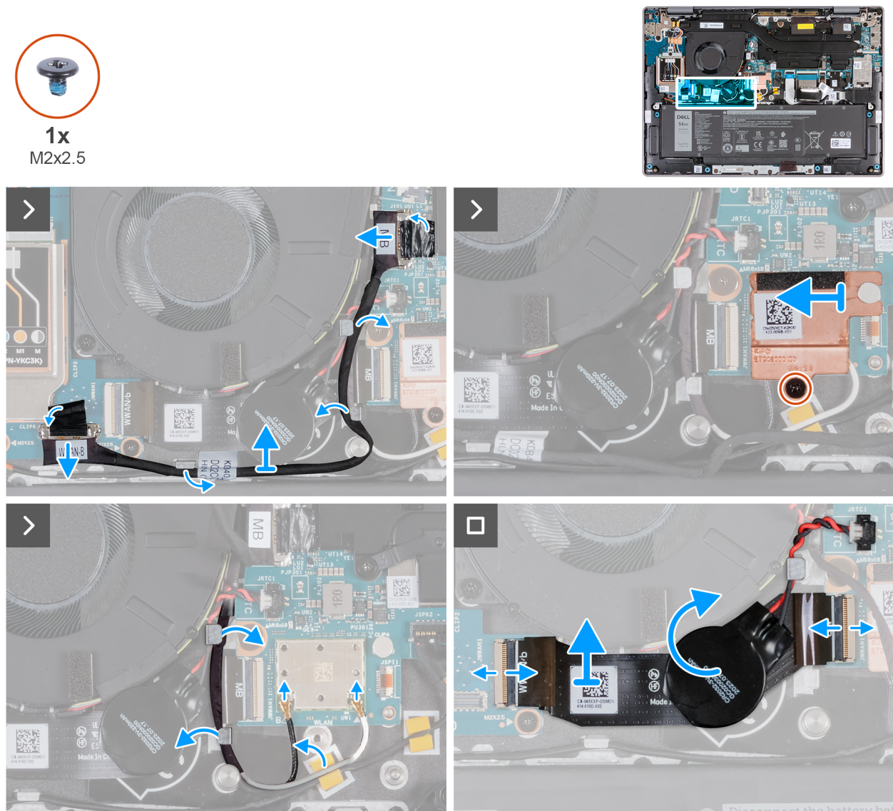
Figure 56. Retrait du câble FPC de la carte d'E/S
