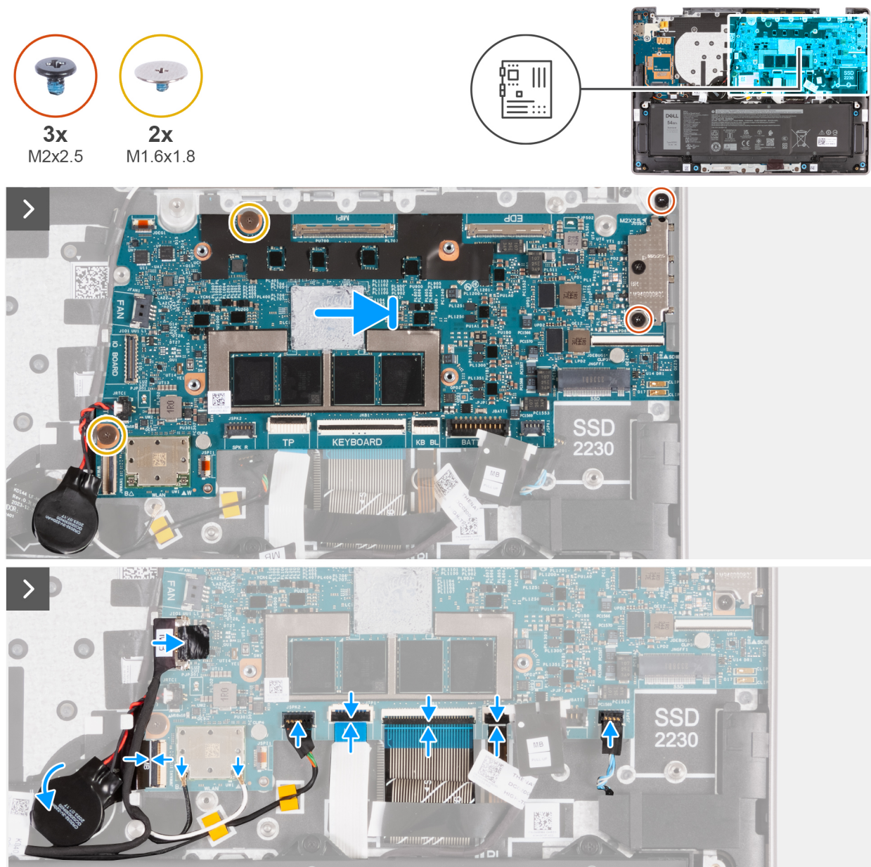
Figure 98. Installation de la carte système
