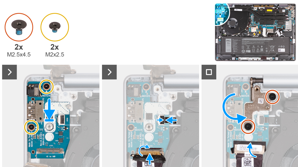
Figure 83. Installation de la carte d'E/S (pour les ordinateurs expédiés avec une prise en charge WLAN uniquement)
