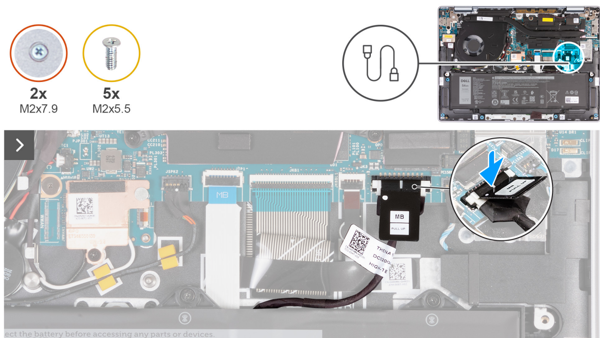
Figure 18. Connexion du câble de la batterie
