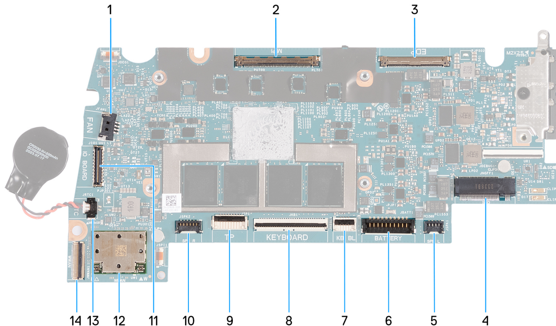
Figure 97. Connecteurs de la carte système
