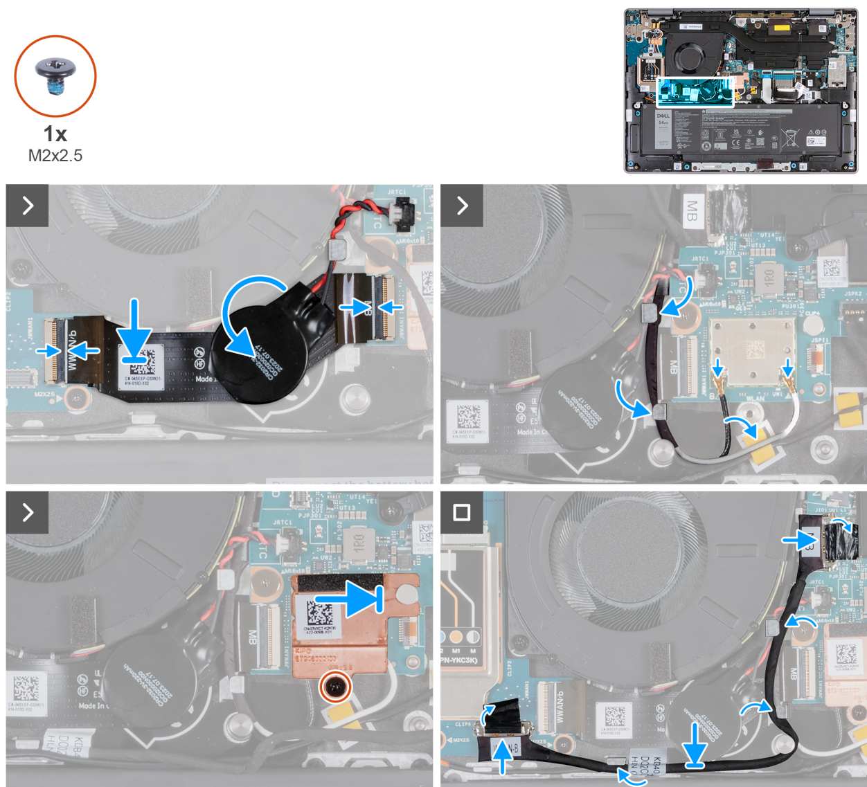
Figure 57. Installation du câble FPC de la carte des E/S
