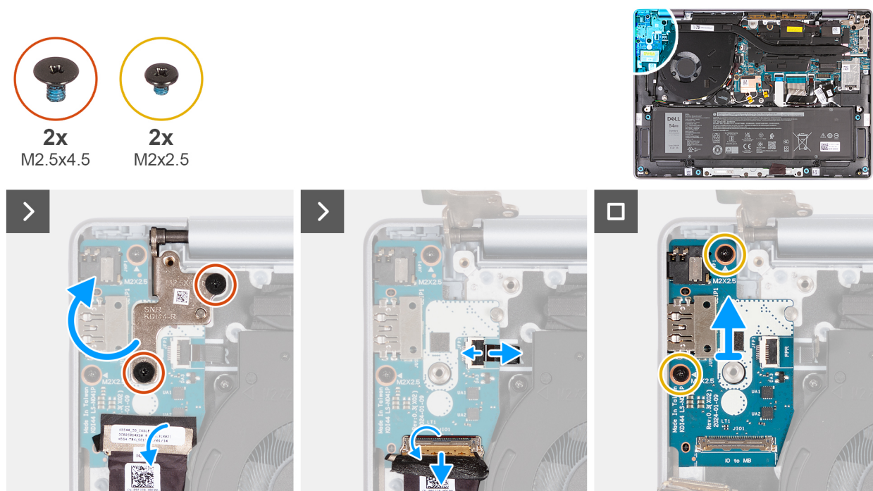
Figure 82. Retrait de la carte d'E/S (pour les ordinateurs expédiés avec une prise en charge WLAN uniquement)
