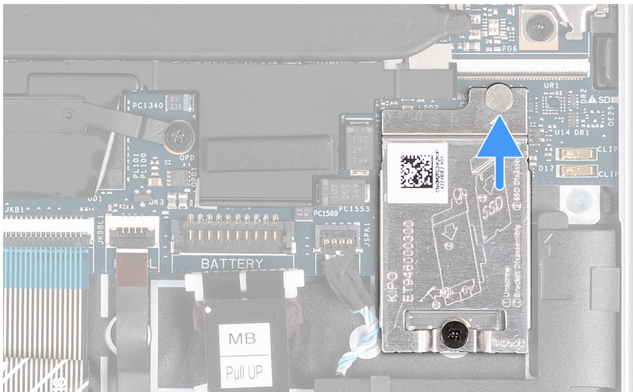
Figure 24. Installation de la protection thermique SSD
