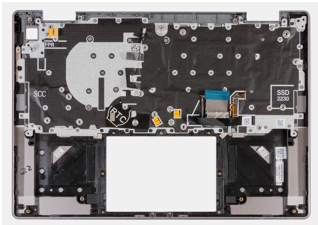
Figure 101. Assemblage du repose-poignets et du clavier
