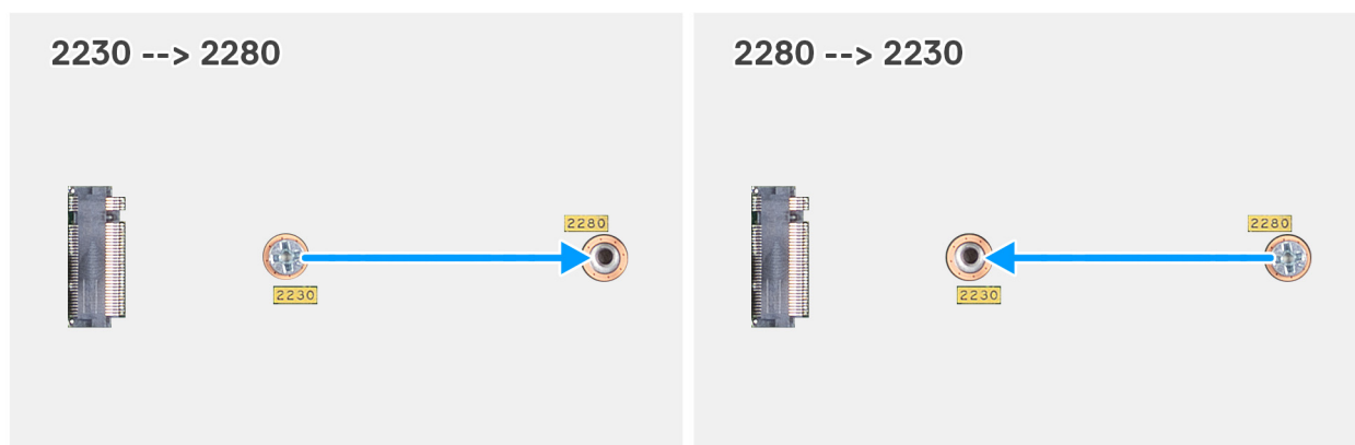
Afbeelding 27. De schroefbevestiging verplaatsen ter ondersteuning van een andere vormfactor (OptiPlex Micro 7020)
