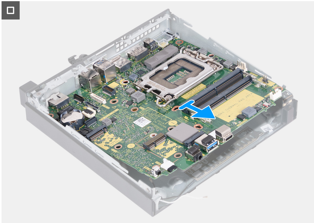
Afbeelding 46. De systeemkaart verwijderen
