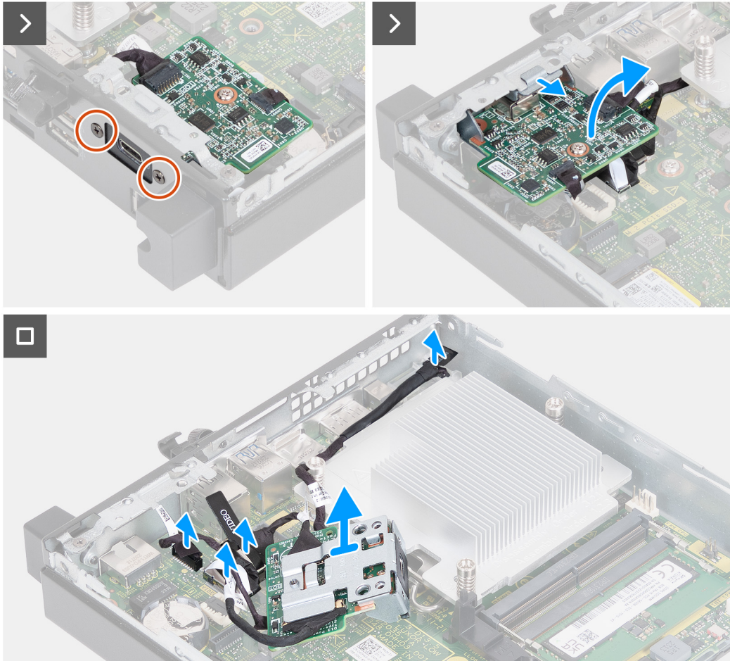
Afbeelding 38. De optionele Type-C-module verwijderen
