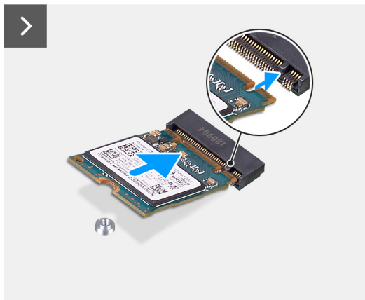
Afbeelding 24. De M.2 2230 SSD in slot 1 installeren
