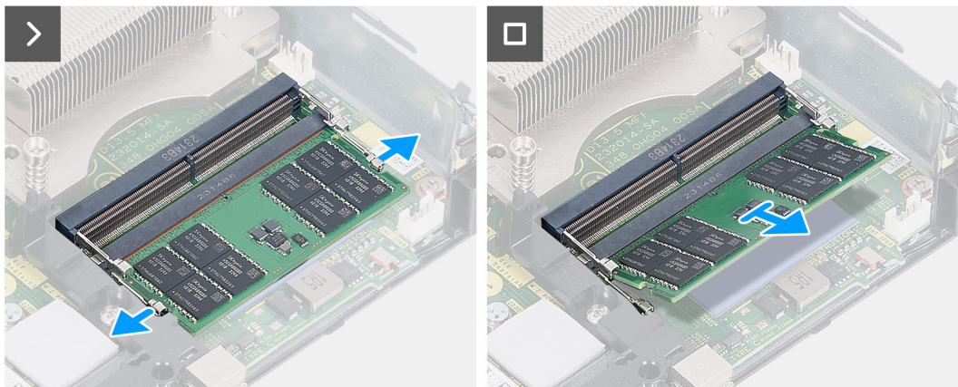
Afbeelding 32. De geheugenmodule verwijderen
