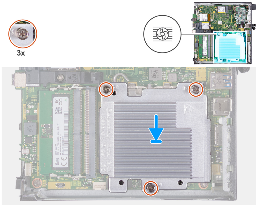
Afbeelding 41. De koelplaat plaatsen
