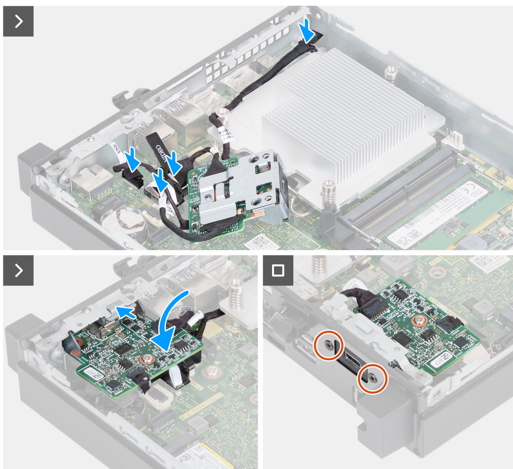
Afbeelding 39. De optionele Type-C-module installeren
