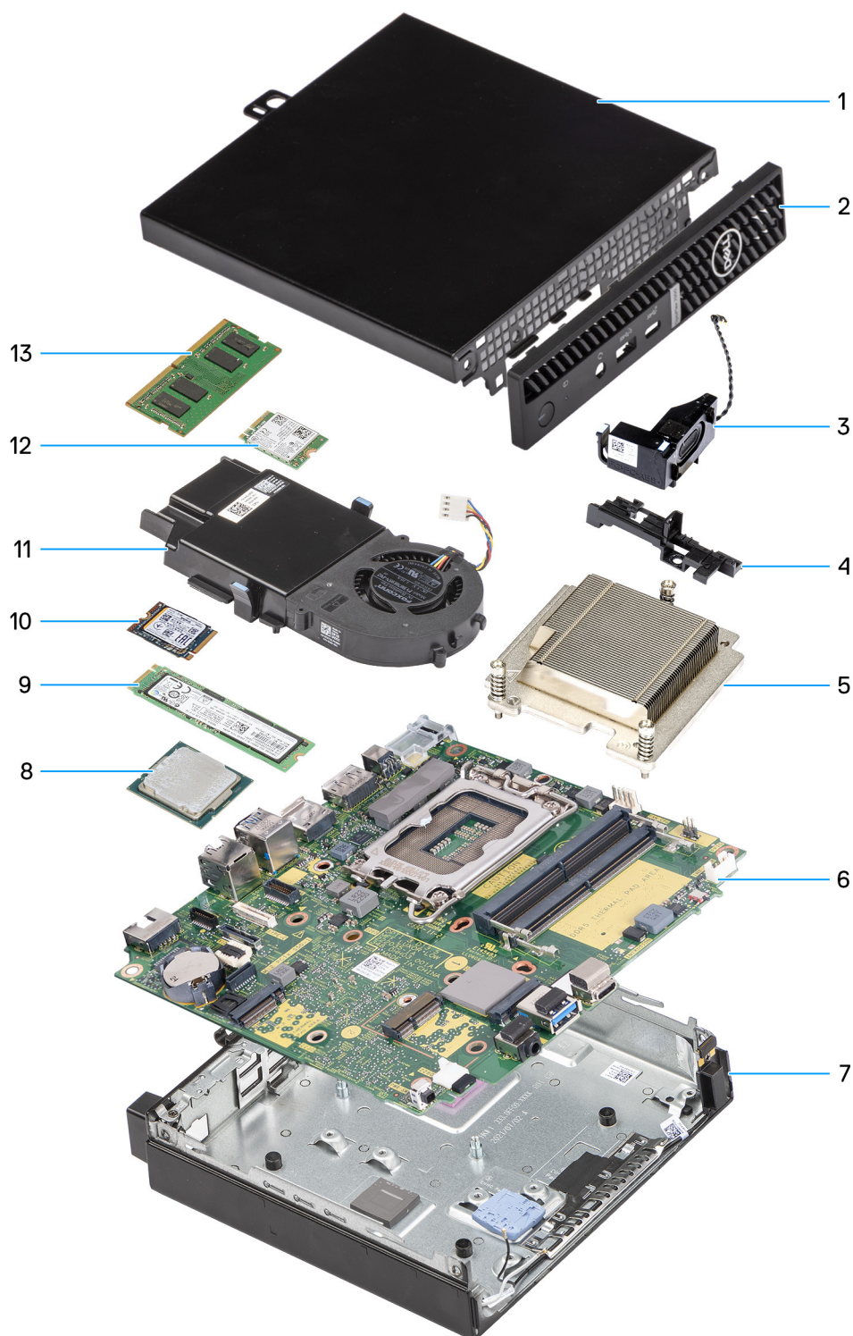
Afbeelding 8. Belangrijke onderdelen van de OptiPlex Micro 7020
