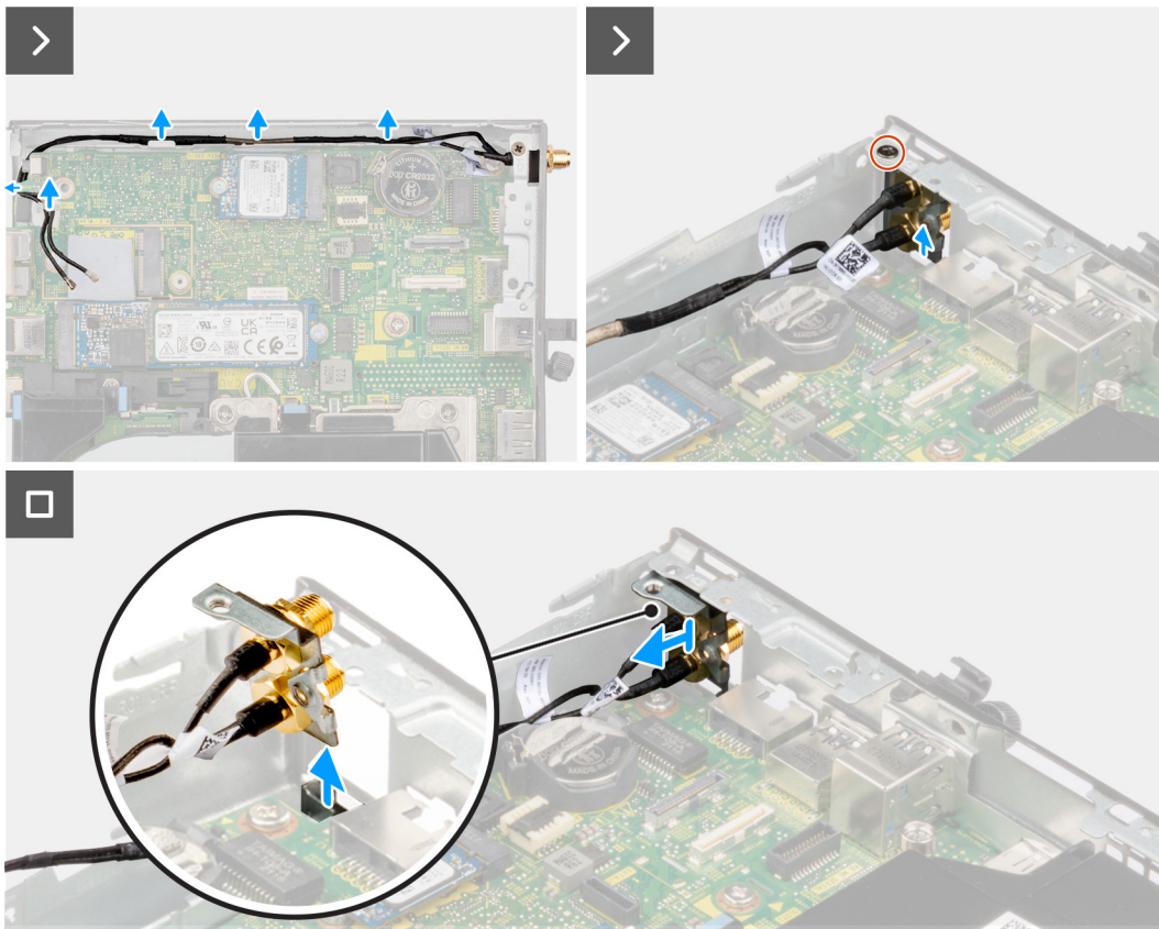
Afbeelding 54. De SMA-antenne verwijderen (locatie 3)
