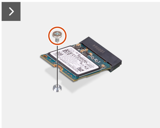
Afbeelding 23. De M.2 2230 SSD uit slot 1 verwijderen
