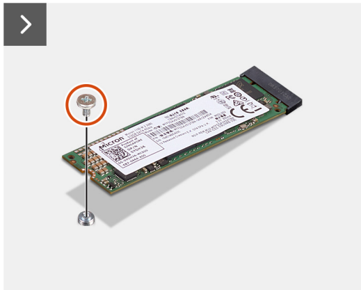
Afbeelding 21. De M.2 2280 SSD uit slot 0 verwijderen
