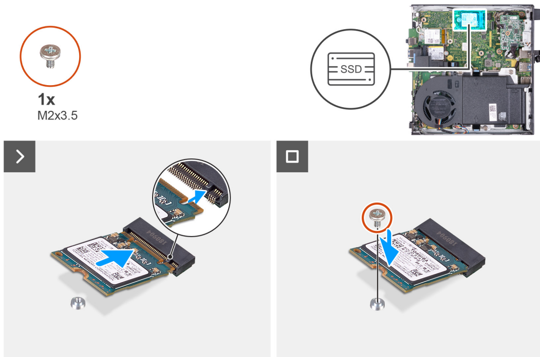
Abbildung 24. Installieren des M.2 2230-Solid-State-Laufwerks in Steckplatz 1
