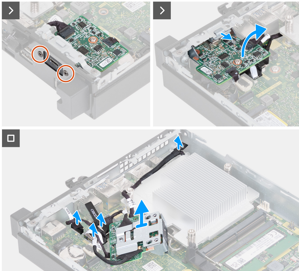
Abbildung 38. Entfernen des optionalen Typ-C-Moduls
