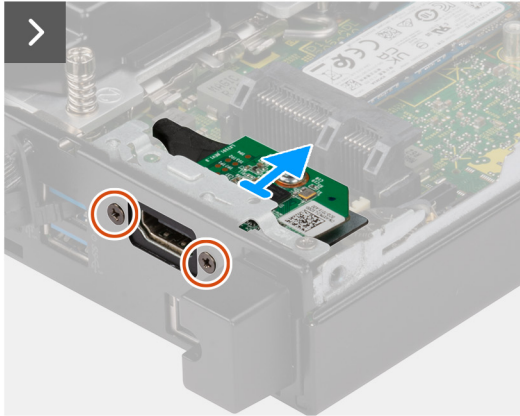
Abbildung 34. Entfernen des optionalen E/A-Moduls (HDMI, DP oder PS2)
