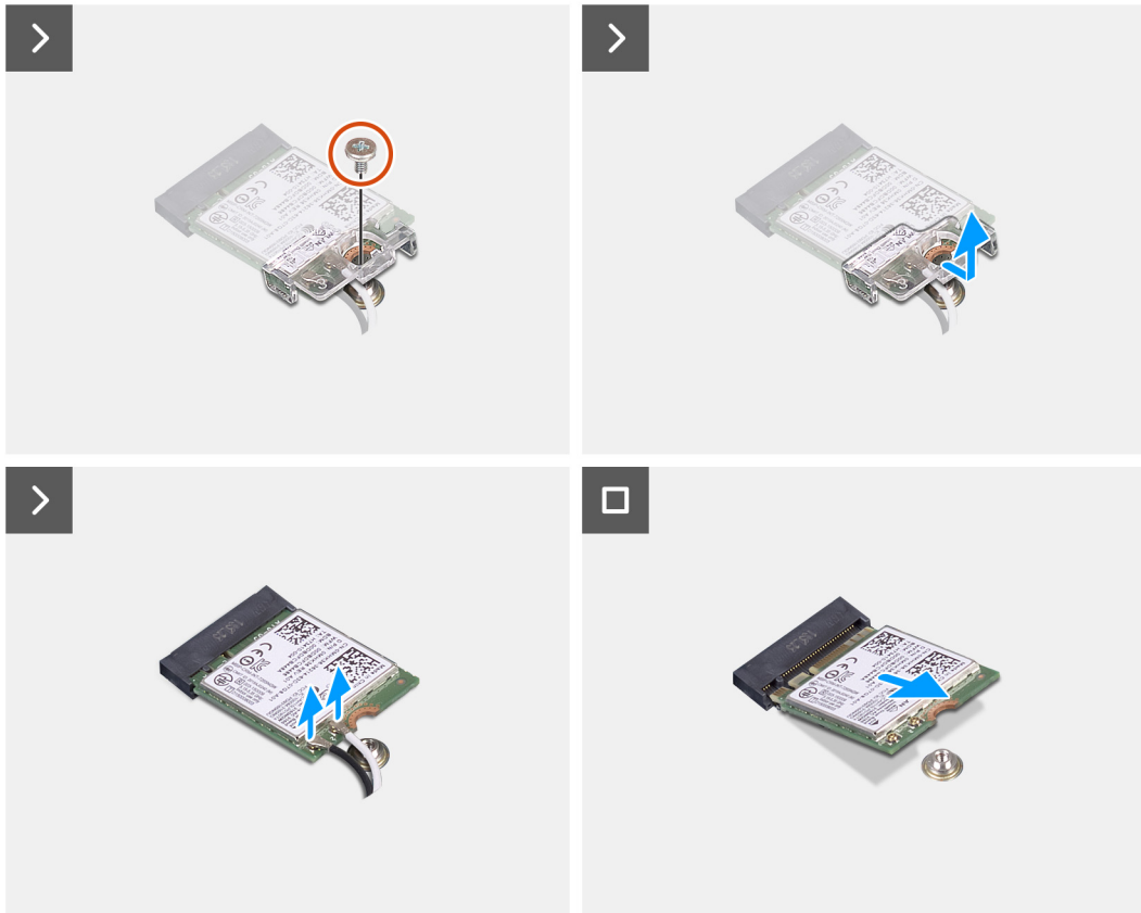
Abbildung 28. Entfernen der Wireless-Karte
