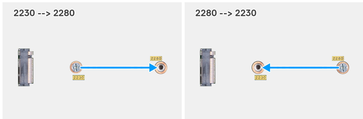
Abbildung 27. Verschieben der Schraubbefestigung zur Unterstützung eines anderen Formfaktors (OptiPlex Micro 7020)
