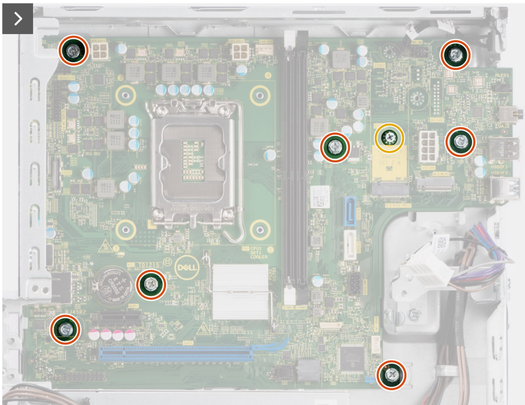
Figure 63. Installation de la carte système
