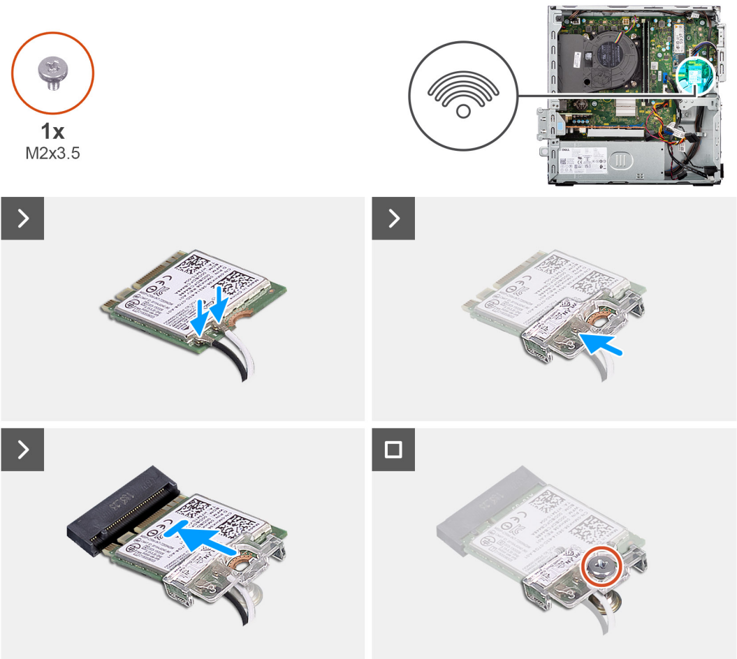
Figure 28. Installation de la carte sans fil
