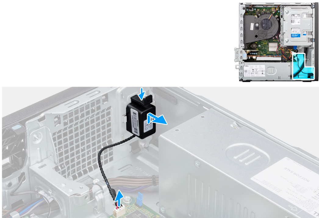
Figure 31. Retrait du haut-parleur
