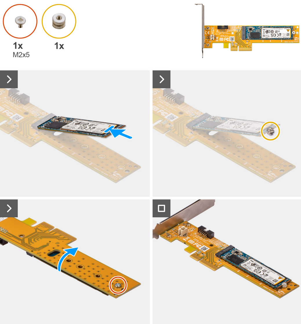
Figure 25. Installation du disque SSD M.2 2280 sur la carte Dell Ultra Speed Drive Gen 3
