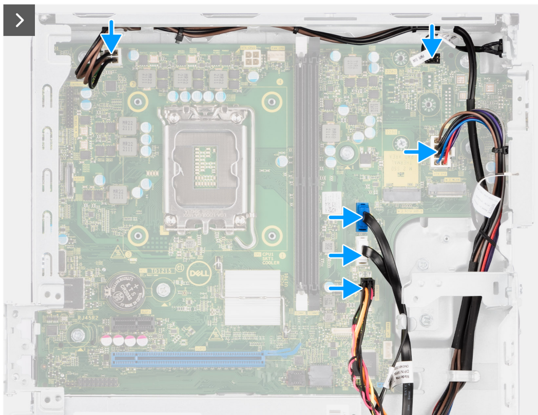
Figure 64. Installation de la carte système
