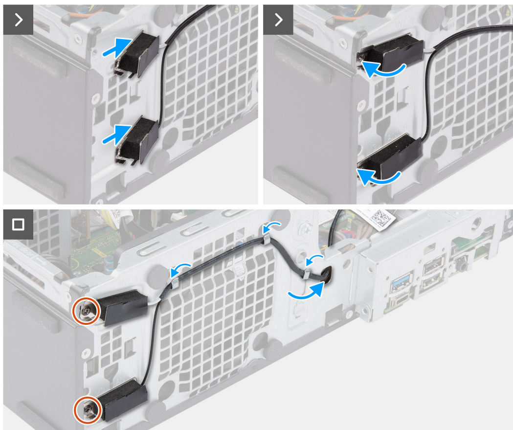
Figure 39. Installation du module d'antenne interne
