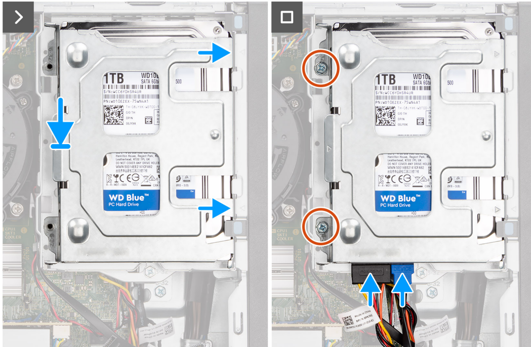
Figure 10. Installation du disque dur de 3,5 pouces
