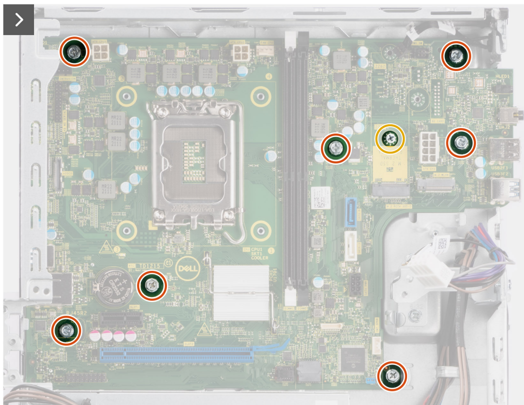
Figure 59. Retrait de la carte système
