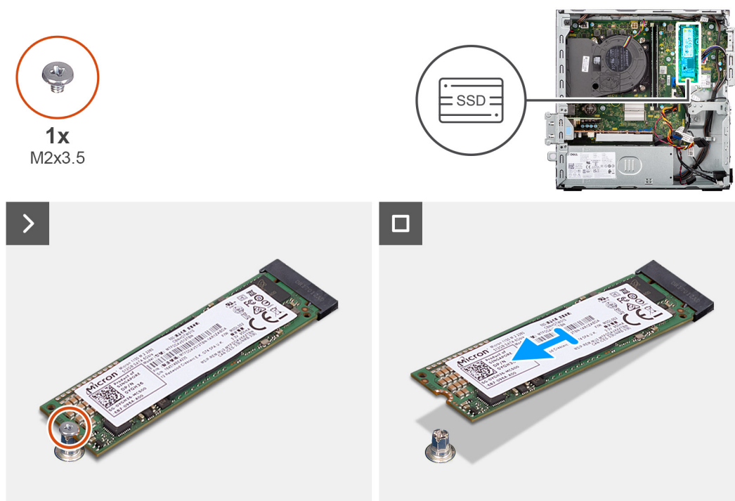
Figure 19. Retrait du disque SSD M.2 2280
