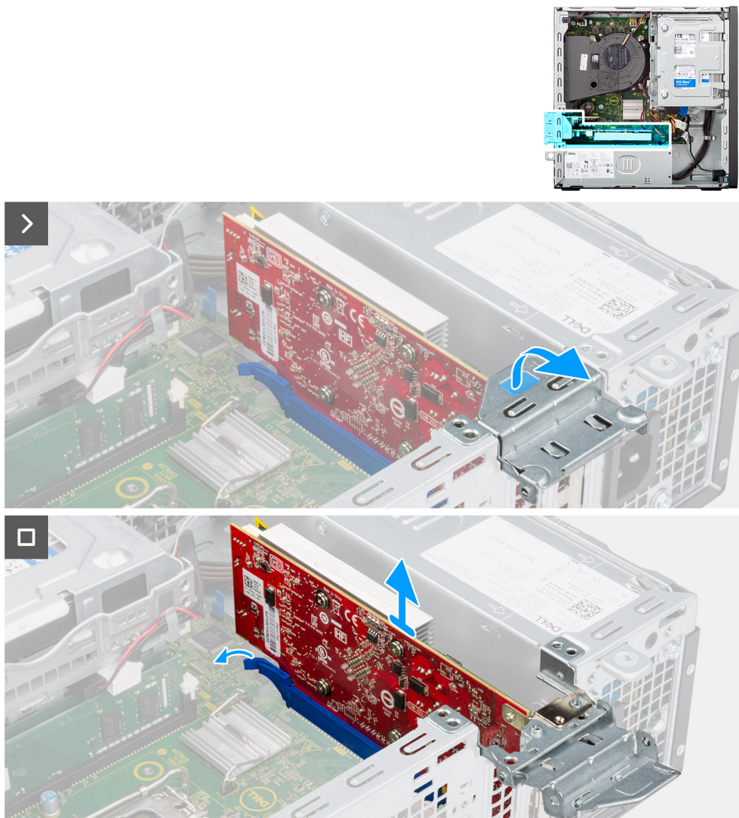
Figure 29. Retrait de la carte graphique
