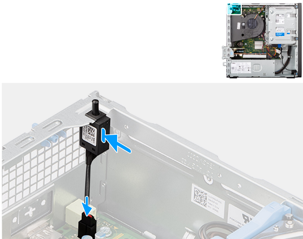
Figure 34. Installation du commutateur d'intrusion
