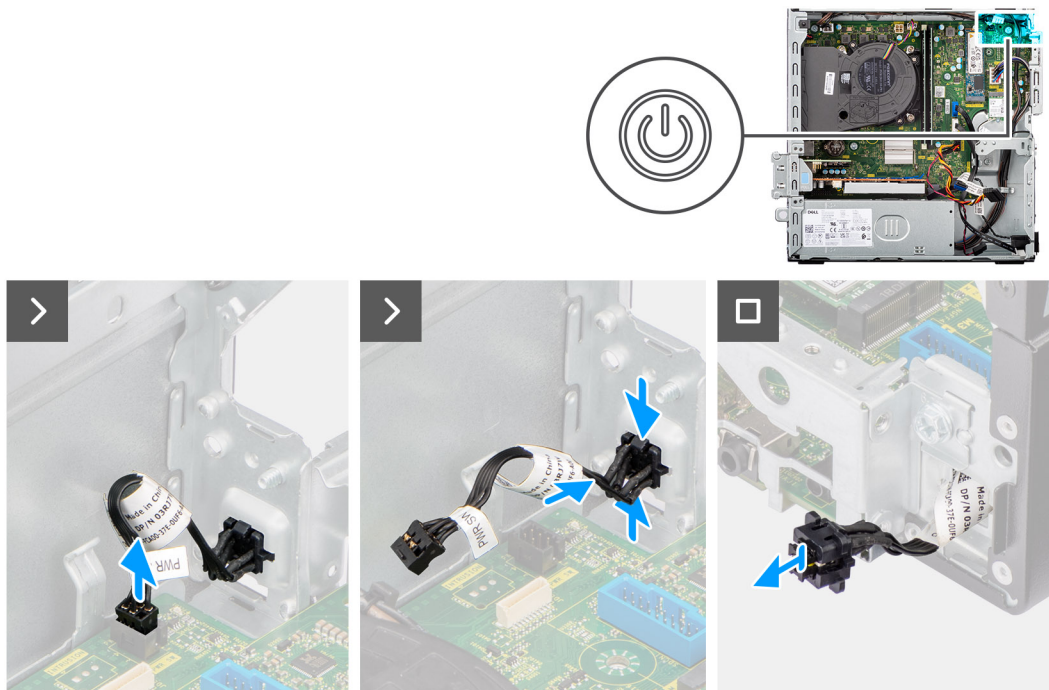
Figure 35. Retrait du bouton d'alimentation
