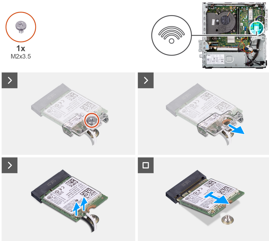
Figure 27. Retrait de la carte sans fil
