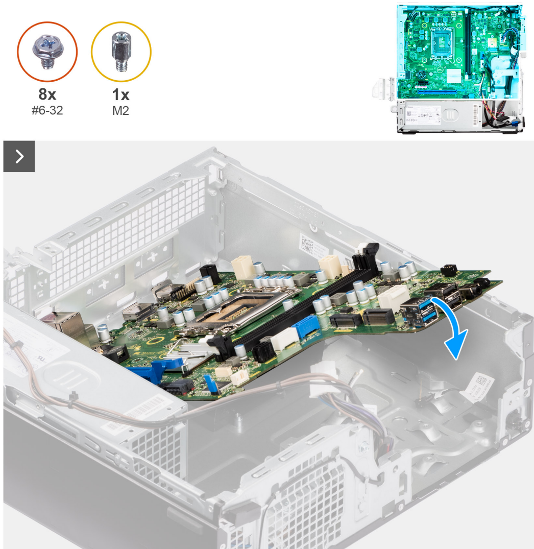
Figure 62. Installation de la carte système
