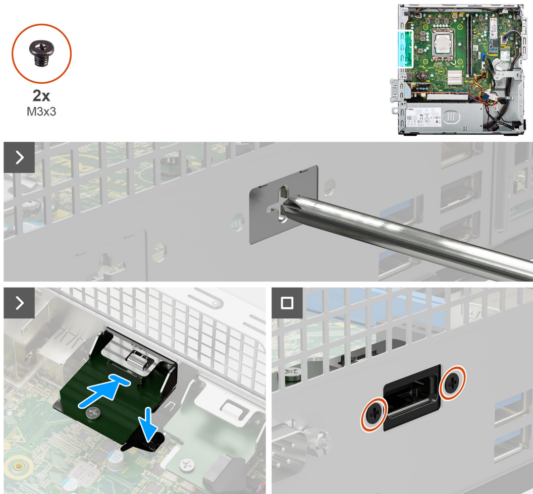
Figure 53. Installation du module DisplayPort
