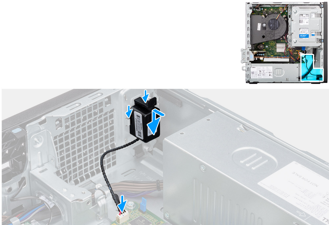
Figure 32. Installation du haut-parleur
