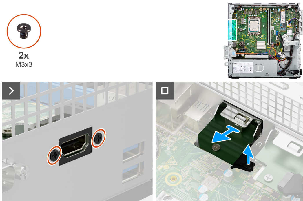
Figure 54. Retrait du module HDMI
