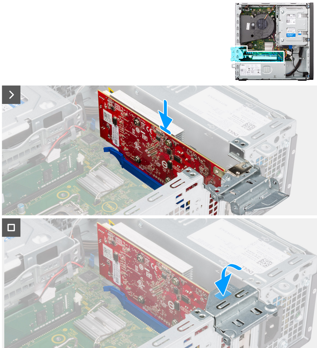
Figure 30. Installation de la carte graphique
