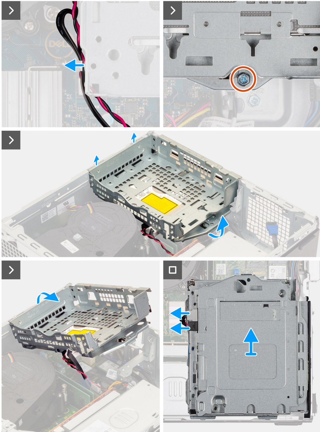
Abbildung 11. Entfernen des Festplattengehäuses
