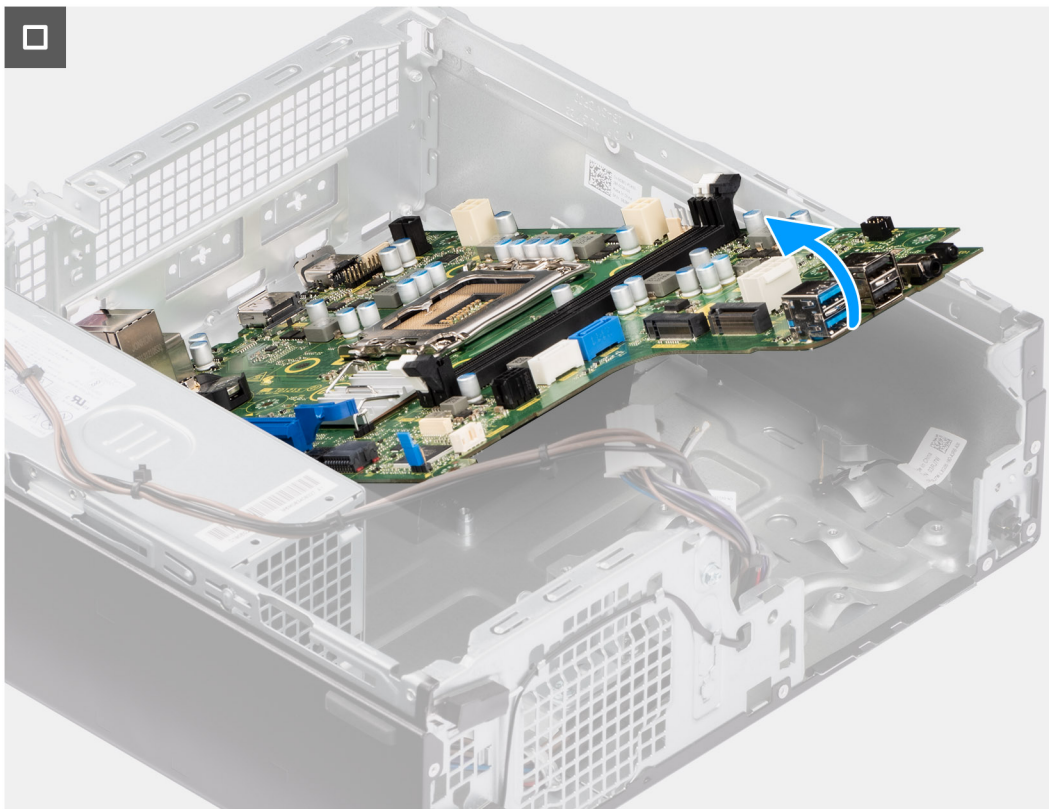
Abbildung 60. Entfernen der Systemplatine
