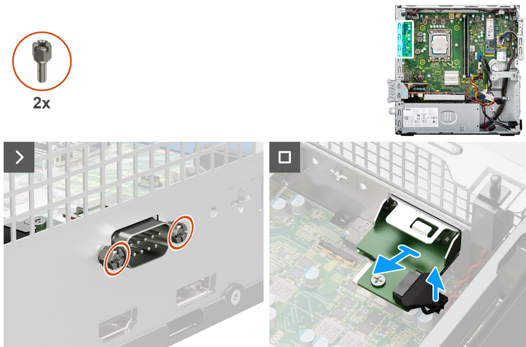
Abbildung 48. Entfernen des seriellen Moduls
