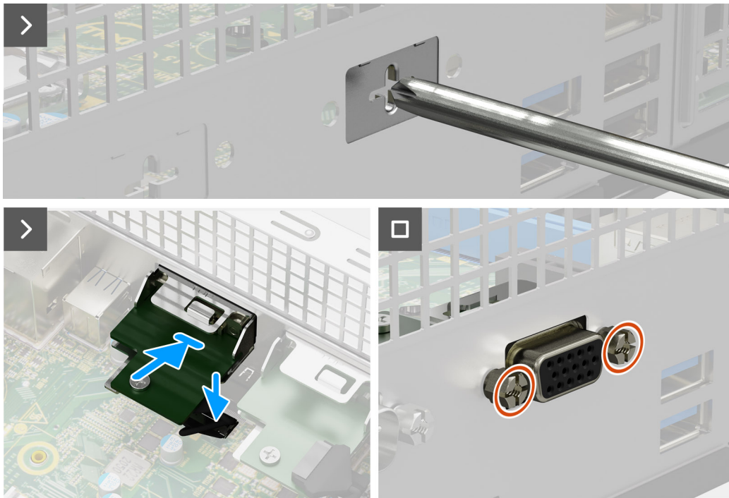
Abbildung 51. Installieren des VGA-Moduls
