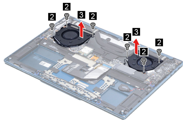
Figure 20. Remove the fan
