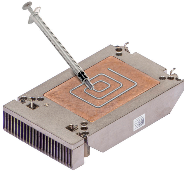
Ilustración 52. Aplicación de la grasa térmica
