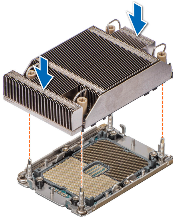
Ilustración 55. Instalación del procesador y del disipador de calor (PHM)
