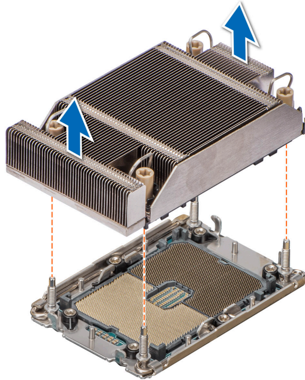
Ilustración 46. Extracción de un módulo del disipador de calor y procesador
