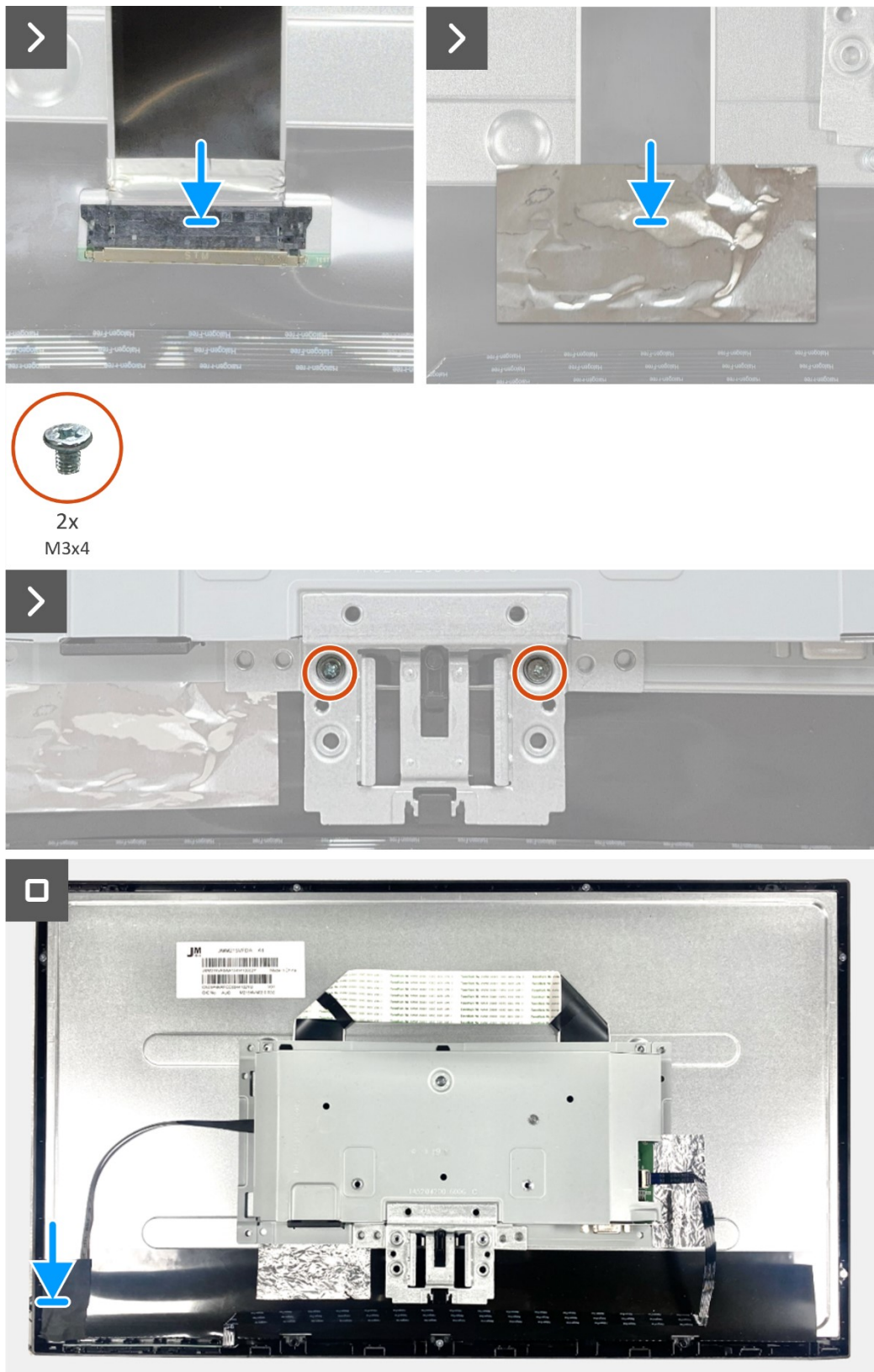
Figura 18. Instalar el conjunto del chasis
