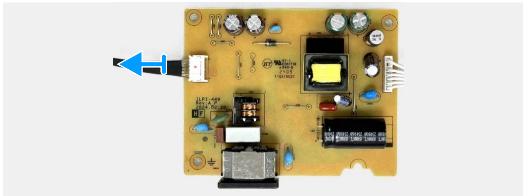
Figura 24. Retire la placa de alimentación
