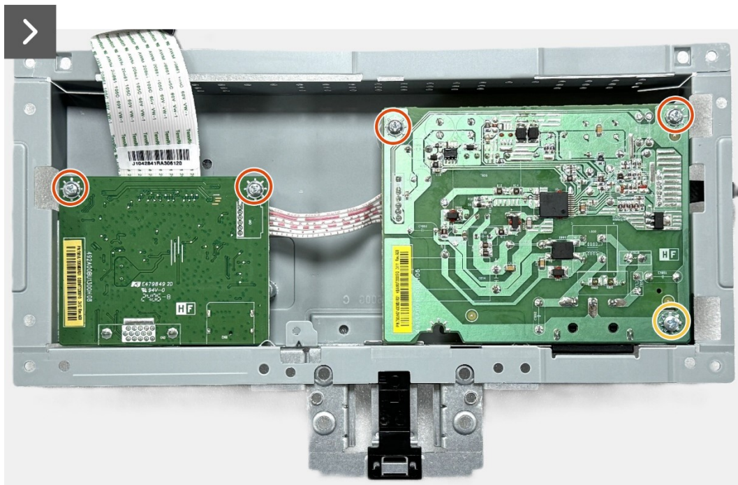
Figura 20. Retire la placa de la interfaz
