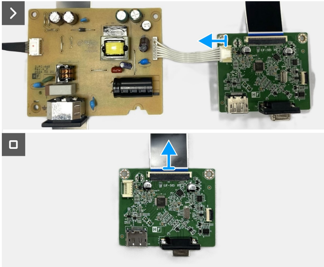
Figura 21. Retire la placa de la interfaz
