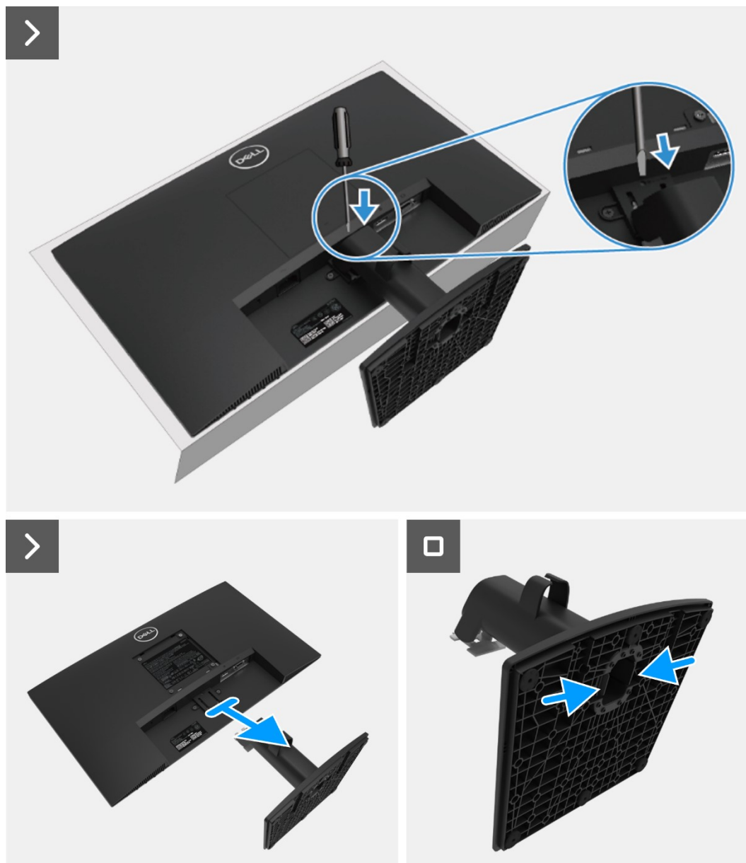
Figura 8. Quitar el pedestal
