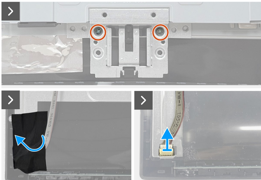
Figura 16. Retirar el conjunto del chasis
