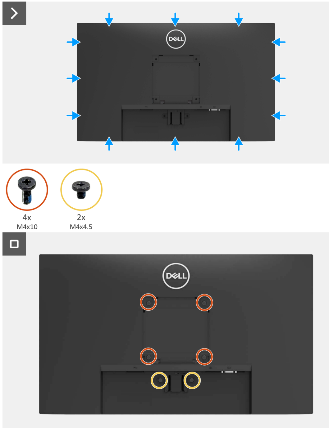
Figura 13. Instalar la cubierta posterior
