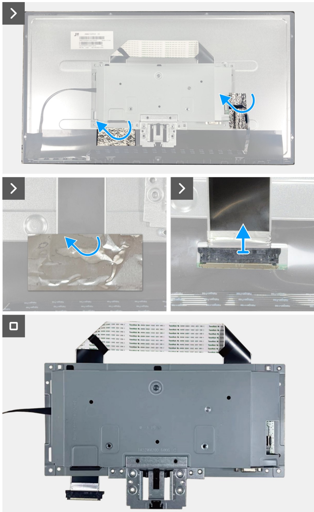
Figura 17. Retirar el conjunto del chasis
