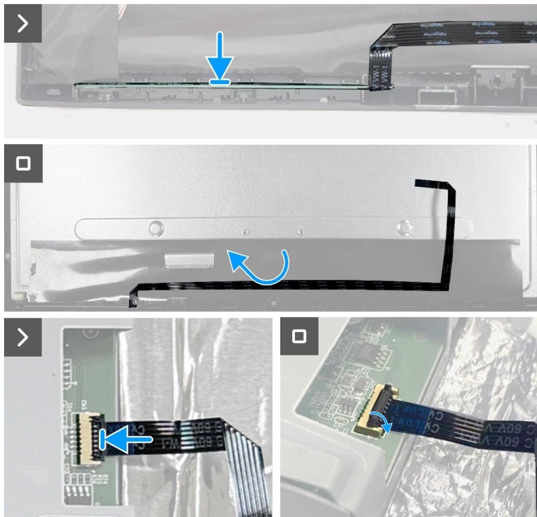
Figura 15. Instalar la placa del teclado
