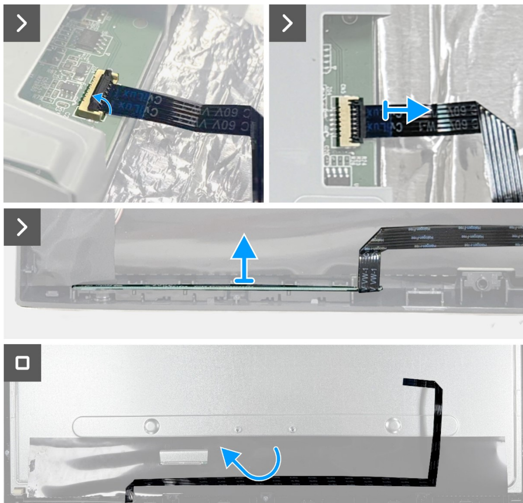
Figura 14. Retire la placa del teclado
