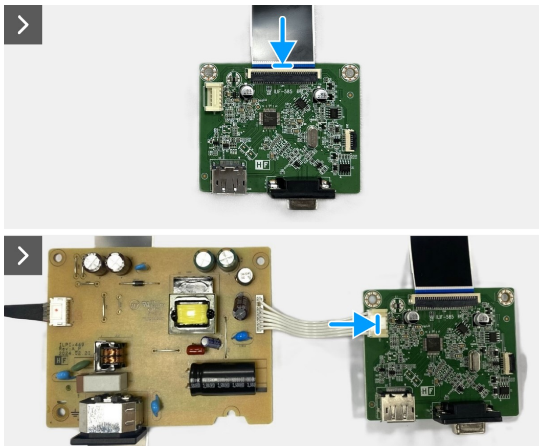
Figura 22. Instalar la placa de la interfaz
