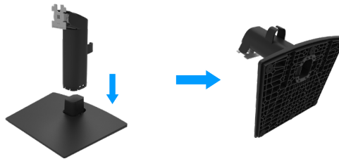
Figura 12. Montar el pedestal
