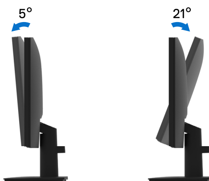
Figura 23. Regolazione dell'inclinazione
