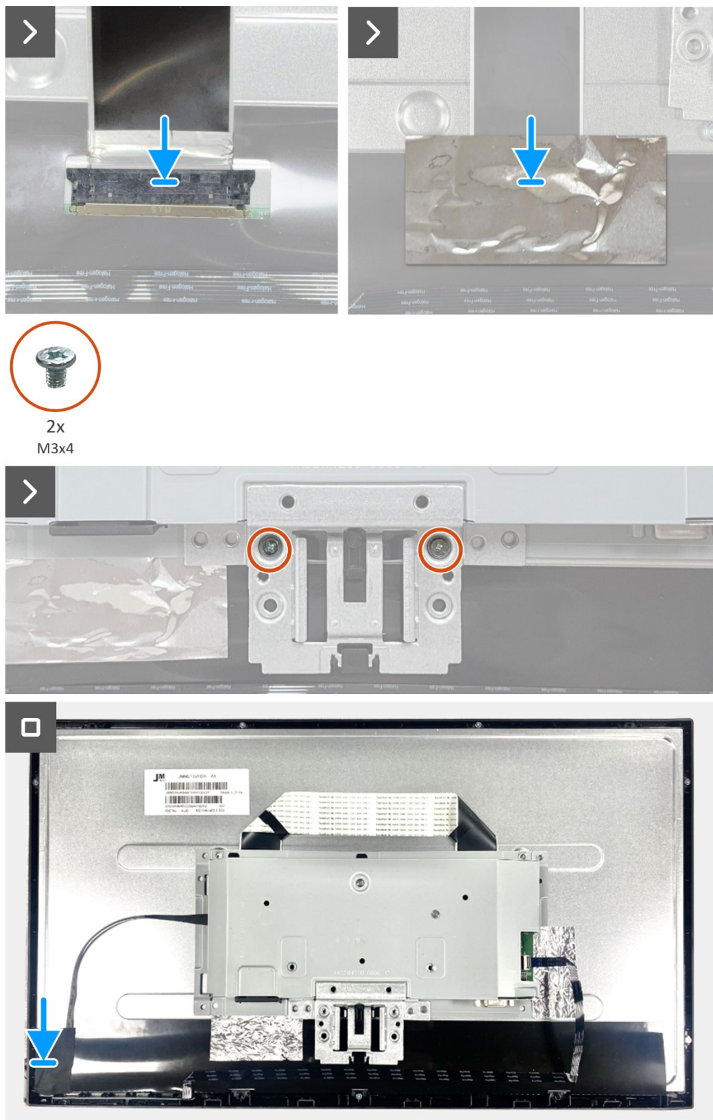
Obrázek 18. Montáž sestavy skříně
