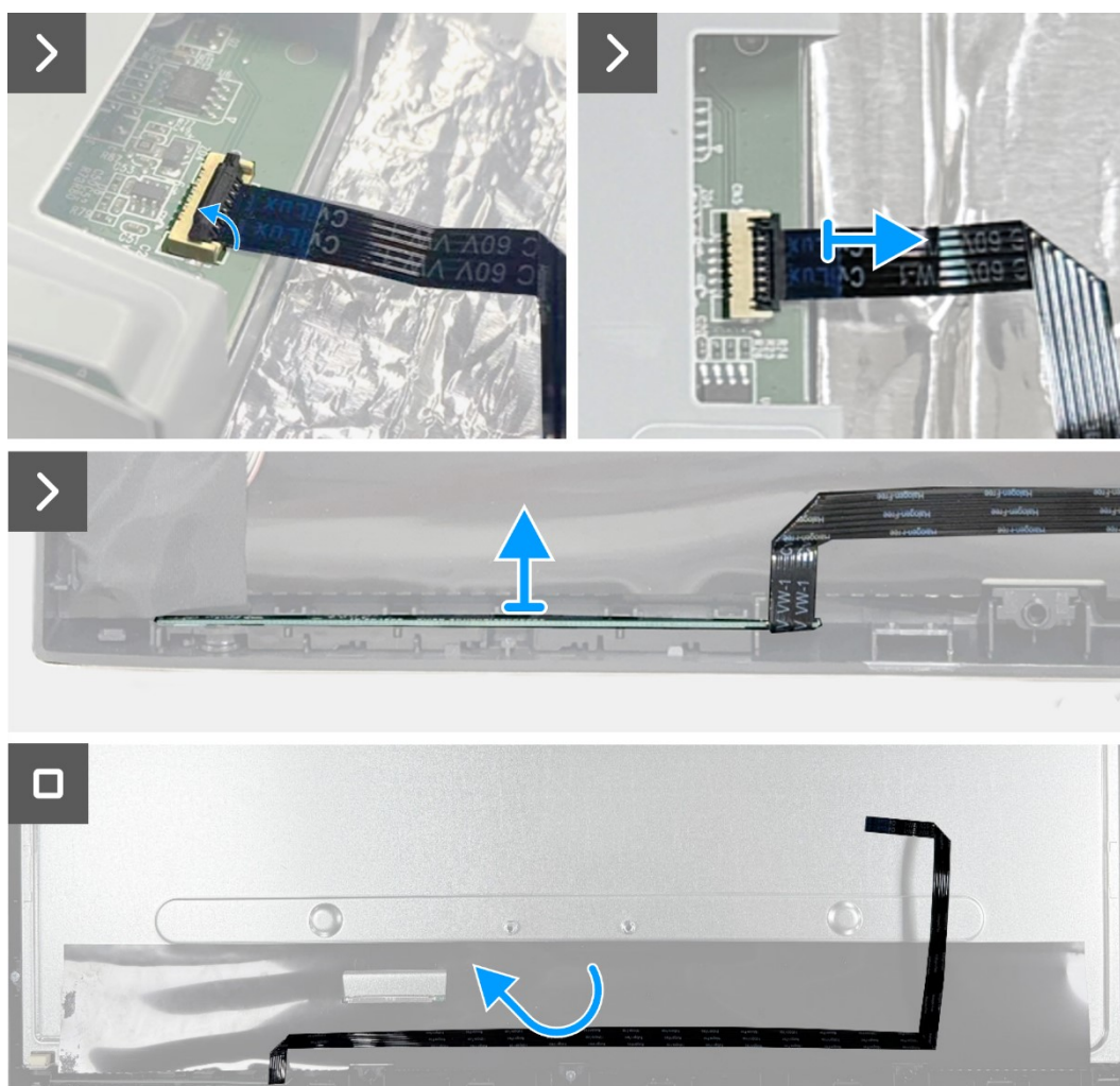
Obrázek 14. Demontáž klávesnice
