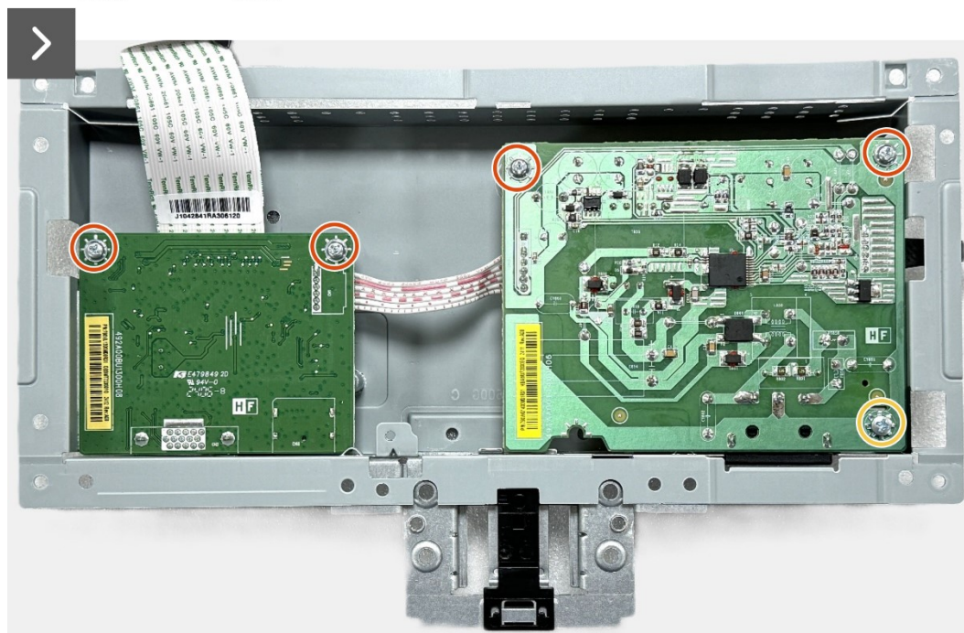
Obrázek 20. Demontáž desky rozhraní
