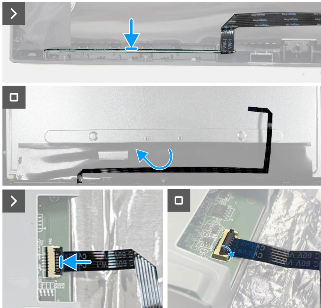
Obrázek 15. Montáž klávesnice
