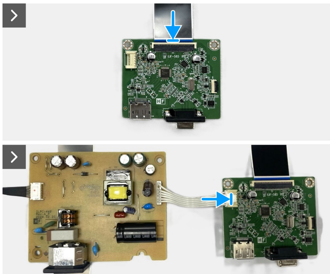
Obrázek 22. Montáž desky rozhraní
