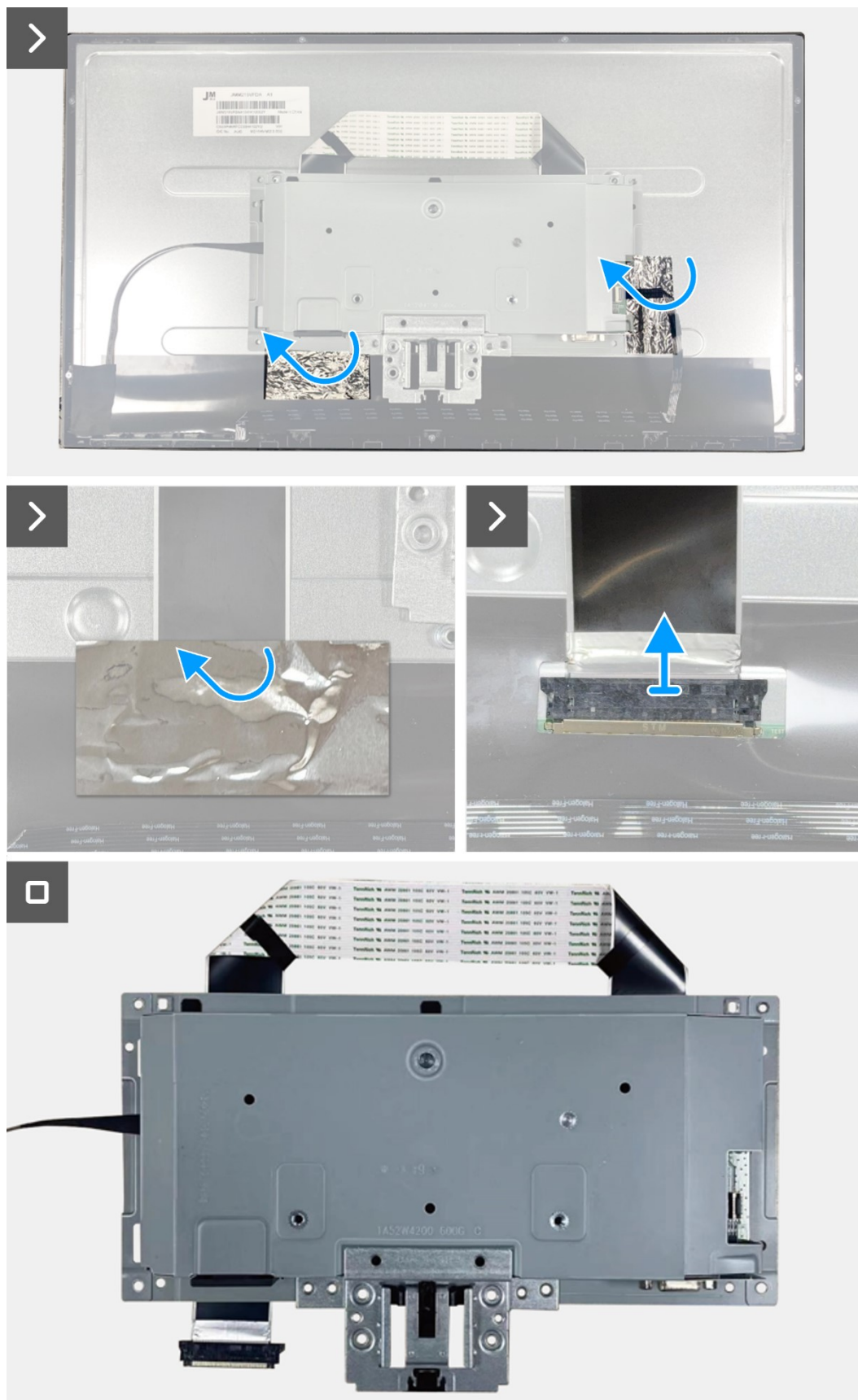
Obrázek 17. Demontáž sestavy skříně
