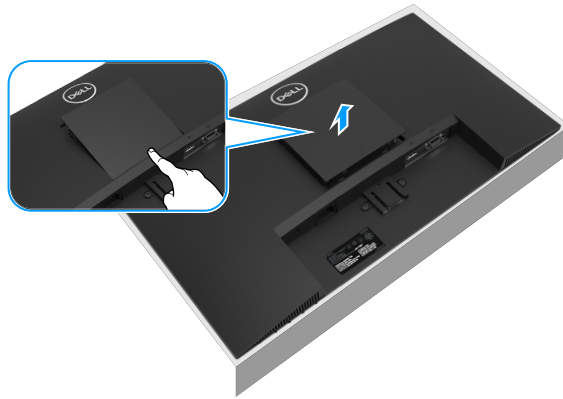
Abbildung 21 Drücken Sie die Spalte zum Entfernen der VESA-Abdeckung
