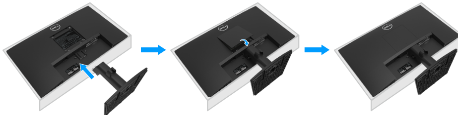
Abbildung 13 Ständer anbringen
