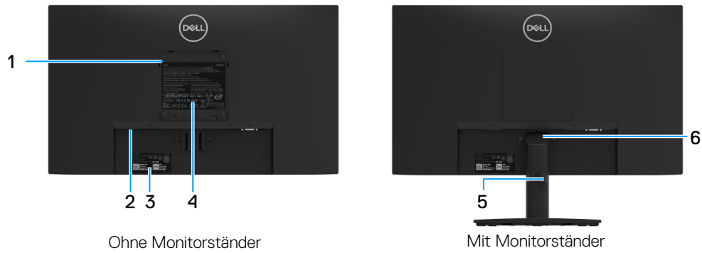
Abbildung 2 Rückansicht des Monitors
