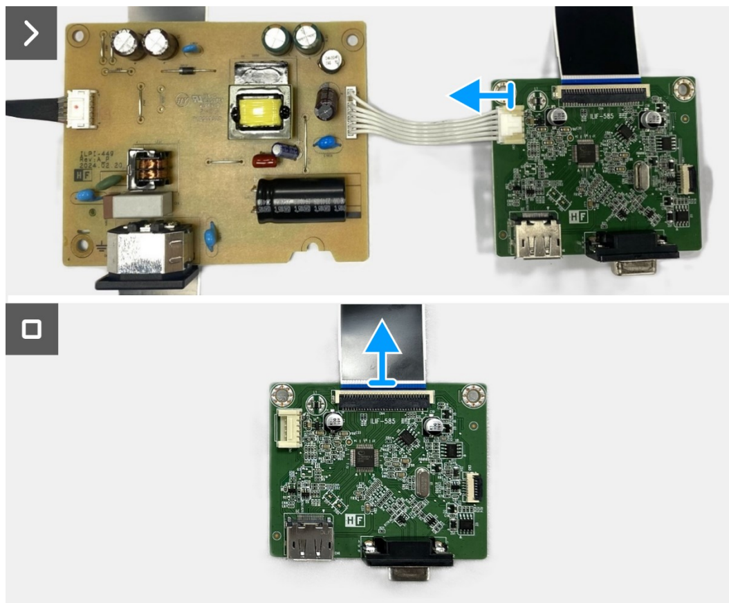
Schéma 21. Retrait de la carte d'interface
