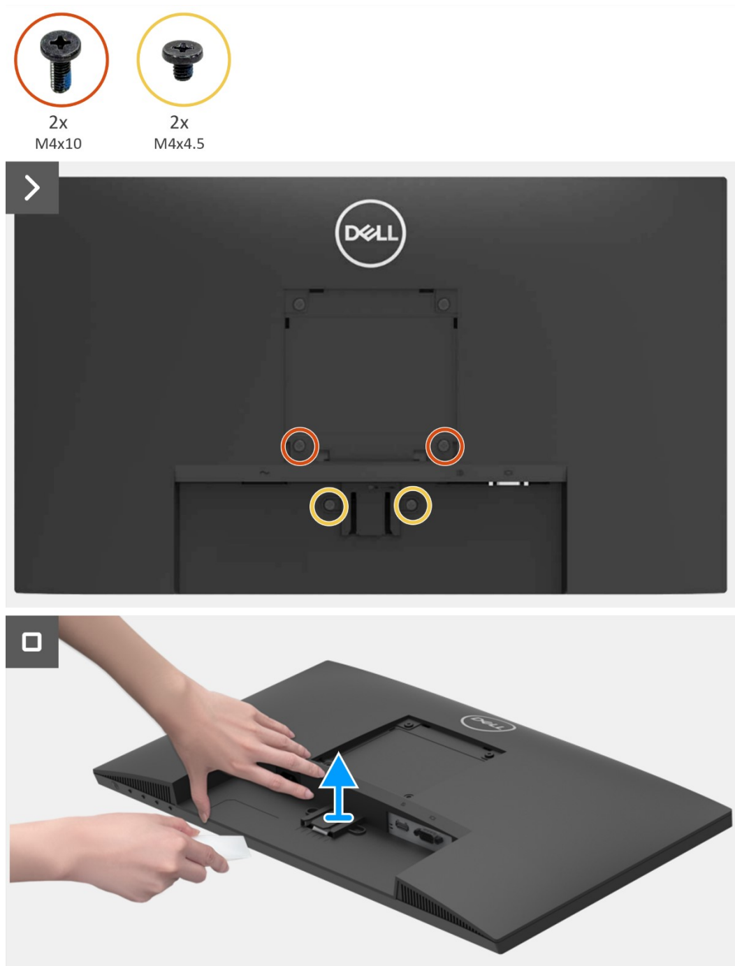
Schéma 12. Retrait du couvercle arrière
