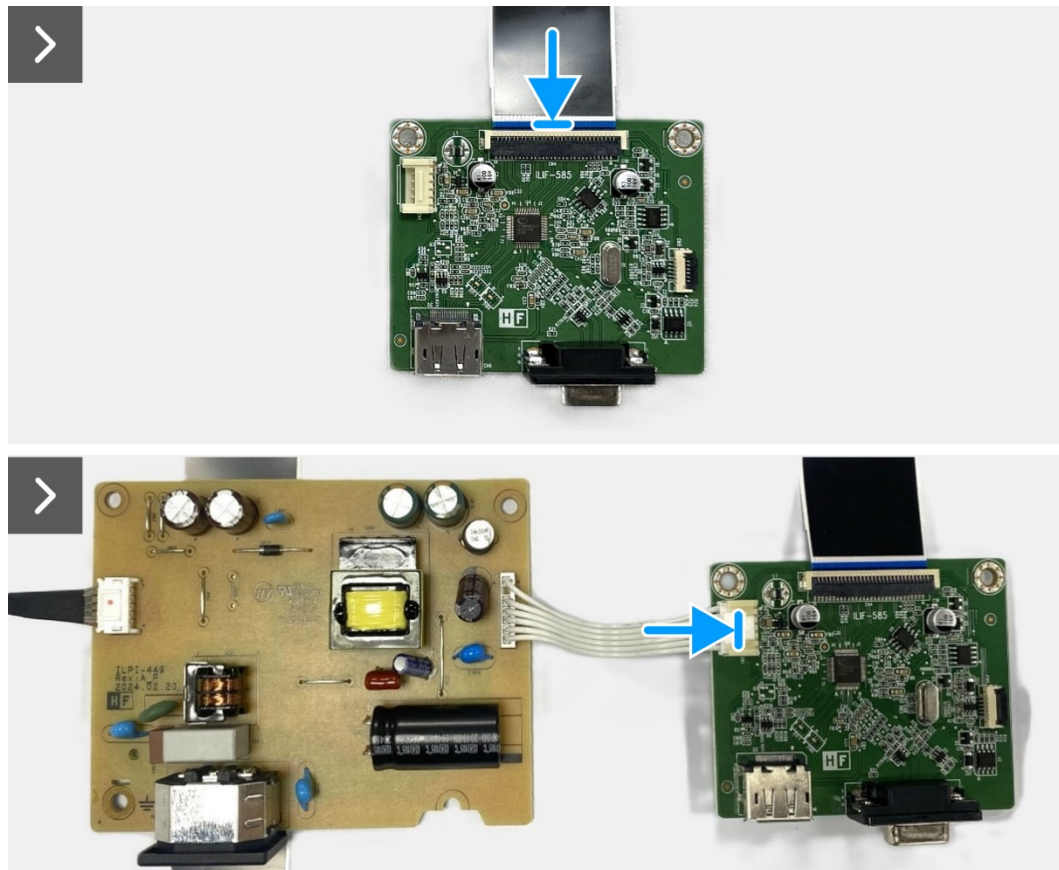
Schéma 22. Installez la carte d'interface
