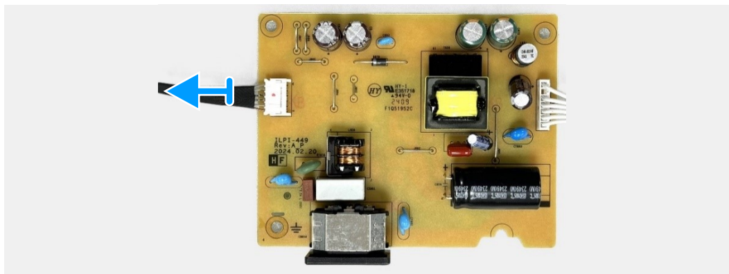
Schéma 24. Retrait de la carte d'alimentation
