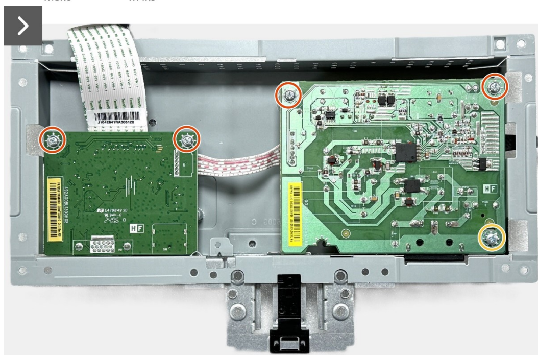
Schéma 20. Retrait de la carte d'interface
