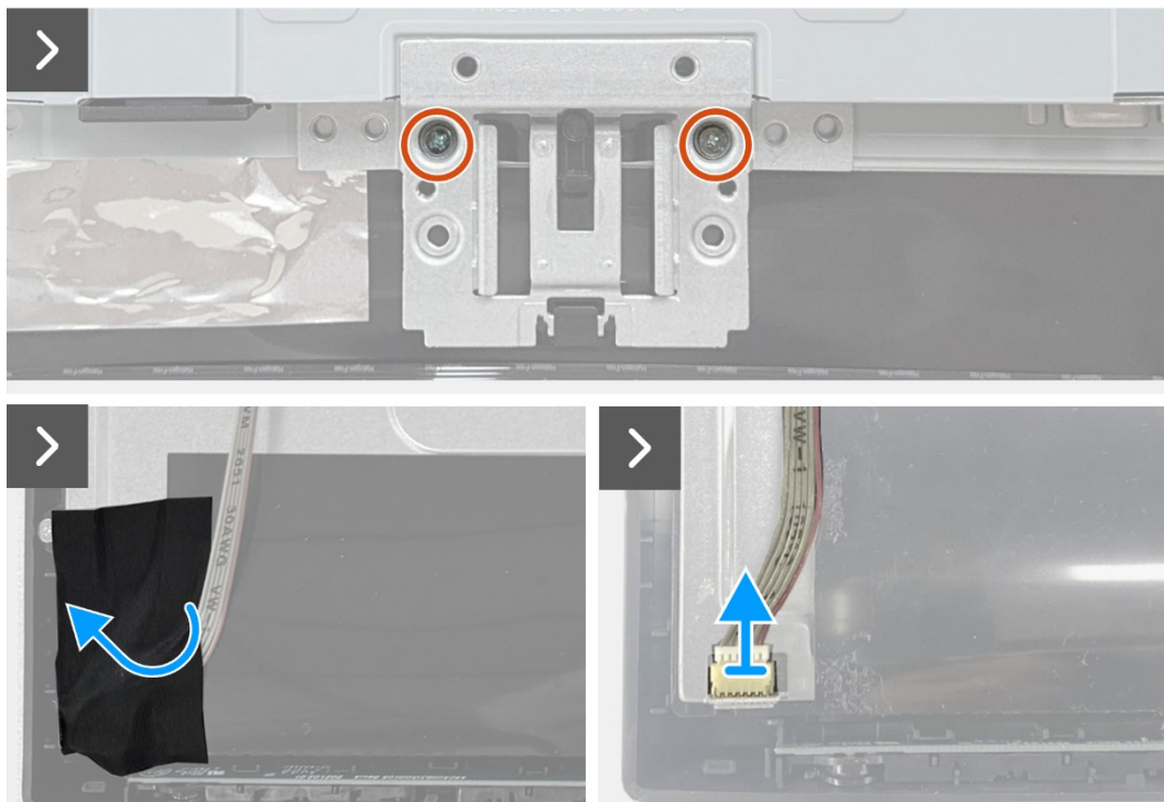
Schéma 16. Retrait de l'ensemble de châssis
