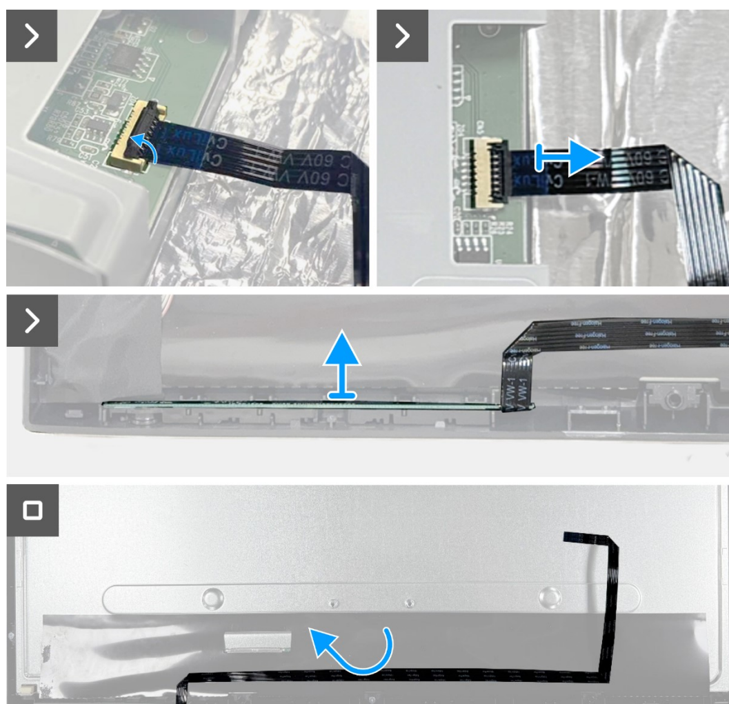
Schéma 14. Retrait du clavier
