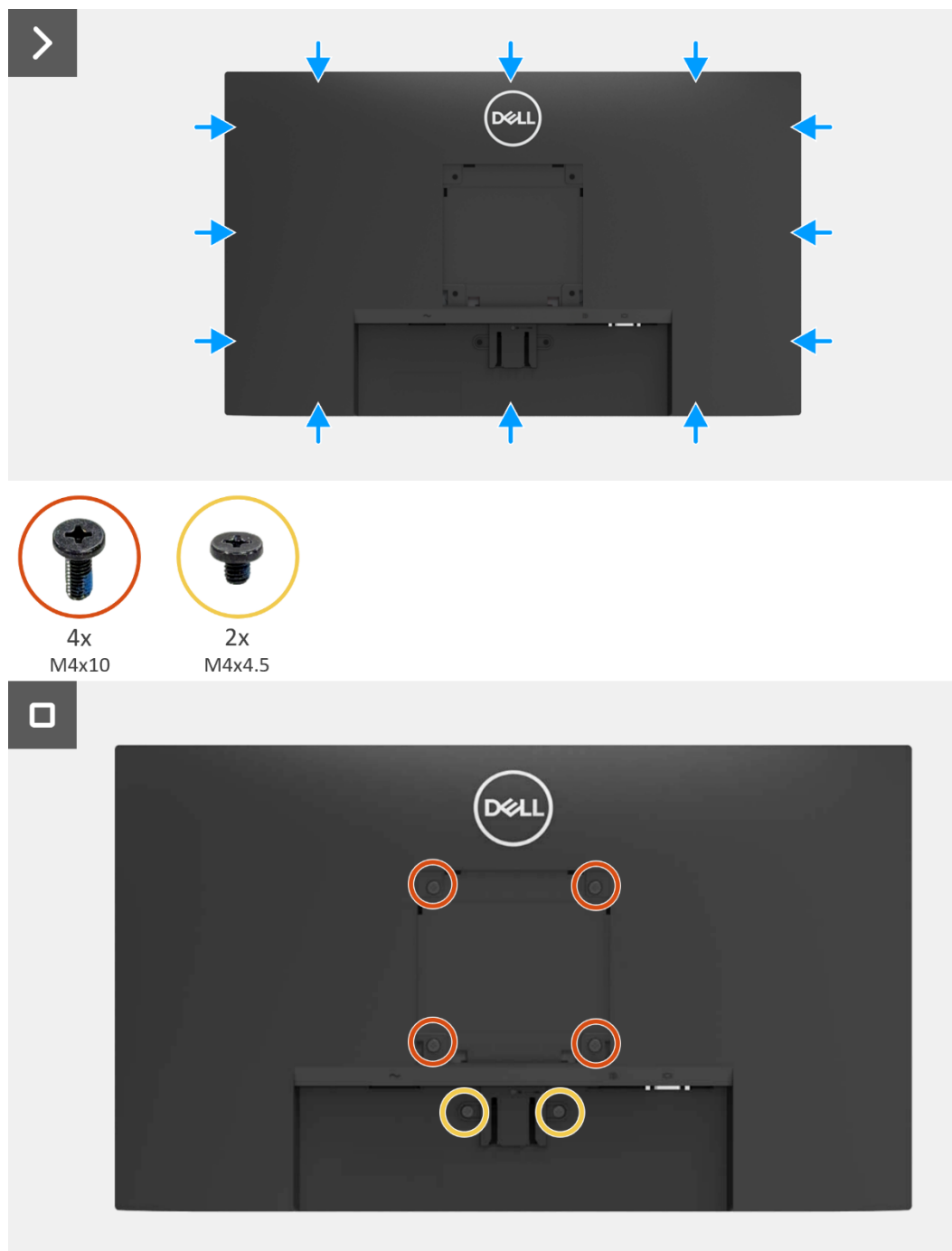
Schéma 13. Installez le couvercle arrière
