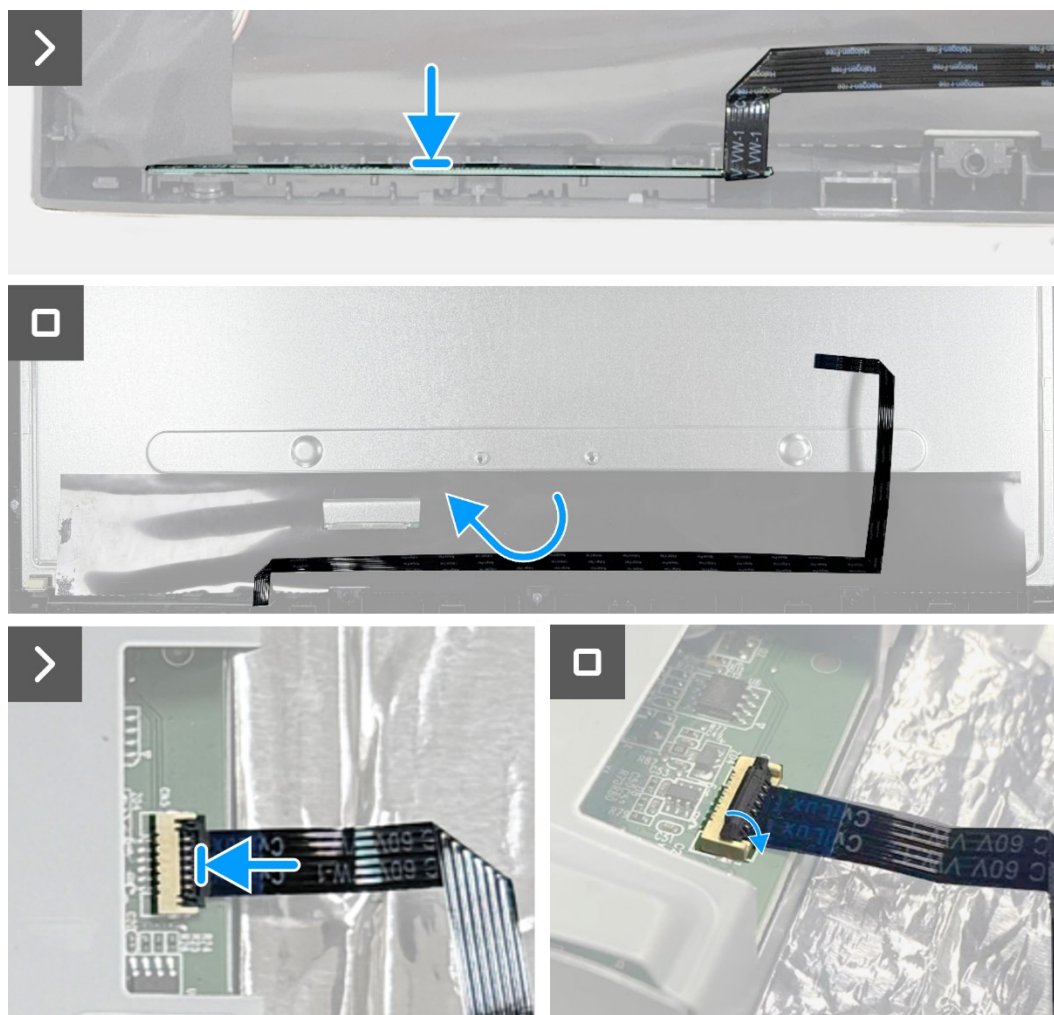
Schéma 15. Installation du clavier
