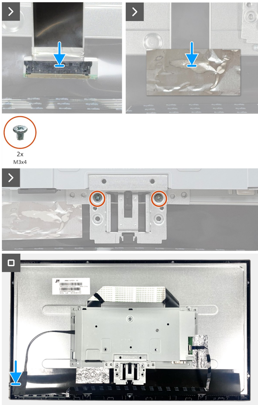
Schéma 18. Installez l'ensemble de châssis
