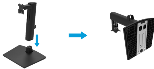
Abbildung 13. Ständer montieren
