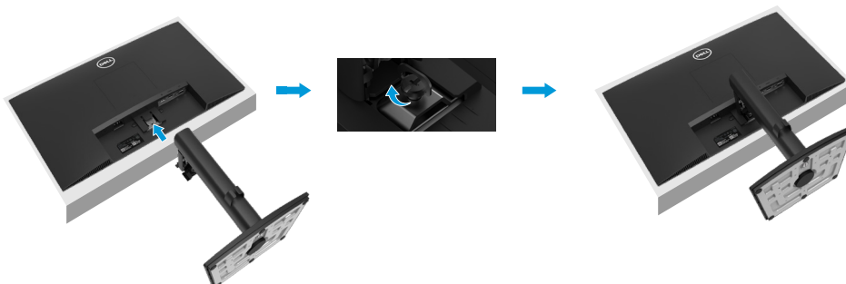
Rysunek 18. Przymocować podstawę
