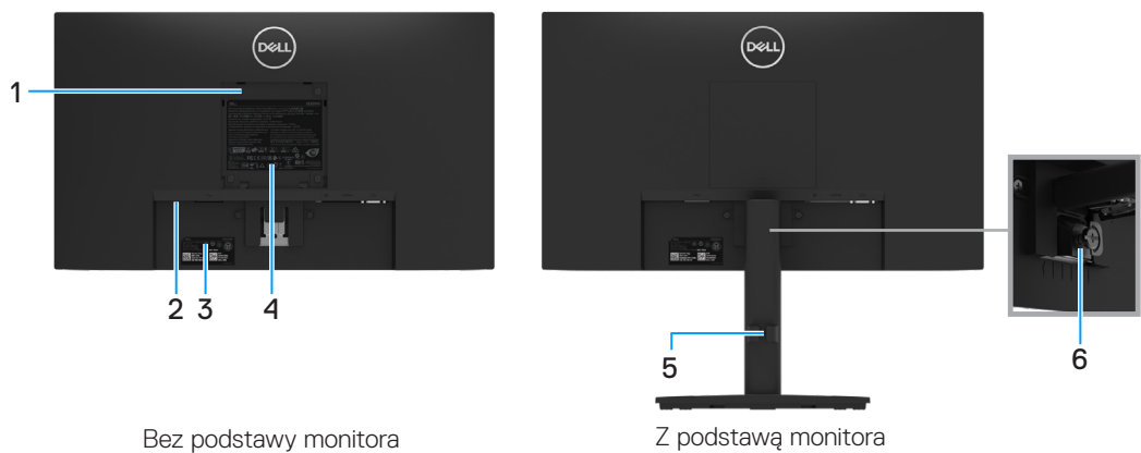
Rysunek 2. Widok monitora z tyłu
