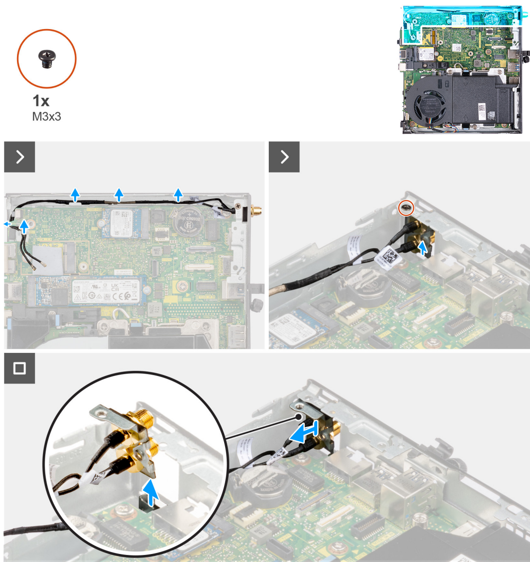
Abbildung 54. Entfernen der SMA-Antenne (Position 3)
