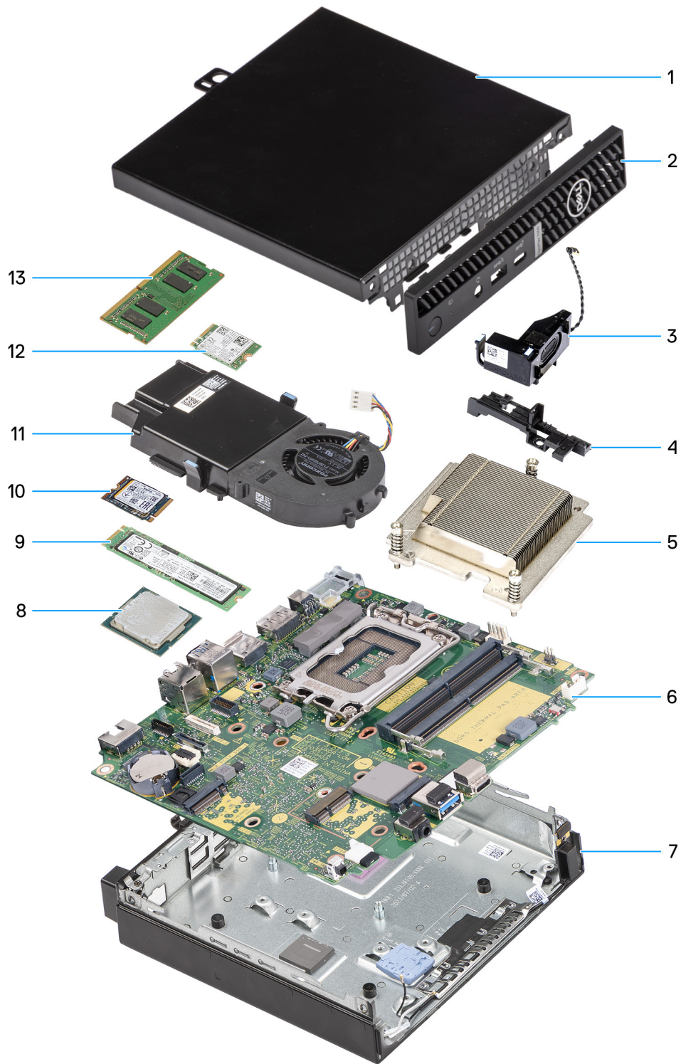
Abbildung 8. Hauptkomponenten des OptiPlex Micro 7020
