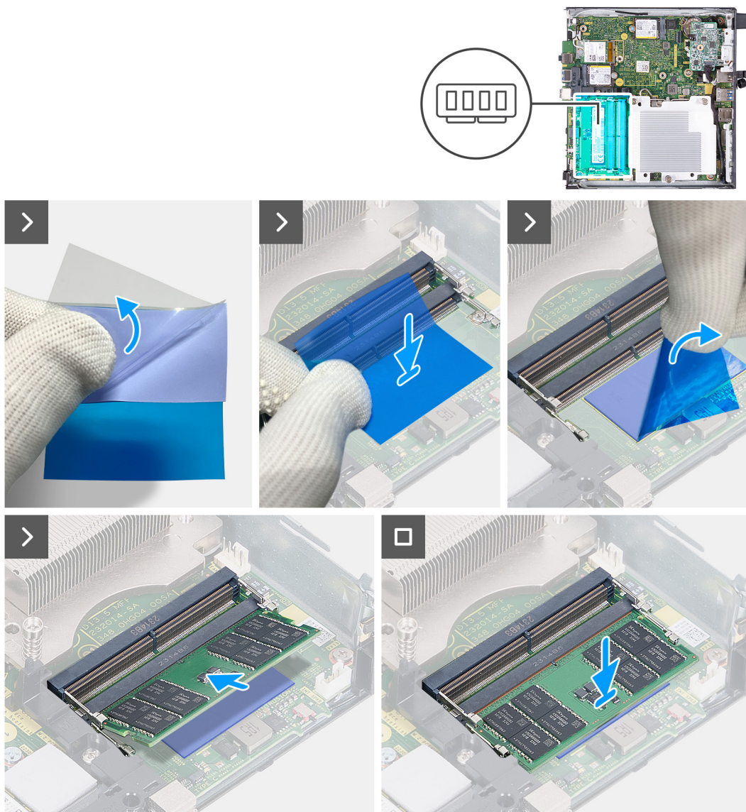
Abbildung 33. Einsetzen des Arbeitsspeichers
