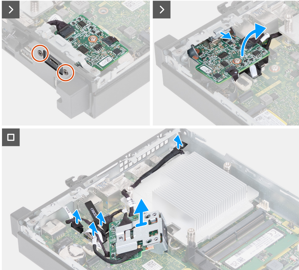
Abbildung 38. Entfernen des optionalen Typ-C-Moduls
