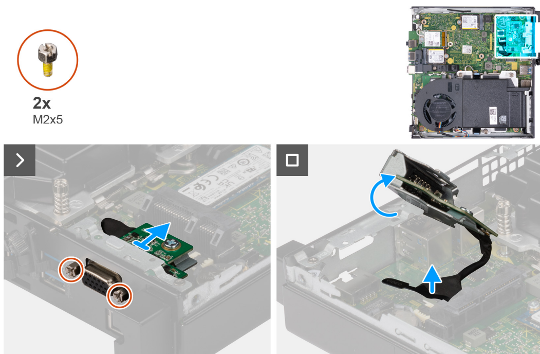
Abbildung 35. Entfernen des optionalen E/A-Moduls (VGA oder Seruell)
