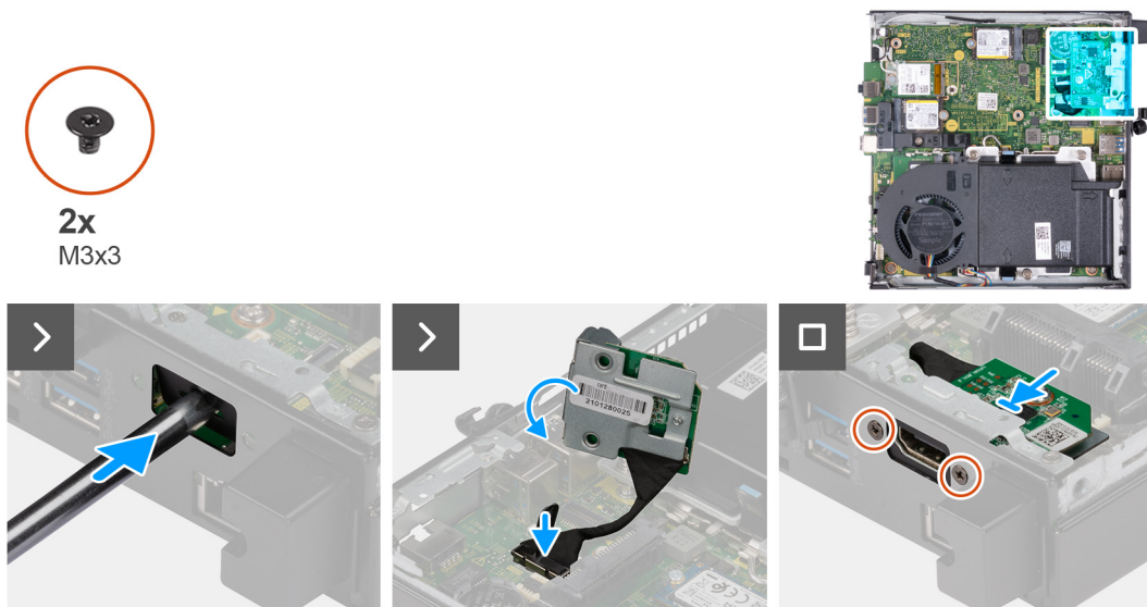
Abbildung 36. Installieren eines optionalen E/A-Moduls (HDMI, DP oder PS2)
