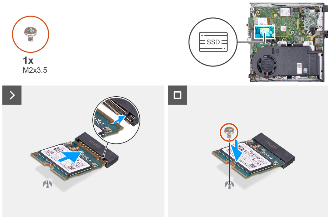
Abbildung 20. Installieren des 2230-Solid-State-Laufwerks in Steckplatz 0
