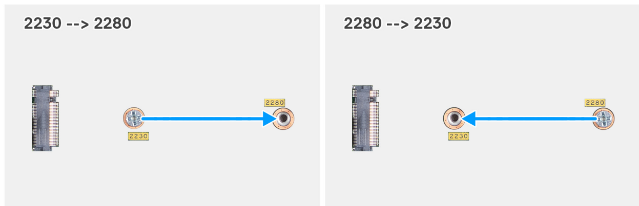
Abbildung 27. Verschieben der Schraubbefestigung zur Unterstützung eines anderen Formfaktors (OptiPlex Micro 7020)
