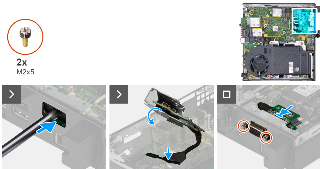
Abbildung 37. Installieren eines optionalen E/A-Moduls (VGA oder Seriell)
