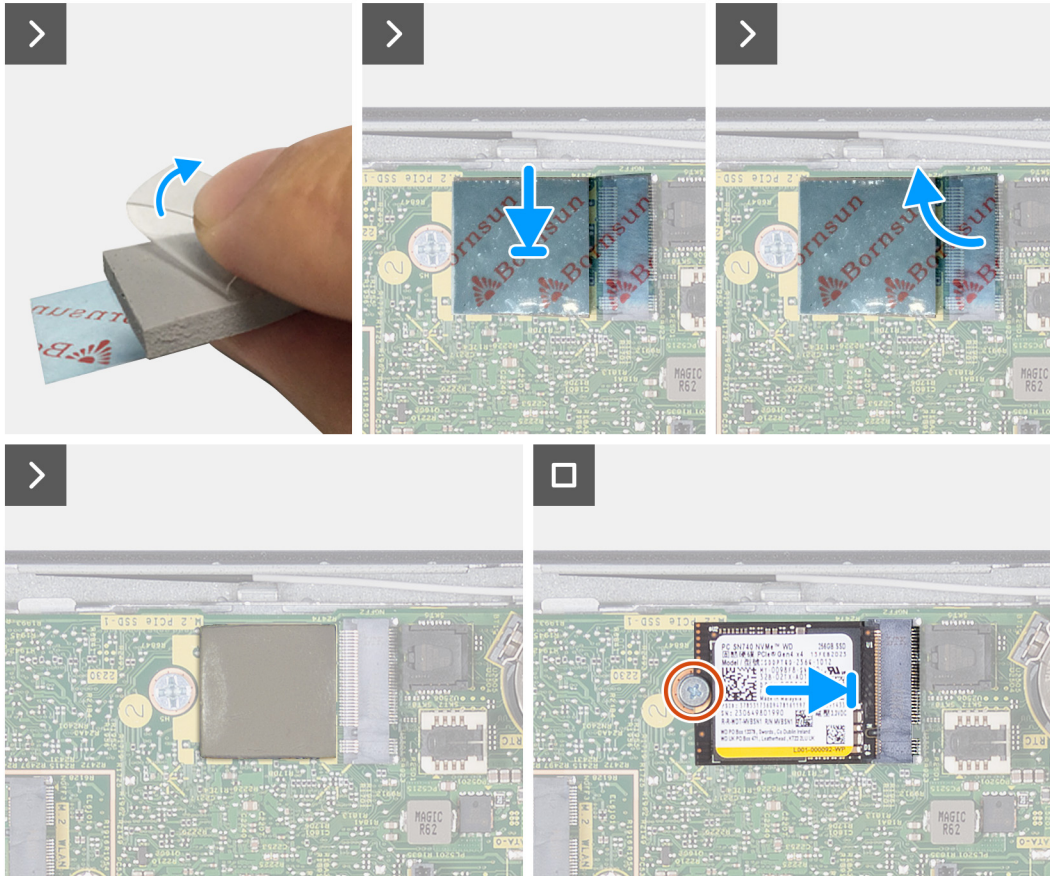
Abbildung 24. Installieren des M.2 2230-Solid-State-Laufwerks in Steckplatz 1
