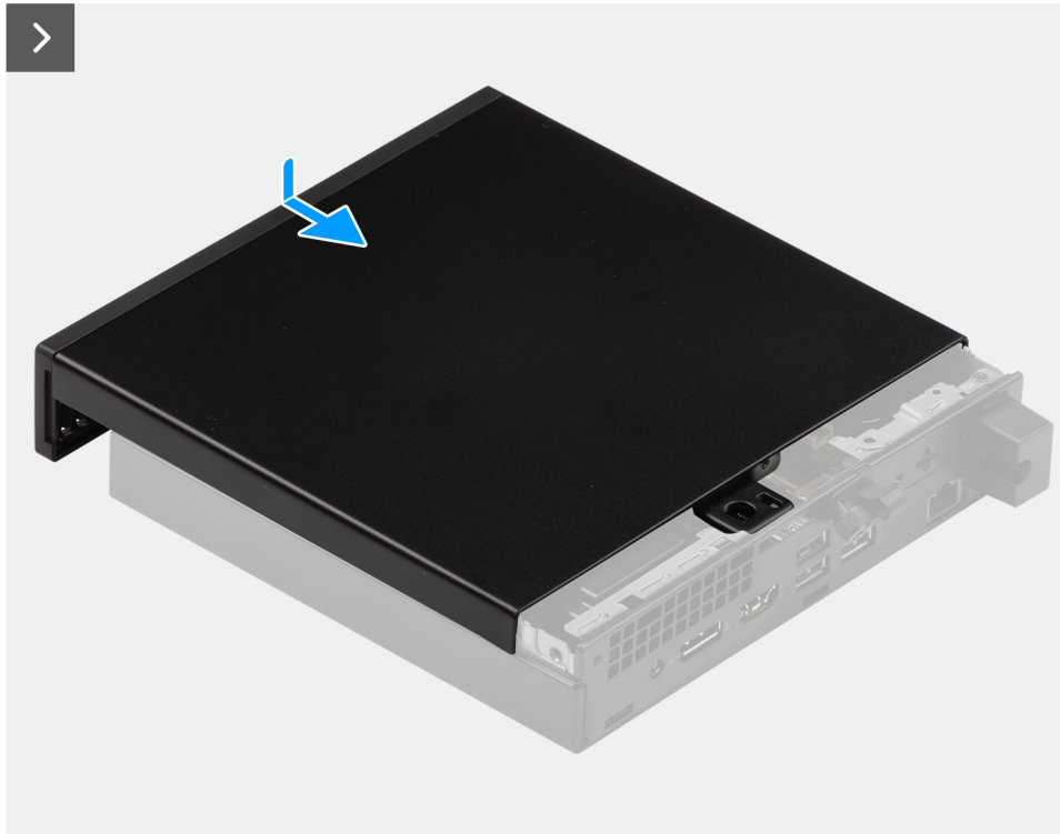
Abbildung 11. Anbringen der Seitenabdeckung
