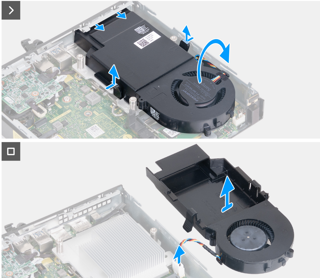
Abbildung 30. Entfernen des Lüfters
