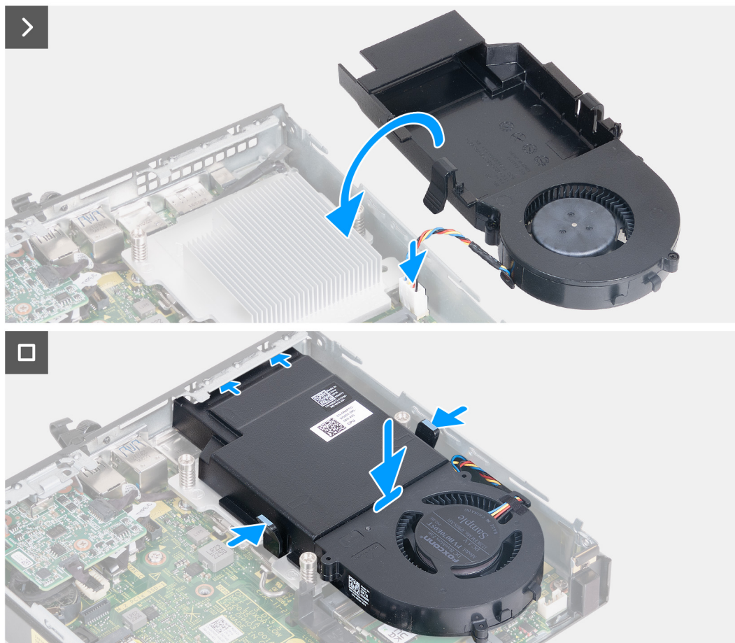
Abbildung 31. Einbauen des Lüfters
