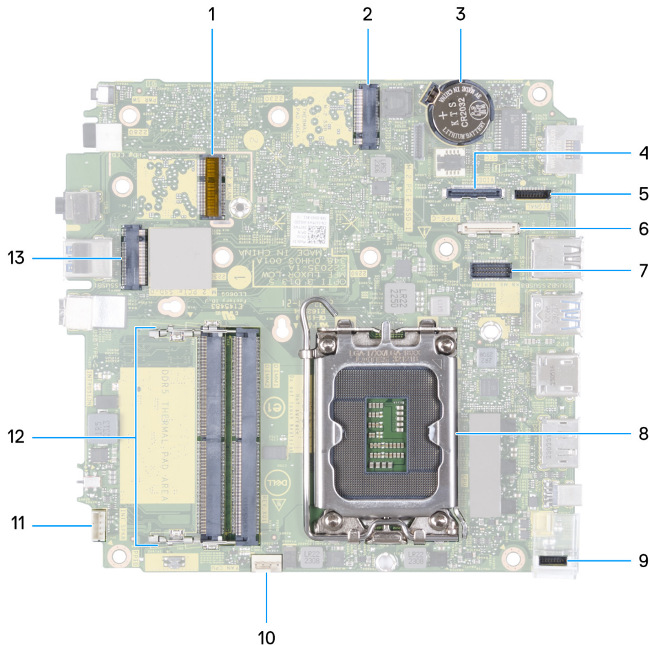
Abbildung 44. Abbildung: Systemplatinenanschlüsse
