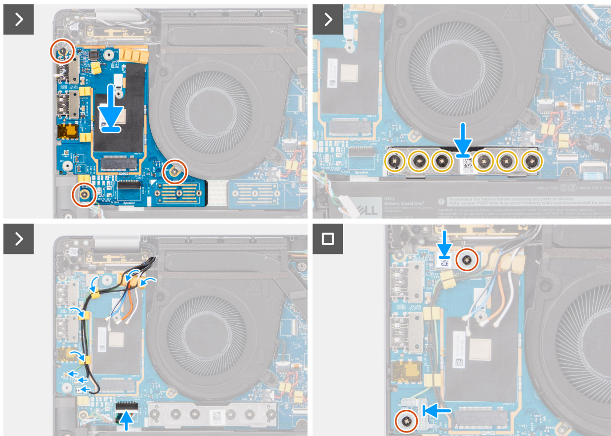
Afbeelding 75. De I/O-dochterkaart plaatsen
