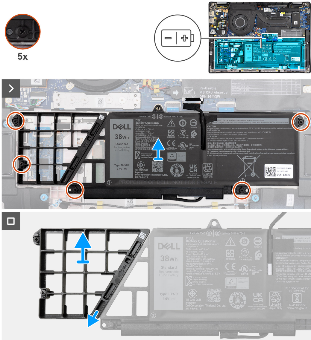
Afbeelding 37. De 2-cels batterij verwijderen
