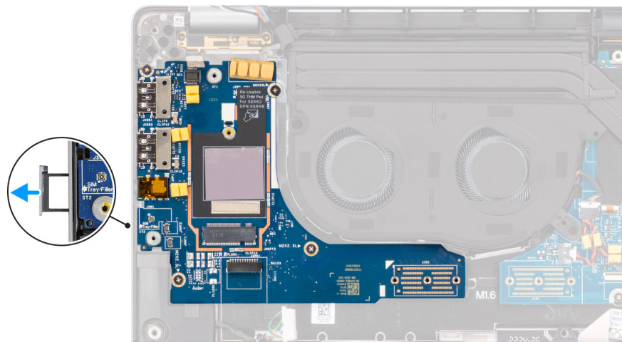
Afbeelding 70. De I/O-dochterkaart verwijderen
