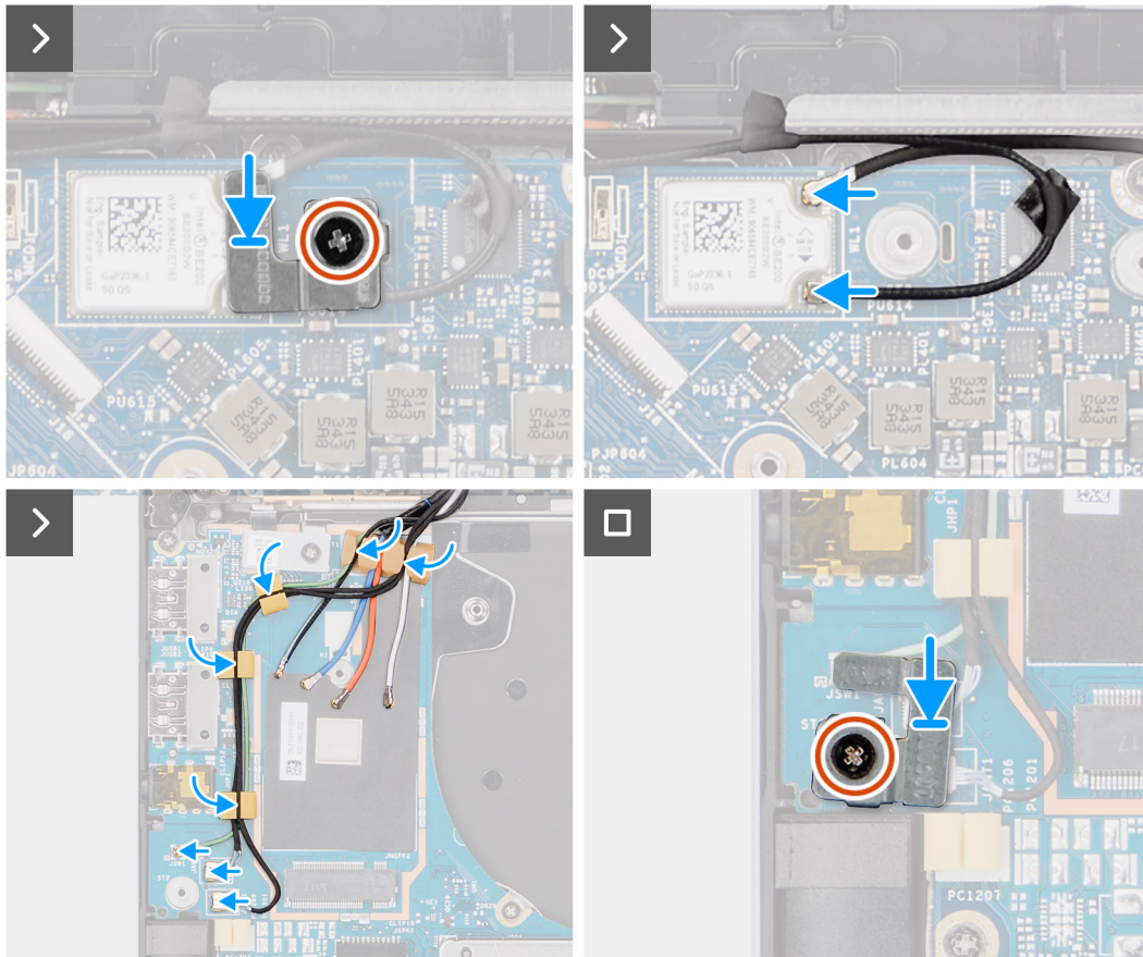
Afbeelding 69. De WLAN-antennemodule installeren
