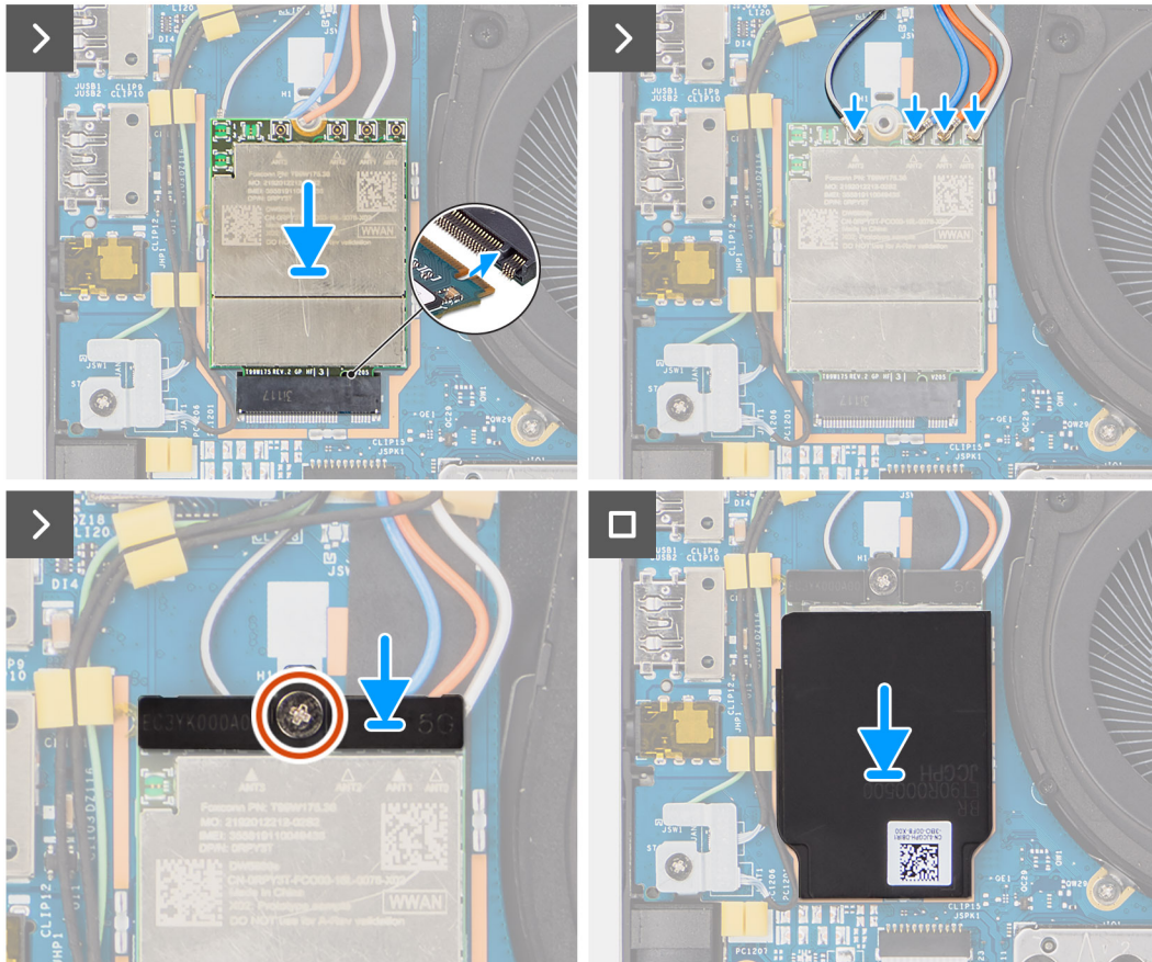
Afbeelding 27. De 5G WWAN-kaart installeren
