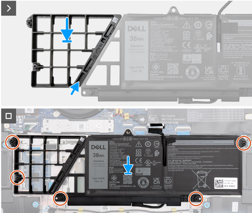
Afbeelding 39. De 2-cels batterij installeren
