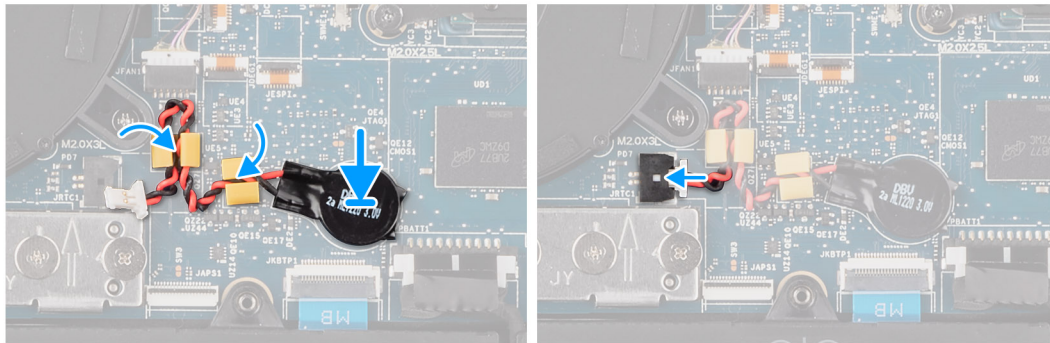
Afbeelding 36. De knoopcelbatterij plaatsen
