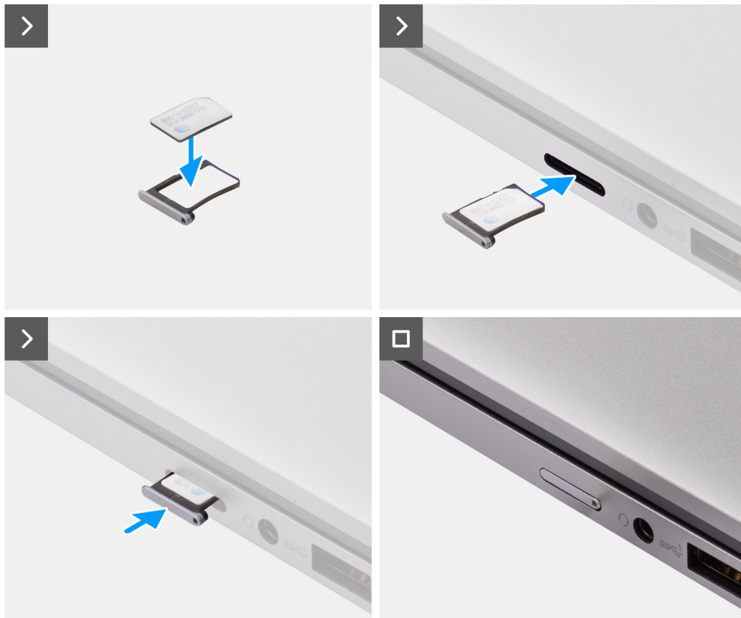
Afbeelding 15. Het simkaartvak plaatsen
