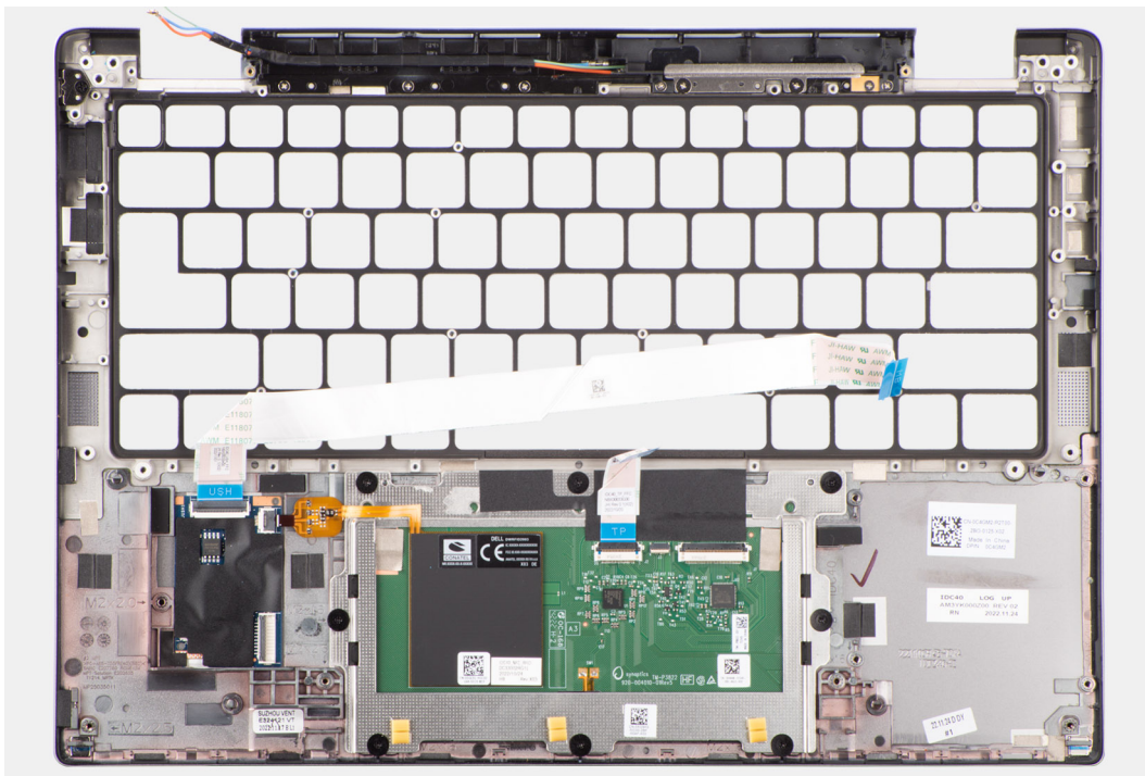
Afbeelding 84. De palmsteuneenheid verwijderen
