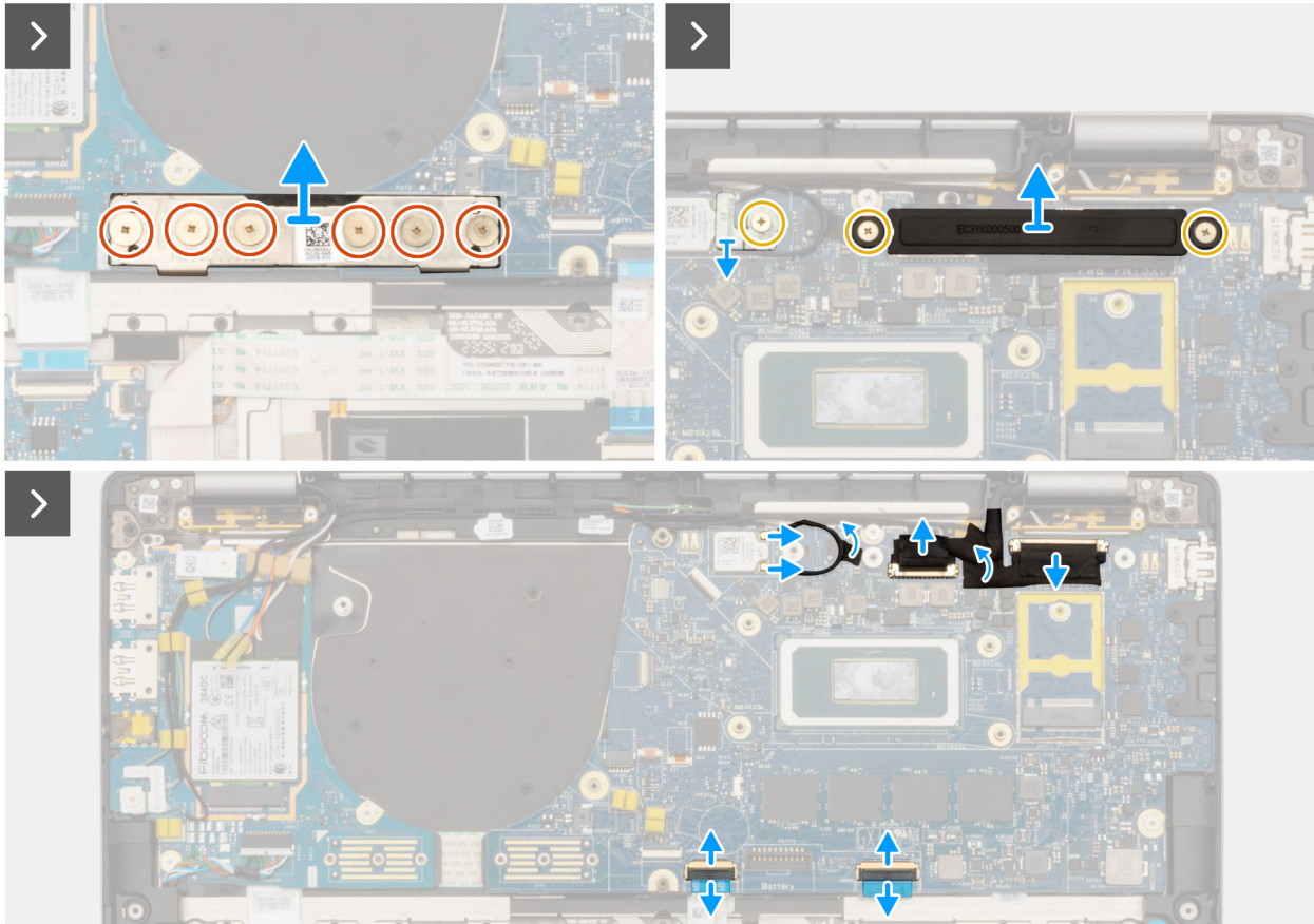
Afbeelding 59. De systeemkaart verwijderen
