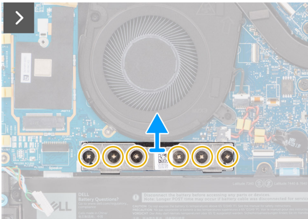
Afbeelding 71. De I/O-dochterkaart verwijderen
