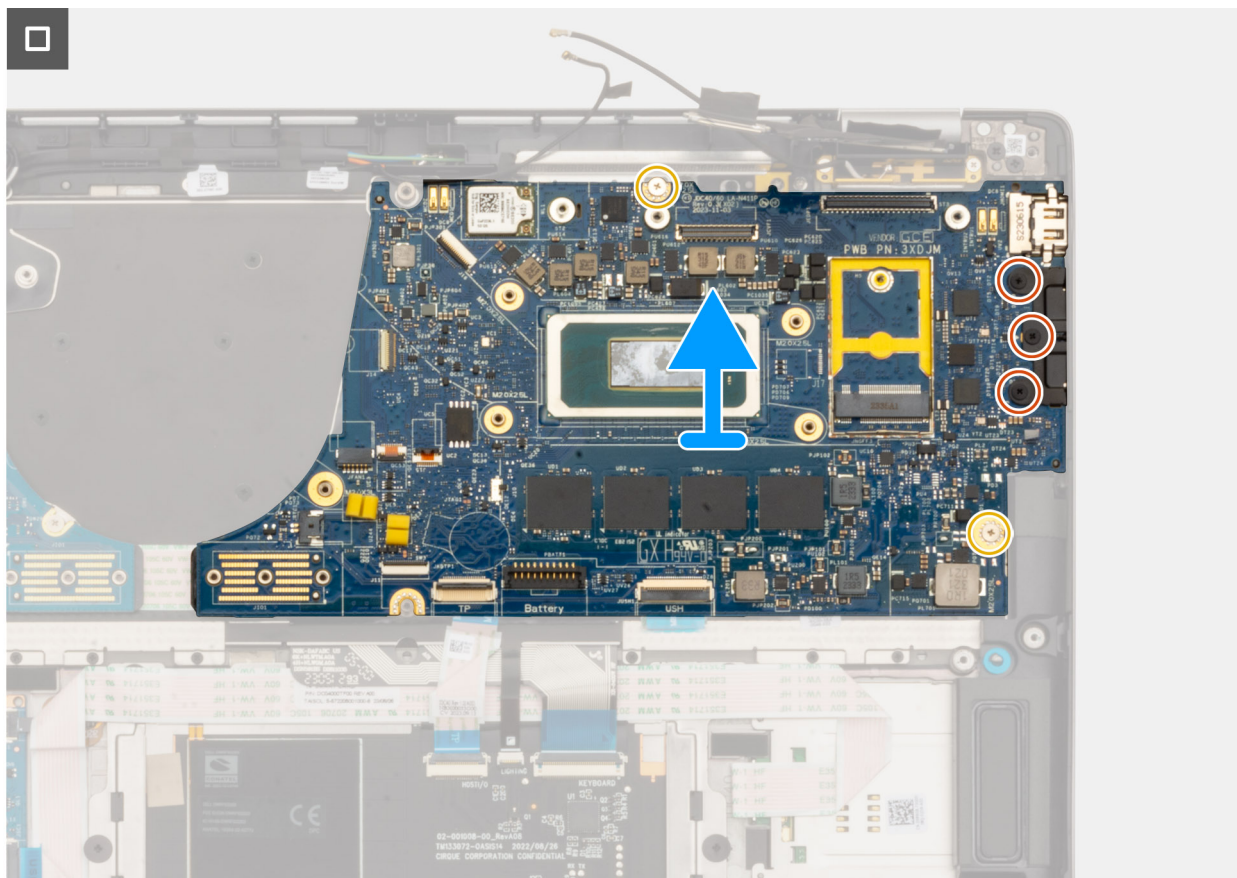
Afbeelding 60. De systeemkaart verwijderen
