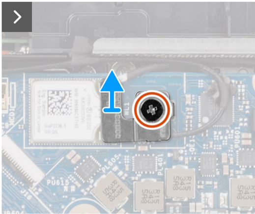
Afbeelding 66. De WLAN-antennemodule verwijderen
