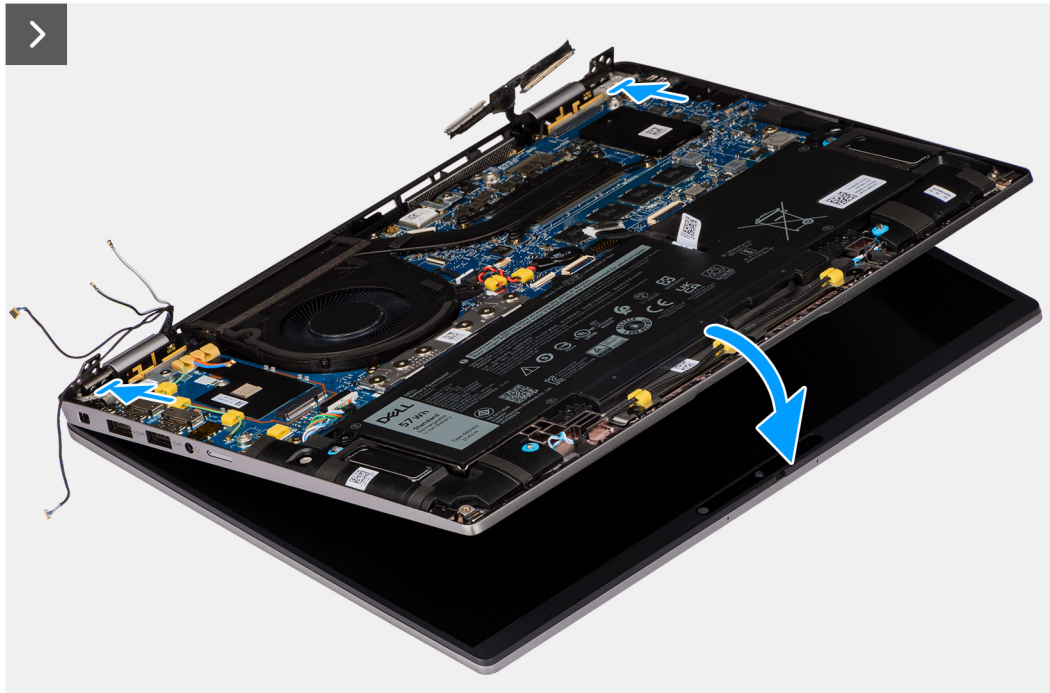
Afbeelding 53. De beeldschermenheid plaatsen
