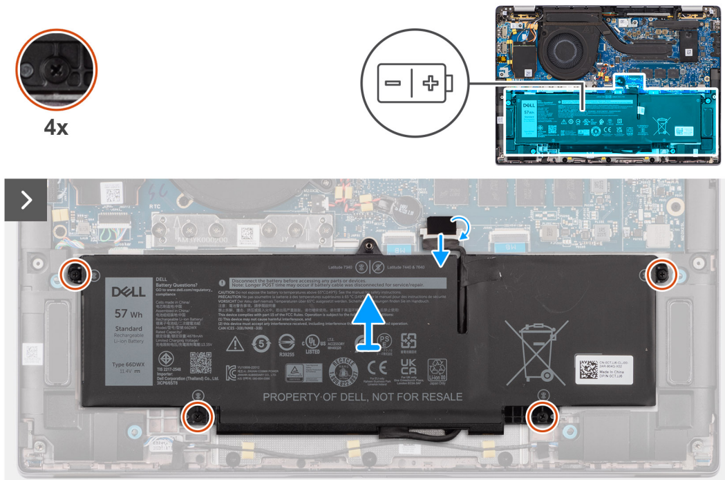
Afbeelding 40. De 3-cels batterij verwijderen
