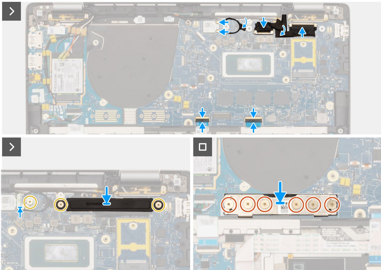
Afbeelding 65. De systeemkaart installeren
