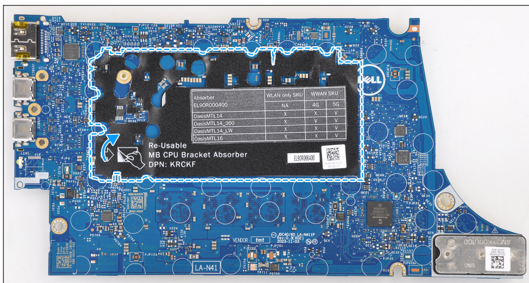
Afbeelding 62. CPU-beugelopnemer
