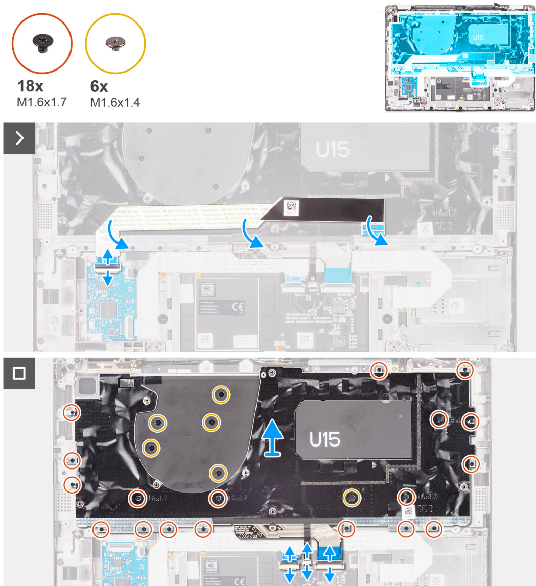
Afbeelding 78. Het toetsenbord verwijderen
