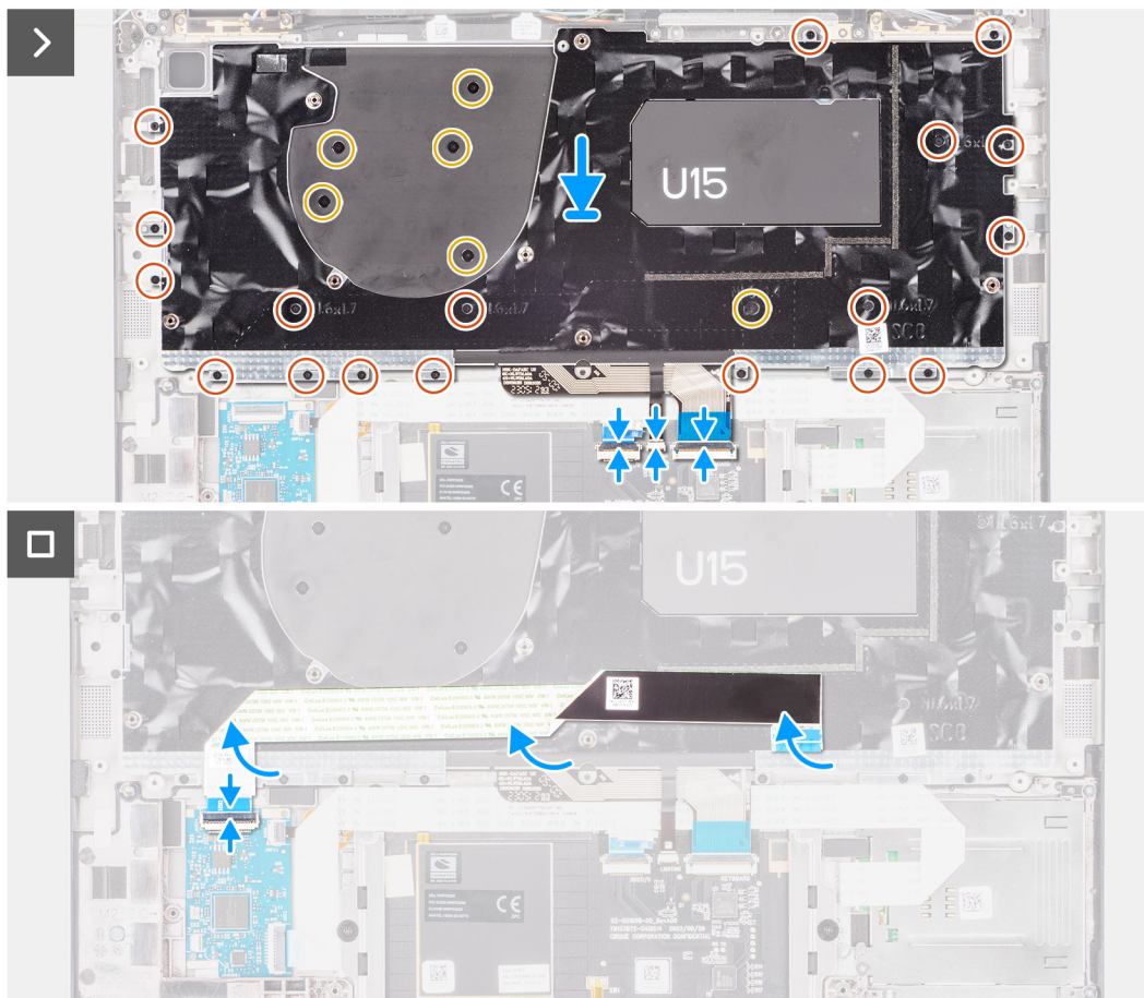
Afbeelding 81. Het toetsbord plaatsen
