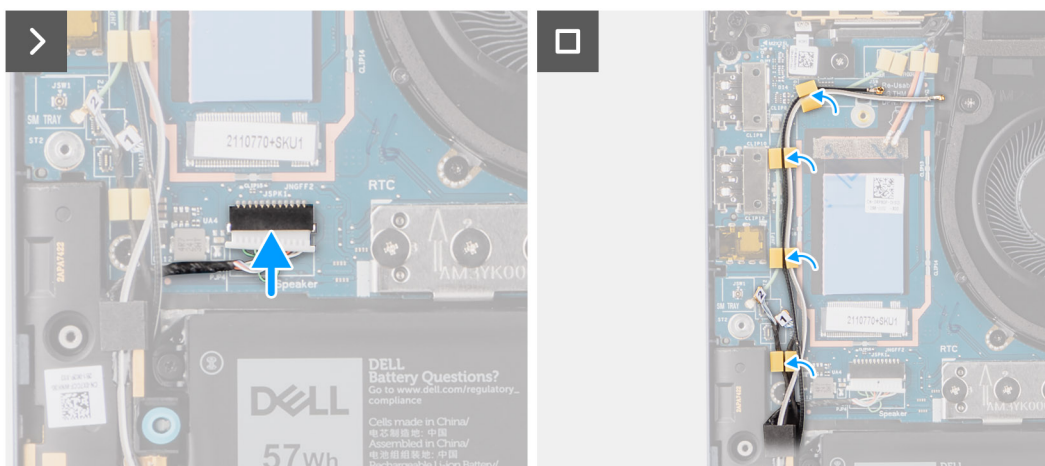
Afbeelding 32. De luidsprekers voor de Ultralight installeren
