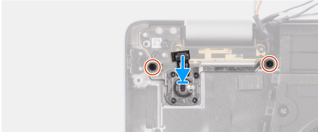
Afbeelding 77. De aan/uit-knop met optionele vingerafdrukkezer plaatsen
