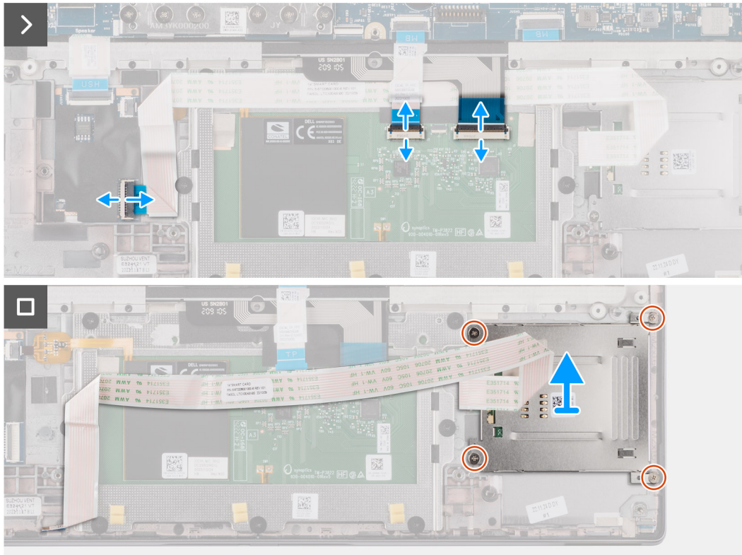
Afbeelding 56. De smartcardlezer verwijderen
