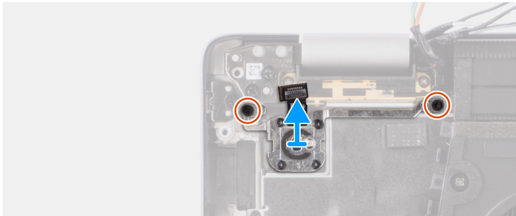
Afbeelding 76. De aan/uit-knop met de optionele vingerafdrukkeuze verwijderen
