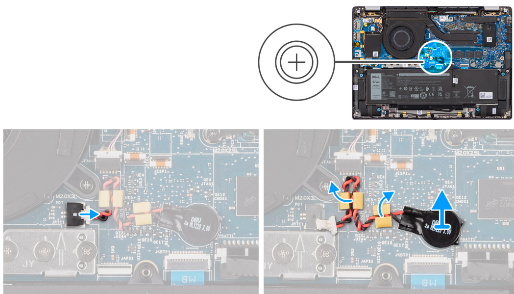
Afbeelding 35. De knoopcelbatterij verwijderen
