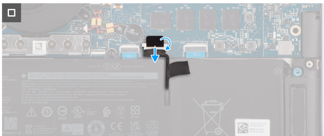
Afbeelding 18. De onderplaat verwijderen
