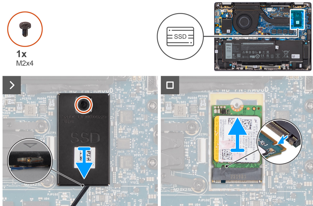
Afbeelding 22. De M.2 2230 SSD verwijderen
