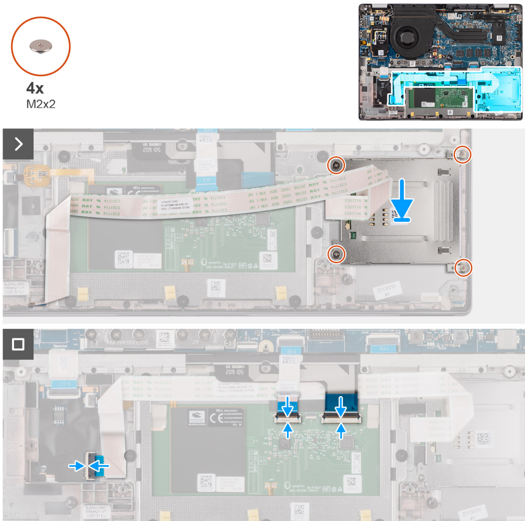
Afbeelding 57. De smartcardlezer installeren
