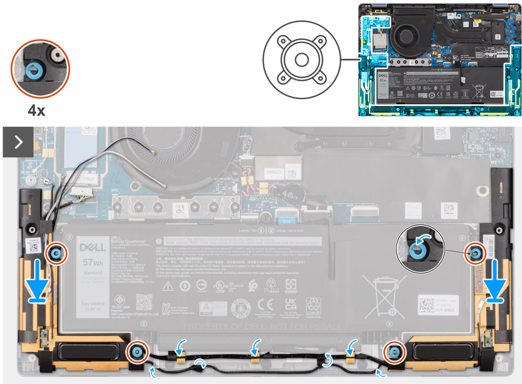
Afbeelding 31. De luidsprekers voor de Ultralight installeren
