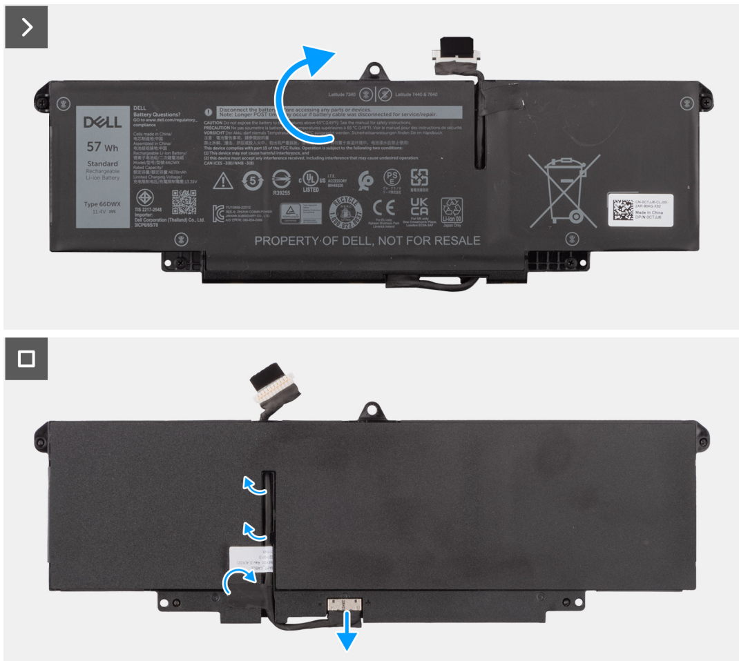
Afbeelding 41. De 3-cels batterij verwijderen
