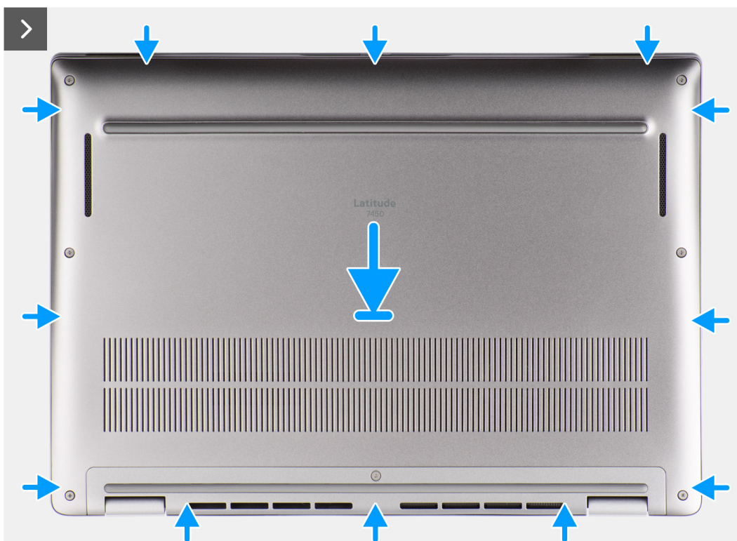
Afbeelding 20. De onderplaat plaatsen
