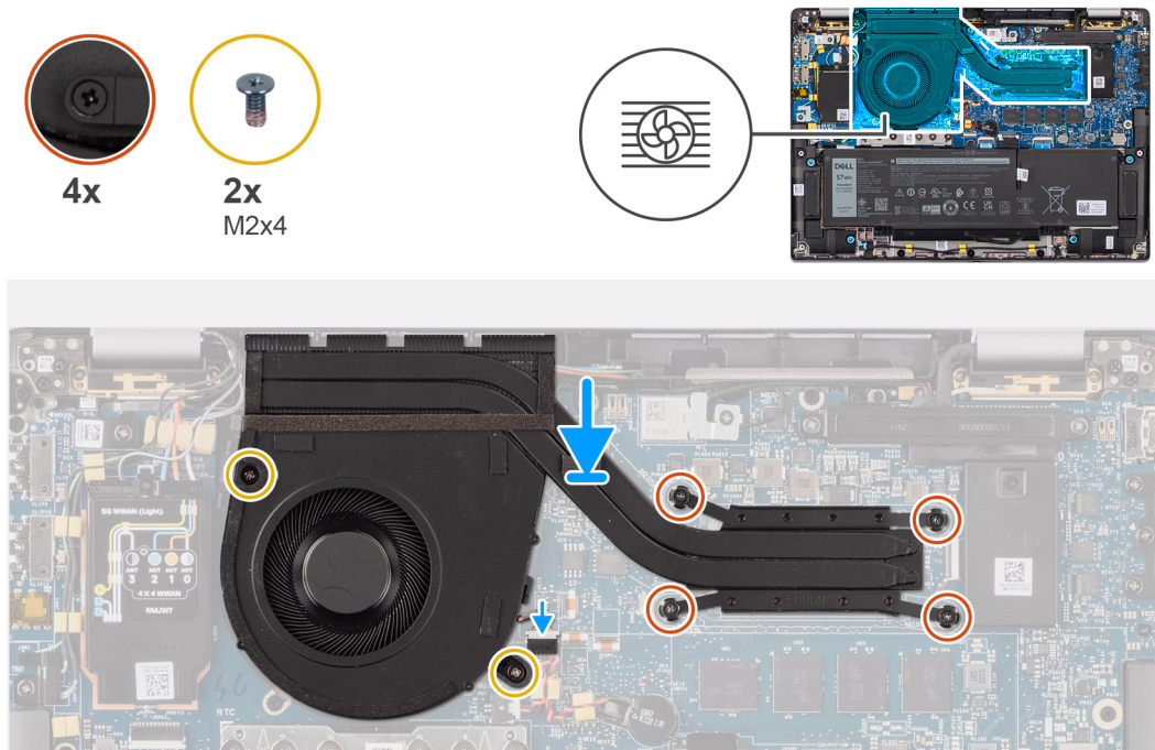
Afbeelding 47. De koelplaat- en ventilatoreenheid installeren
