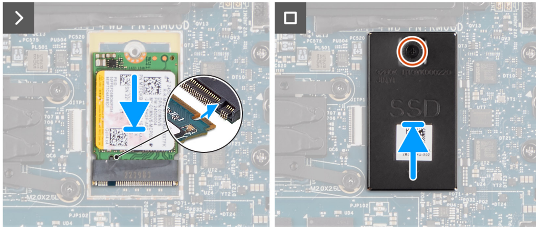
Afbeelding 23. De M.2 2230 SSD plaatsen
