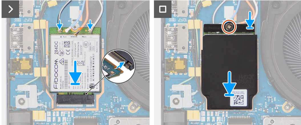
Afbeelding 25. De 4G WWAN-kaart installeren
