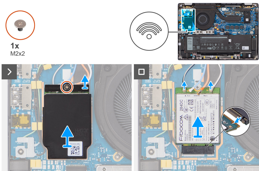
Afbeelding 24. De 4G WWAN-kaart verwijderen
