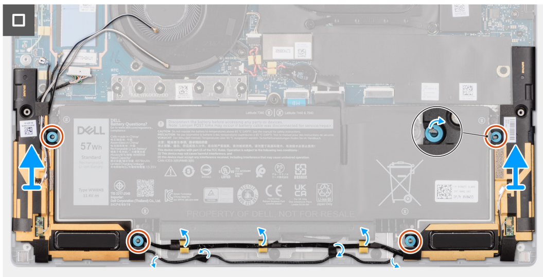
Afbeelding 30. De luidsprekers verwijderen voor de Ultralight
