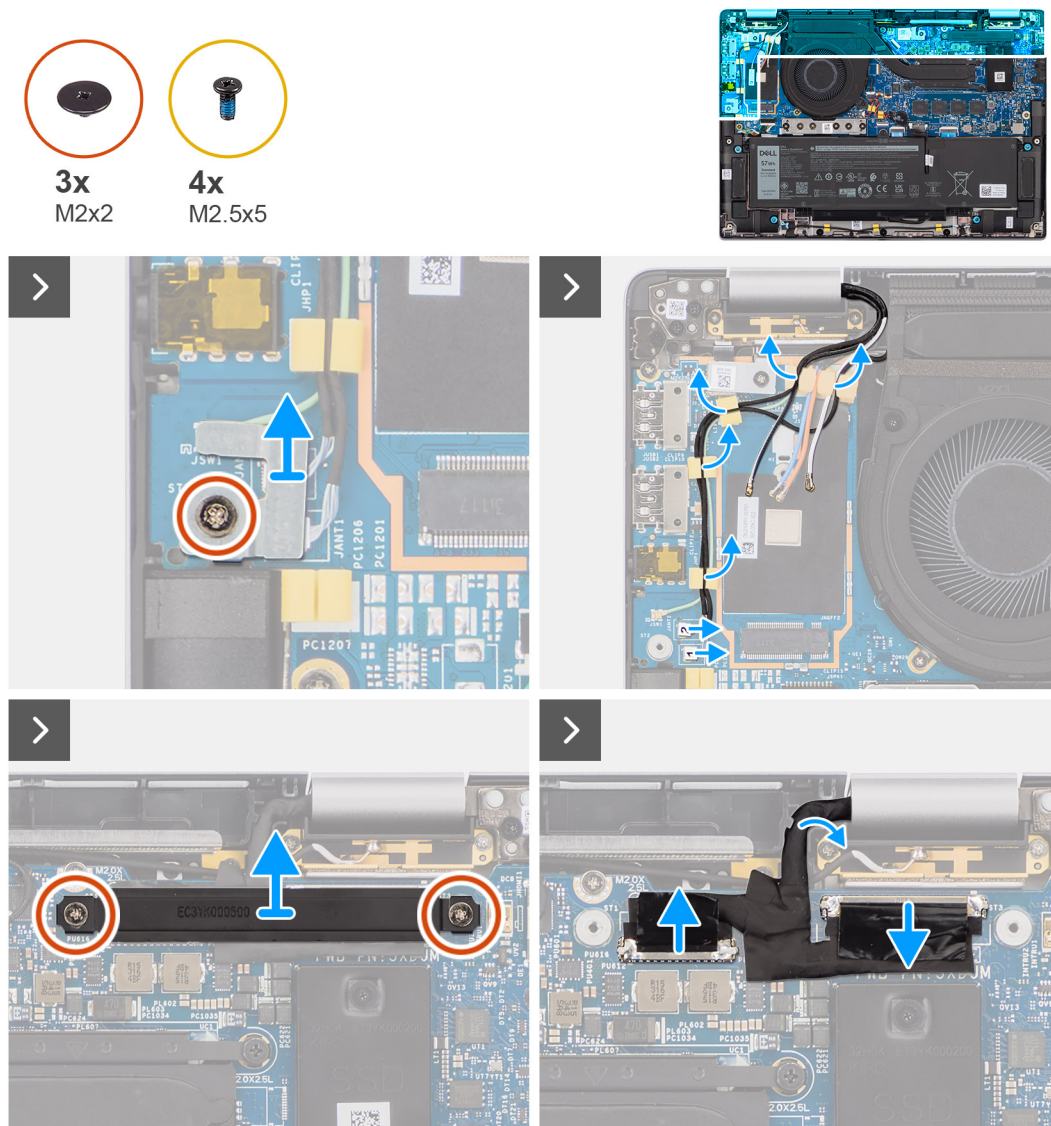
Afbeelding 48. De beeldschermeenheid verwijderen
