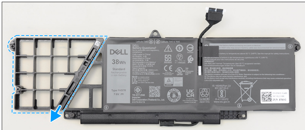
Afbeelding 38. De 2-cels batterij verwijderen
