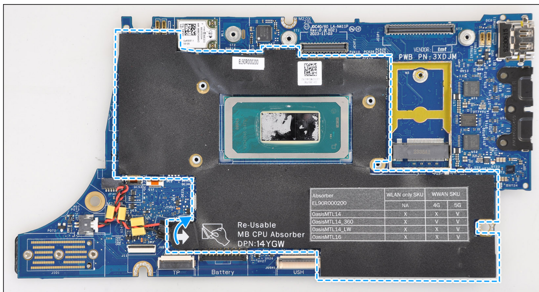
Afbeelding 61. CPU-opnemer
