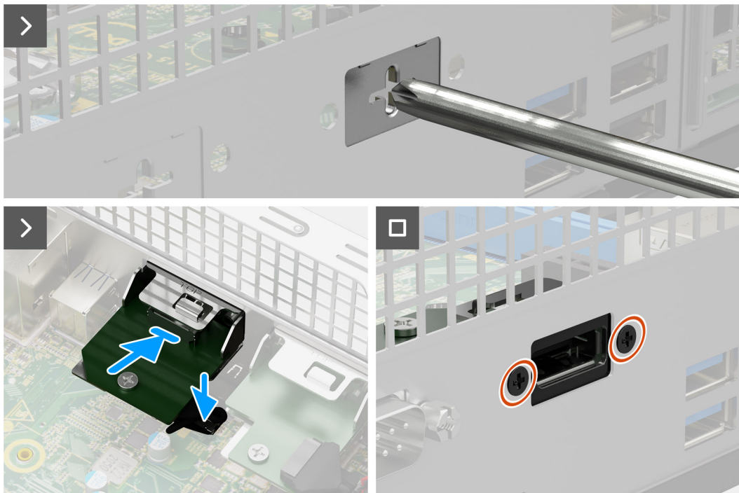
Figure 53. Installation du module DisplayPort
