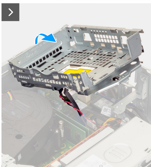
Figure 11. Retrait du bâti du lecteur de disque
