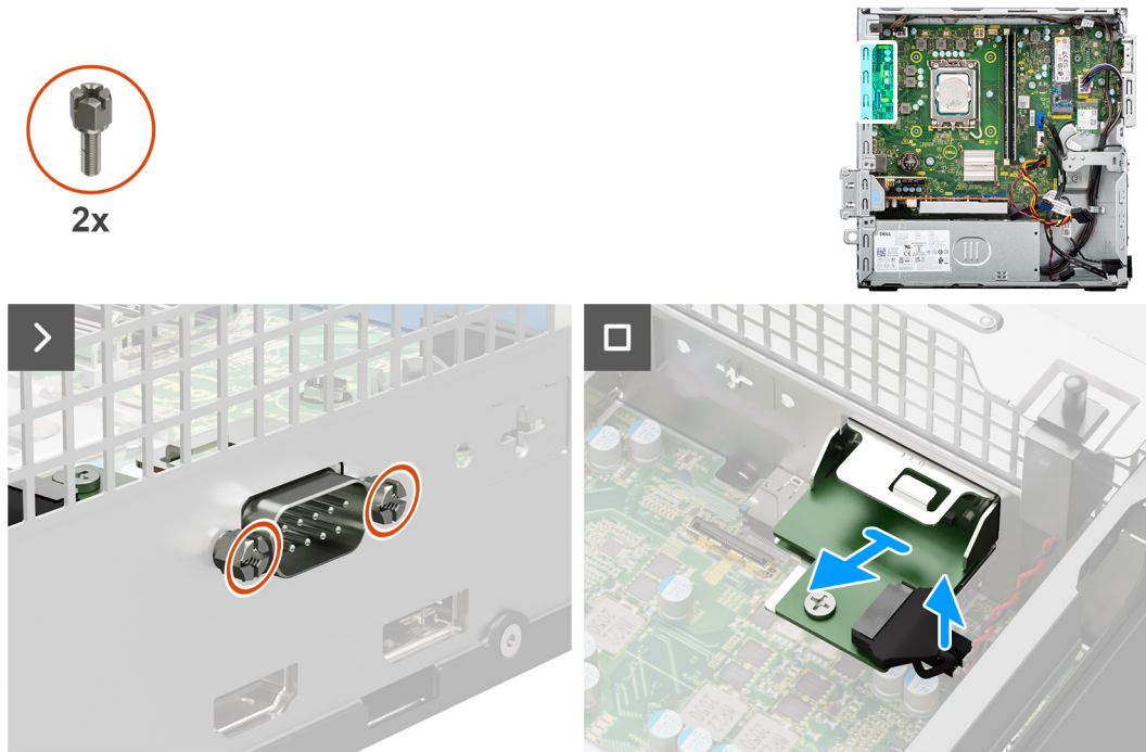
Figure 48. Retrait du module série
