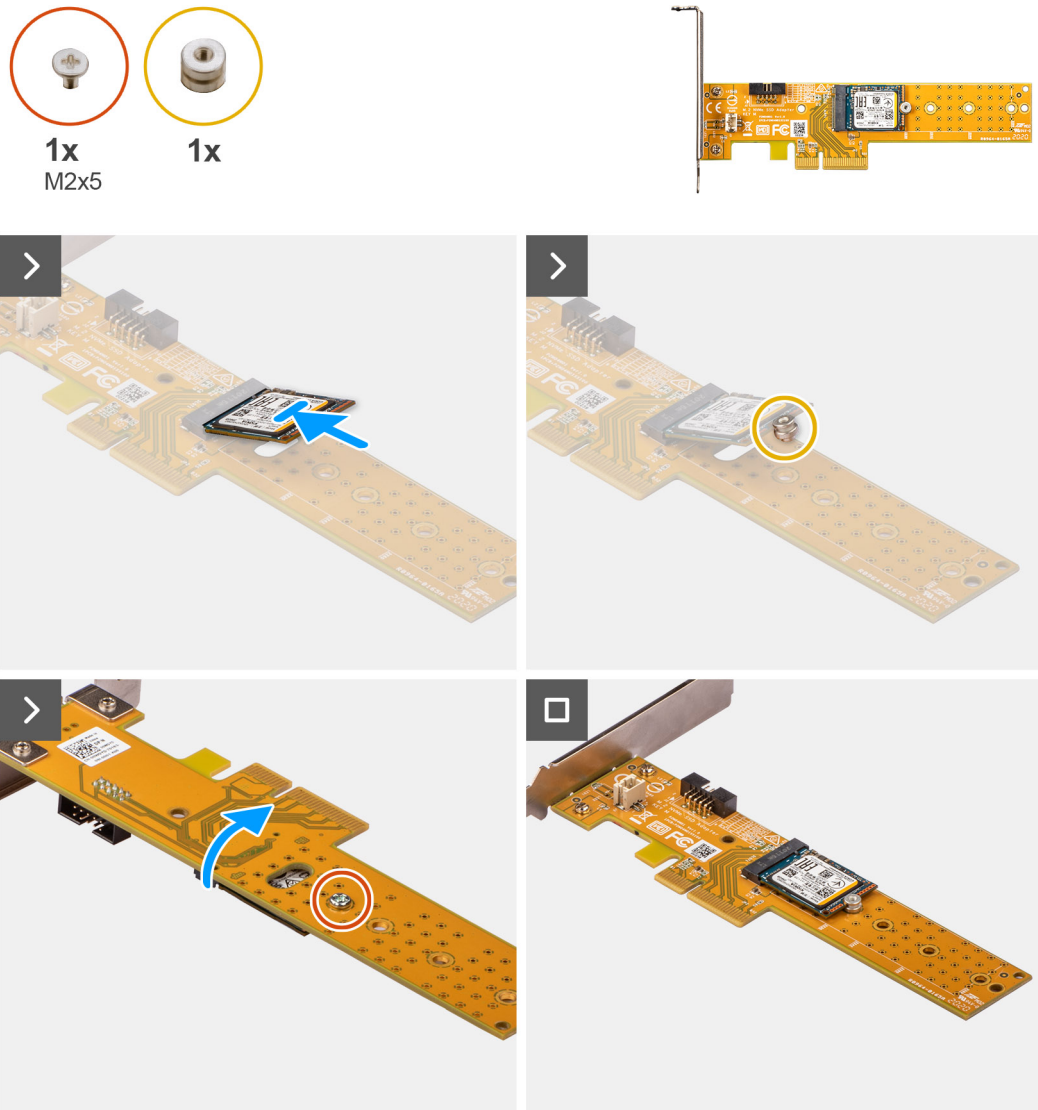
Figure 24. Installation du disque SSD M.2 2230 sur la carte Dell Ultra Speed Drive Gen 3
