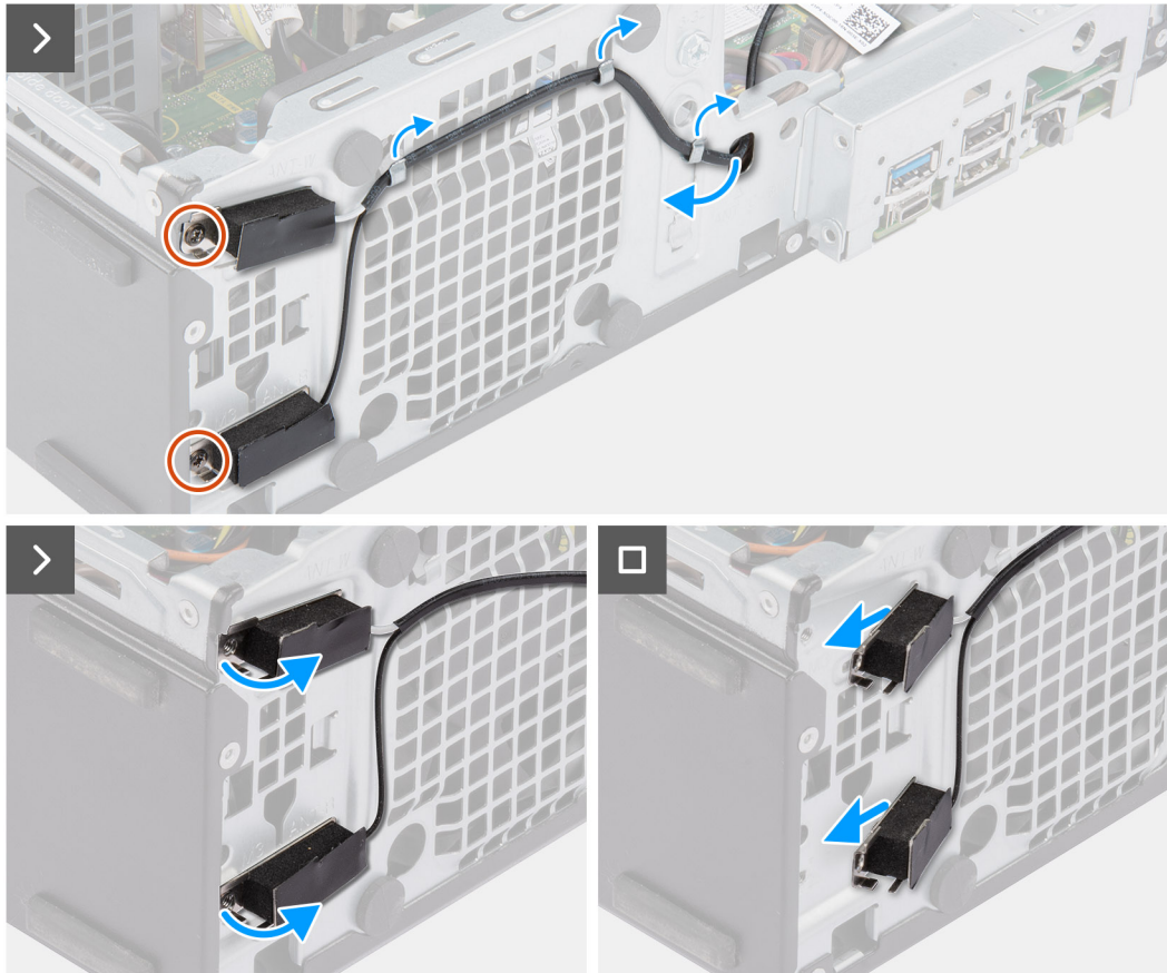
Figure 37. Retrait du module d'antenne interne
