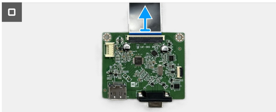
Schéma 21. Retrait de la carte d'interface
