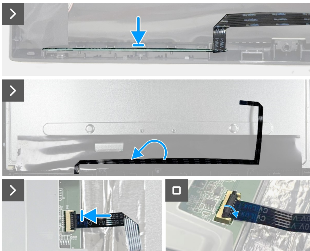
Schéma 15. Installation du clavier
