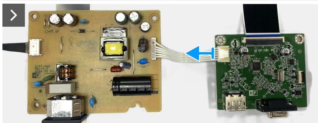
Schéma 20. Retrait de la carte d'interface
