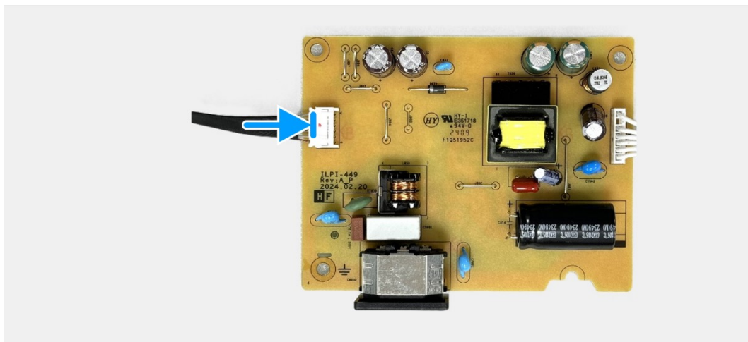
Schéma 25. Installation de la carte d'alimentation
