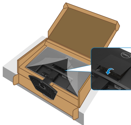
Abbildung 14. Installieren Sie die VESA-Abdeckung
