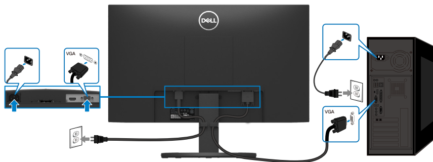
Abbildung 17. Anschließen des VGA-Kabels
