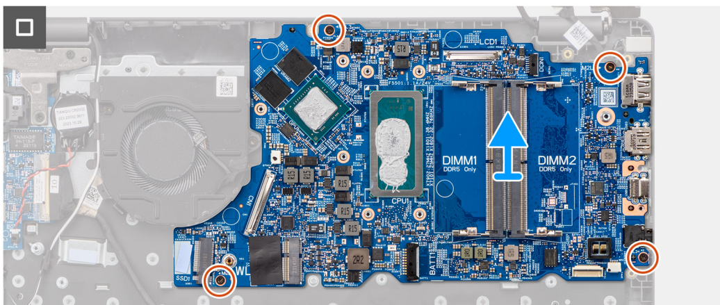
Figure 42. Retrait de la carte système
