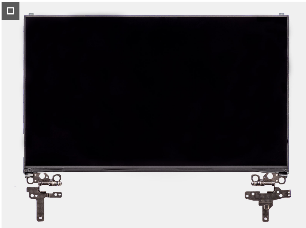
Figure 58. Retrait du panneau d'écran
