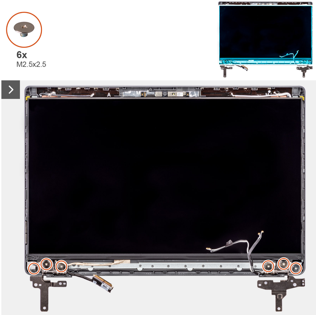
Figure 54. Retrait du panneau d'écran
