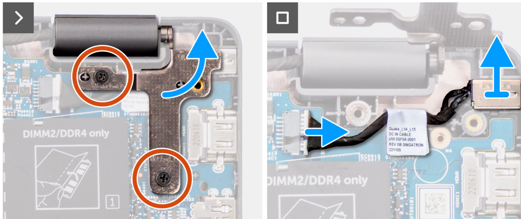
Figure 27. Retrait du port de l'adaptateur secteur
