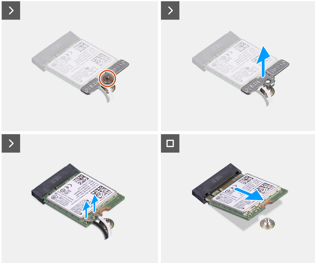
Figure 15. Retrait de la carte sans fil
