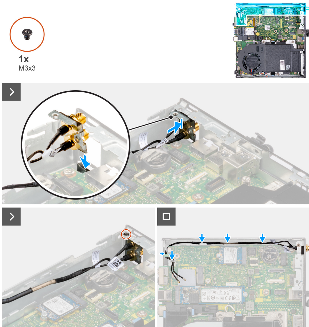
Ilustración 55. Instalación de la antena de SMA (ubicación 3)
