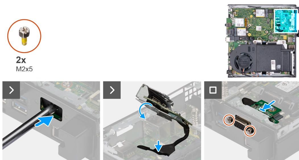
Ilustración 37. Instalación del módulo de I/O opcional (VGA o Serial)
