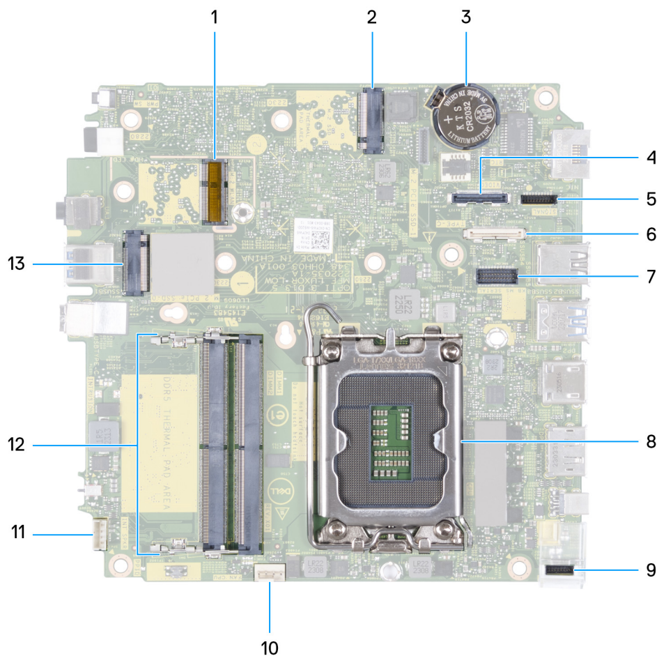
Ilustración 44. Imagen: conectores de la tarjeta madre
