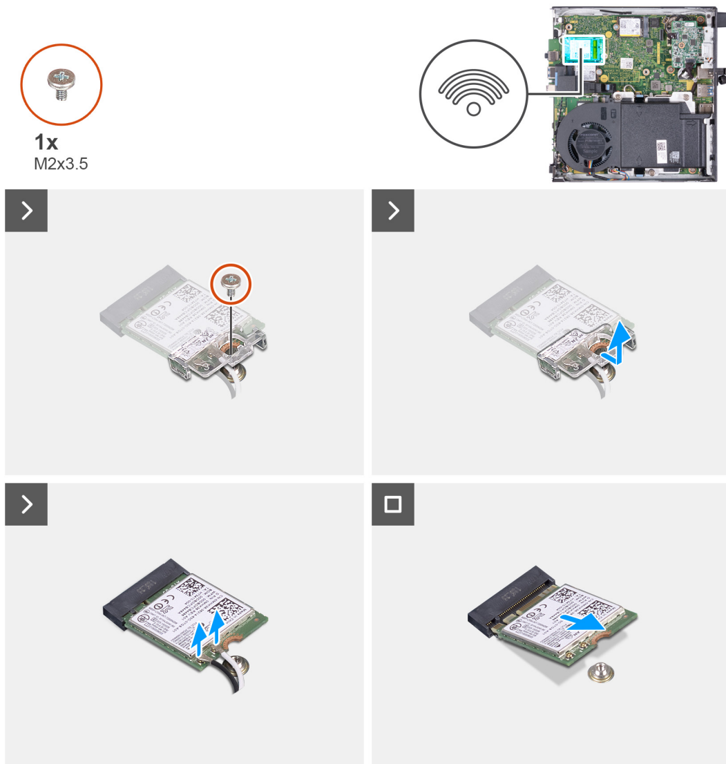
Ilustración 28. Extracción de la tarjeta inalámbrica
