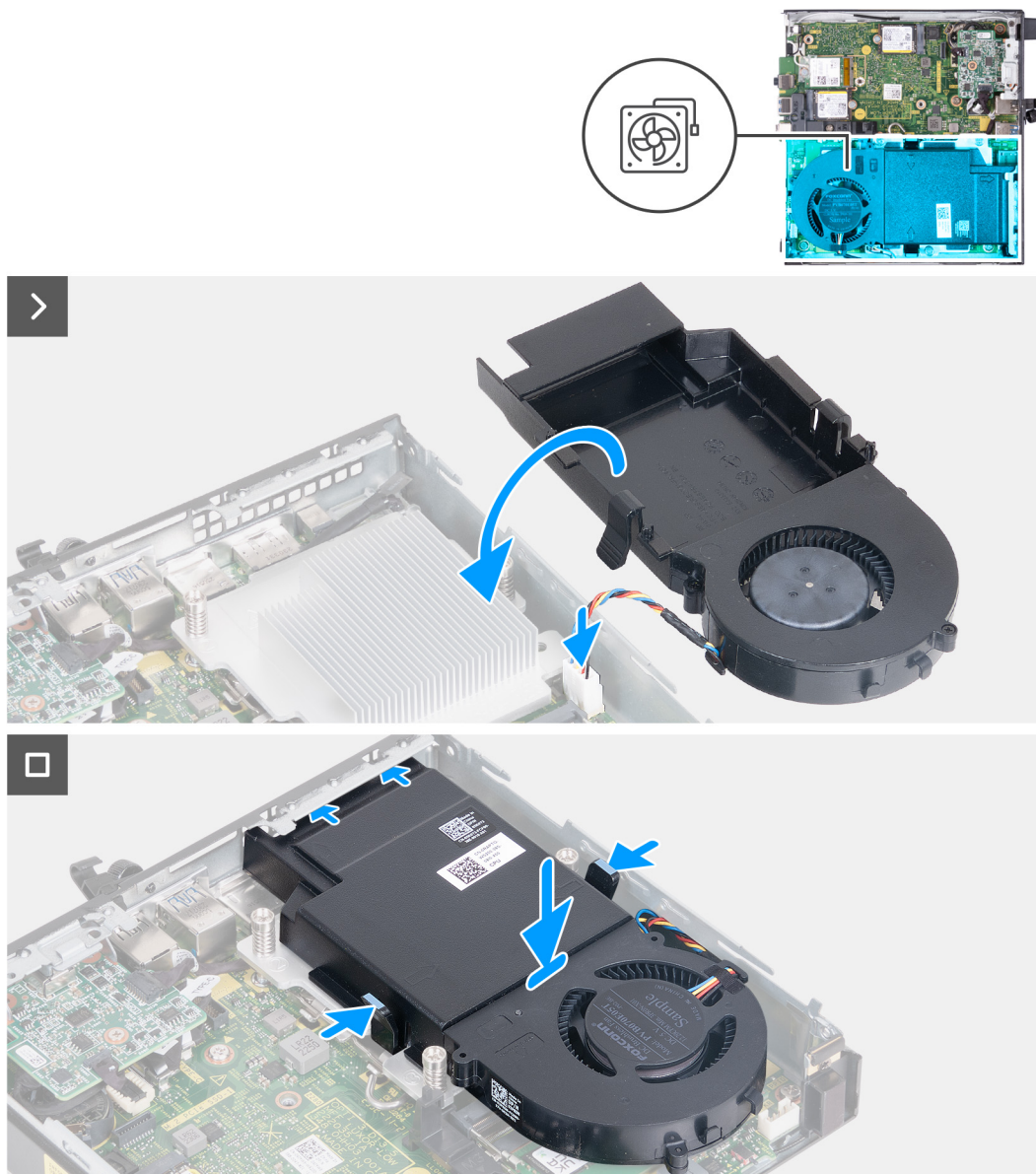
Ilustración 31. Instalación del ventilador
