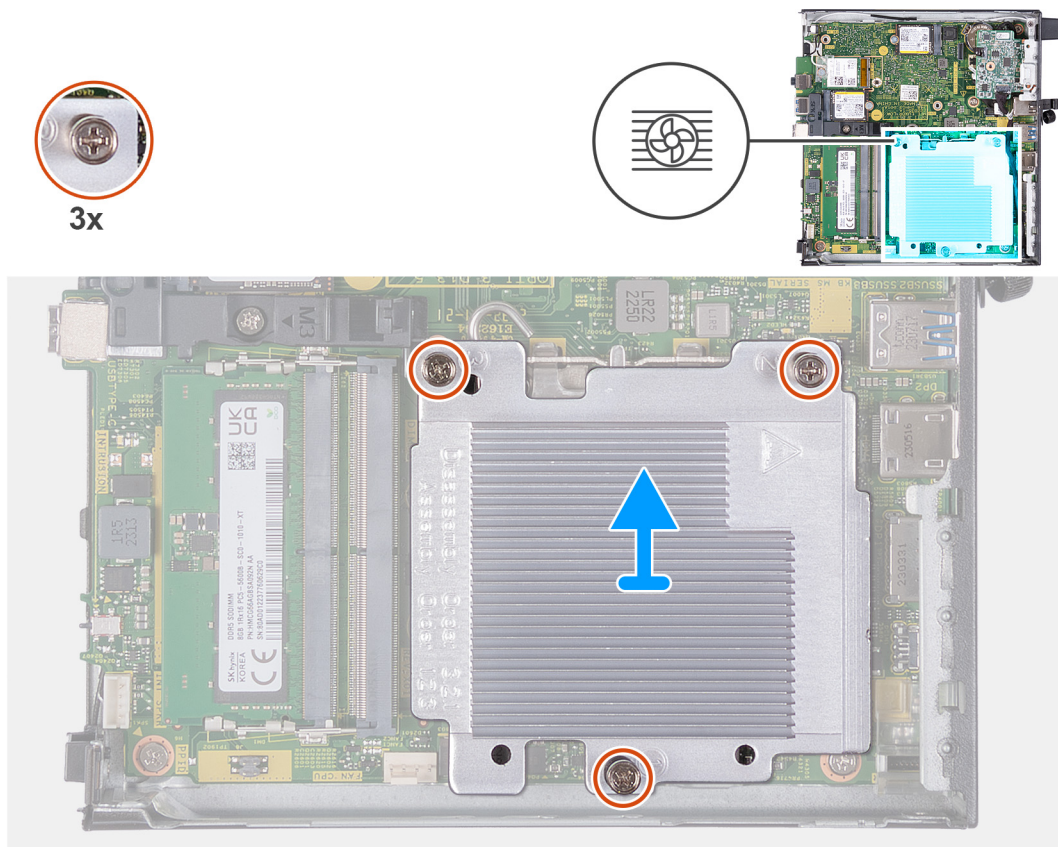
Ilustración 40. Extracción del disipador de calor
