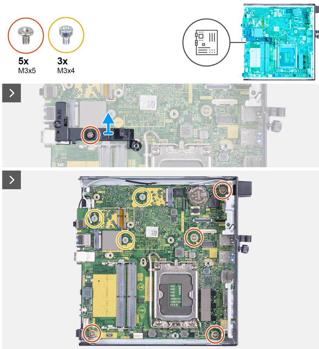
Ilustración 45. Extracción de la tarjeta madre
