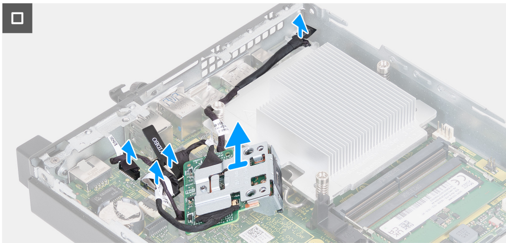
Ilustración 38. Extracción del módulo Type-C opcional
