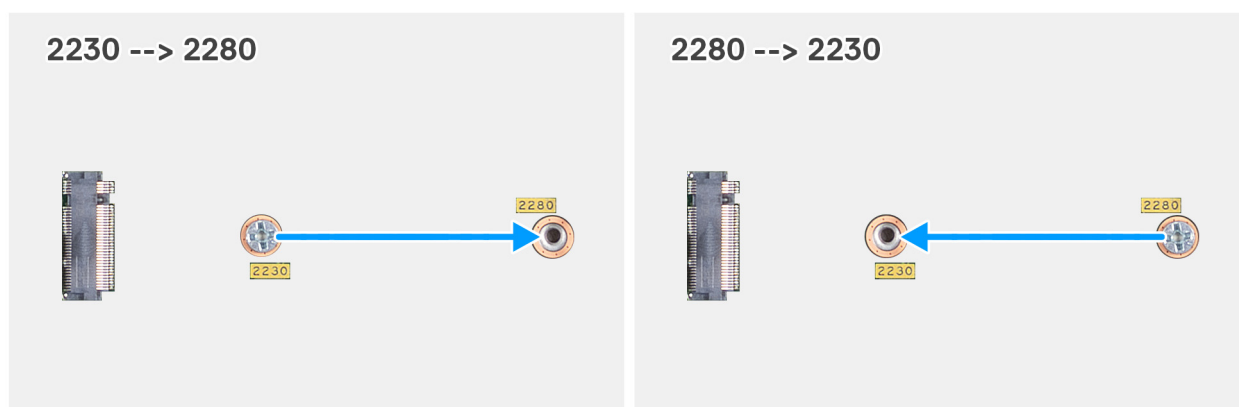
Ilustración 27. Movimiento del montaje de tornillos para admitir un factor de forma diferente (OptiPlex Micro 7020)
