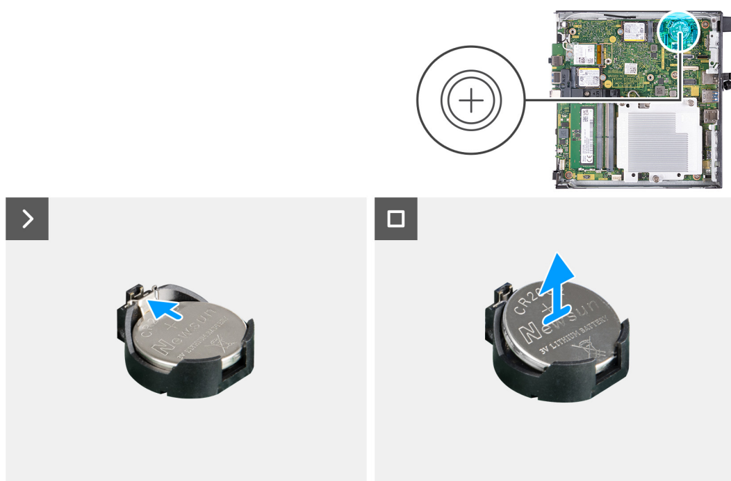
Ilustración 13. Extracción de la batería de tipo botón
