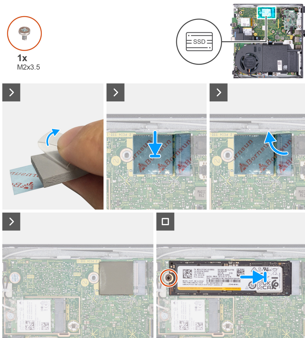
Ilustración 26. Instalación de la unidad de estado sólido M.2 2280 en la ranura 1
