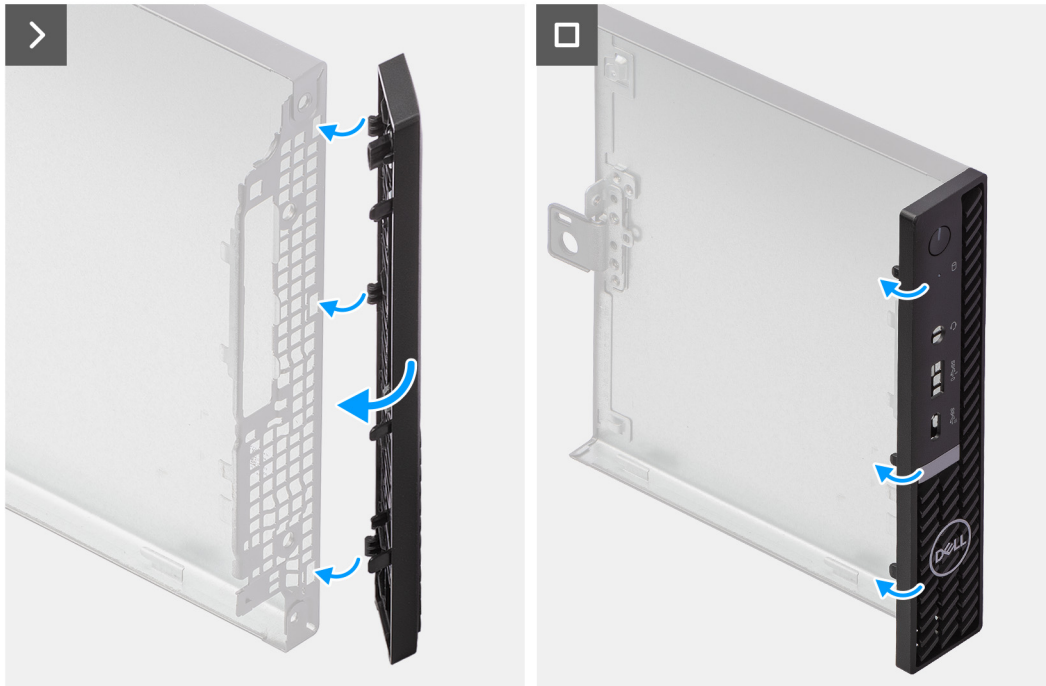
Ilustración 16. Instalación del bisel frontal
