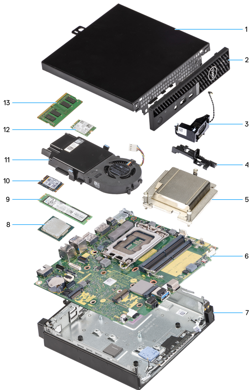
Ilustración 8. Componentes principales de la OptiPlex Micro 7020
