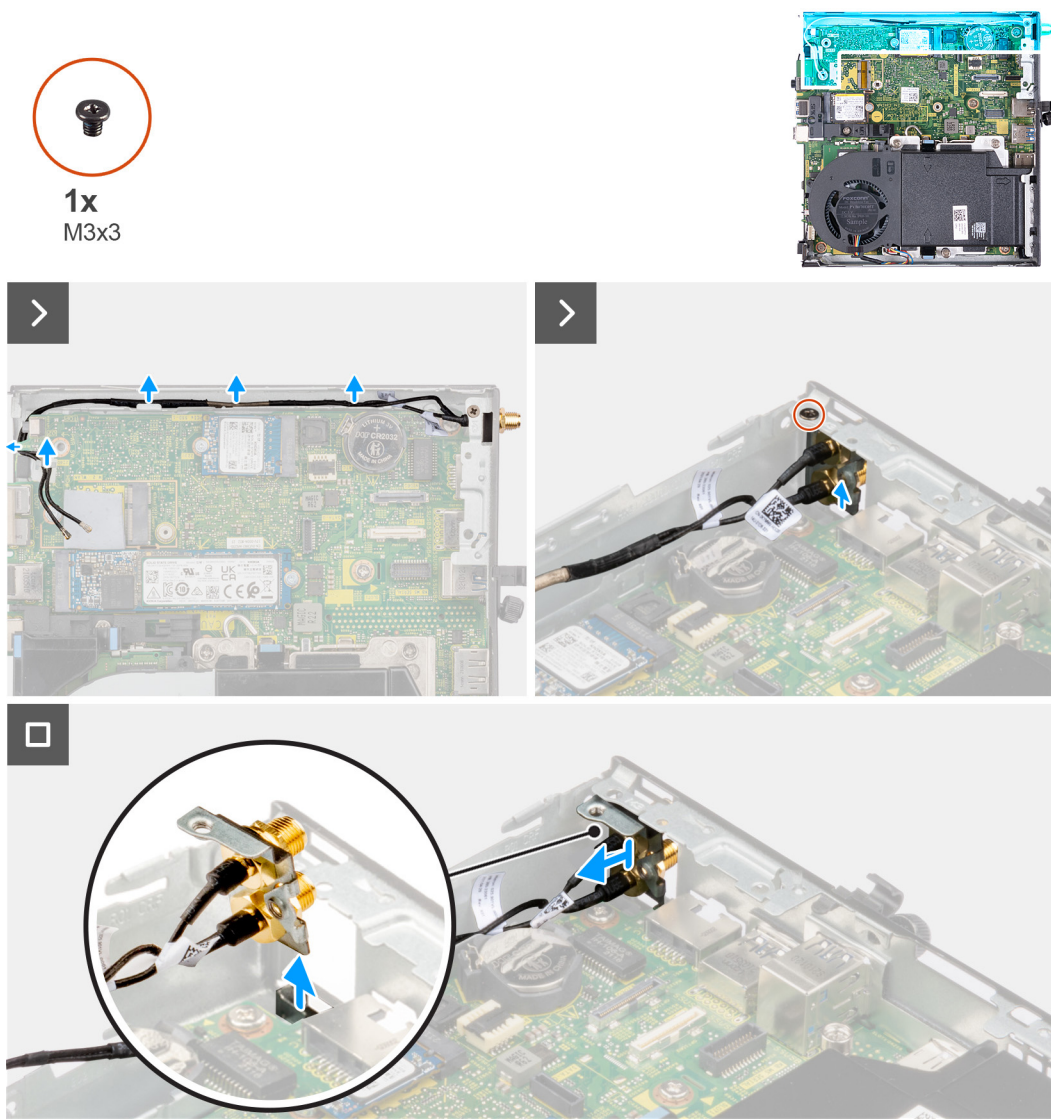
Ilustración 54. Extracción de la antena de SMA (ubicación 3)
