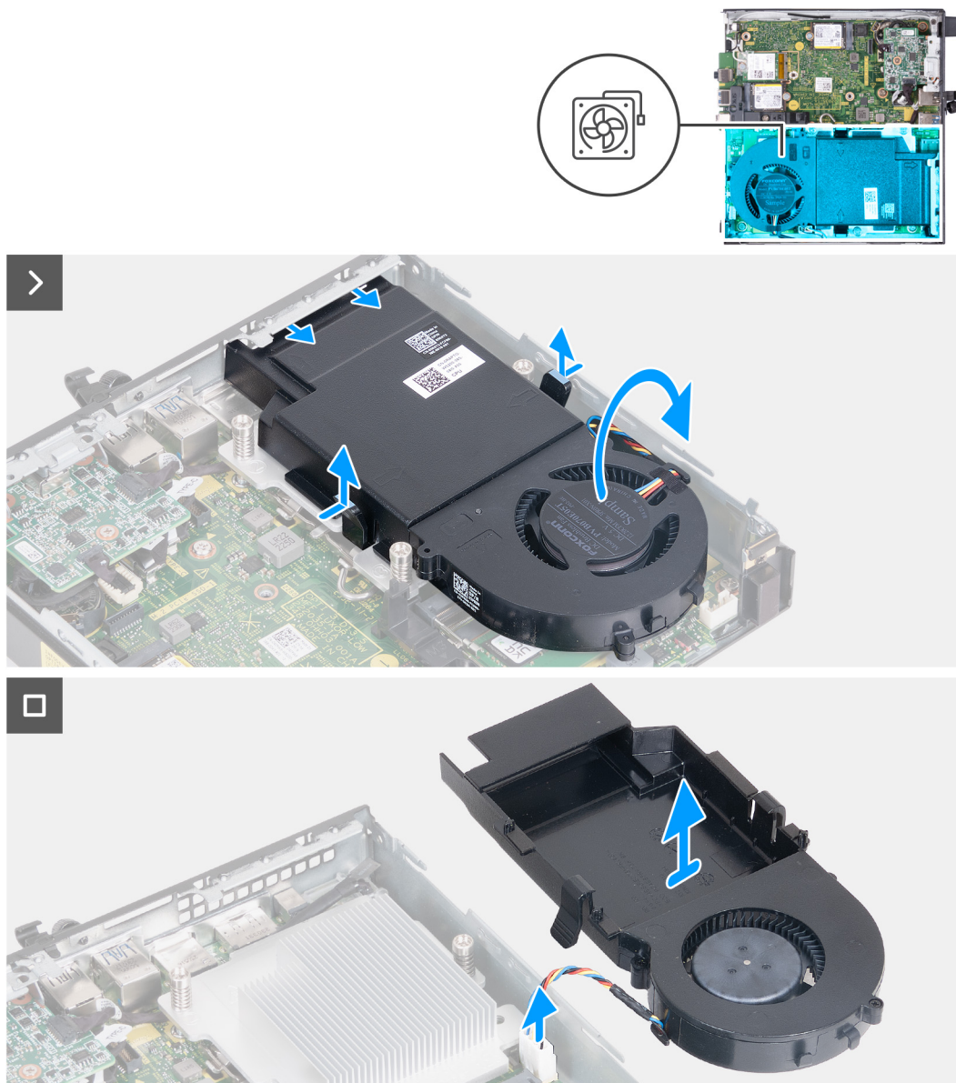
Ilustración 30. Extracción del ventilador
