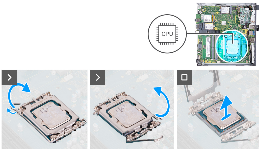
Ilustración 42. Extracción del procesador
