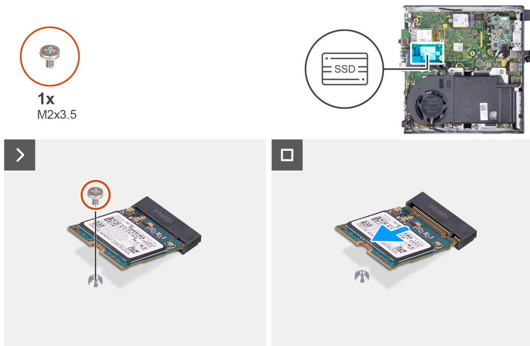
Ilustración 19. Extracción de la unidad de estado sólido 2230 de la ranura 0
