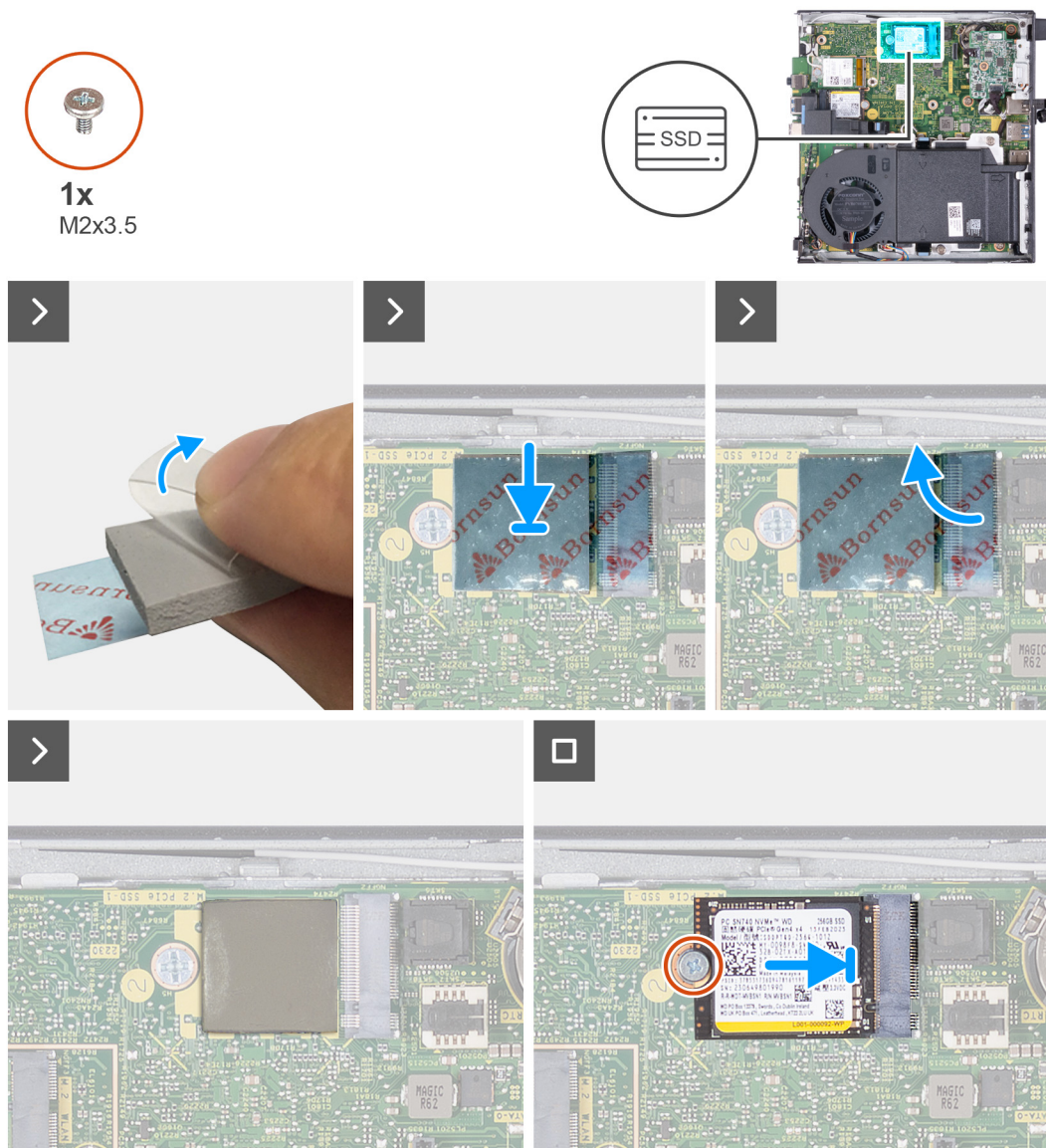
Ilustración 24. Instalación de la unidad de estado sólido M.2 2230 en la ranura 1
