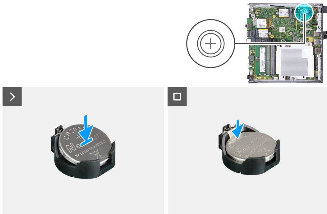
Ilustración 14. Instalación de la batería de tipo botón
