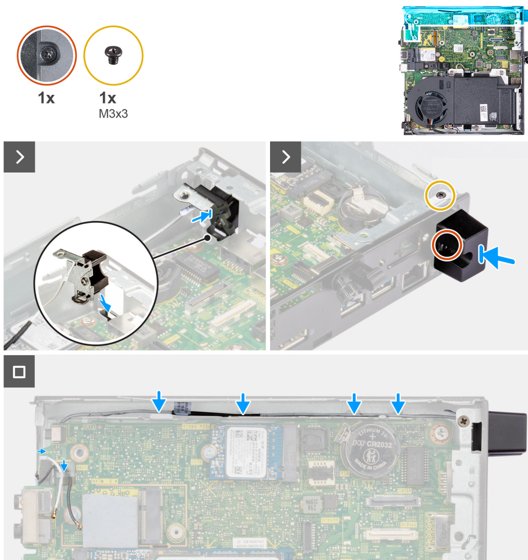
Ilustración 51. Instalación del módulo de la antena (cable blanco)
