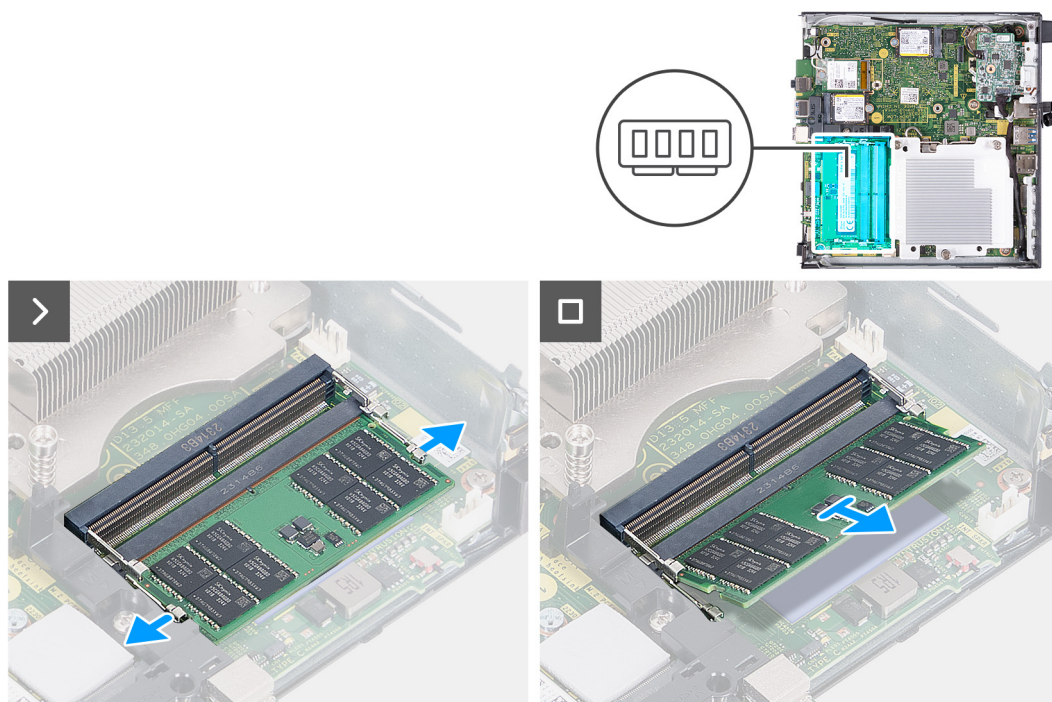
Ilustración 32. Extracción del módulo de memoria
