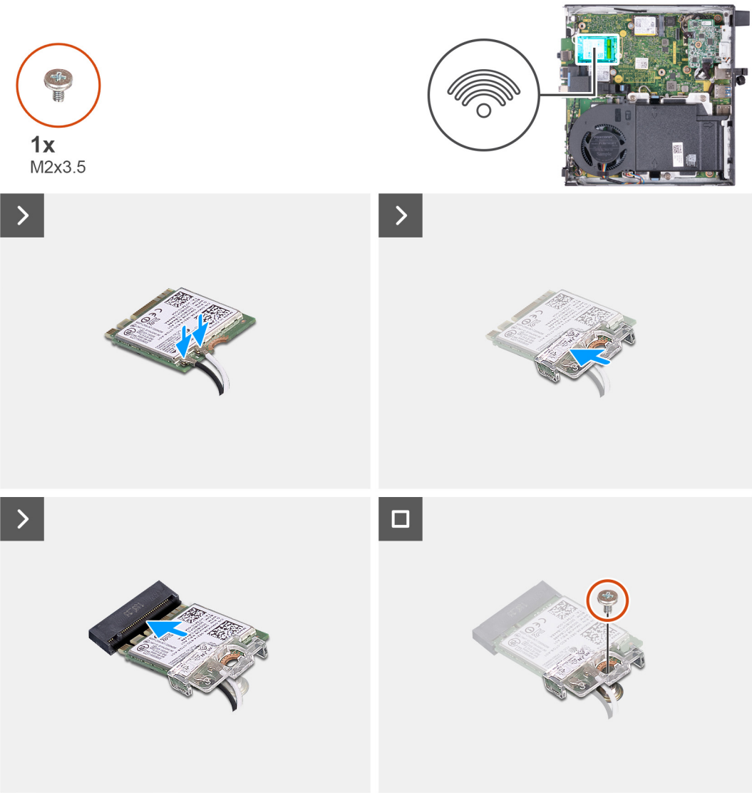
Ilustración 29. Instalación de la tarjeta inalámbrica
