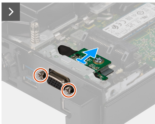
Ilustración 35. Extracción del módulo de I/O opcional (VGA o Serial)
