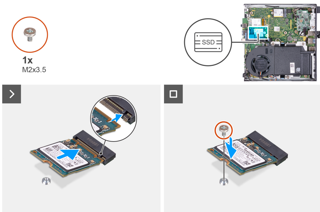
Ilustración 20. Instalación de la unidad de estado sólido 2230 en la ranura 0
