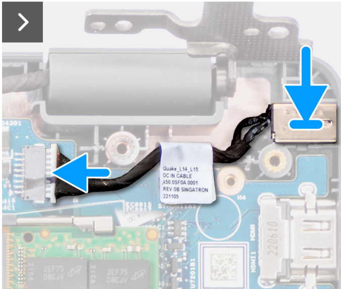
Ilustración 28. Instalación del puerto del adaptador de alimentación
