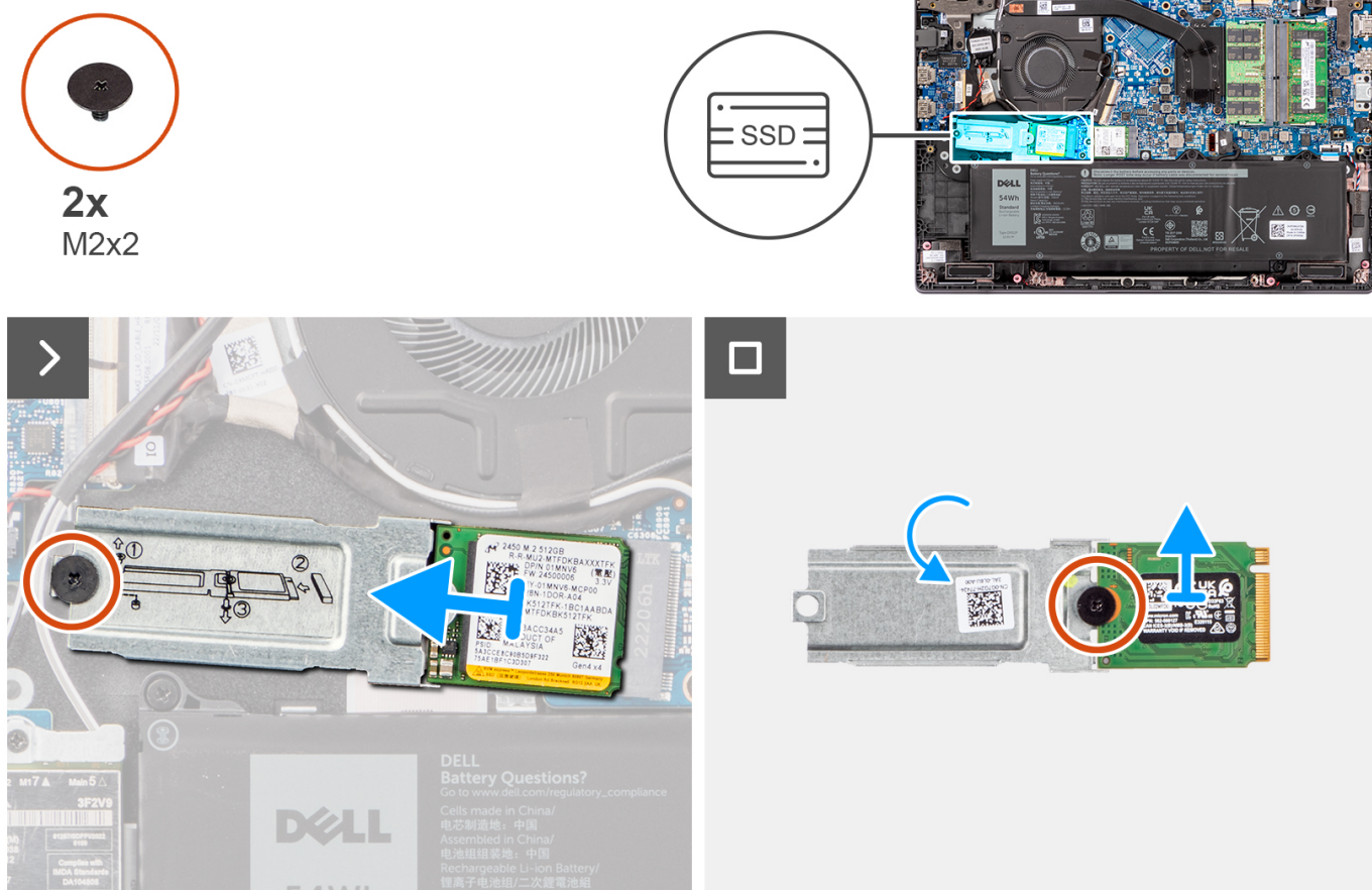
Ilustración 19. Extracción de la unidad de estado sólido M.2 2230
