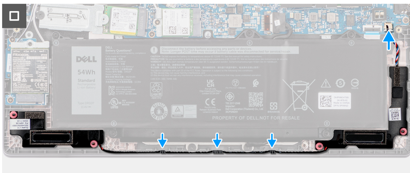
Ilustración 22. Instalación de los parlantes
