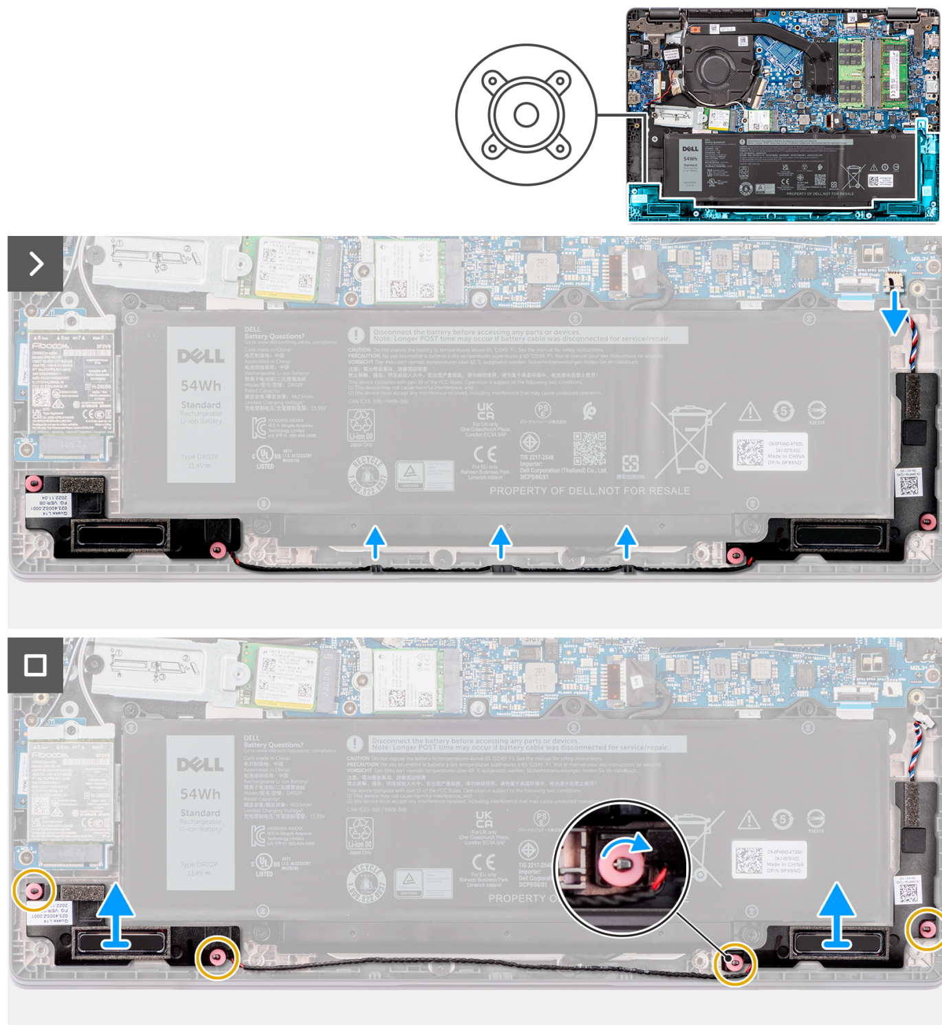
Ilustración 21. Extracción de los parlantes
