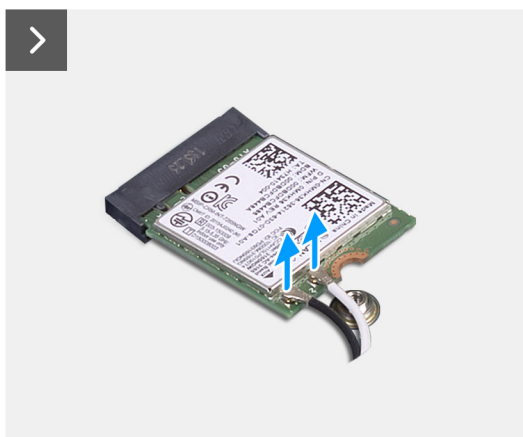
Ilustración 15. Extracción de la tarjeta inalámbrica
