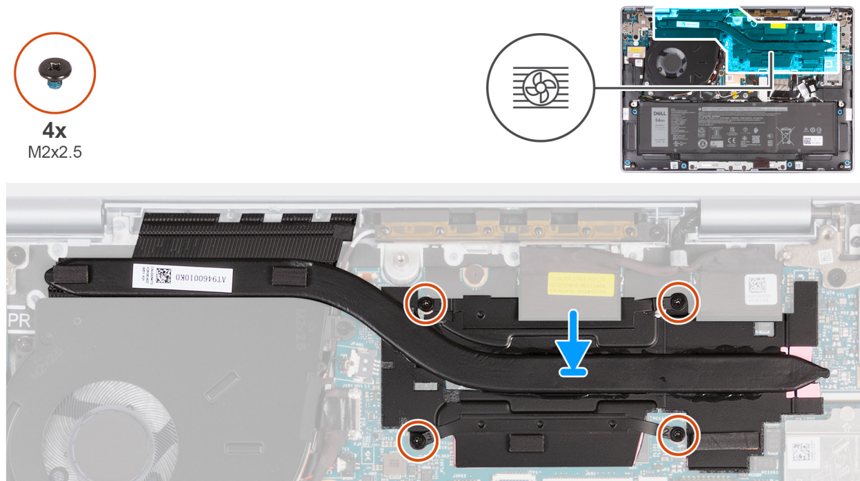
Figura 33. Installazione del dissipatore di calore
