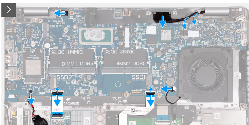
Afbeelding 54. De systeemkaartkabels loskoppelen
