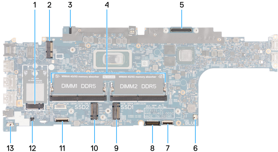
Afbeelding 52. Systeemkaartconnectoren
