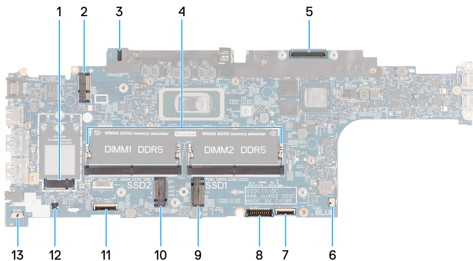
Afbeelding 57. Systeemkaartconnectoren
