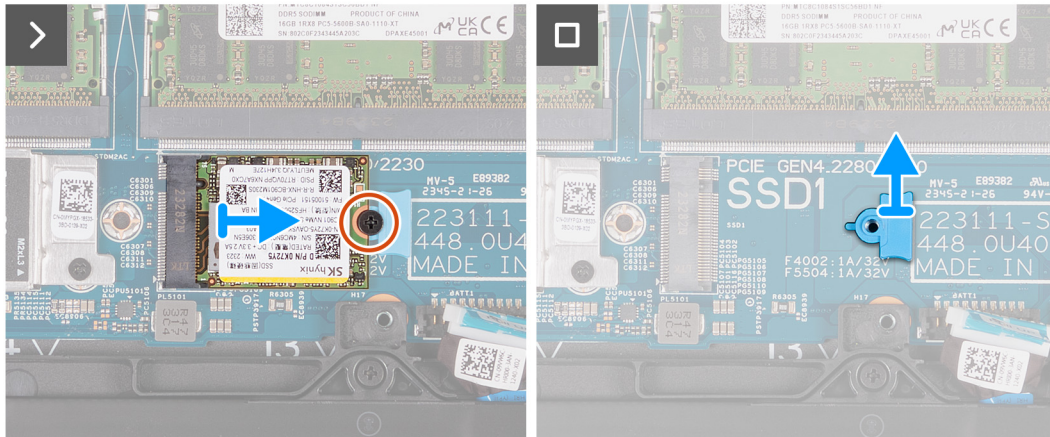
Afbeelding 27. De M.2 2230 SSD verwijderen uit slot 1
