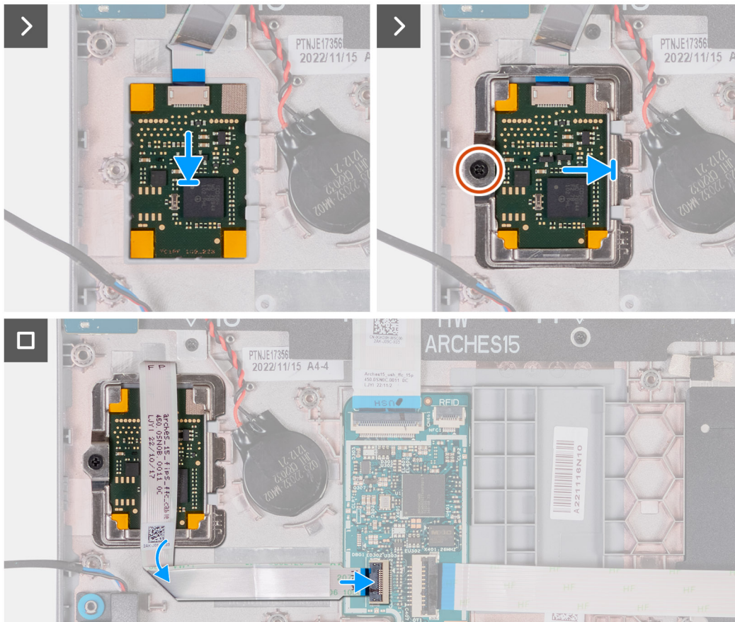
Afbeelding 95. De vingerafdruklezer plaatsen
