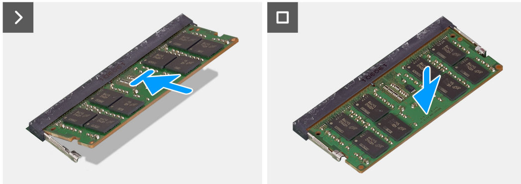
Afbeelding 26. De geheugenmodule plaatsen
