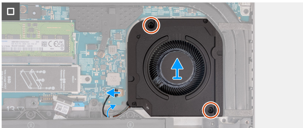
Afbeelding 33. De ventilator verwijderen
