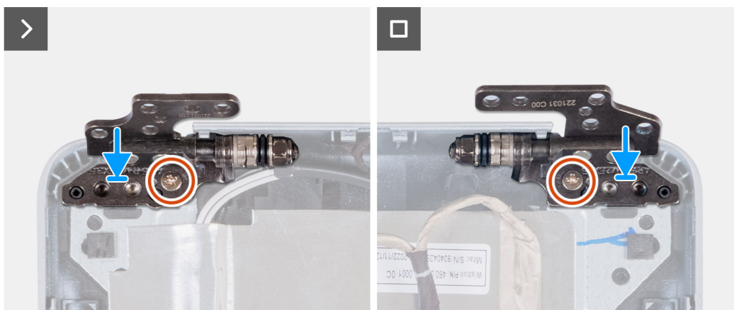
Afbeelding 87. De beeldschermcharnieren installeren
