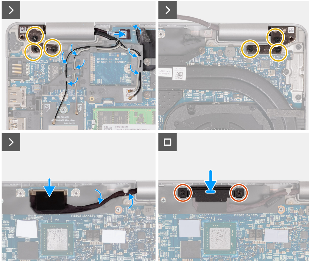
Afbeelding 73. De beeldschermenunit plaatsen
