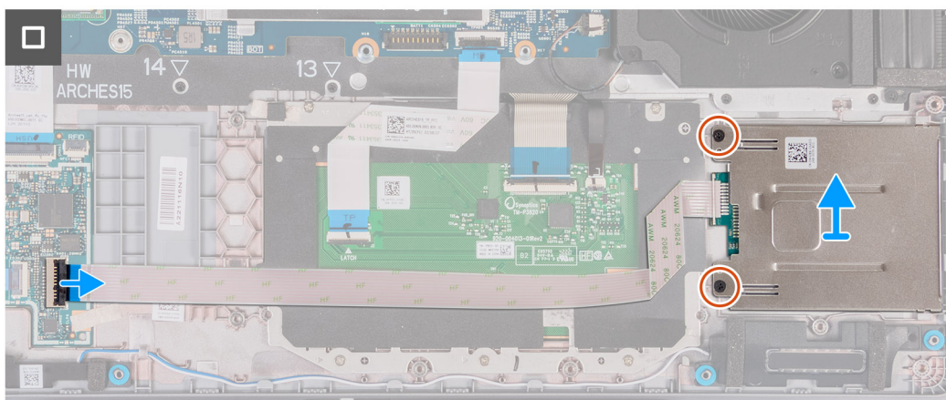
Afbeelding 96. De smartcardlezer verwijderen
