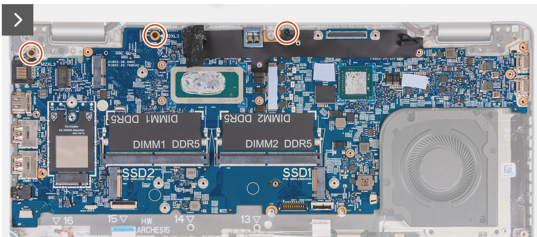
Afbeelding 58. De systeemkaart installeren
