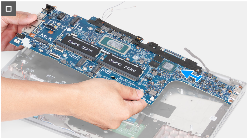
Afbeelding 56. De systeemkaart verwijderen
