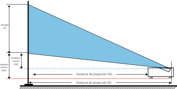
• Di: distancia desde el borde de la unidad hasta la pantalla • D: distancia desde la lente hasta la pantalla • Hd: altura desde el centro de la lente hasta la parte inferior de la pantalla • Hd2: altura desde la superficie de montaje del proyector hasta la parte inferior de la pantalla
