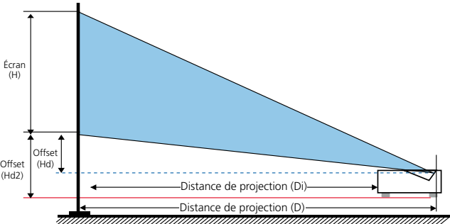
• Di : distance entre le bord de l'appareil et l'écran • D : distance entre l'objectif et l'écran • Hd : hauteur entre le centre de l'objectif et le bas de l'écran • Hd2 : hauteur entre la surface de montage du projecteur et le bas de l'écran
