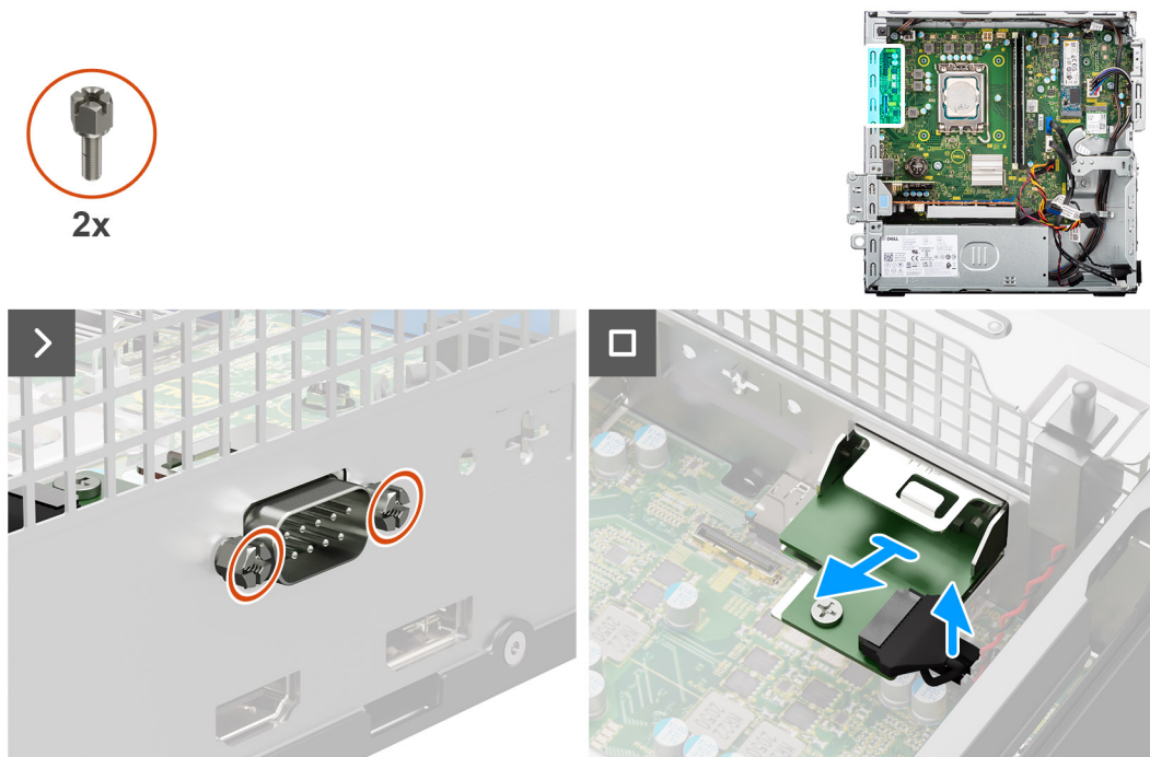
Figur 48. Ta bort den seriella modulen
