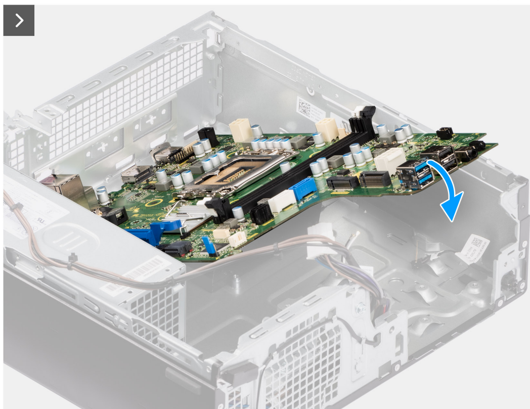
Figur 62. Installera moderkortet
