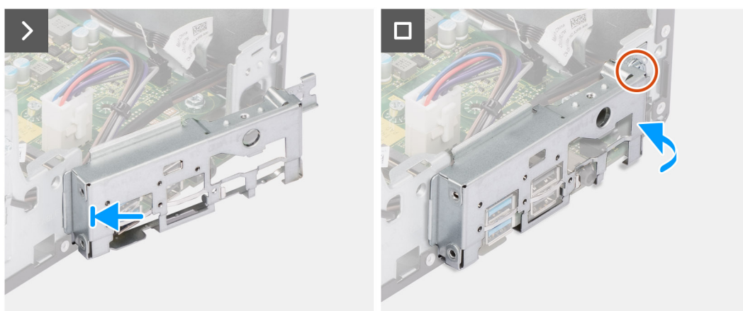
Figur 65. Installera moderkortet
