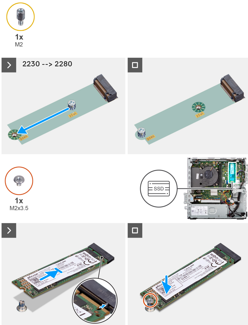
Figur 20. Installera M.2 2280 SSD-disken
