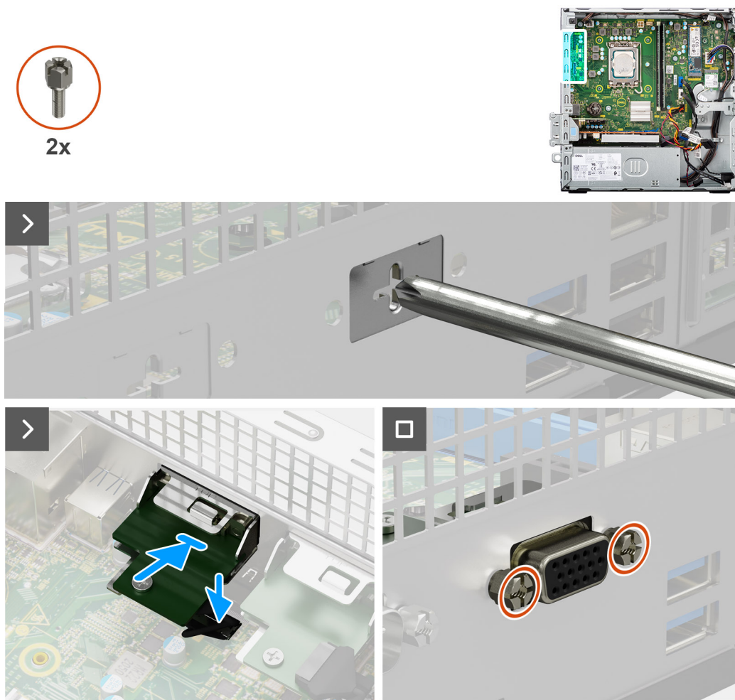
Figur 51. Installera VGA-modulen
