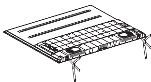
Винты: M6 × 35 мм × 4 шт.
