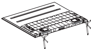
Parafusos: M6 x 35 mm x 4pçs
