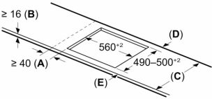
Afmeting in mm
