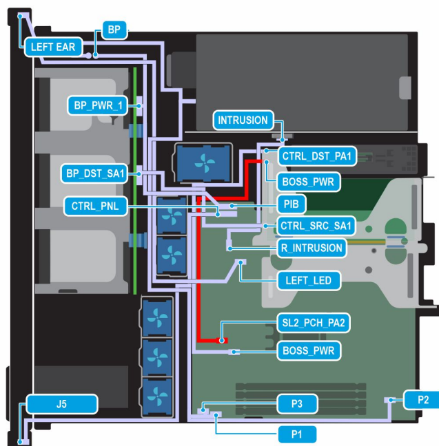
Ilustración 43. Configuración 4: seis unidades SAS/SATA de 2,5 pulgadas con PSU cableada y BOSS-N1 (opcional)
