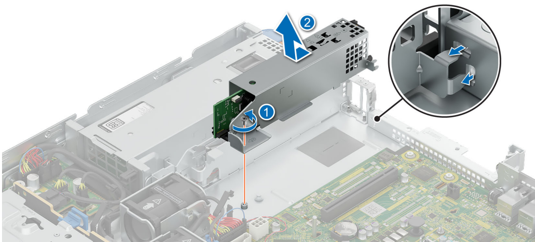
Ilustración 72. Extracción de la canastilla para BOSS-N1
