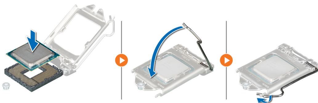
Ilustración 58. Instalación del procesador
