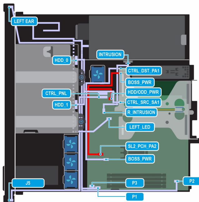
Ilustración 41. Configuración 2: dos unidades PERC SAS/SATA de 3,5 pulgadas, sin backplane con PSU cableada y BOSS-N1 (opcional)
