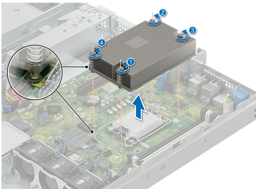
Ilustración 56. Extracción del módulo del disipador de calor
