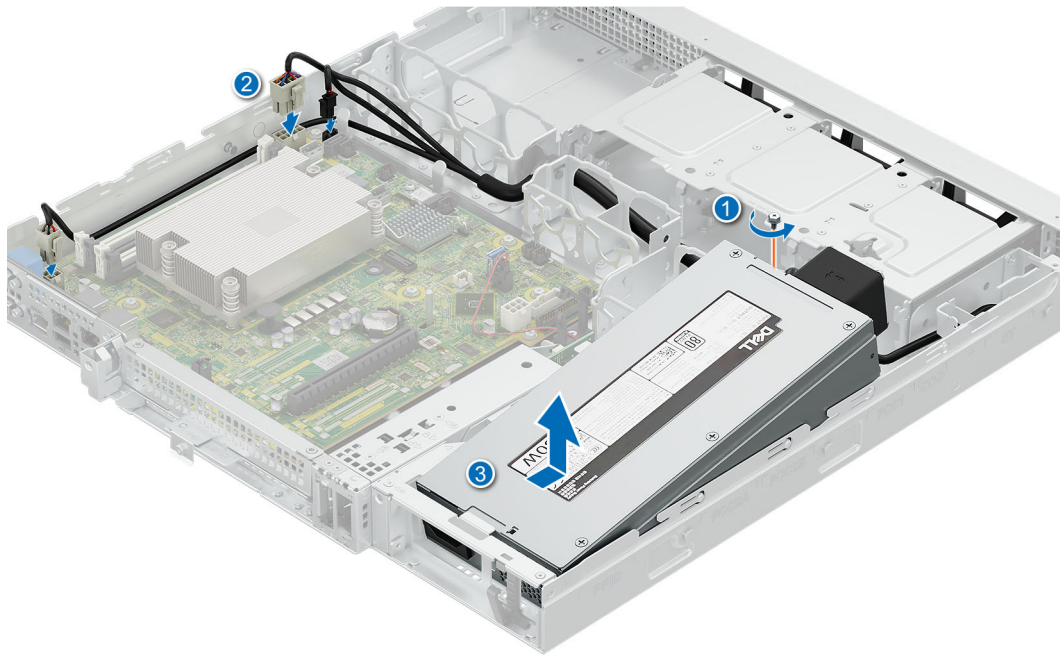
Ilustración 83. Extracción de una unidad de fuente de alimentación cableada
