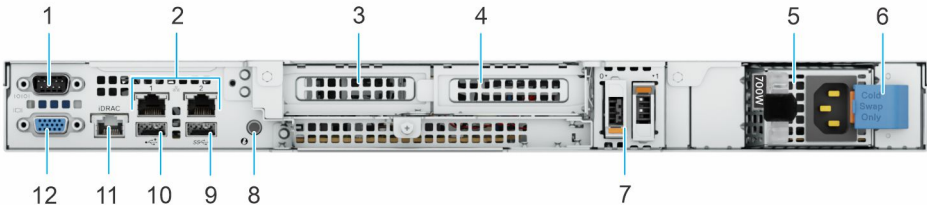
Ilustración 5. Vista posterior del sistema con PSU no cableada
