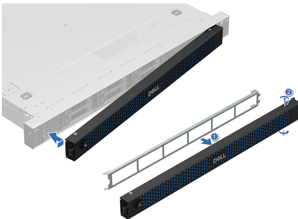
Ilustración 97. Instalación del bisel del filtro
