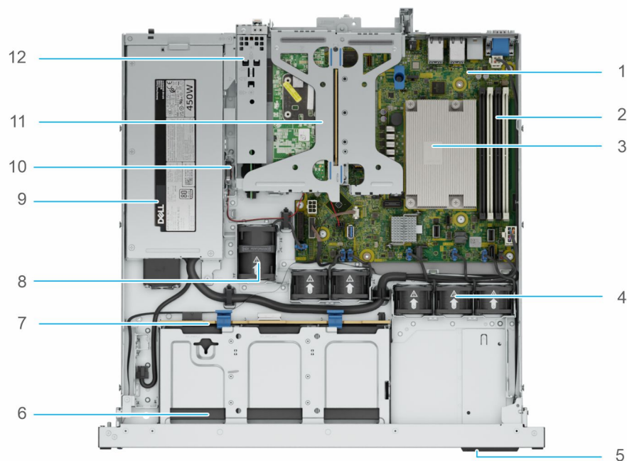
Ilustración 9. Vista interior del sistema con PSU cableada y unidades de 2,5 pulgadas sin cubierta para flujo de aire
