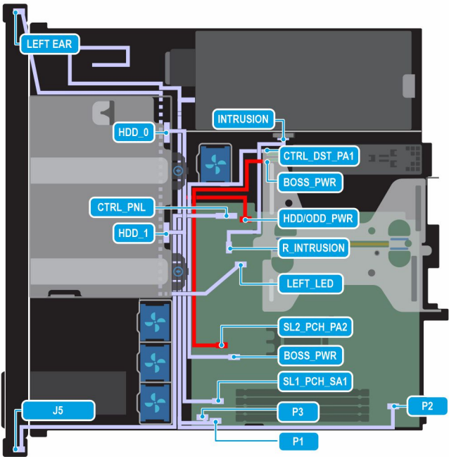
Ilustración 39. Configuración 0: dos unidades SATA de 3,5 pulgadas, sin backplane con PSU cableada y BOSS-N1 (opcional)
