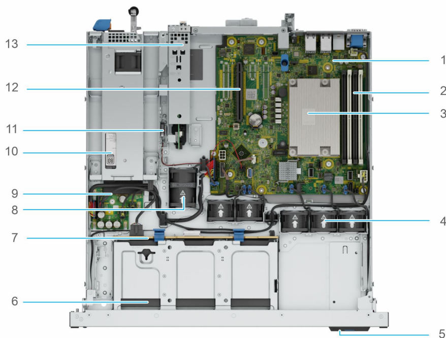
Ilustración 8. Vista interior del sistema con PSU no cableada y unidades de 2,5 pulgadas sin cubierta para flujo de aire y tarjeta elevadora
