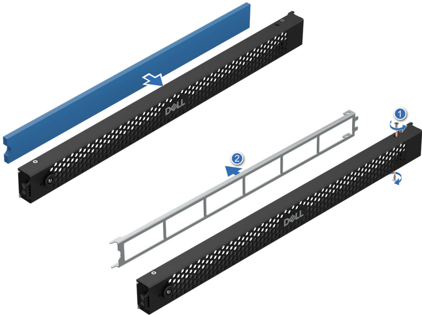
Ilustración 96. Instalación del filtro
