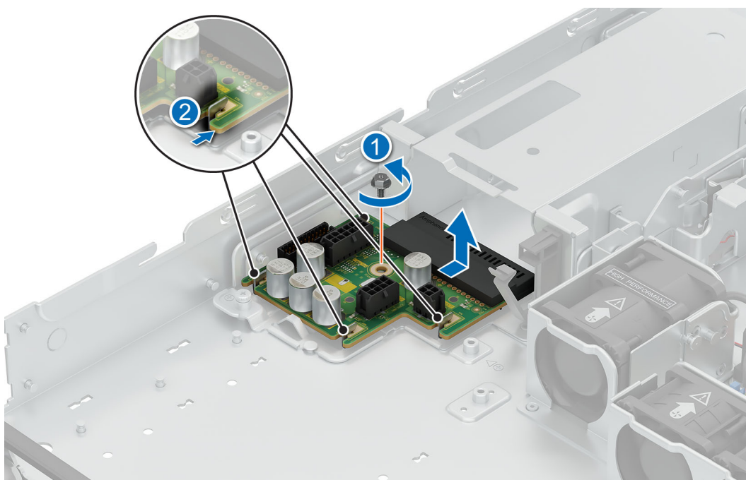
Ilustración 87. Extracción de la PIB
