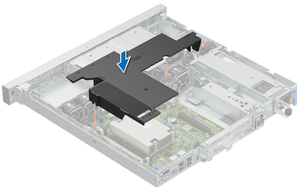
Ilustración 30. Instalación de la cubierta para flujo de aire para la configuración de unidades de 3,5 pulgadas
