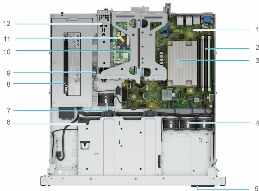
Ilustración 12. Vista interior del sistema con PSU cableada y unidades de 3,5 pulgadas sin cubierta para flujo de aire
