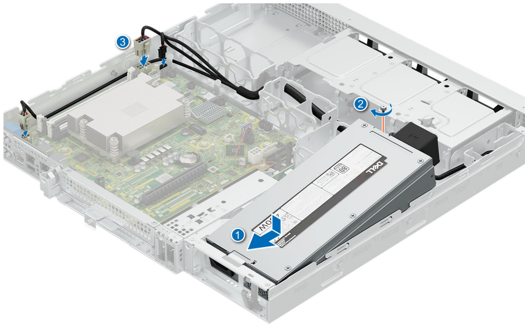
Ilustración 84. Instalación de una fuente de alimentación cableada (PSU)
