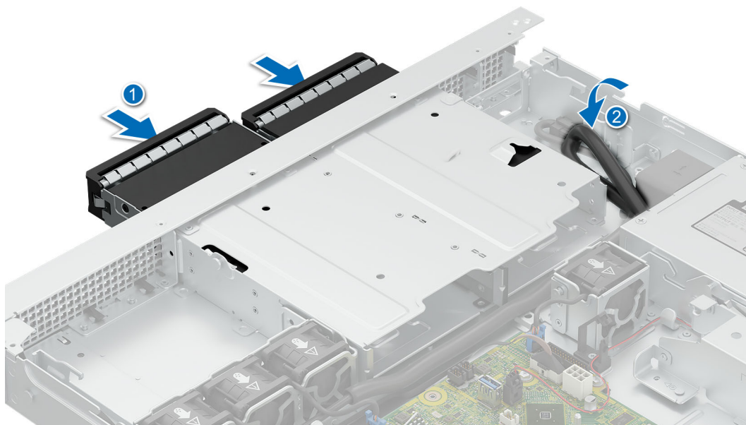
Ilustración 52. Instalación de un disco duro cableado de 3,5 pulgadas
