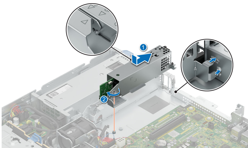
Ilustración 76. Instalación de la canastilla para BOSS-N1
