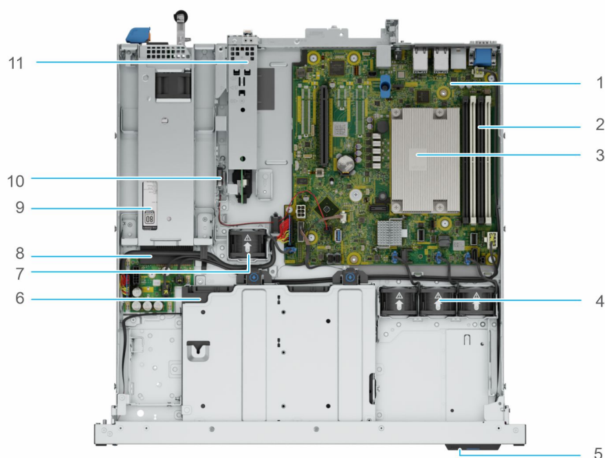
Ilustración 11. Vista interior del sistema con PSU no cableada y unidades de 3,5 pulgadas con cubierta para flujo de aire y tarjeta elevadora
