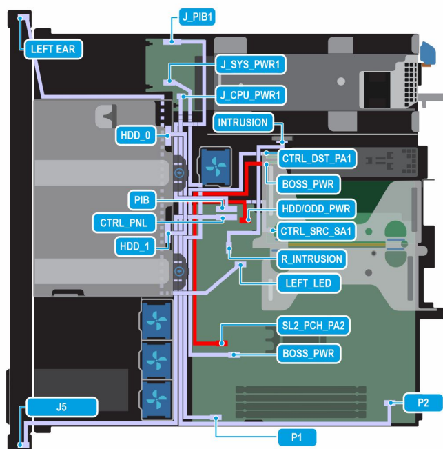
Ilustración 42. Configuración 3: dos unidades PERC SAS/SATA de 3,5 pulgadas, sin backplane con PSU no cableada y BOSS-N1 (opcional)
