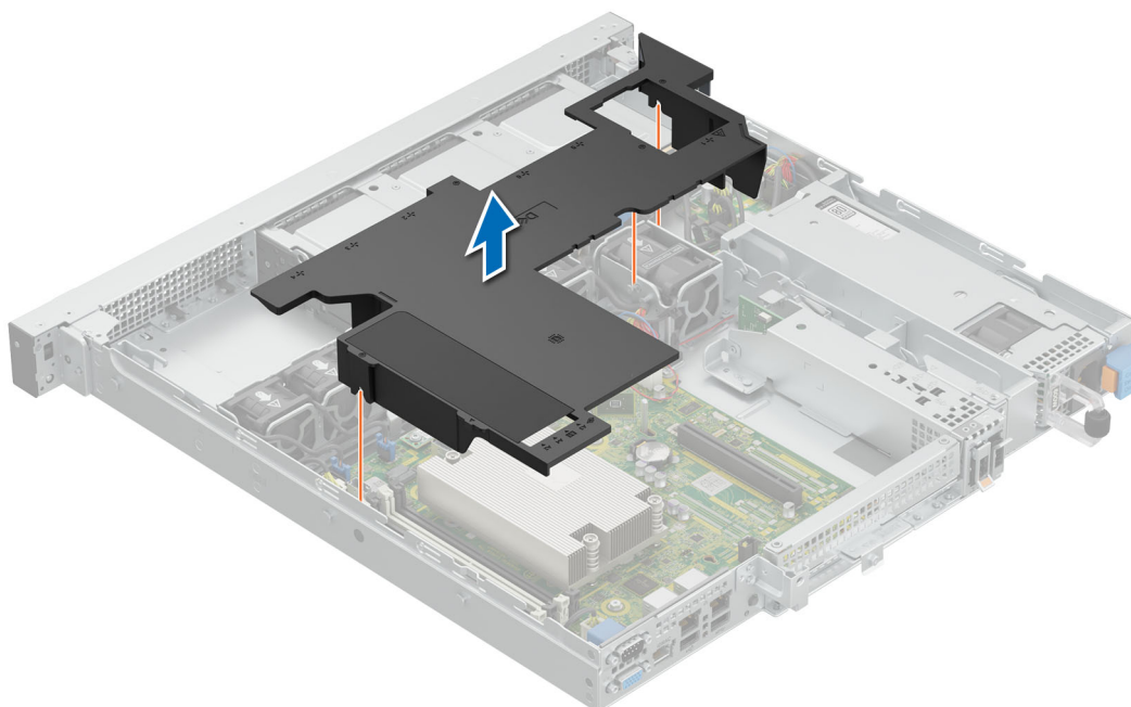
Ilustración 27. Extracción de la cubierta para flujo de aire para la configuración de unidades de 2,5 pulgadas
