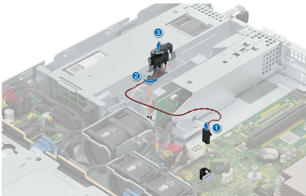
Ilustración 34. Extracción del interruptor de intrusiones
