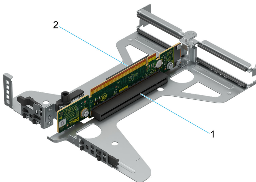
Ilustración 63. Tarjeta elevadora de mariposa
