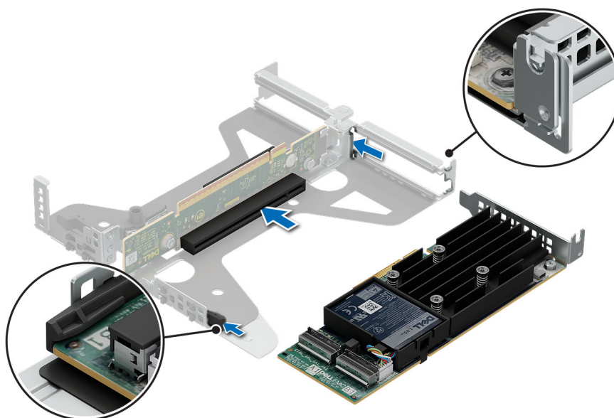
Ilustración 67. Instalación de una tarjeta de expansión en la tarjeta elevadora
