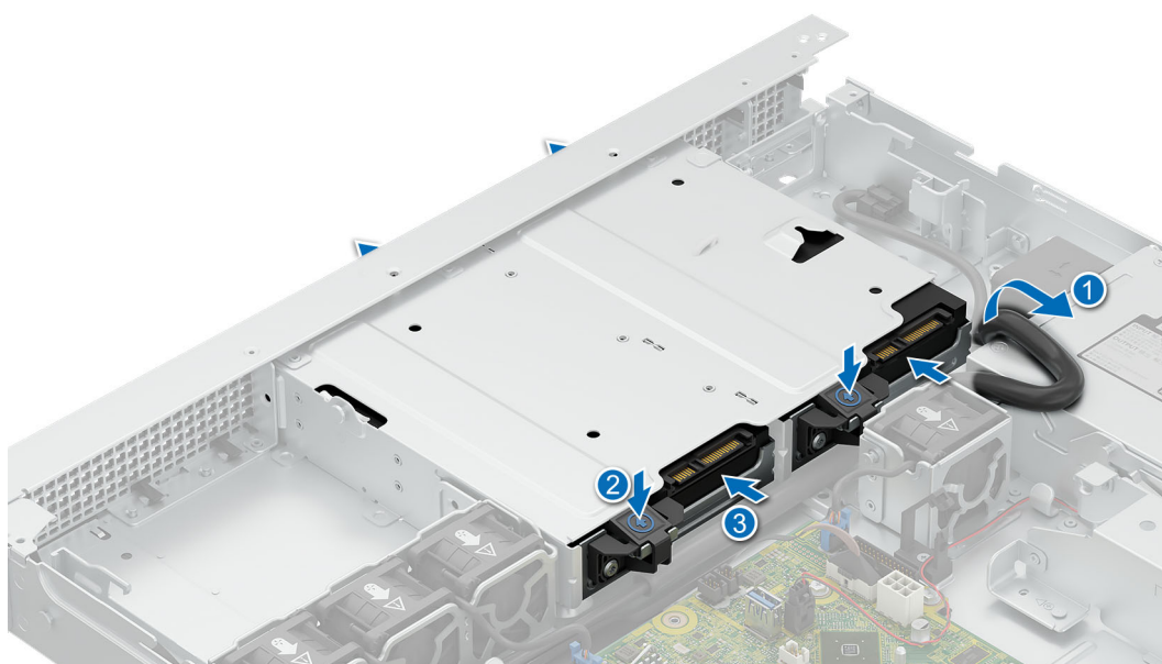
Ilustración 51. Extracción del disco duro cableado de 3,5 pulgadas
