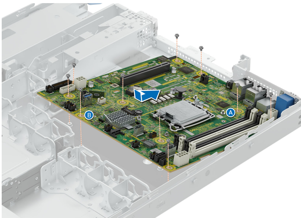
Ilustración 90. Instalación de la tarjeta madre
