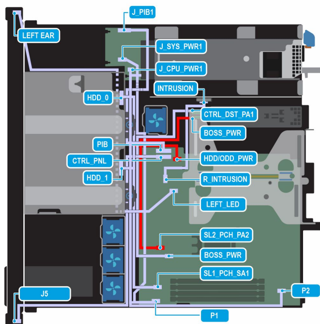
Ilustración 40. Configuración 1: dos unidades SATA de 3,5 pulgadas, sin backplane con PSU no cableada y BOSS-N1 (opcional)
