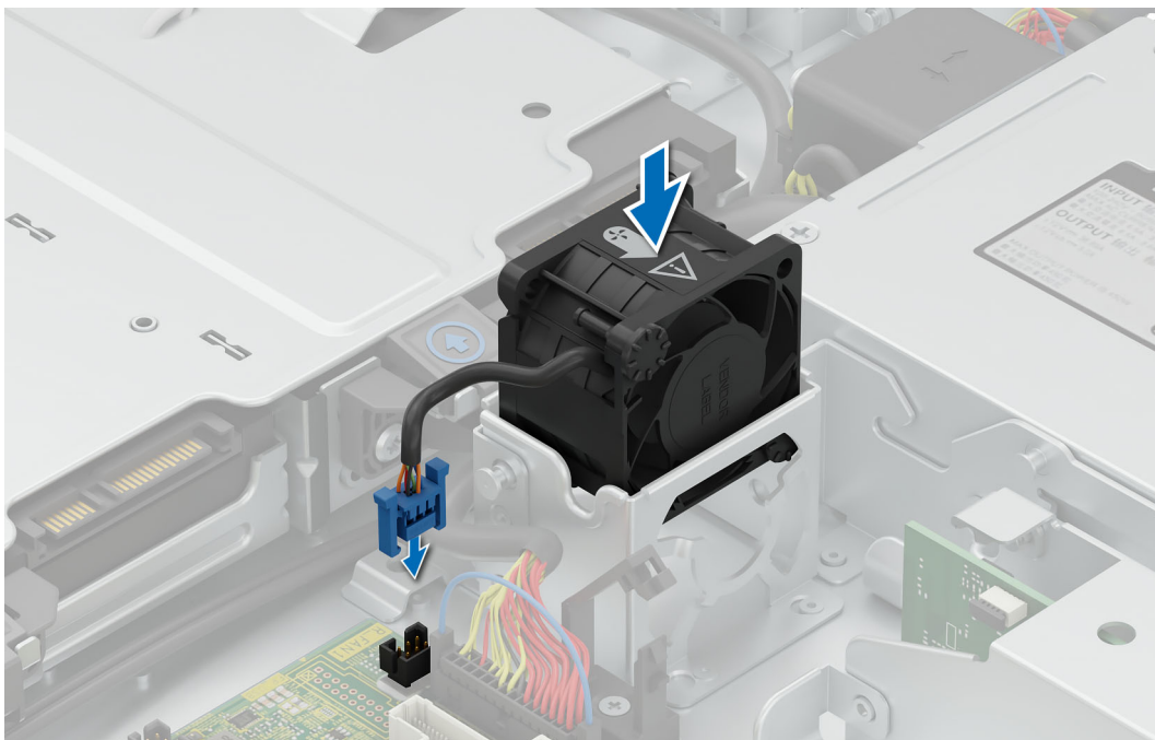
Ilustración 33. Instalación del ventilador para BOSS-N1 o tarjeta elevadora PCIe
