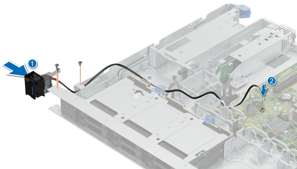
Ilustración 95. Instalación del panel de control izquierdo
