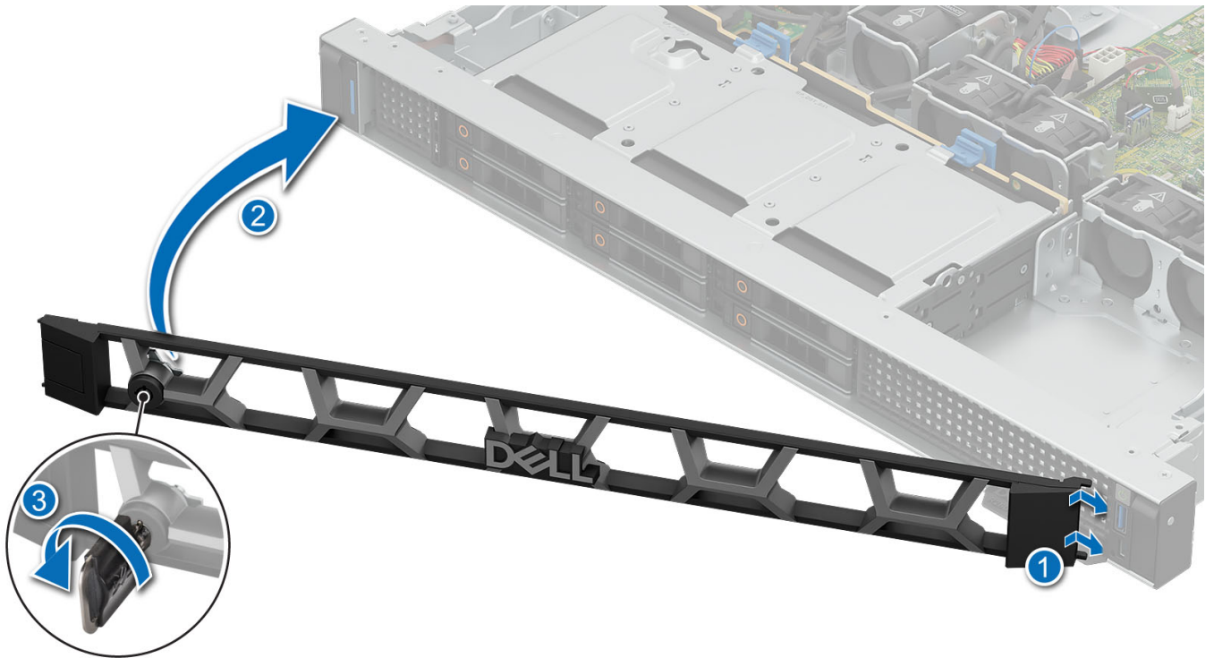
Ilustración 24. Instalación del bisel frontal
