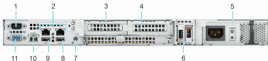
Ilustración 6. Vista posterior del sistema con PSU cableada
