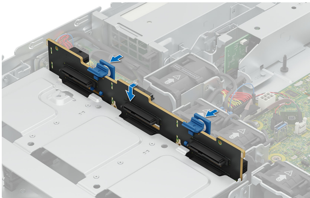
Ilustración 38. Instalación del backplane de la bahía de unidad frontal
