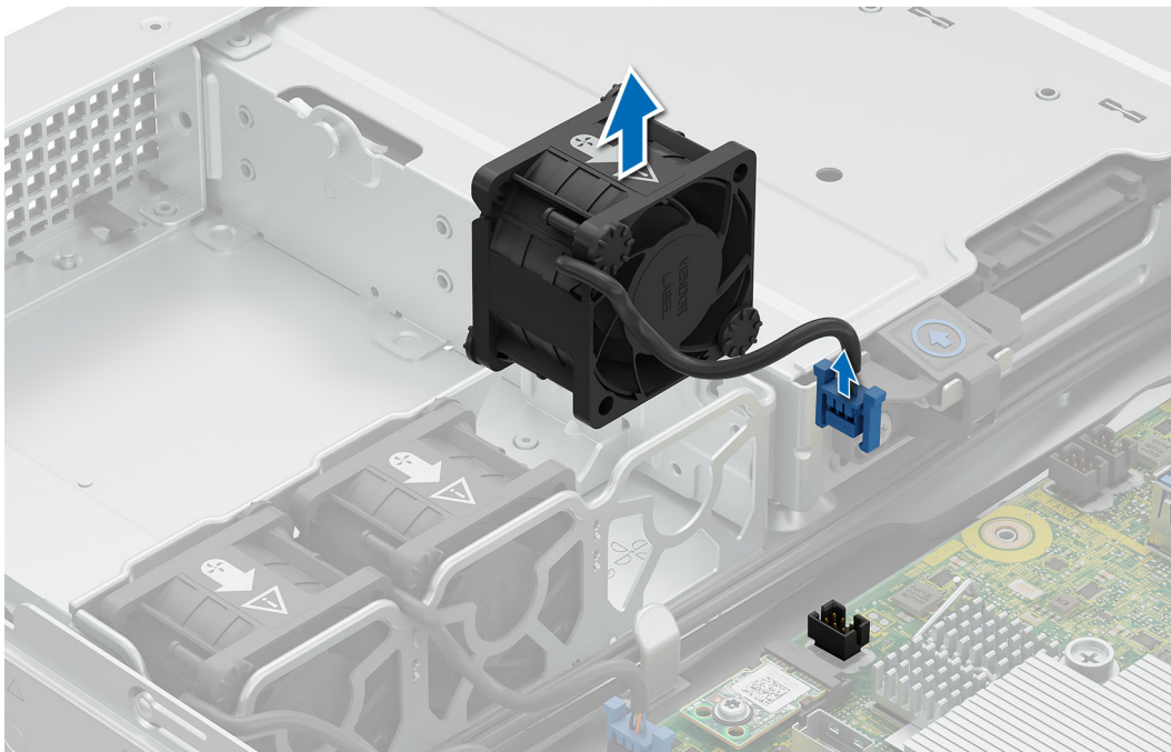
Ilustración 31. Extracción del ventilador de enfriamiento
