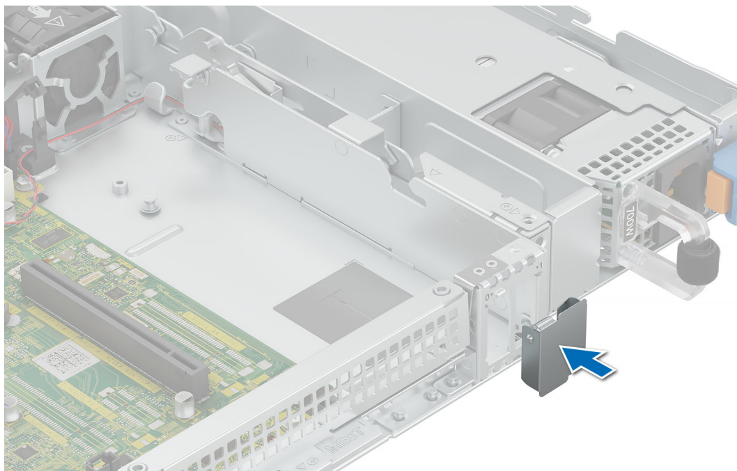
Ilustración 70. Instalación del panel de relleno de BOSS N1
