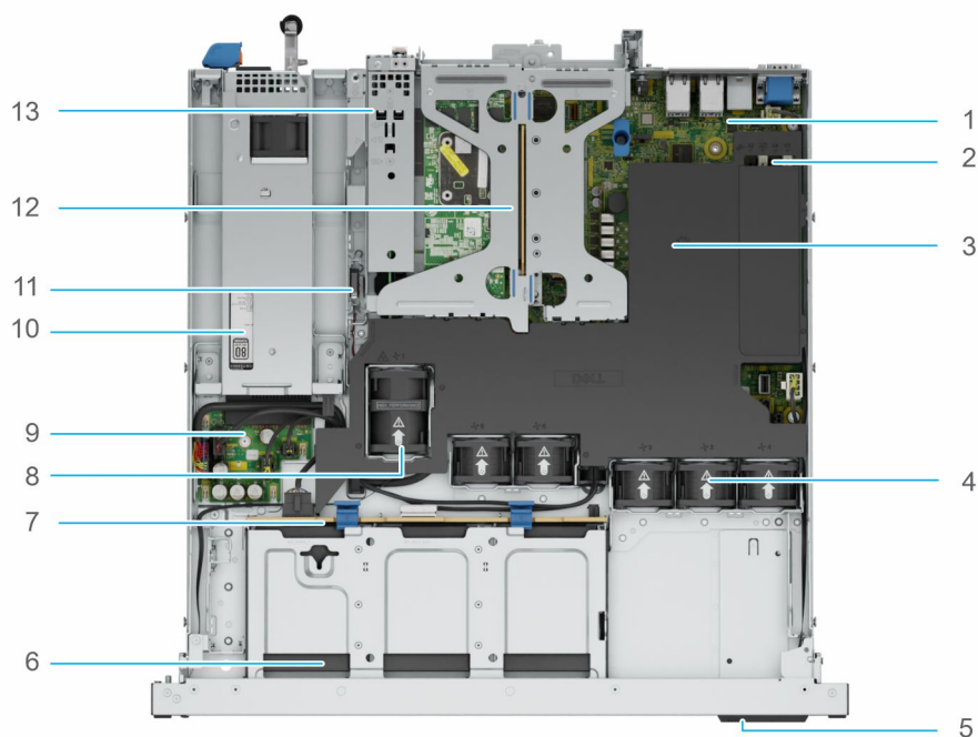
Ilustración 7. Vista interior del sistema con PSU no cableada y unidades de 2,5 pulgadas con cubierta para flujo de aire y tarjeta elevadora
