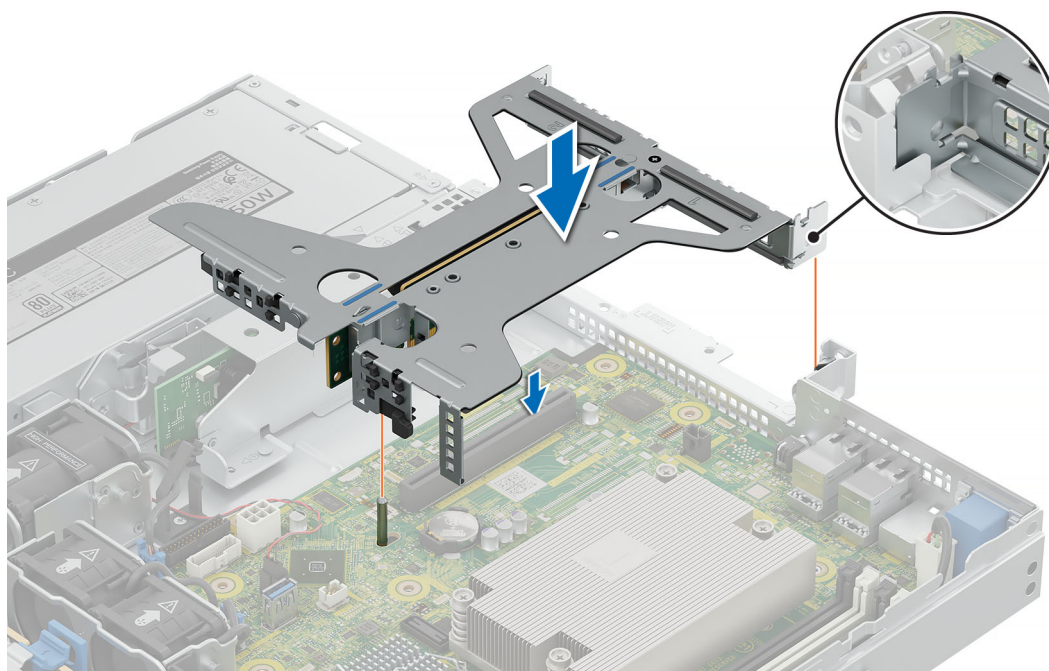
Ilustración 68. Instalación del soporte vertical
