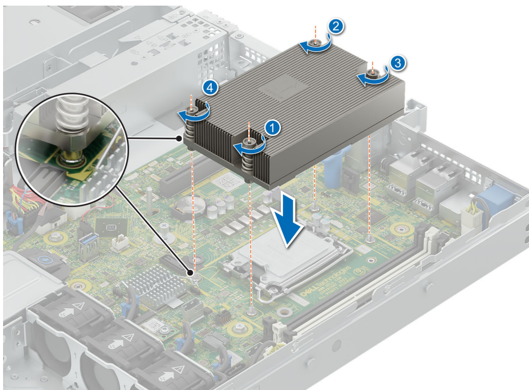
Ilustración 61. Instalación del disipador de calor
