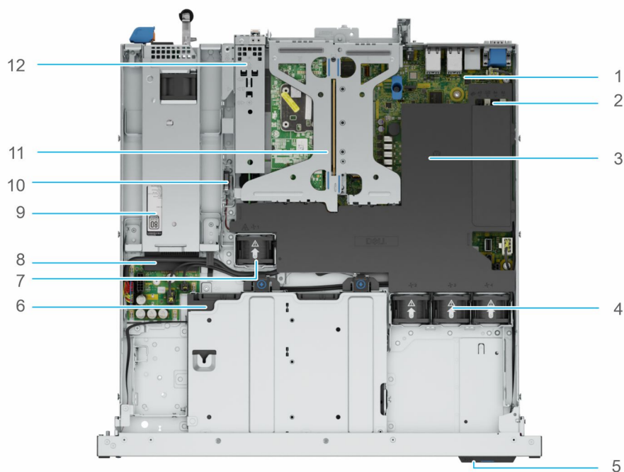
Ilustración 10. Vista interior del sistema con PSU no cableada y unidades de 3,5 pulgadas con cubierta para flujo de aire y tarjeta elevadora
