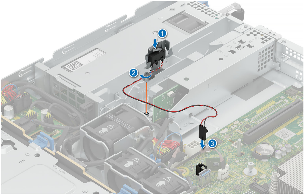
Ilustración 35. Instalación del interruptor de intrusiones
