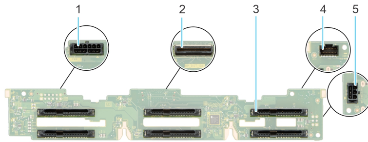
Ilustración 36. Backplane de seis unidades SAS/SATA/SSD de 2,5 pulgadas
