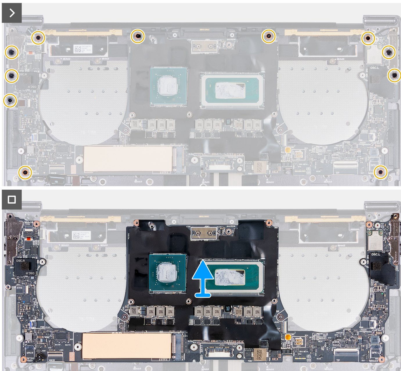
Ilustración 34. Extracción de la tarjeta madre
