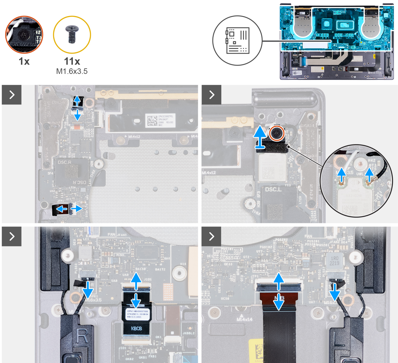
Ilustración 33. Extracción de la tarjeta madre
