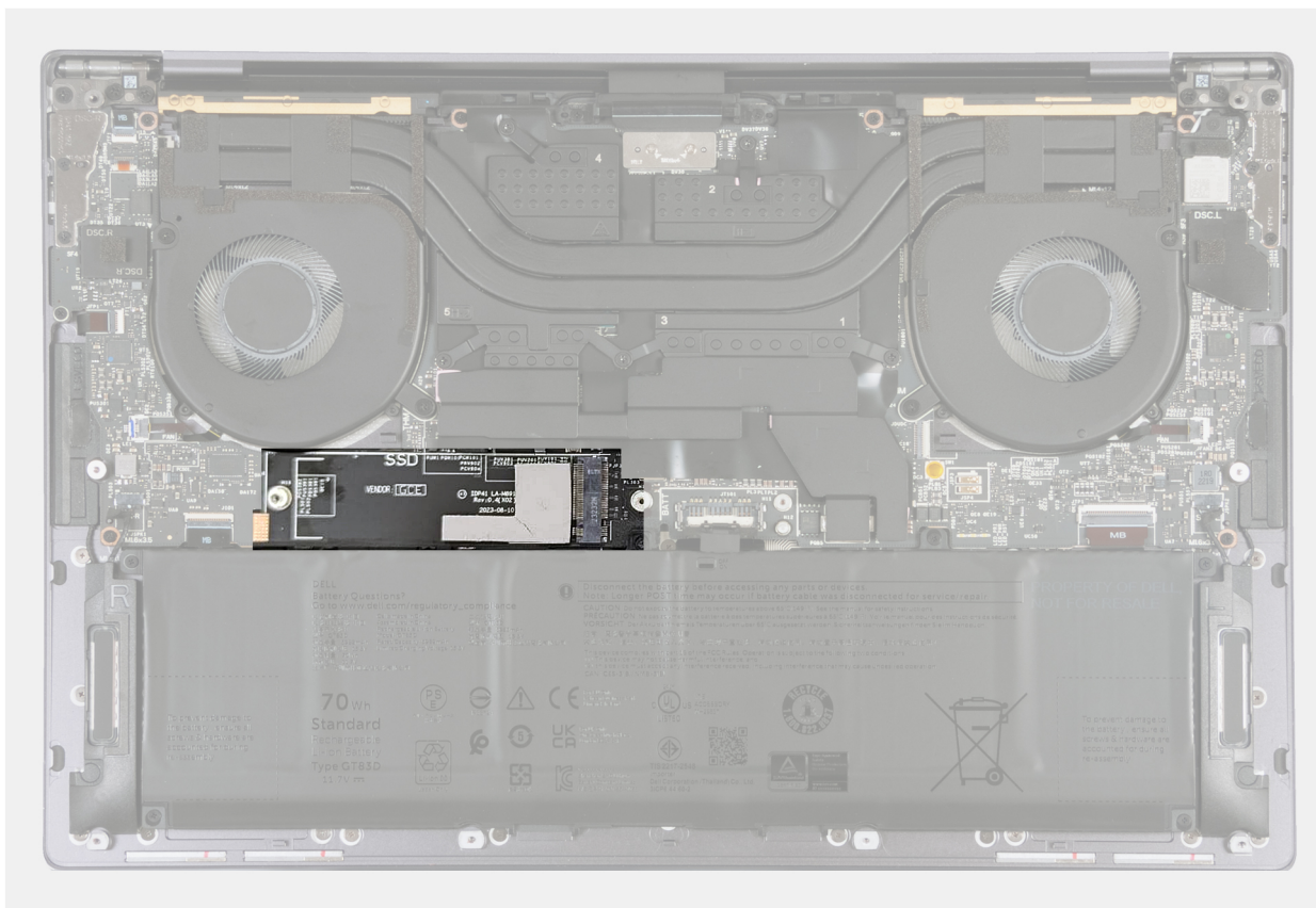
Ilustración 19. Almohadilla térmica de la SSD M.2
