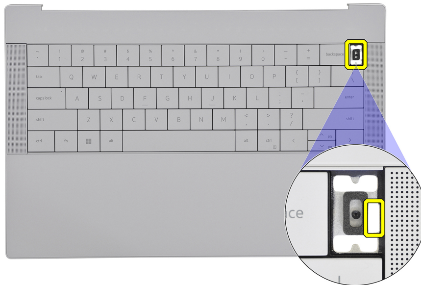
Ilustración 39. Botón de encendido con lector de huellas digitales
