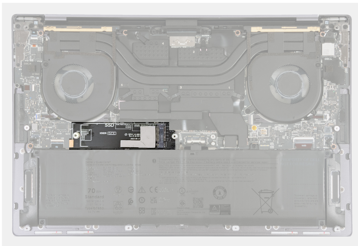
Ilustración 20. Almohadilla térmica de la SSD M.2
