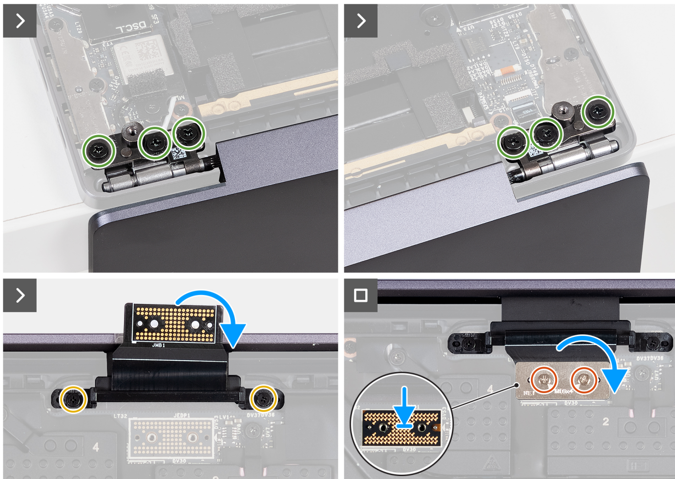
Ilustración 31. Instalación del ensamblaje de la pantalla
