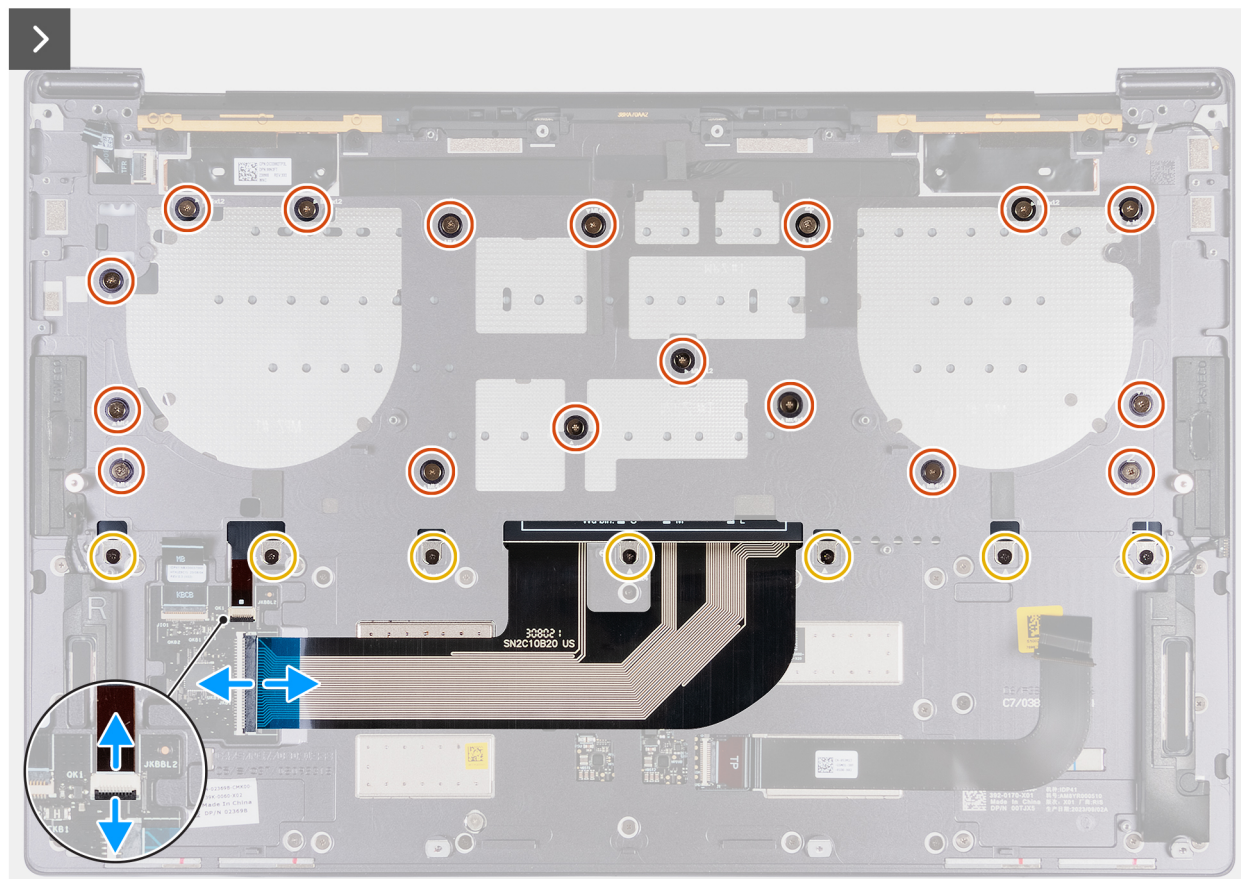
Ilustración 41. Extracción del teclado
