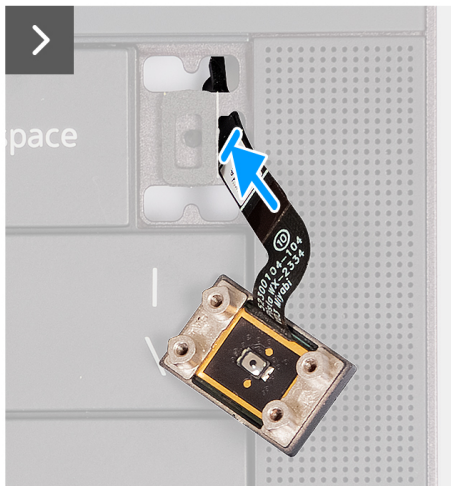
Ilustración 40. Instalación del botón de encendido con lector de huellas digitales
