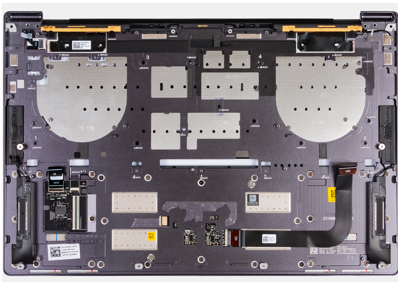
Ilustración 47. Ensamblaje del reposamanos
