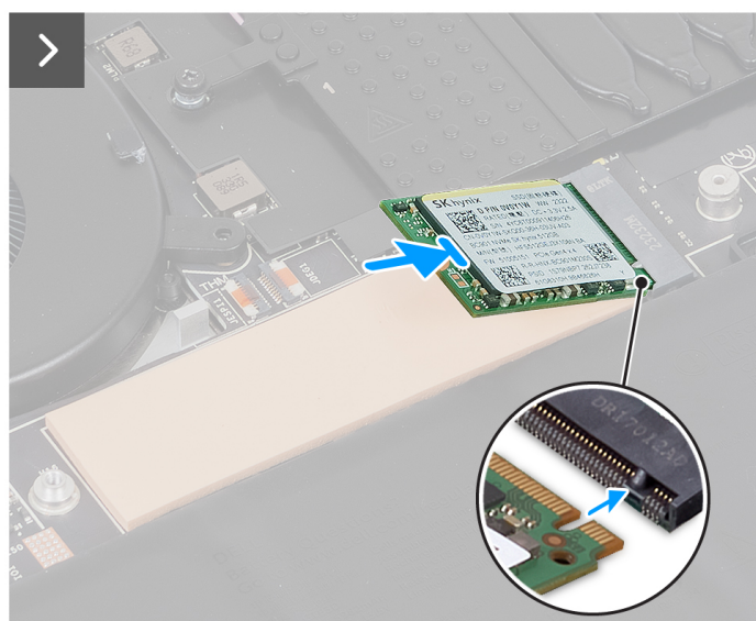
Ilustración 21. Instalación de la unidad de estado sólido M.2 2230
