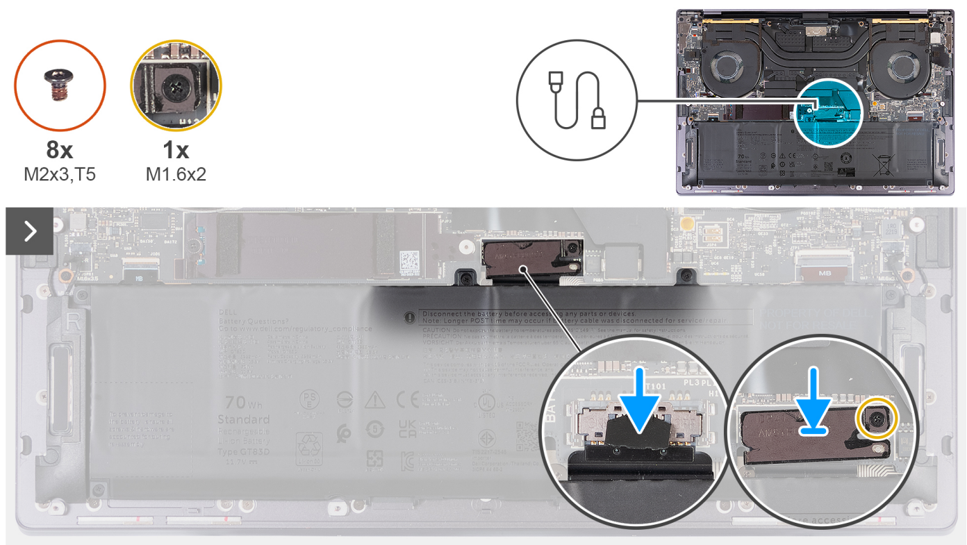
Ilustración 13. Instalación de la cubierta de la base
