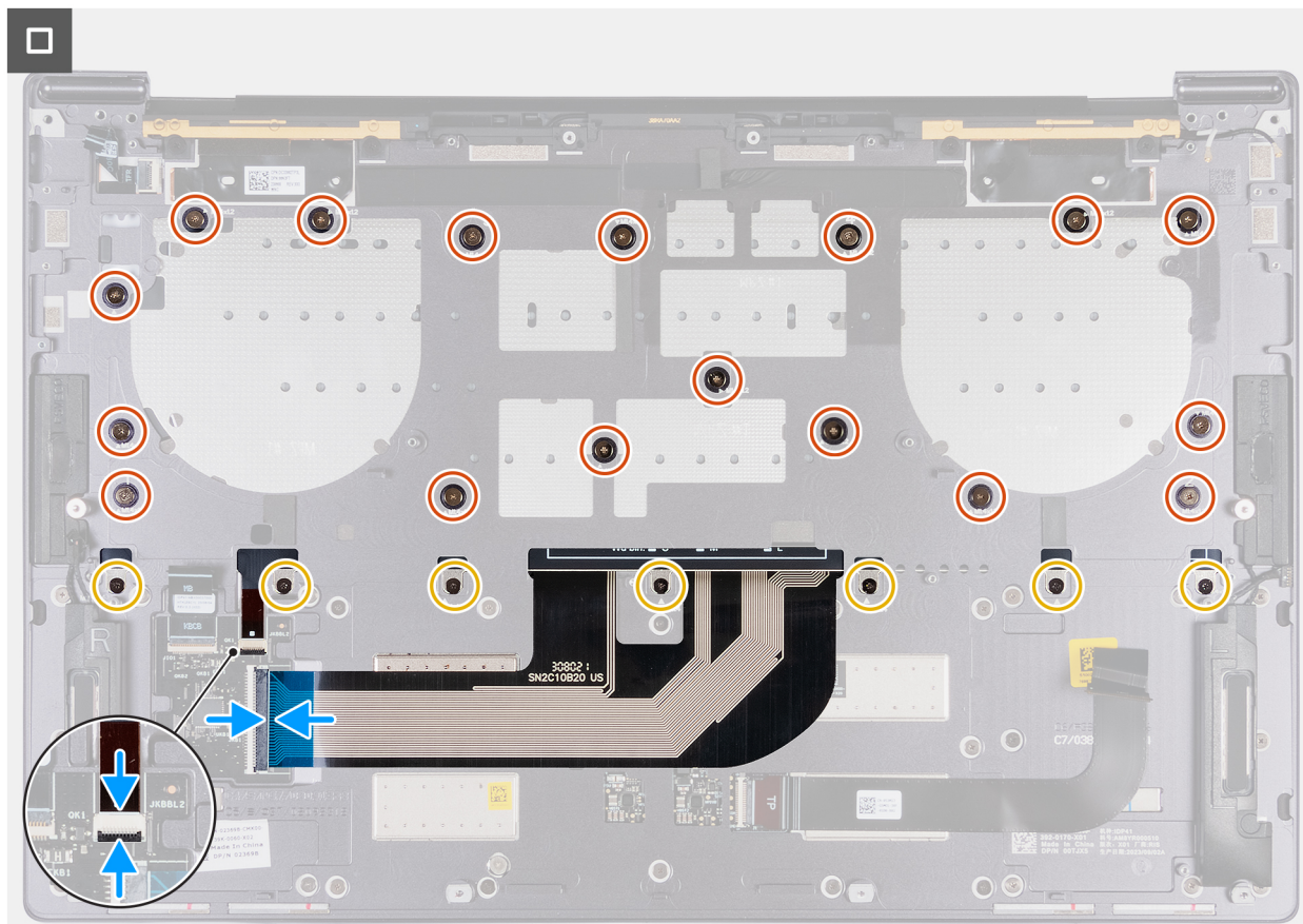
Ilustración 44. Instalación del teclado
