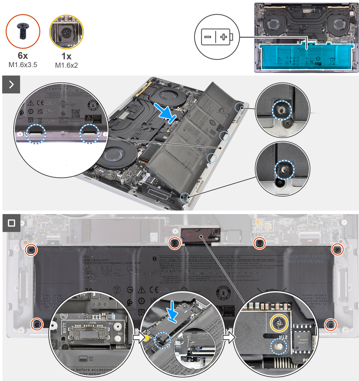
Ilustración 18. Instalación de la batería
