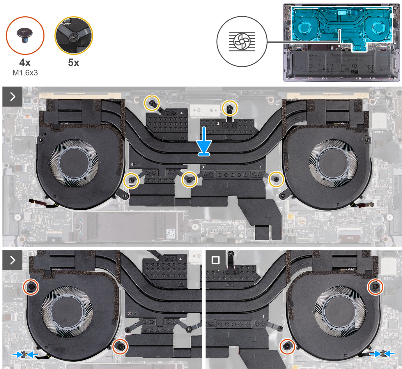
Ilustración 26. Instalación del ensamblaje del disipador de calor
