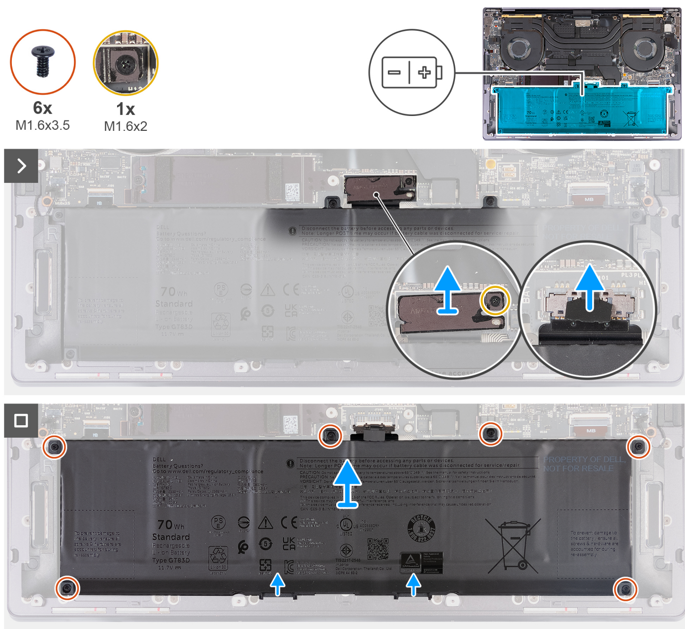
Ilustración 17. Extracción de la batería
