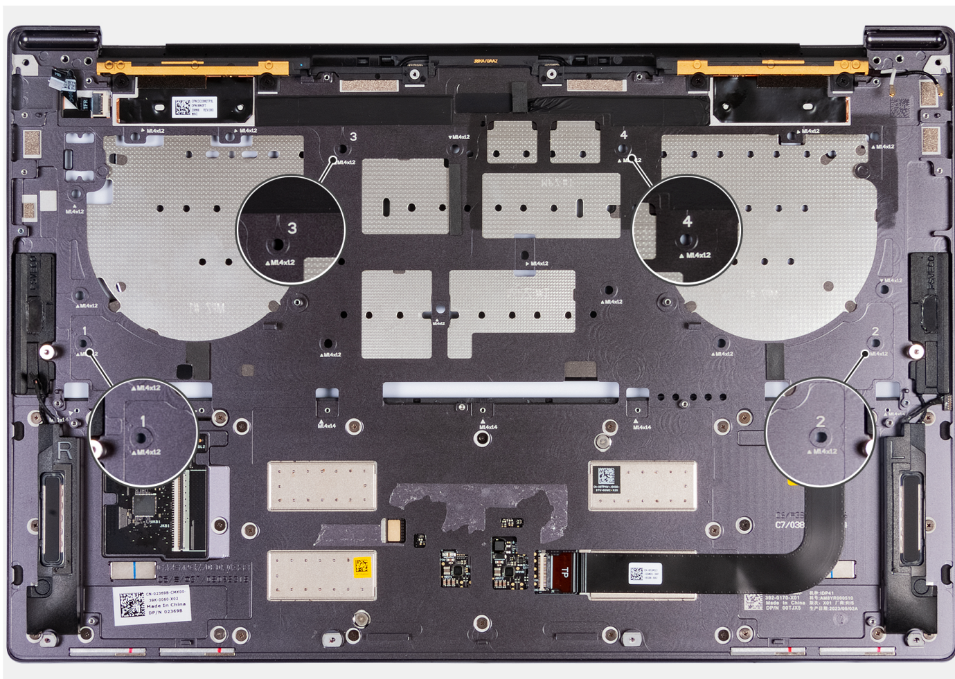
Ilustración 45. Instalación de los cuatro tornillos en secuencia cuando se fija el teclado al ensamblaje del reposamanos
