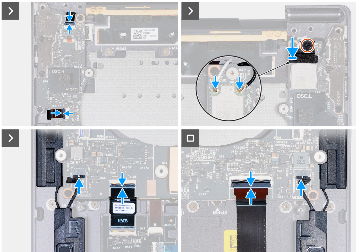
Ilustración 37. Instalación de la tarjeta madre
