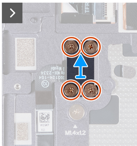
Ilustración 38. Extracción del botón de encendido con lector de huellas digitales
