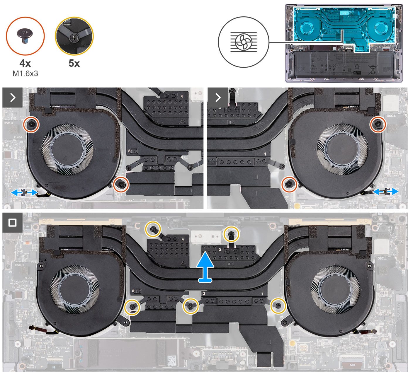
Ilustración 25. Extracción del ensamblaje del disipador de calor
