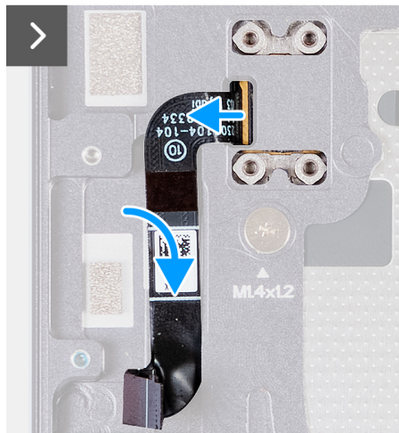
Ilustración 40. Instalación del botón de encendido con lector de huellas digitales
