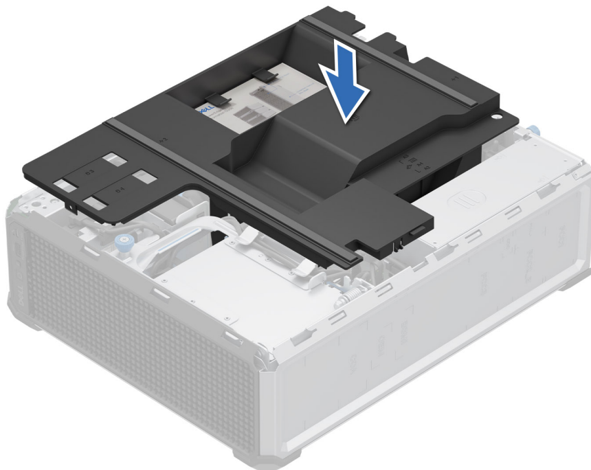
Figure 15. Installation du carénage d'aération
