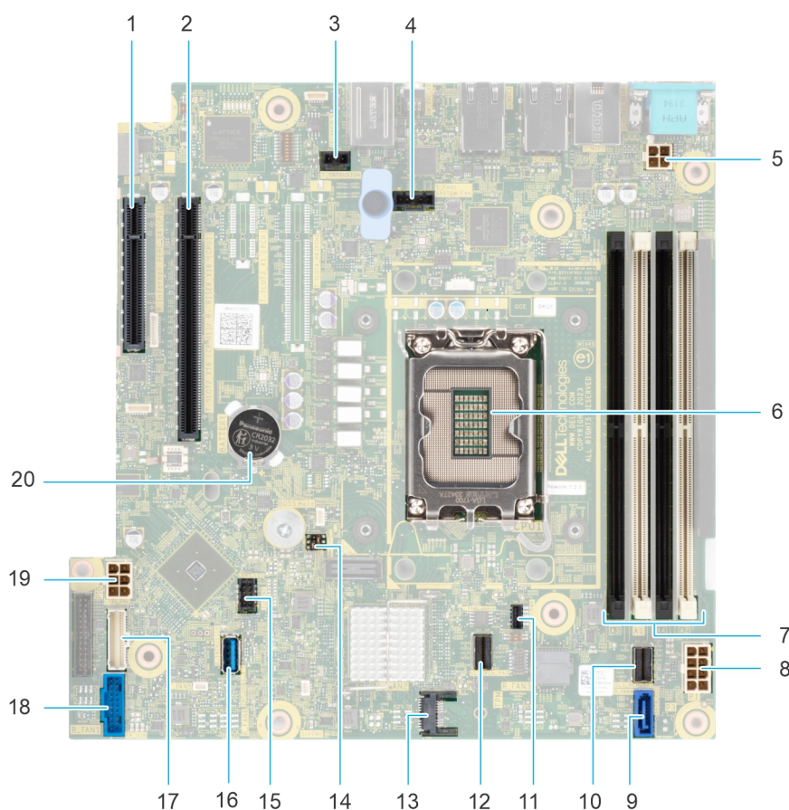
Figure 70. Disposition de la carte système
