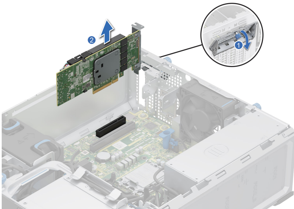
Figure 43. Retrait d'une carte d'extension
