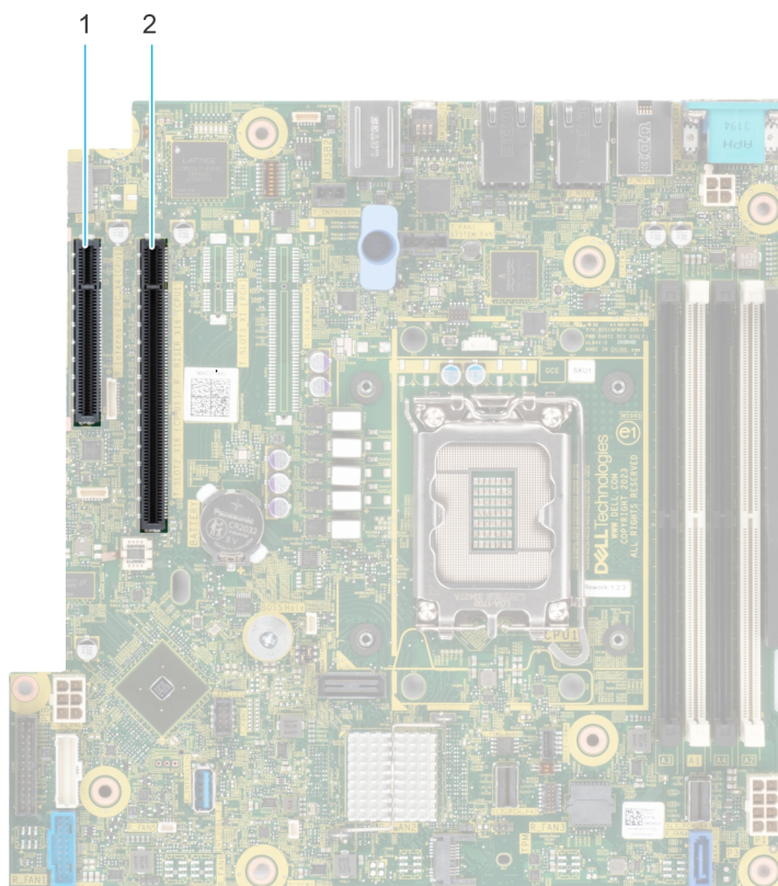
Figure 42. Logements du connecteur PCIe sur la carte système
