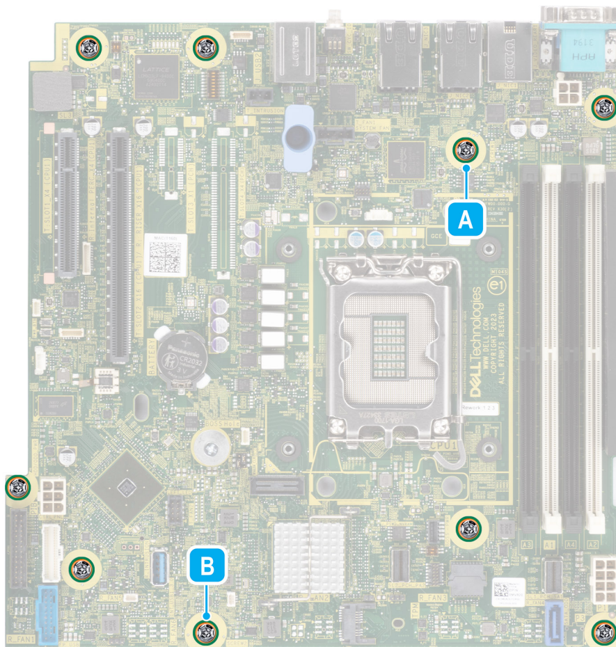
Figure 61. Emplacement des vis de la carte système
