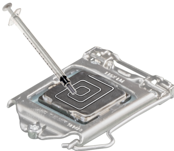
Figure 40. Application de graisse thermique sur la partie supérieure du processeur
