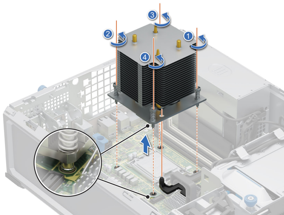
Figure 37. Retrait du dissipateur de chaleur
