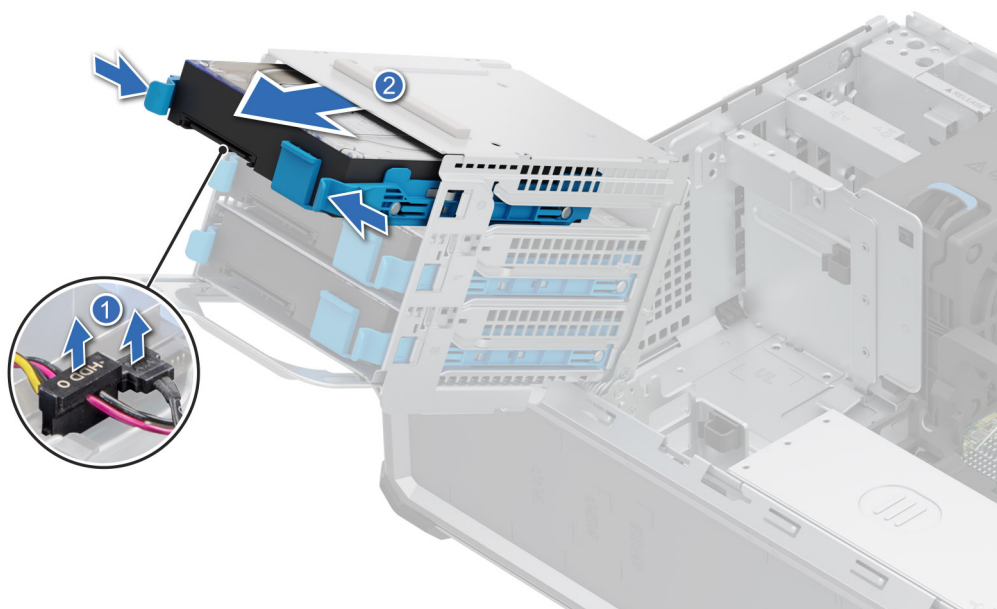
Figure 19. Retrait d'un disque dur du bâti de disques durs
