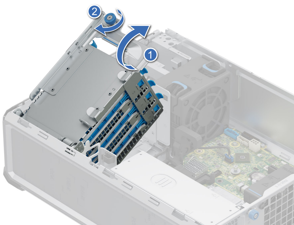
Figure 22. Installation d'un support de disque
