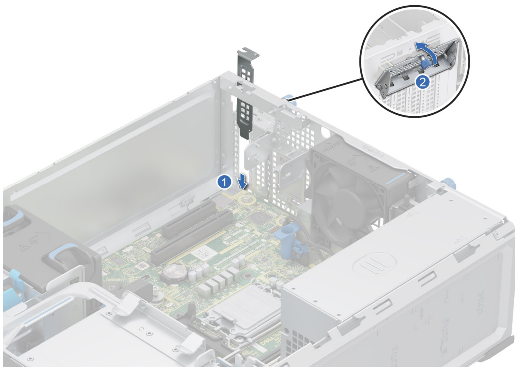
Figure 44. Installation de la languette métallique de remplissage
