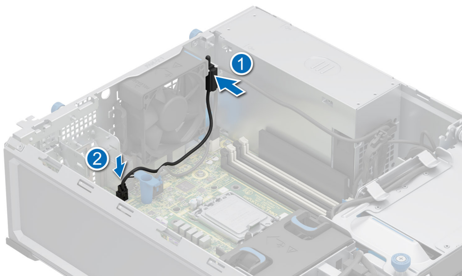
Figure 17. Installation du module du commutateur d'intrusion
