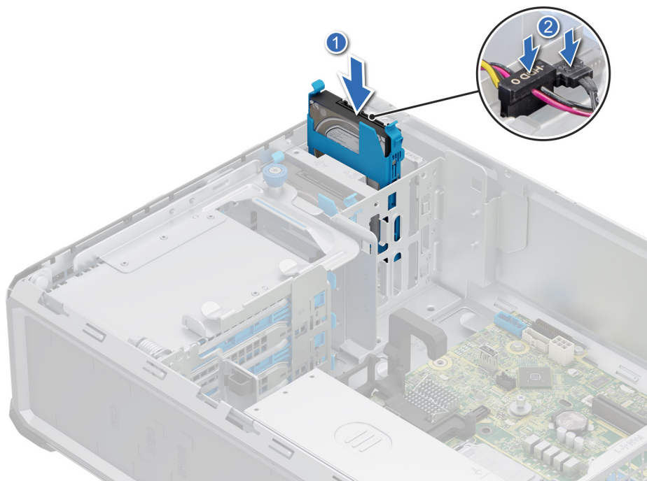
Figure 23. Installation d'un support de disque
