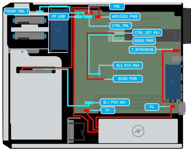
Figure 30. Acheminement des câbles : 3 disques puce SATA de 3,5 pouces
