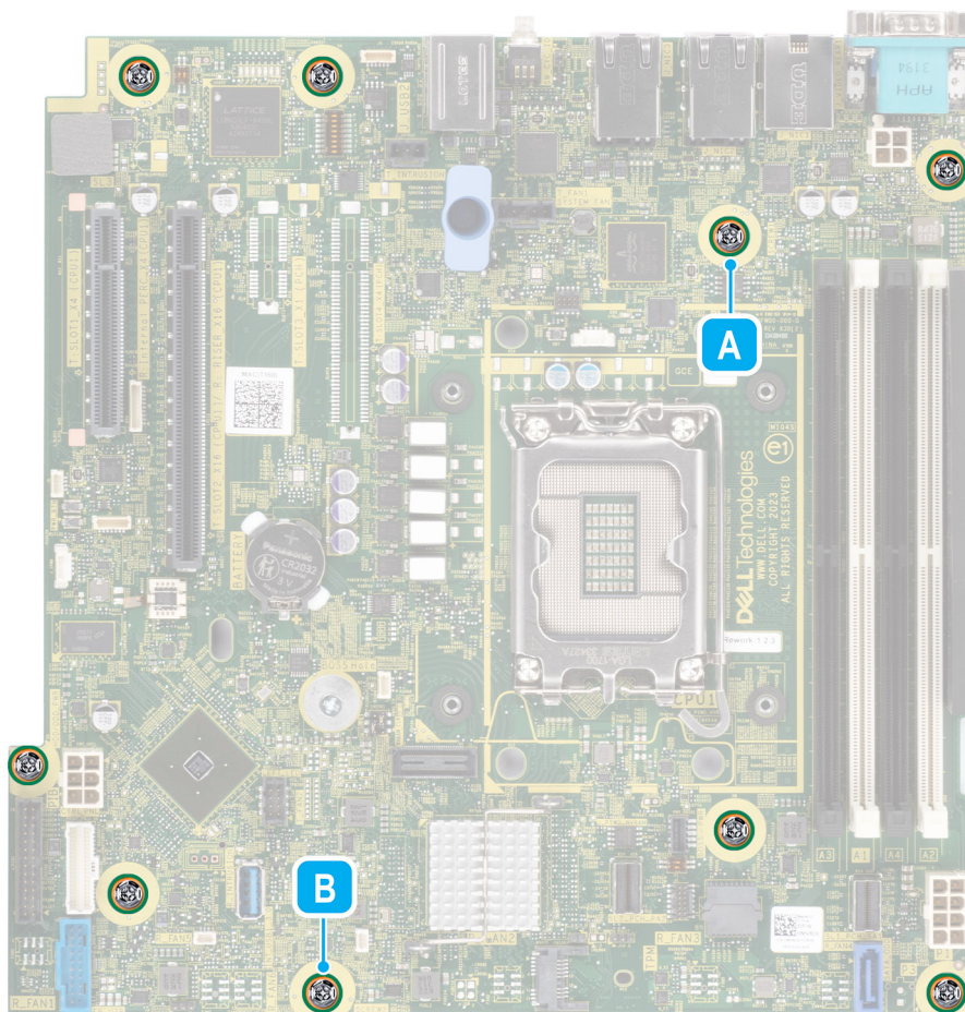
Figure 64. Emplacement des vis de la carte système
