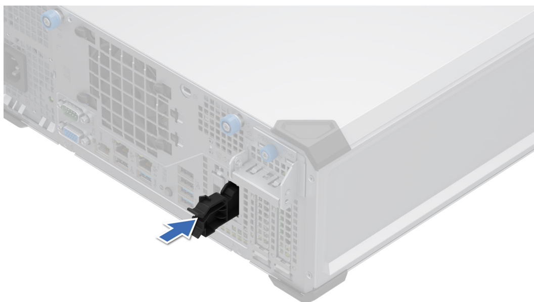
Figure 48. Installation du cache du module BOSS-N1
