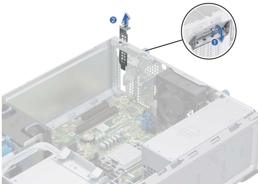
Figure 45. Retrait de la plaque de recouvrement métallique
