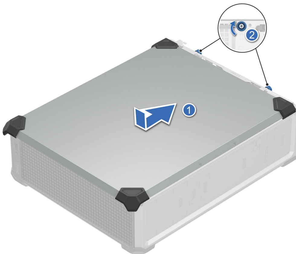
Figure 13. Installation du capot du système
