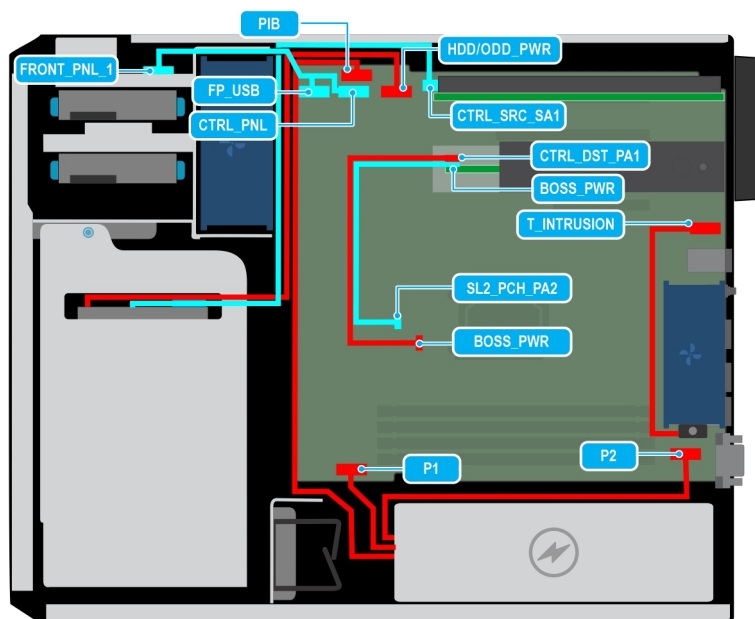
Figure 31. Acheminement des câbles : 3 disques durs PERC SATA de 3,5 pouces
