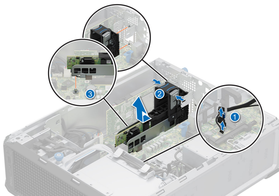
Figure 47. Retrait du module BOSS-N1
