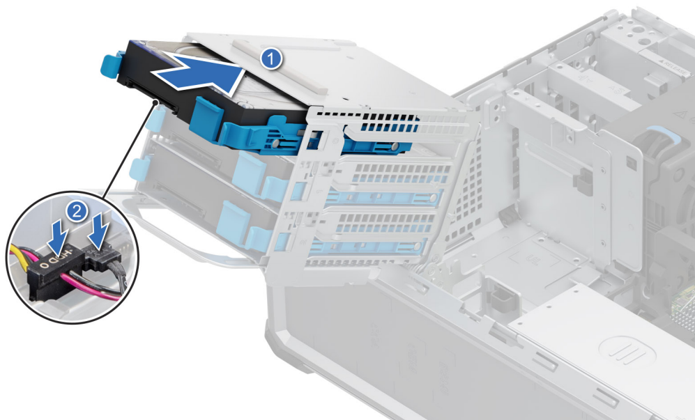
Figure 21. Installation d'un support de disque
