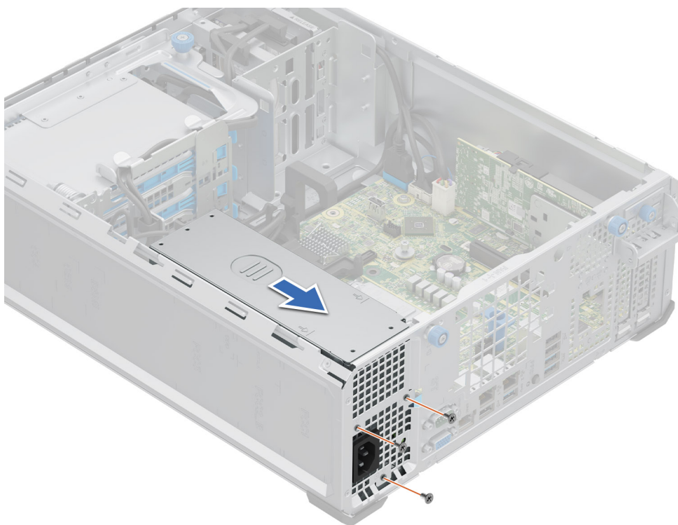
Figure 58. Installation du bloc d'alimentation câblé
