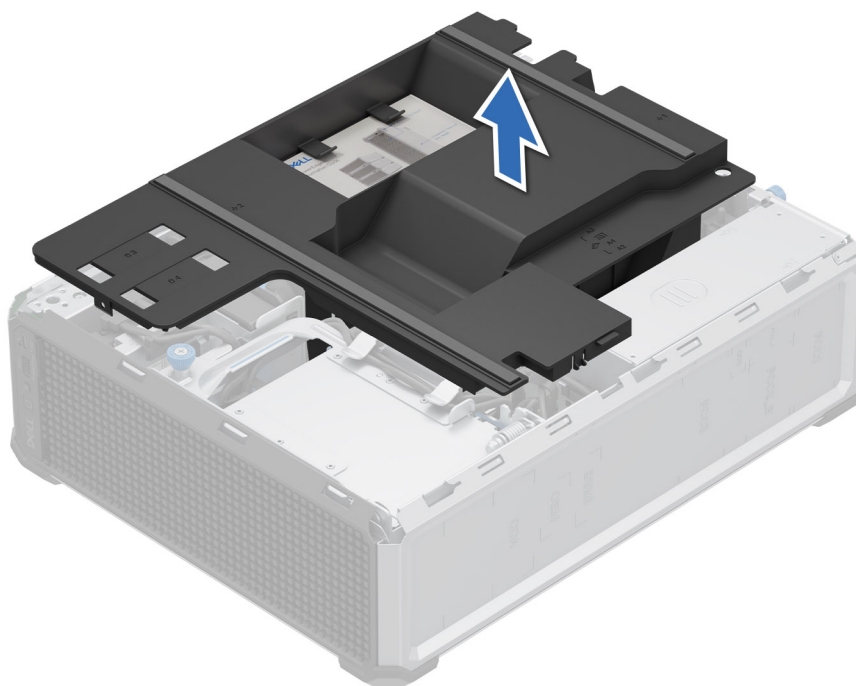
Figure 14. Retrait du carénage d'aération
