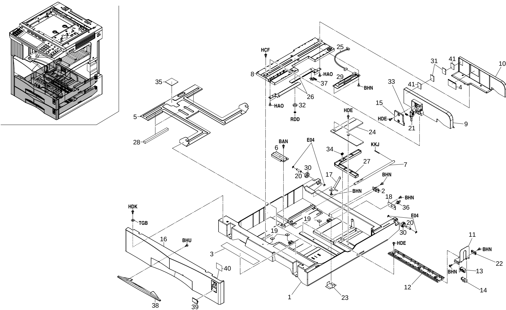
FIG. 3 CASSETTE
