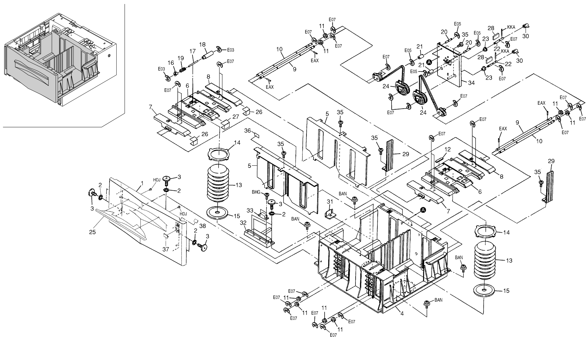
FIG. 2 CASSETTE
