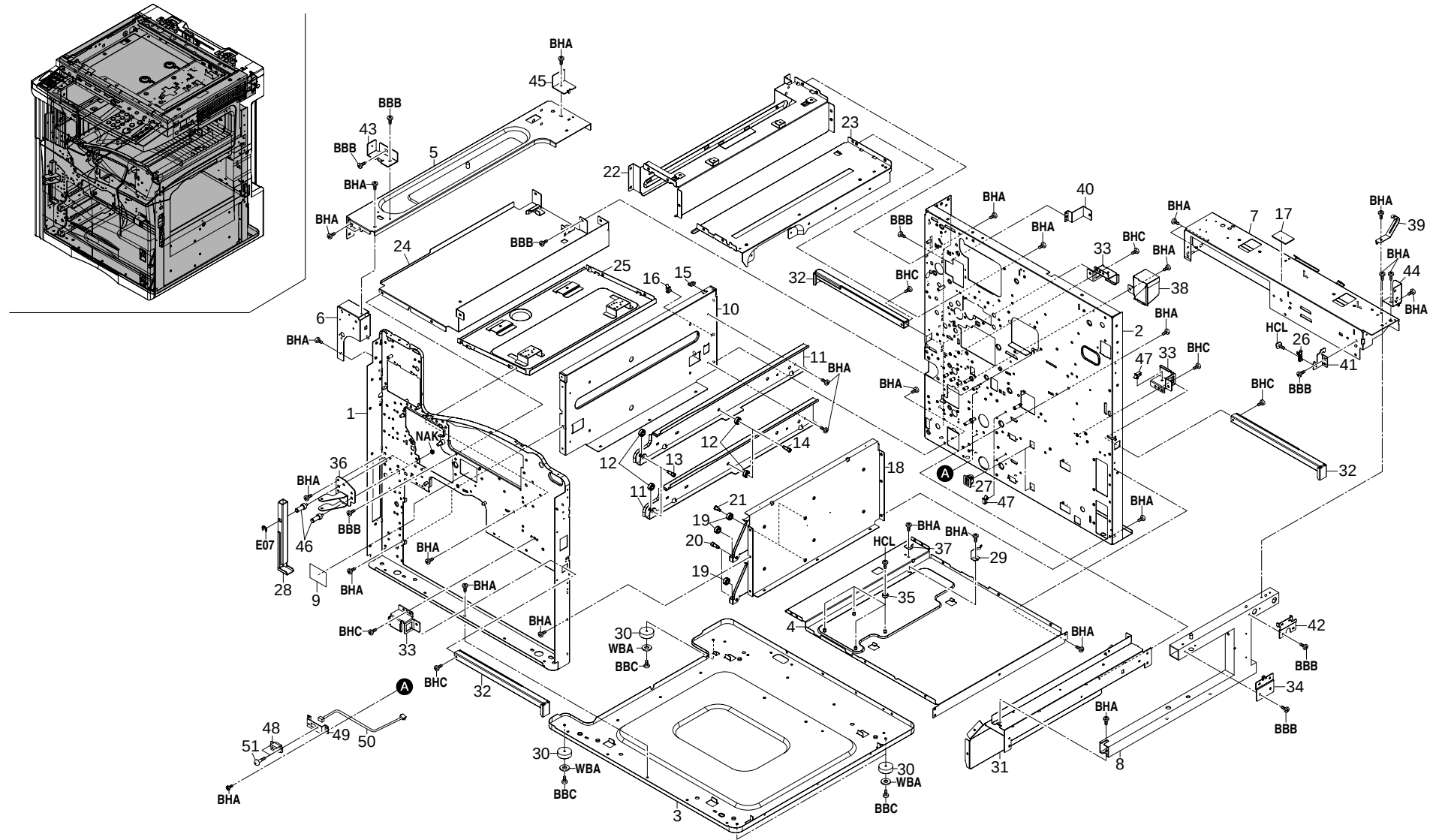
FIG. 2 FRAMES
