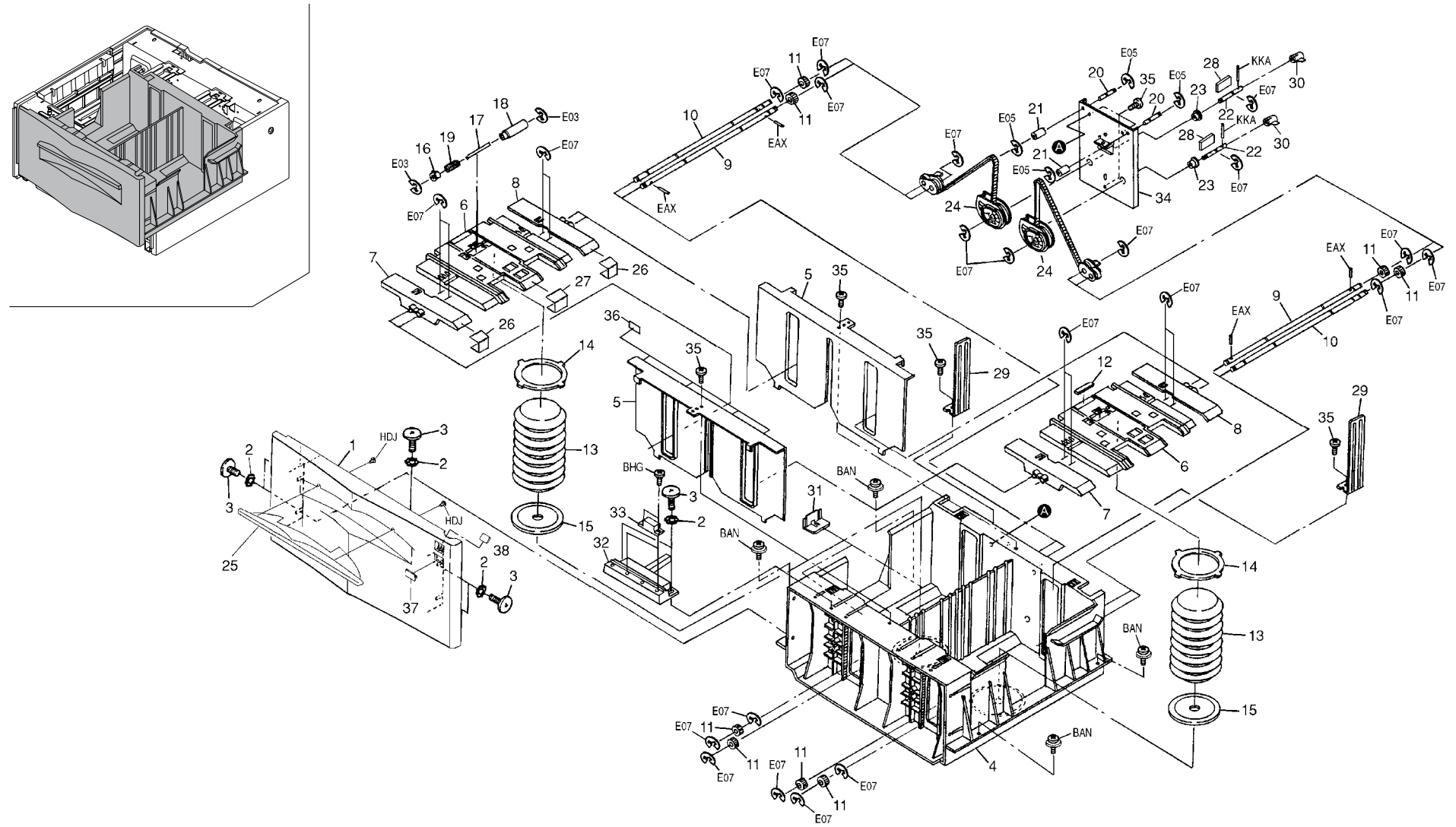
FIG. 2 CASSETTE
