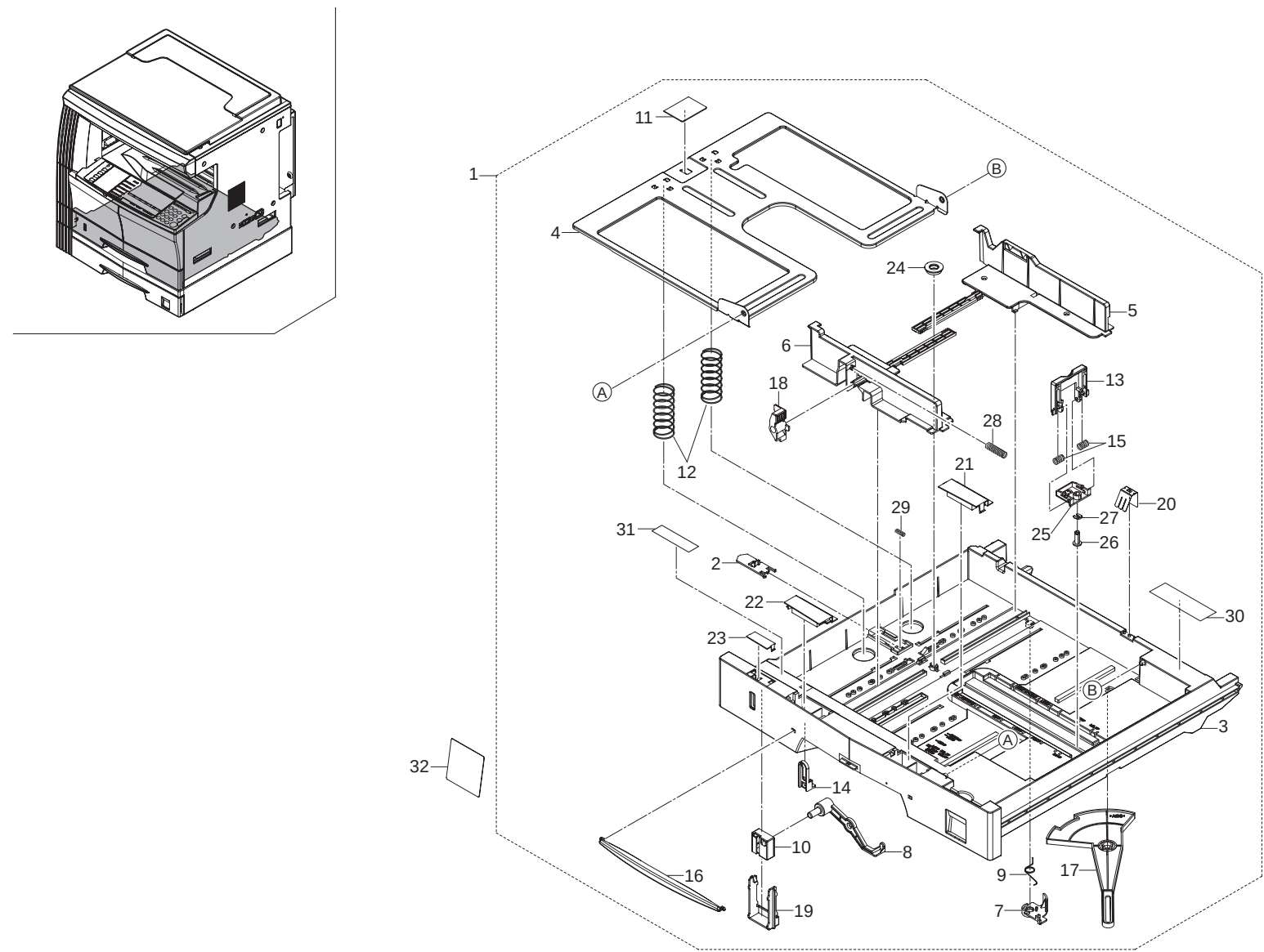
FIG. 5 Cassette
