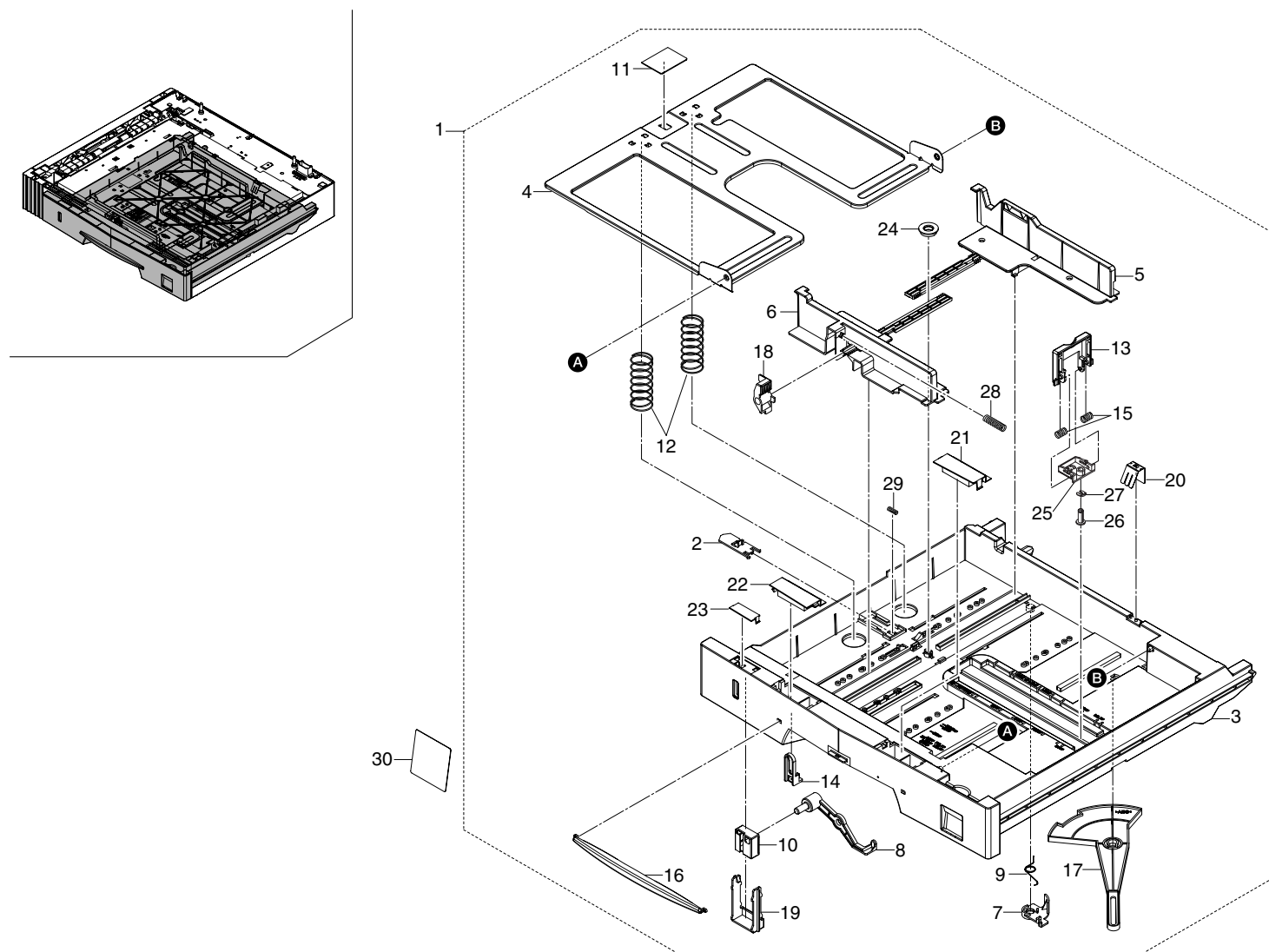
FIG. 3 CASSETTE
