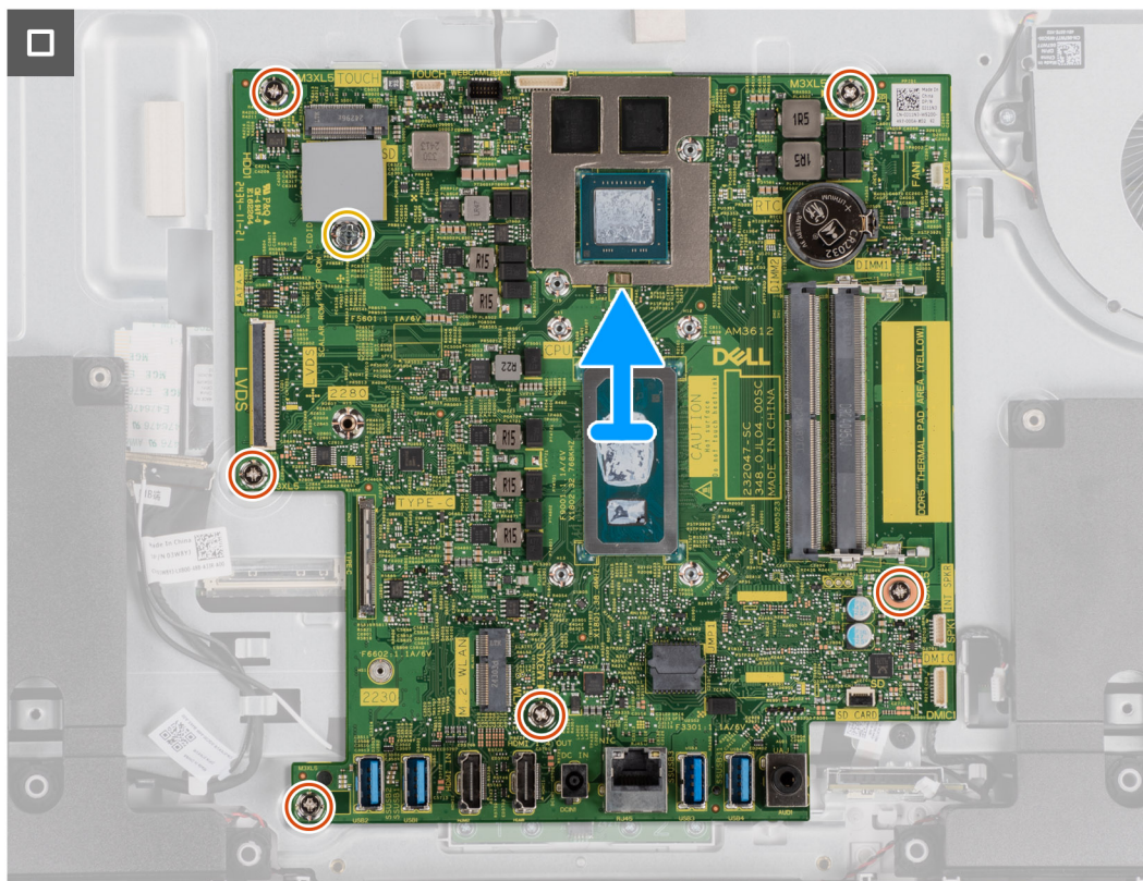
Rysunek 52. Wyjmowanie płyty głównej z obudowy komputera
