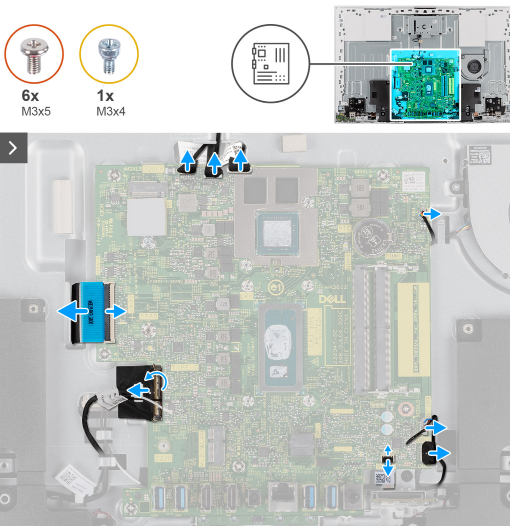
Rysunek 51. Wymontowywanie płyty głównej
