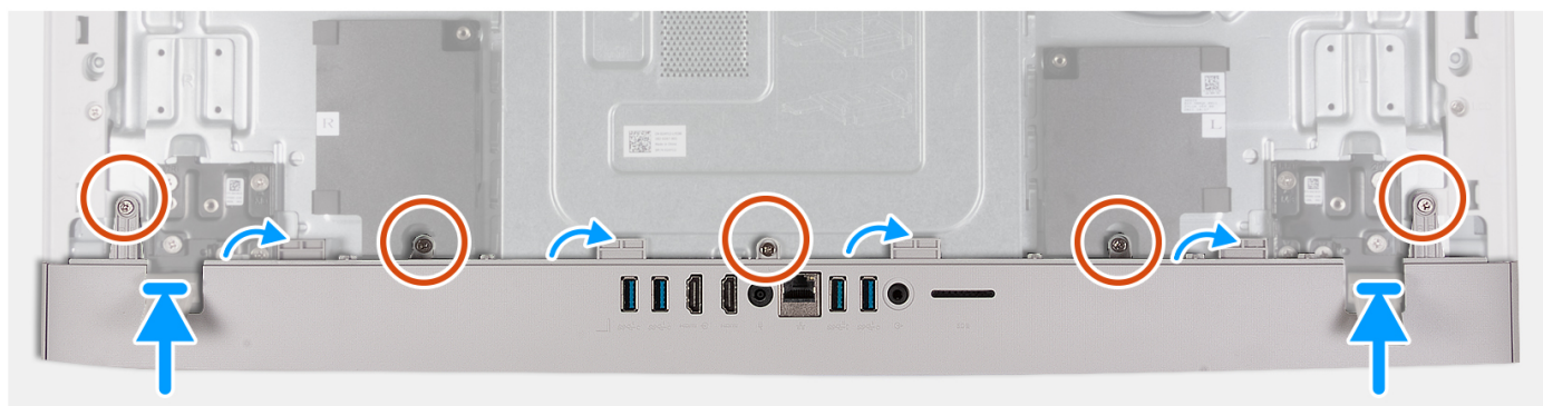
Rysunek 23. Instalowanie pokrywy dolnej
