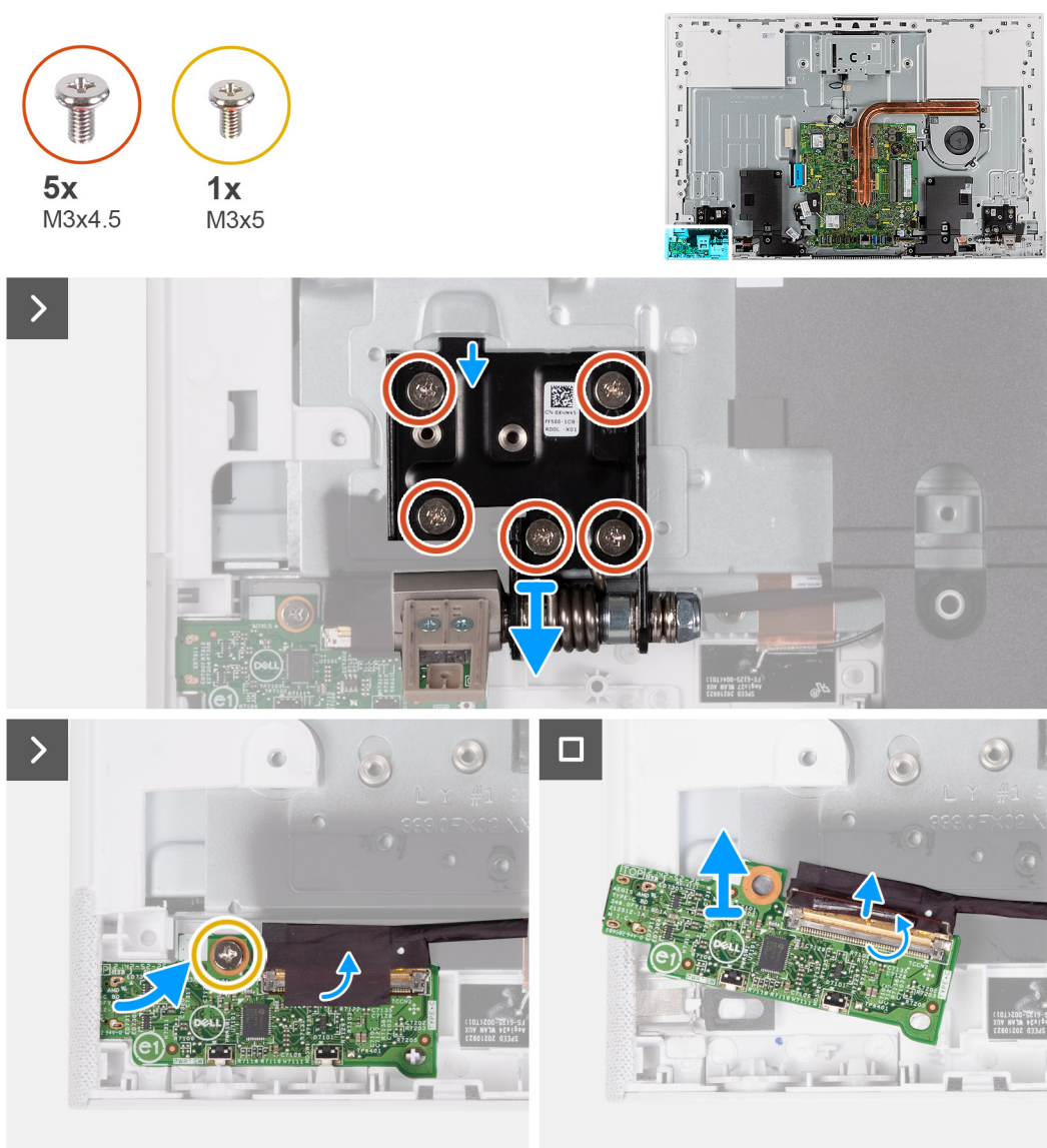
Rysunek 48. Wymontowywanie karty przycisku zasilania ze złączem USB
