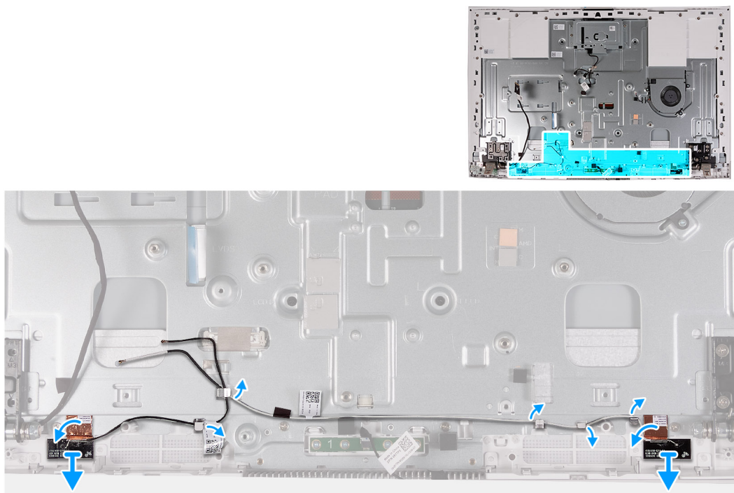
Rysunek 58. Wymontowywanie anten
