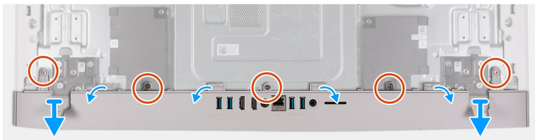
Rysunek 22. Wymontowywanie pokrywy złączy we/wy
