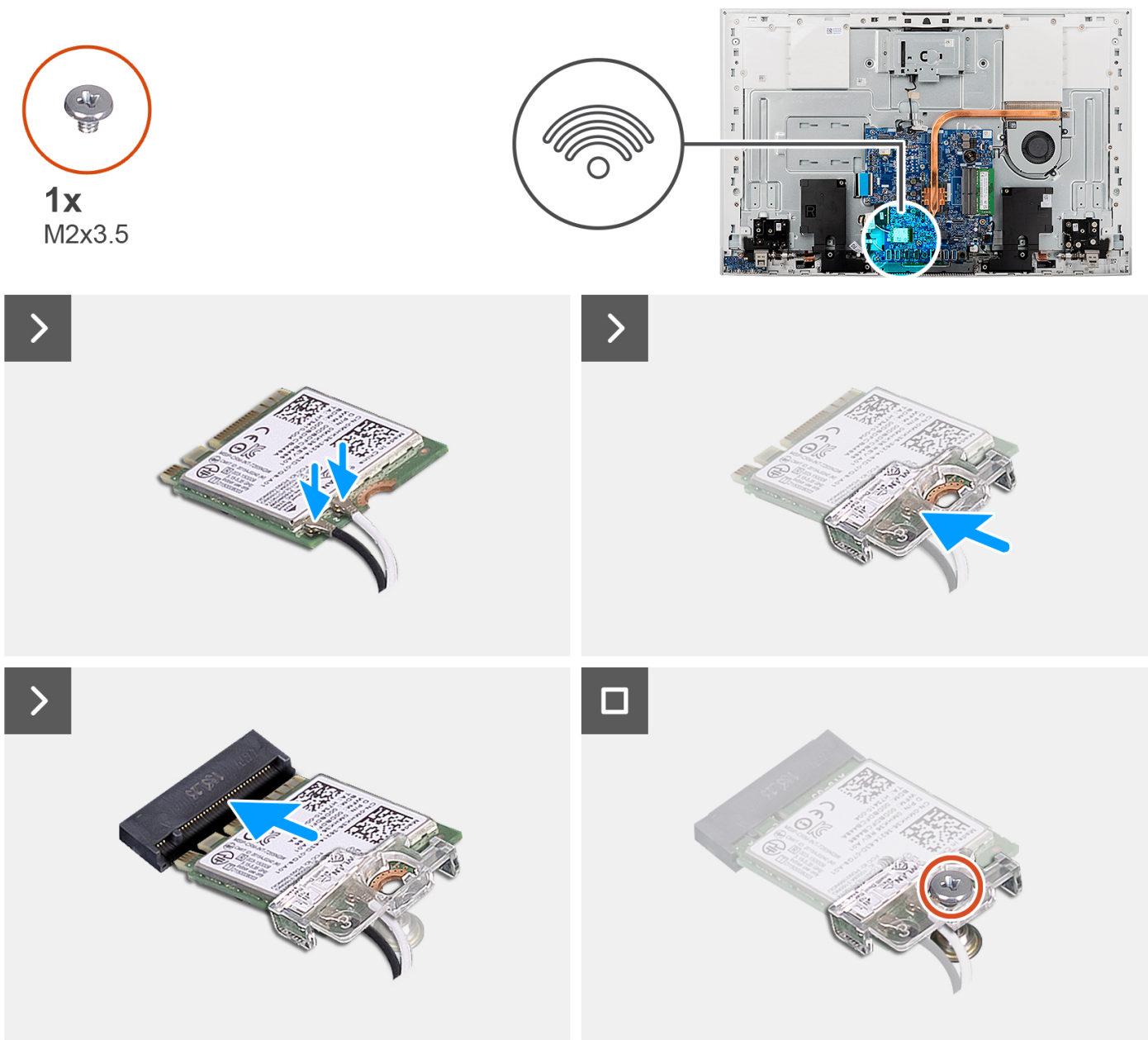
Rysunek 33. Instalowanie karty sieci bezprzewodowej
