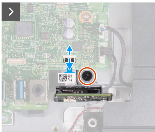
Rysunek 46. Wymontowywanie czytnika kart pamięci
