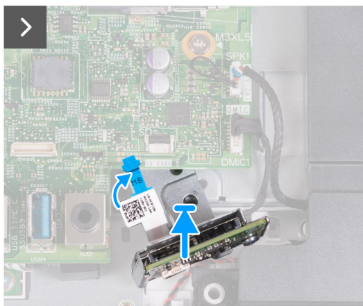
Rysunek 47. Instalowanie czytnika kart pamięci
