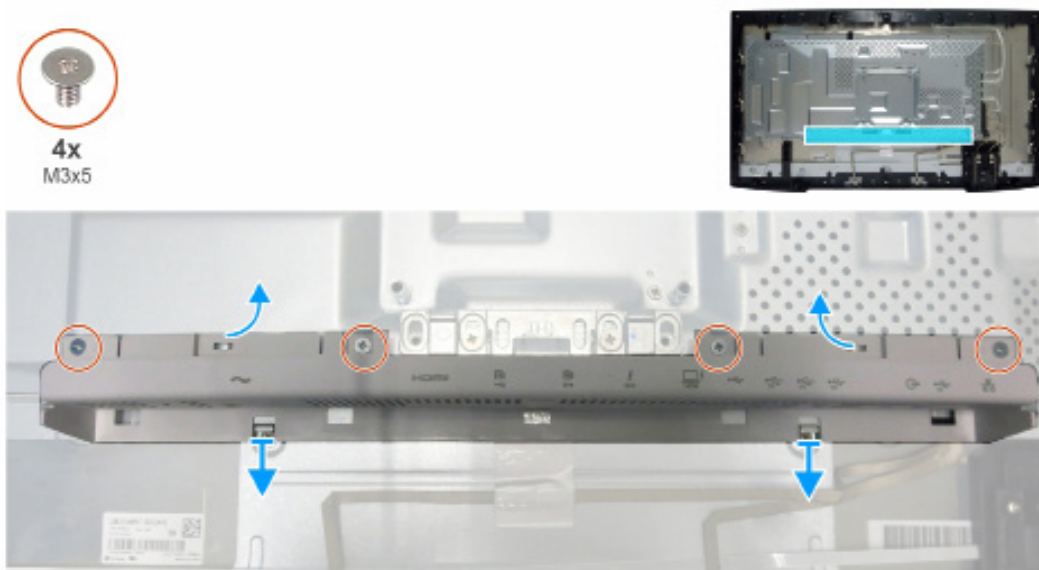
Obrázek 5. Demontáž krytu I/O
