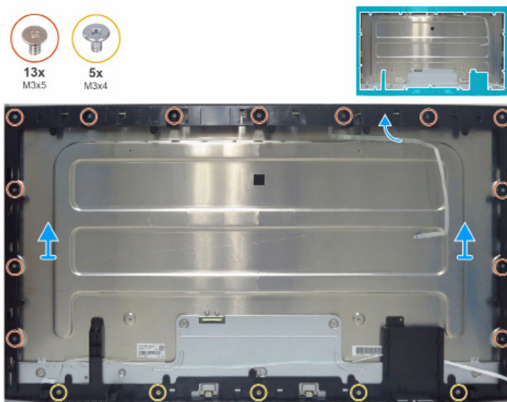
Obrázek 9. Demontáž středního rámu
