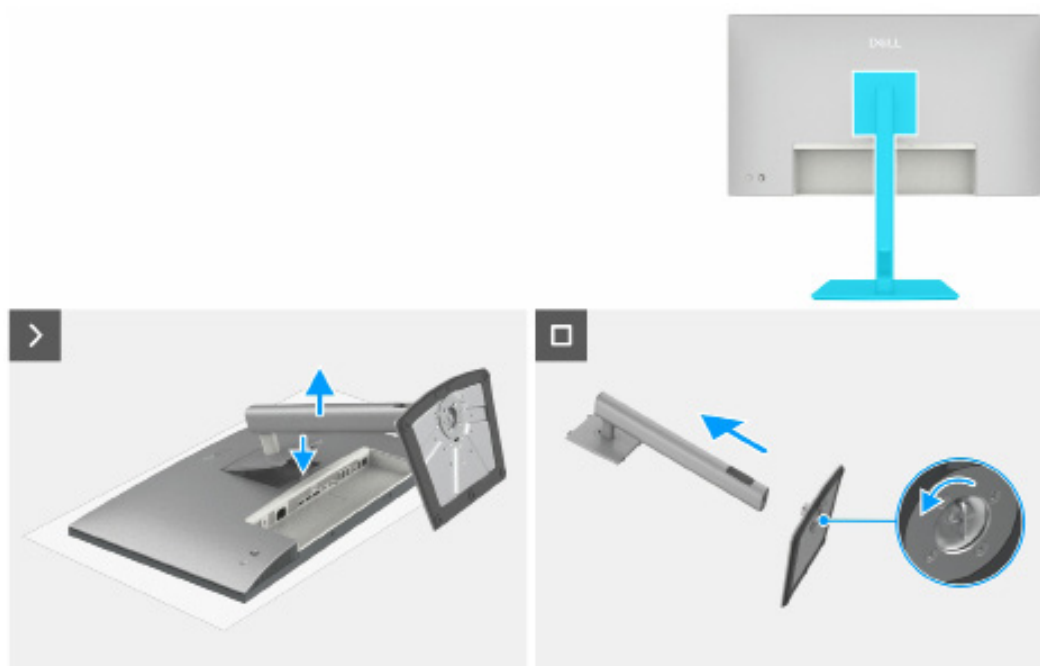
Obrázek 1. Demontáž stojánku
