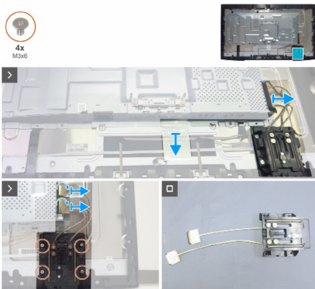
Obrázek 6. Demontáž QAP
