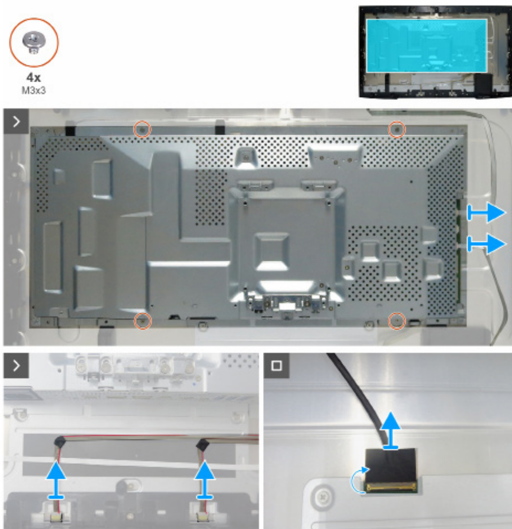
Obrázek 8. Demontáž základní desky
