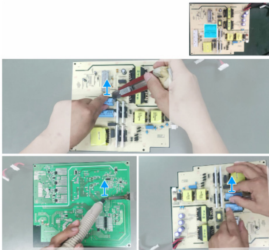
Obrázek 16. Demontáž elektrolytických kondenzátorů
