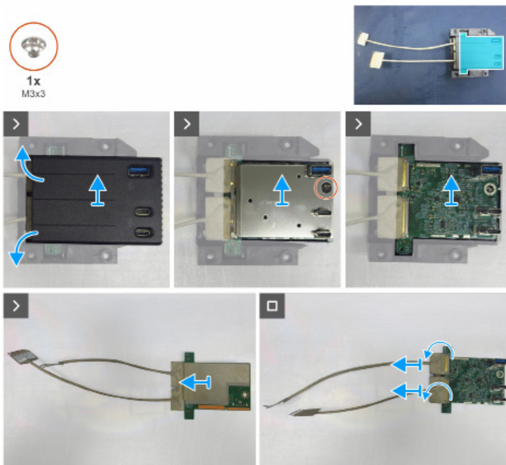
Obrázek 7. Demontáž desky USB
