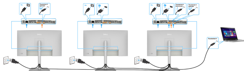
איור 36. חיבור המוניטור לפונקציית שרשרת דיזיין TBT-DP-2
