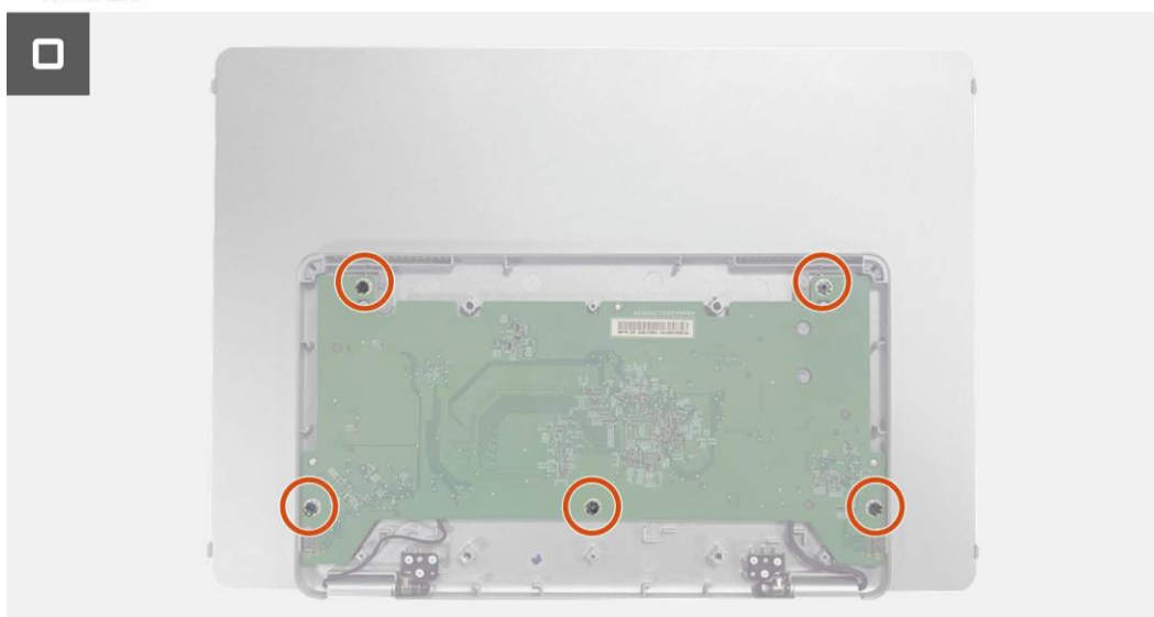
Obrázek 10. Instalace hlavní desky
