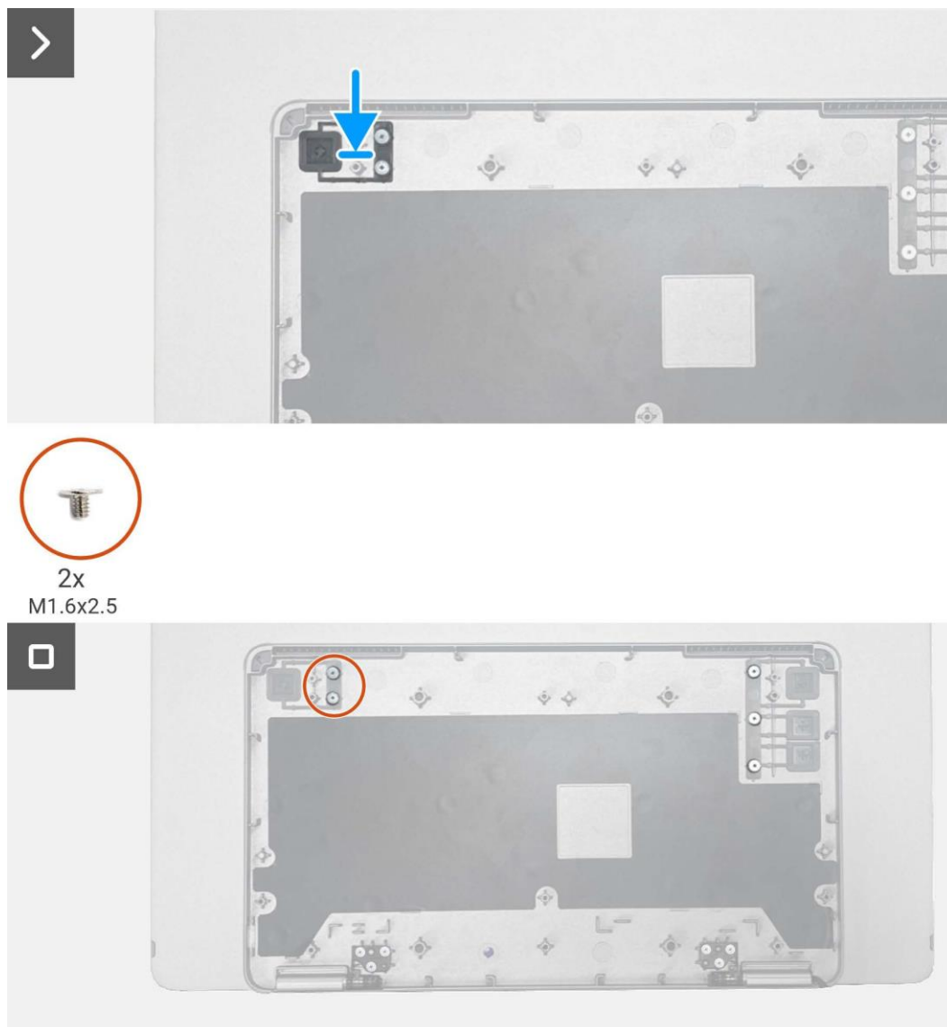
Obrázek 20. Instalace tlačítka napájení
