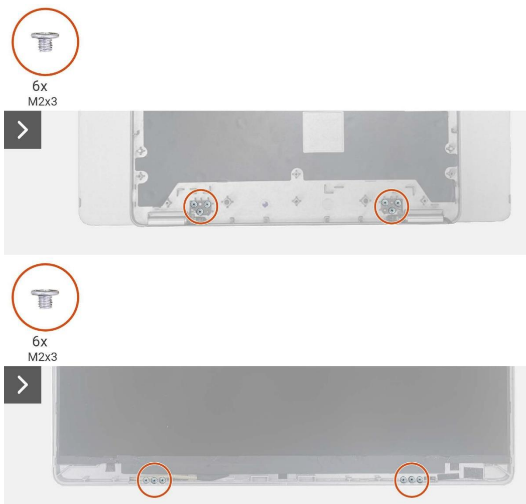
Obrázek 15. Odmontování závěsu
