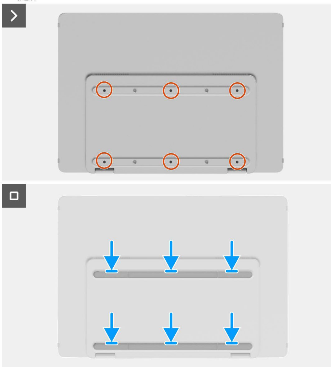
Obrázek 5. Instalace krytu dolní části základny
