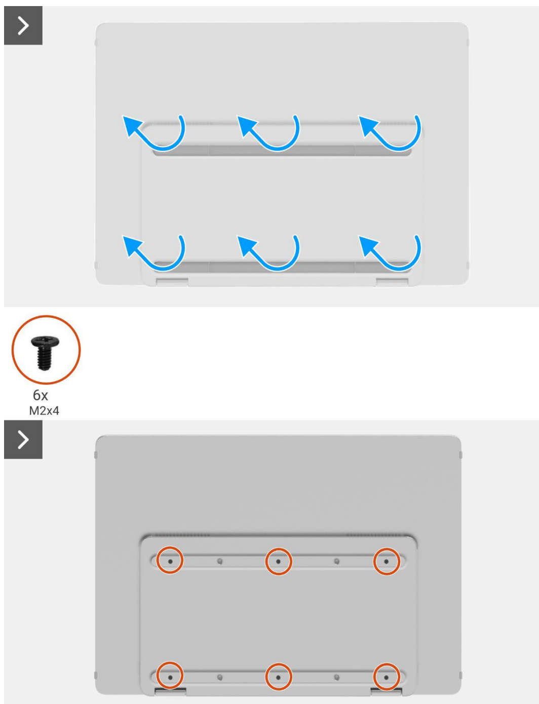
Obrázek 3. Odmontování krytu dolní části základny
