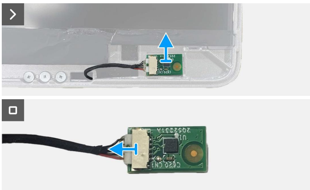
Obrázek 12. Odmontování desky snímače automatického otáčení
