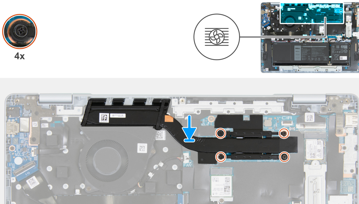
Rysunek 51. Instalowanie radiatora
