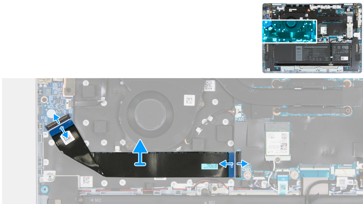
Rysunek 32. Wymontowywanie kabla płyty we/wy
