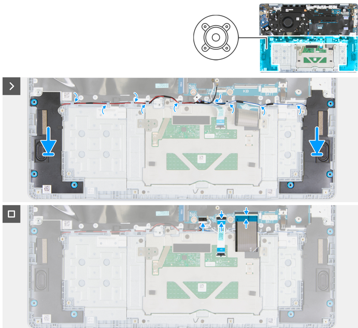
Rysunek 26. Instalowanie zestawu głośników
