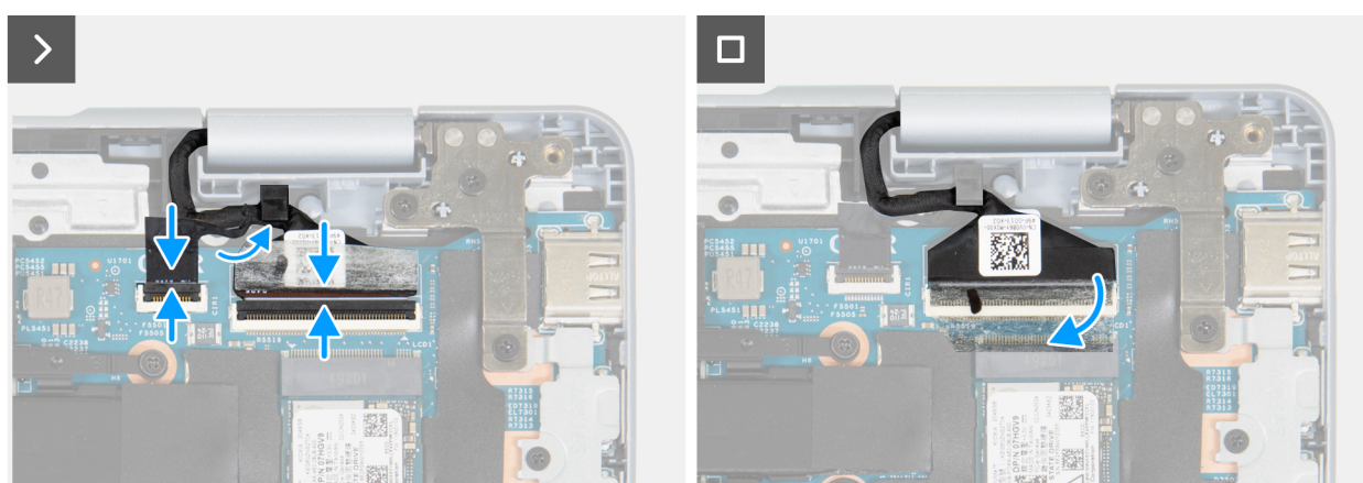
Rysunek 31. Instalowanie zestawu wyświetlacza — krok 2
