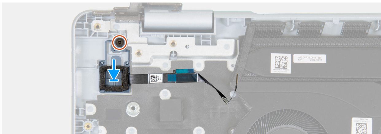
Rysunek 39. Instalowanie przycisku zasilania z opcjonalnym czytnikiem linii papilarnych
