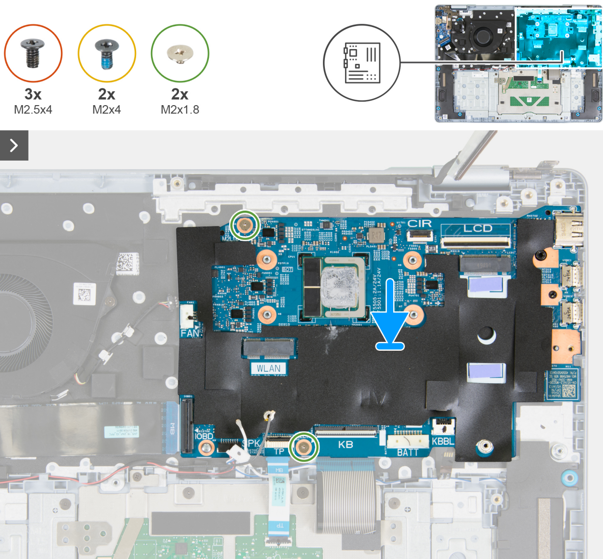
Rysunek 46. Instalowanie płyty głównej 1
