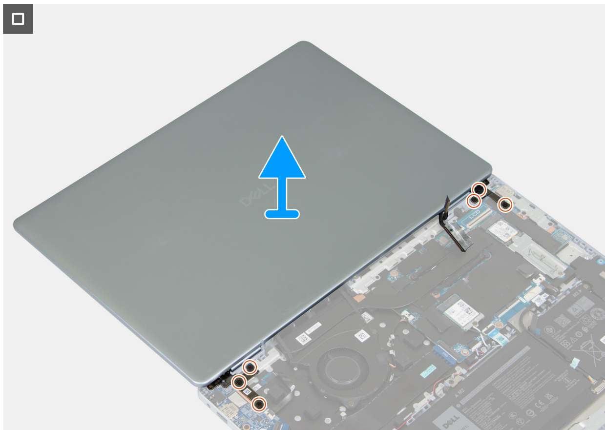
Rysunek 28. Wymontowywanie zestawu wyświetlacza — krok 2
