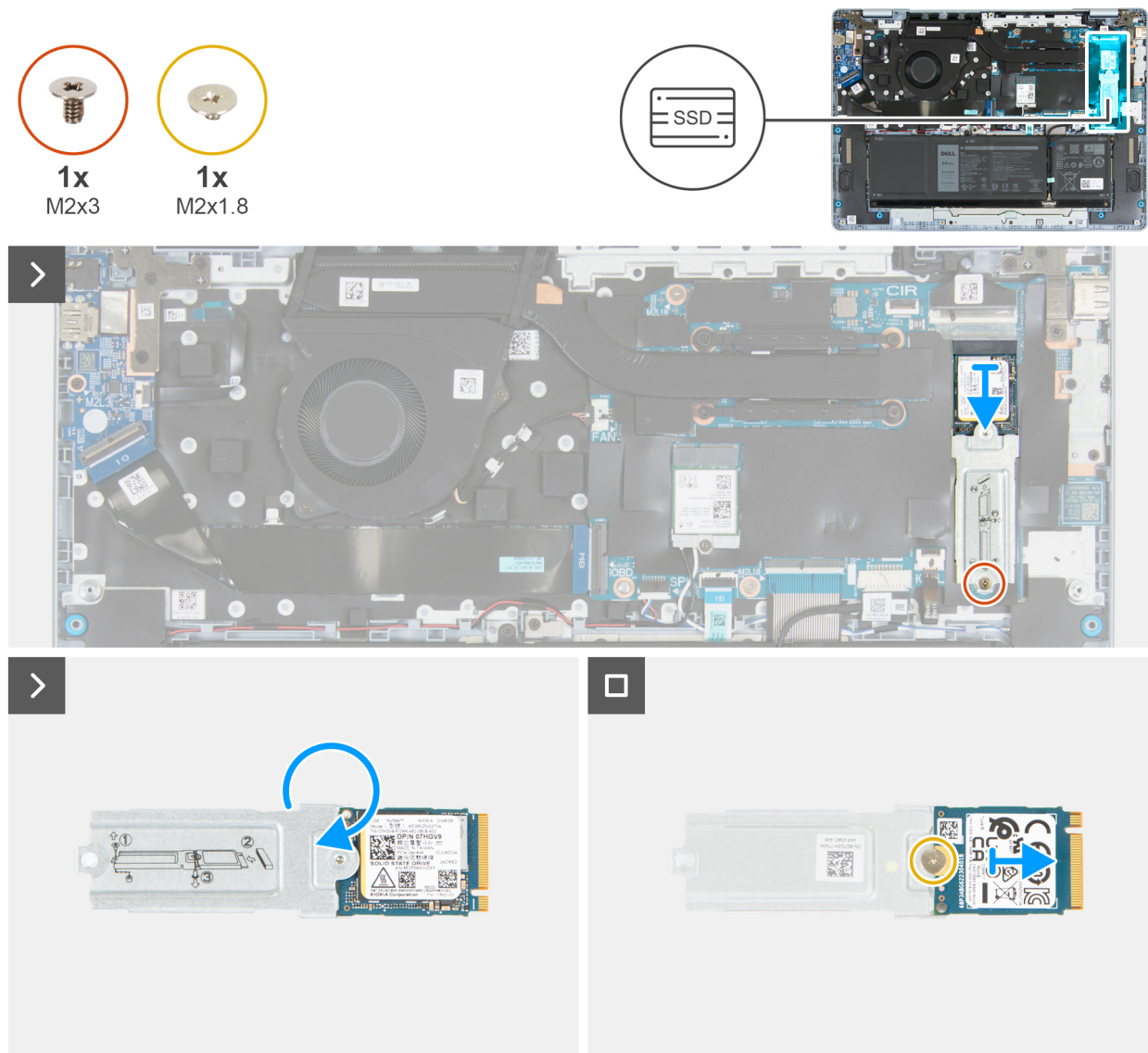
Rysunek 19. Wymontowywanie dysku SSD M.2 2230
