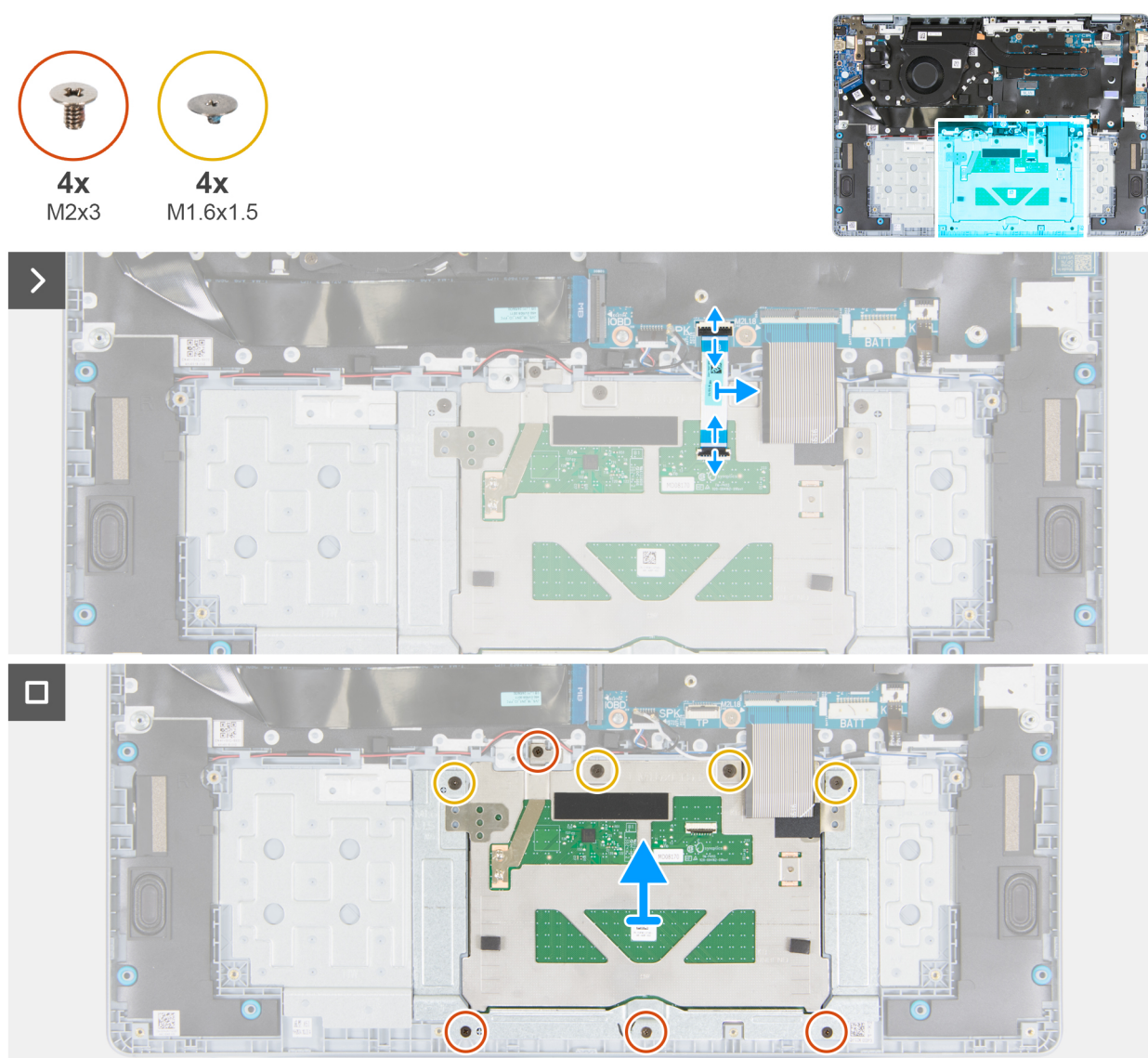
Rysunek 52. Wymontowywanie touchpada
