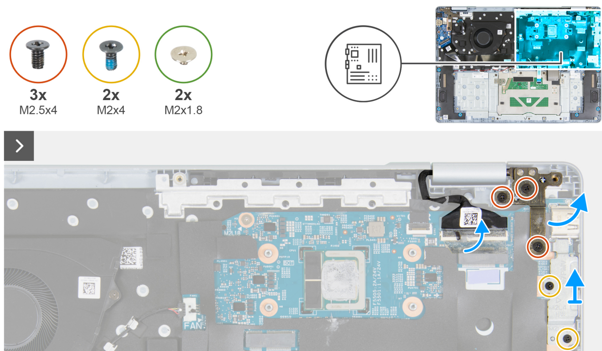
Rysunek 41. Wymontowywanie płyty głównej
