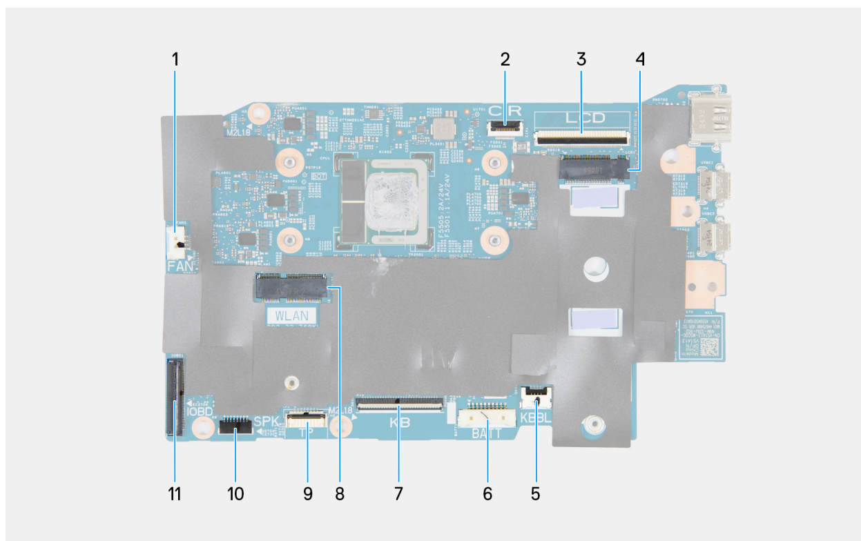
Rysunek 40. Elementy płyty głównej
