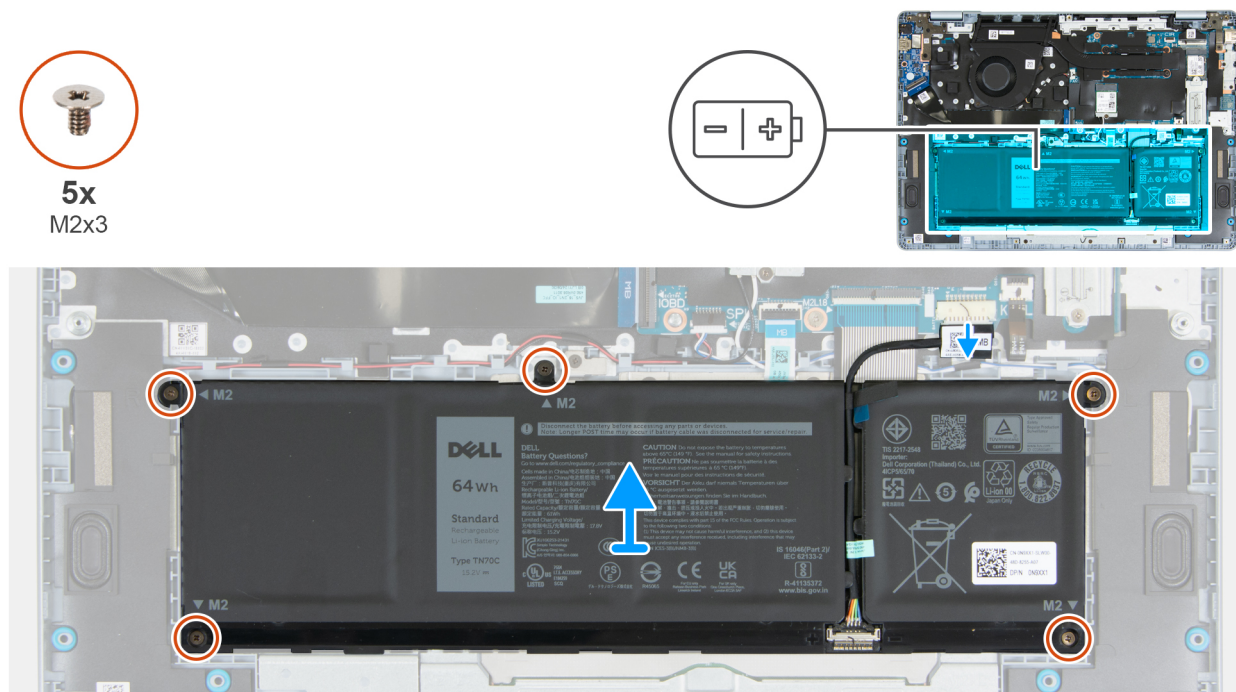
Rysunek 15. Wymontowywanie baterii
