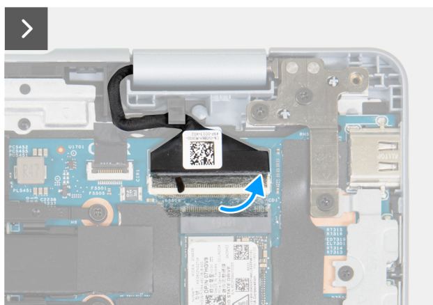
Rysunek 27. Wymontowywanie zestawu wyświetlacza — krok 1
