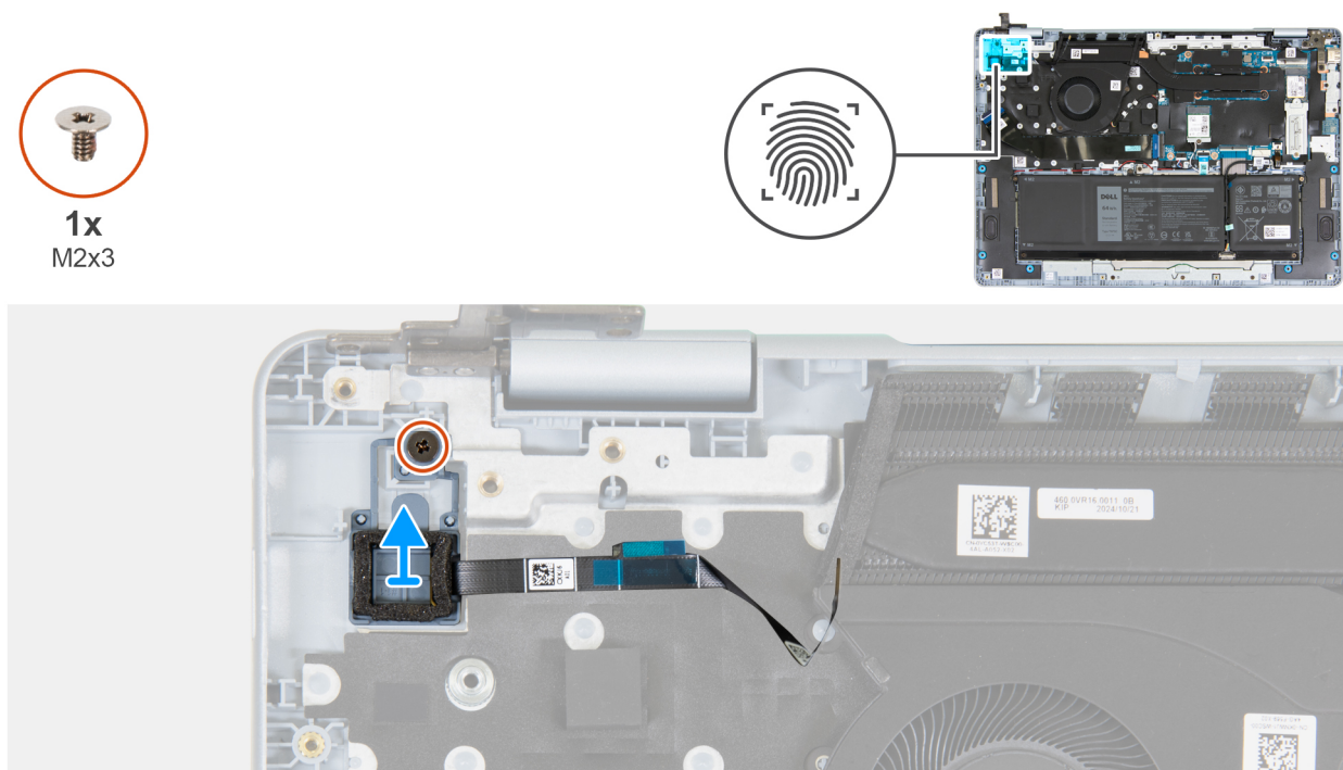
Rysunek 38. Wymontowywanie przycisku zasilania z opcjonalnym czytnikiem linii papilarnych
