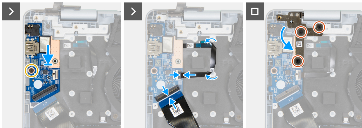
Rysunek 35. Instalowanie płyty we/wy
