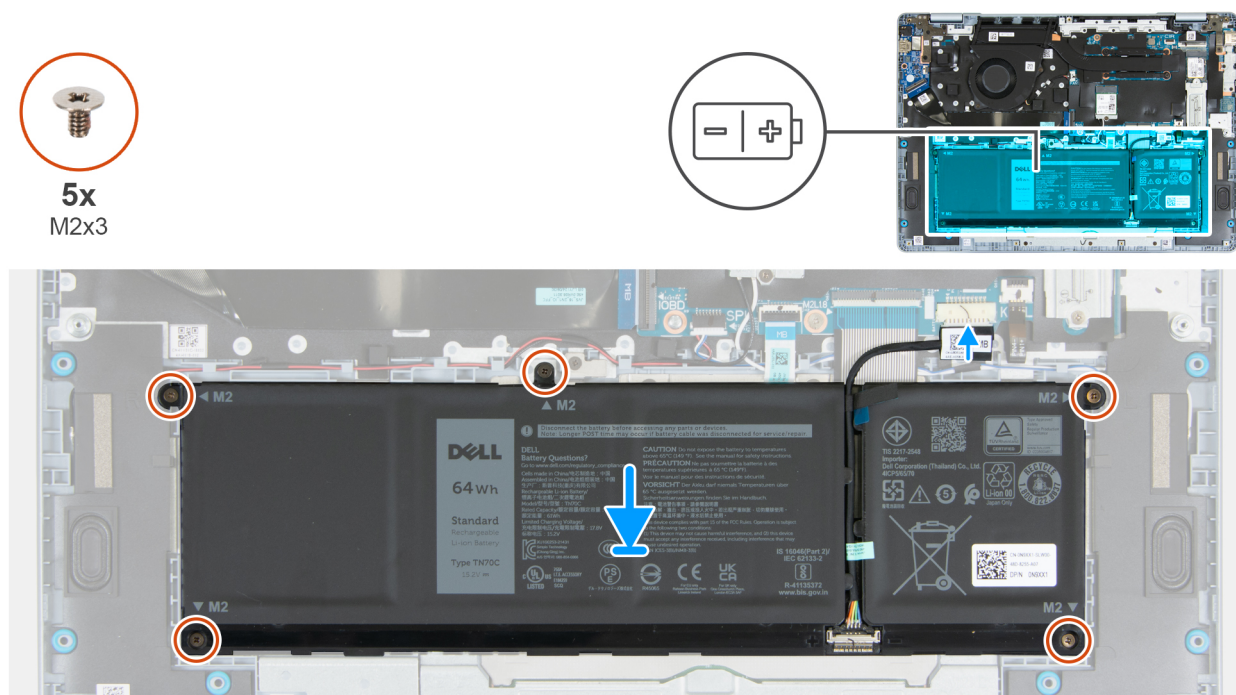
Rysunek 16. Instalowanie baterii
