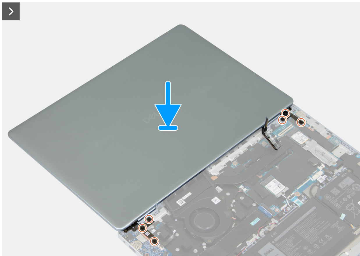
Rysunek 30. Instalowanie zestawu wyświetlacza — krok 1
