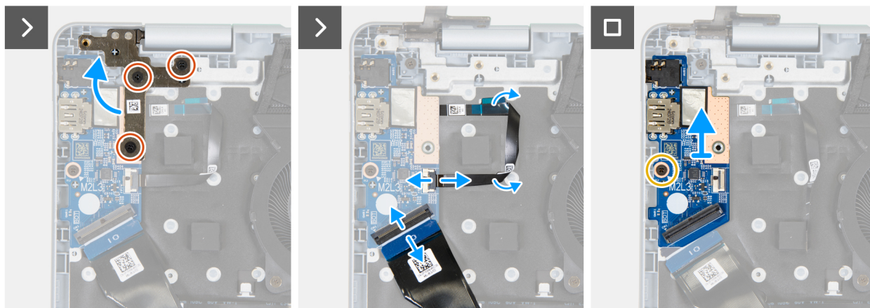
Rysunek 34. Wymontowywanie płyty we/wy
