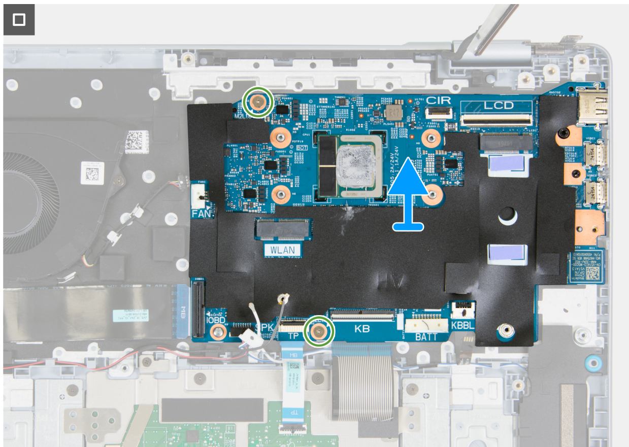
Rysunek 43. Wymontowywanie płyty głównej
