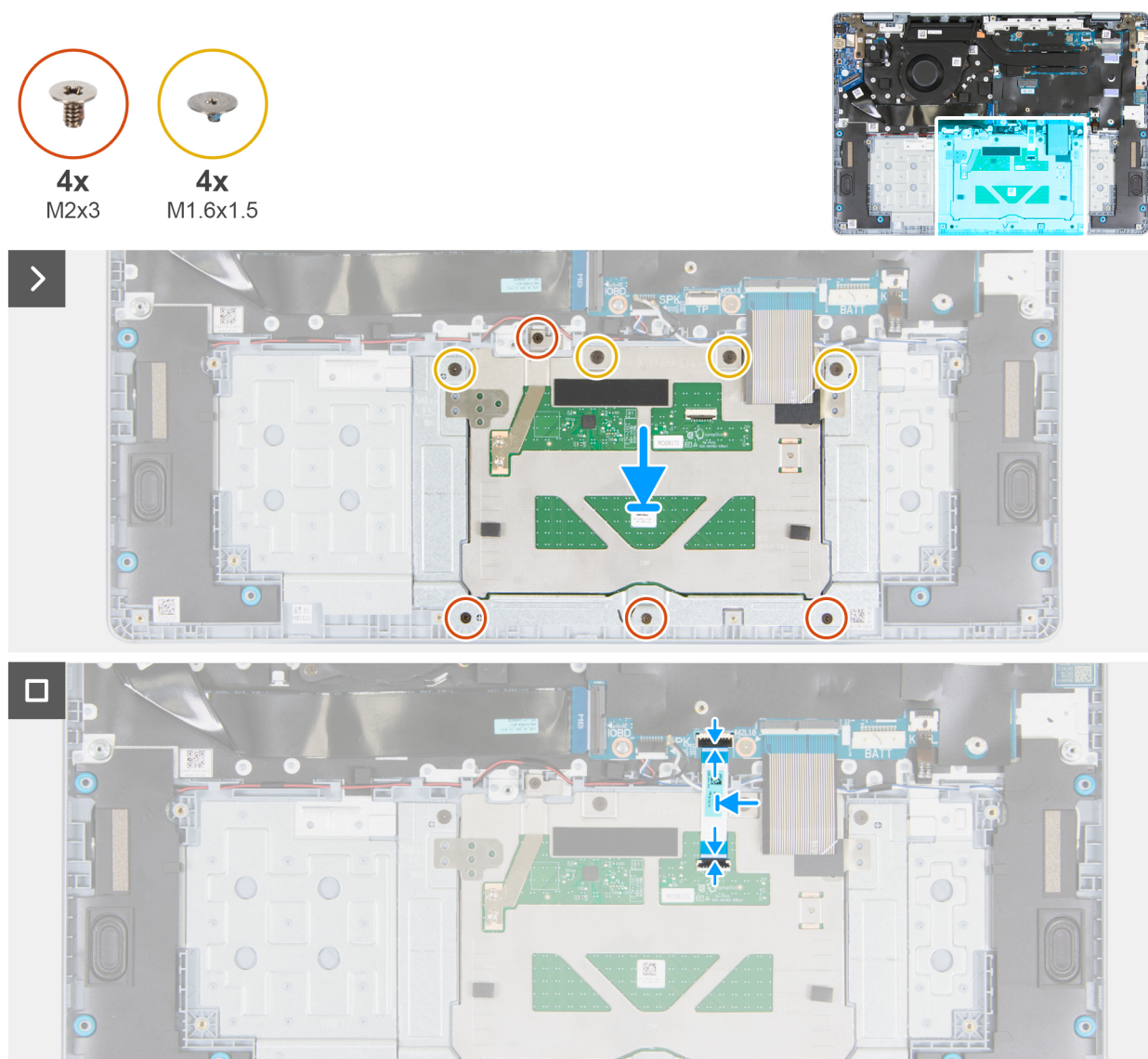
Rysunek 53. Instalowanie touchpada
