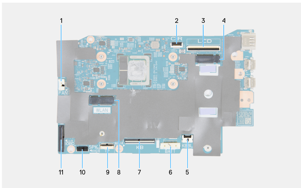
Rysunek 45. Elementy płyty głównej
