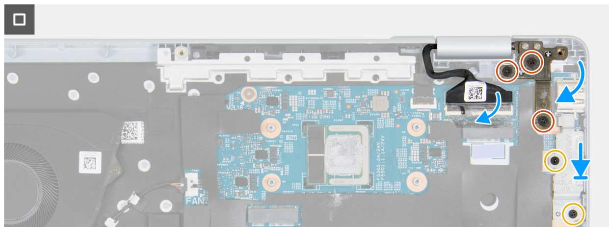
Rysunek 48. Instalowanie płyty głównej
