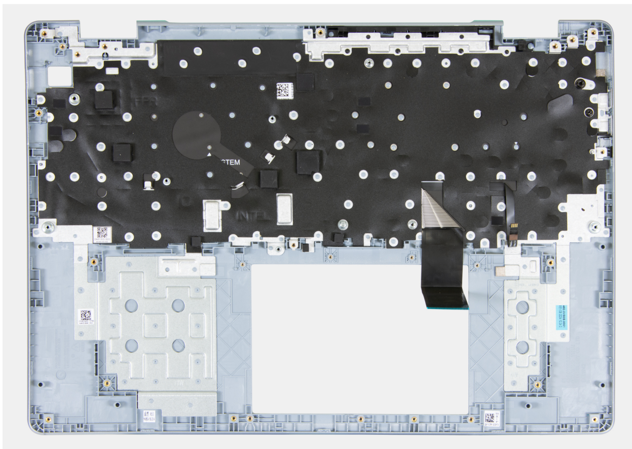
Rysunek 54. Zestaw podpórki na nadgarstek i klawiatury
