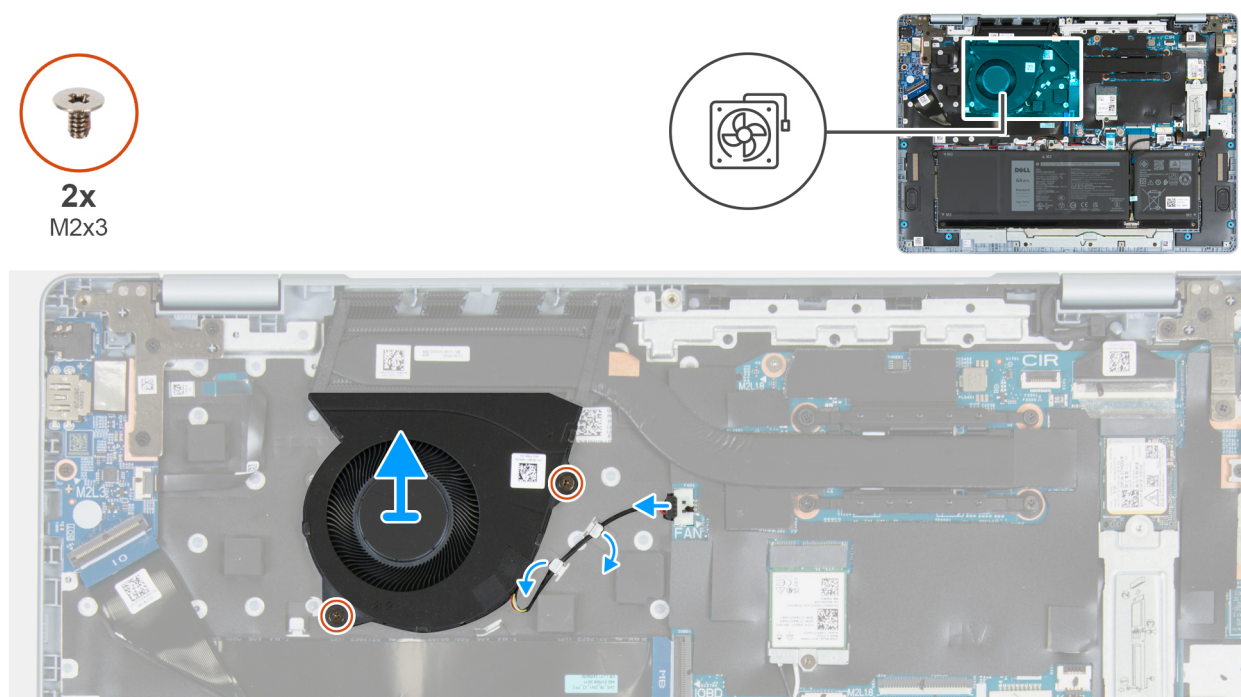
Rysunek 21. Wymontowywanie wentylatora
