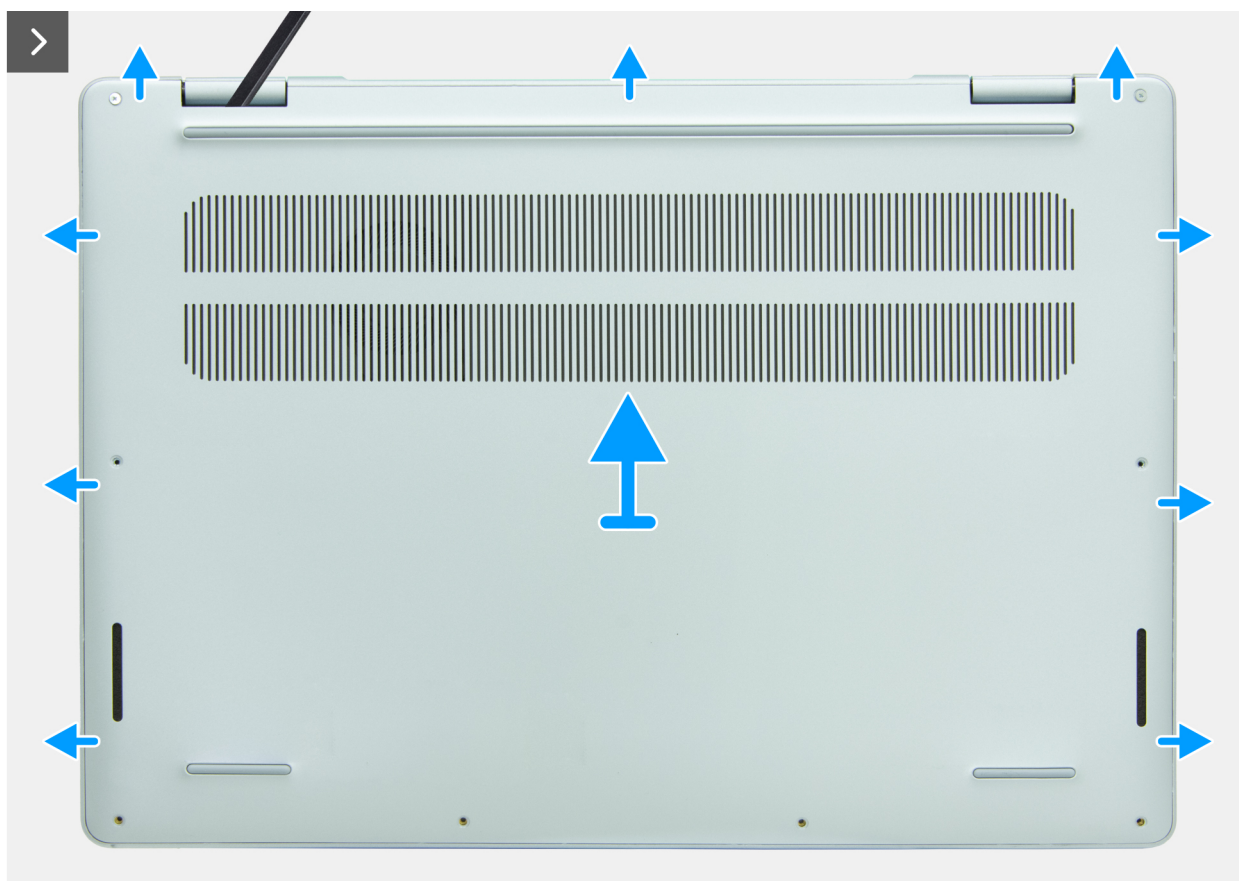
Rysunek 10. Wymontowywanie pokrywki dolnej
