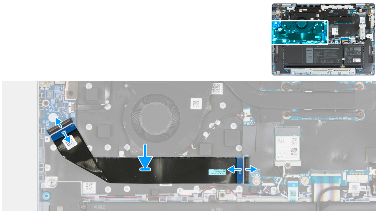
Rysunek 33. Instalowanie kabla płyty we/wy
