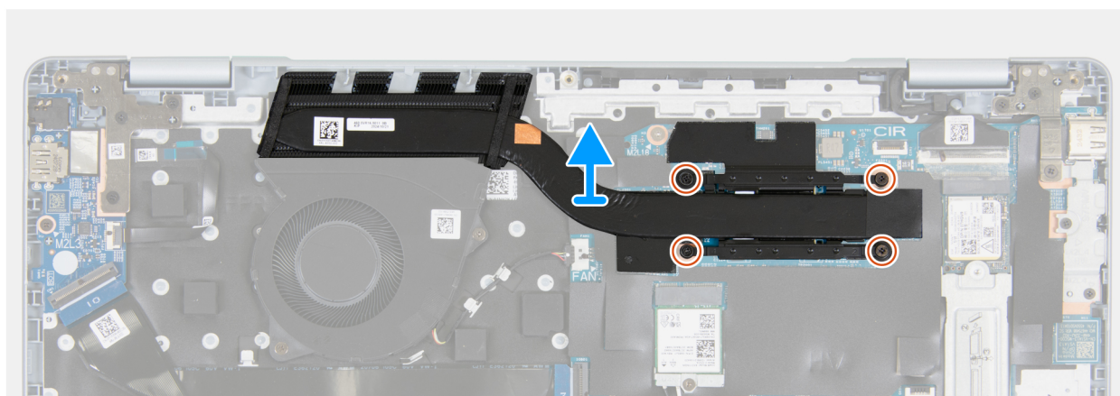
Rysunek 50. Wymontowywanie radiatora
