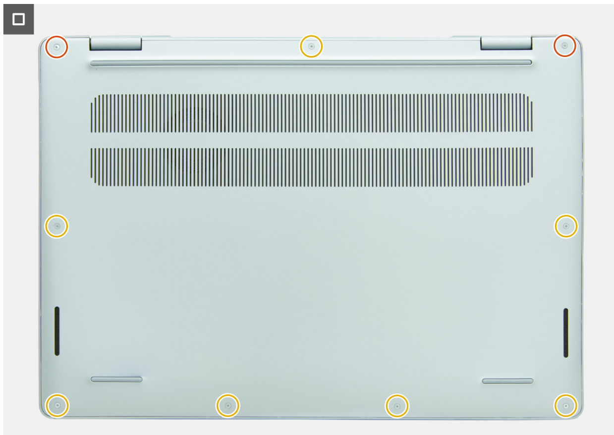
Rysunek 14. Instalowanie pokryw dolnej
