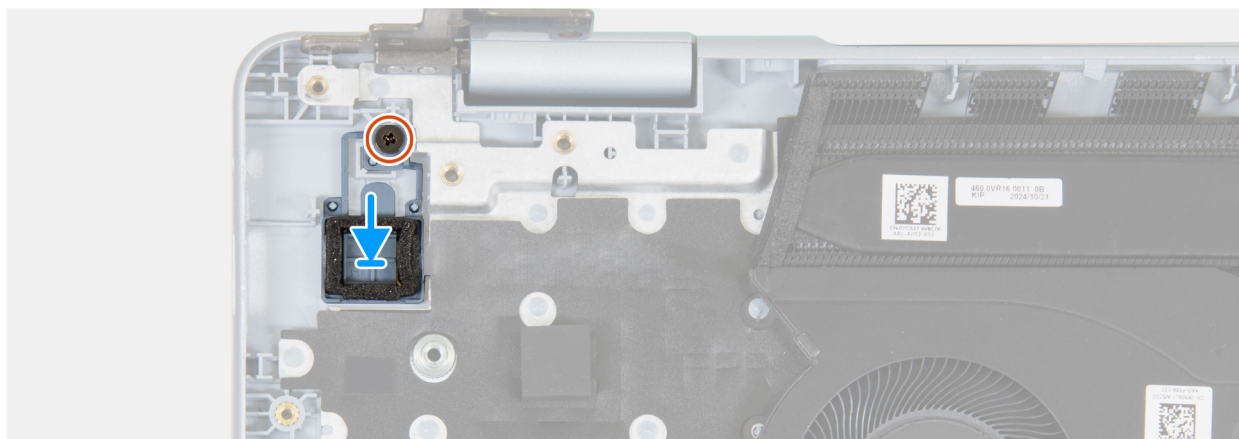
Rysunek 37. Instalowanie przycisku zasilania
