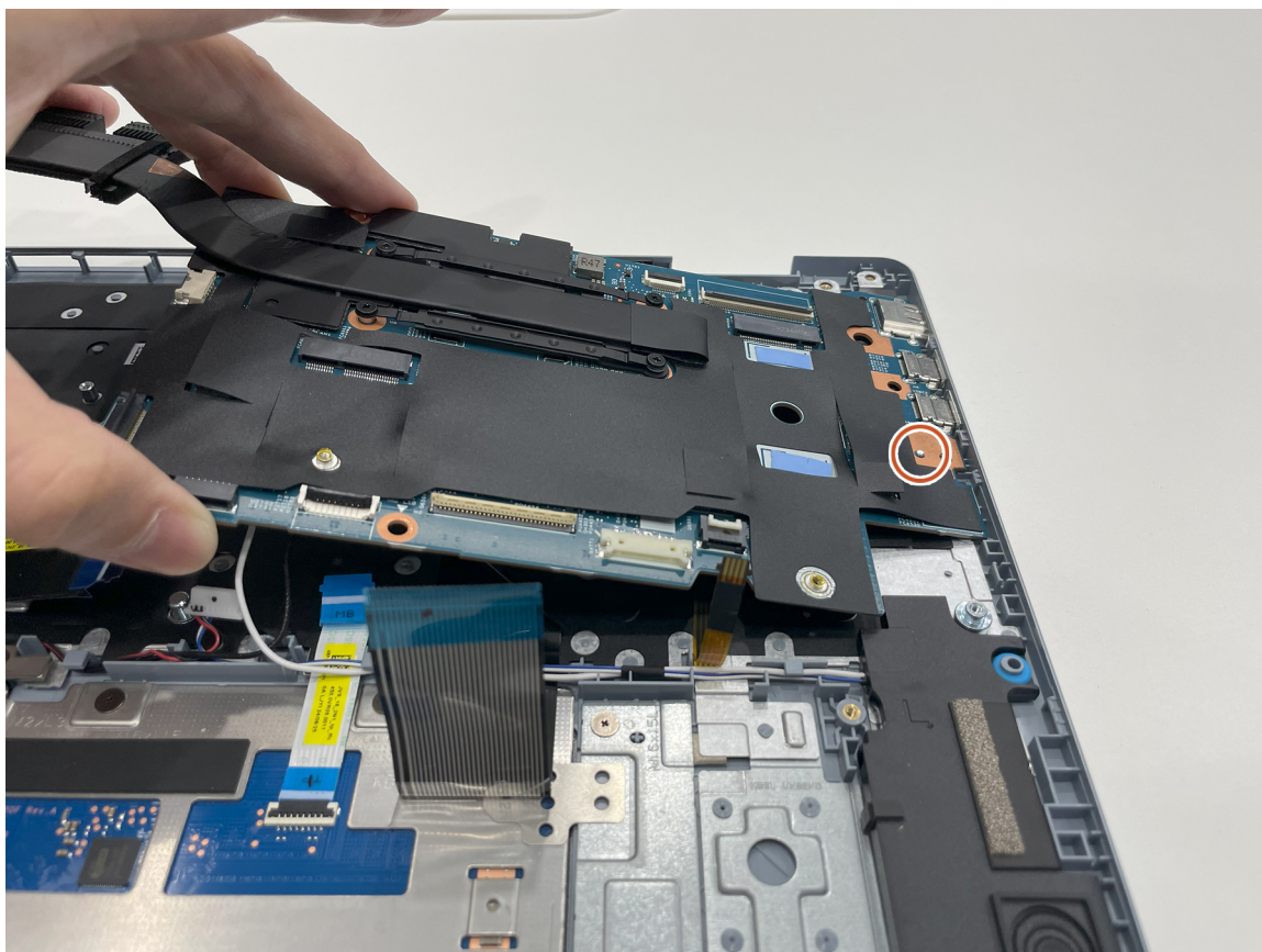
Rysunek 49. Instalowanie płyty głównej bez jej uszkodzenia
