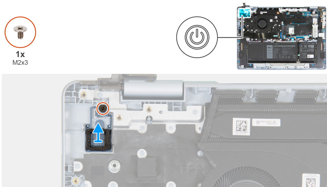
Rysunek 36. Wymontowywanie przycisku zasilania
