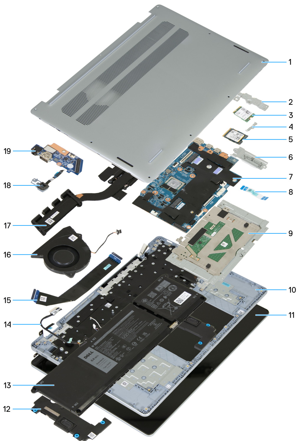
Rysunek 8. Ilustracja: główne elementy komputera Dell 16 Plus DB16250
