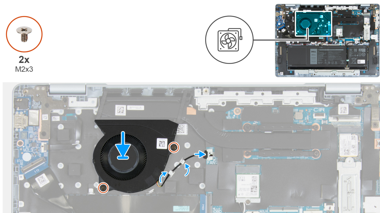
Rysunek 22. Instalowanie wentylatora
