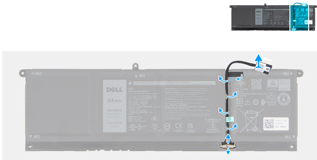
Rysunek 17. Wymontowywanie kabla baterii
