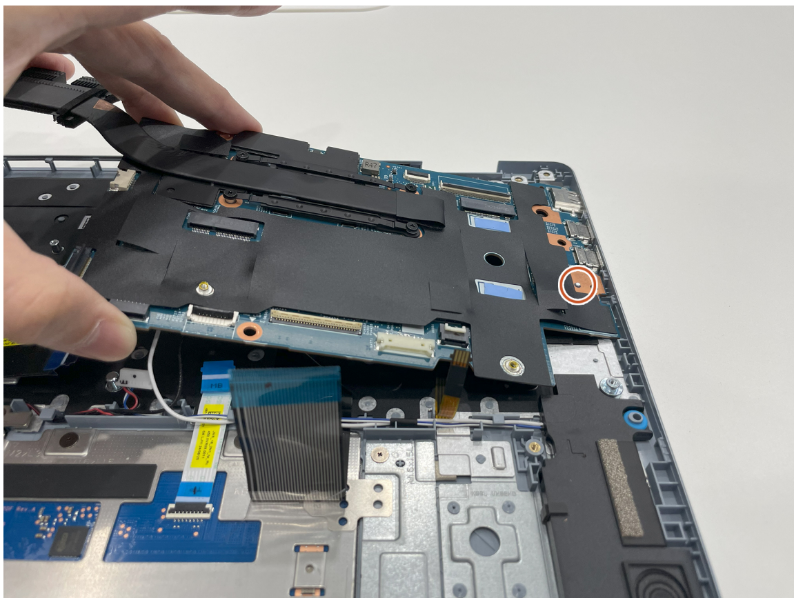
Rysunek 42. Wymontowywanie płyty głównej bez jej uszkodzenia
