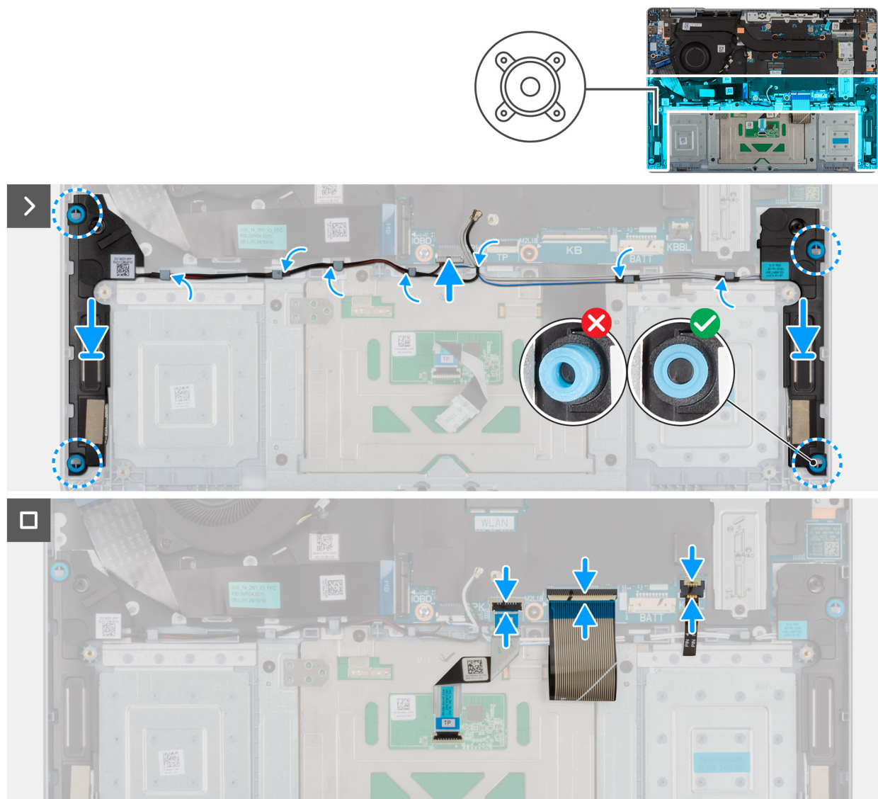
Rysunek 35. Instalowanie zestawu głośników
