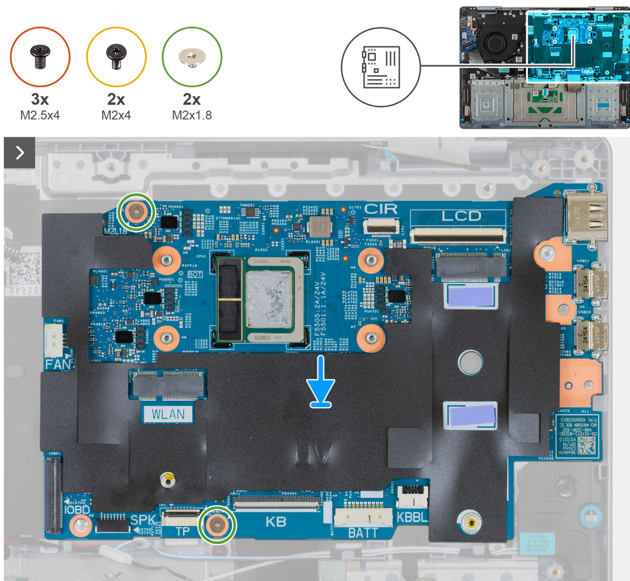
Rysunek 44. Instalowanie płyty głównej
