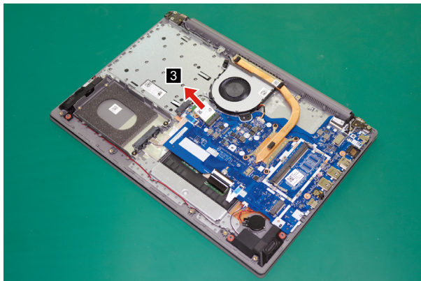
Figure 14. Remove the PCI Express mini card
