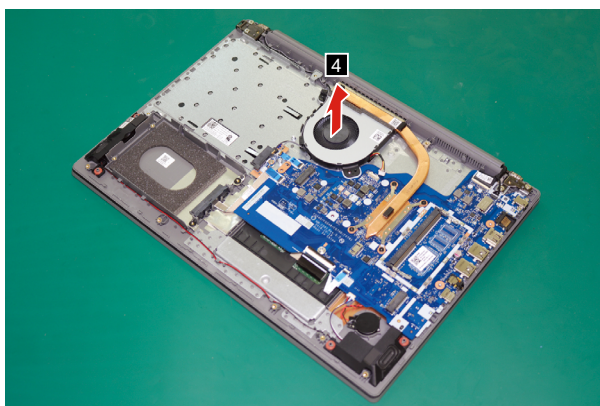
Figure 17. Remove the fan
