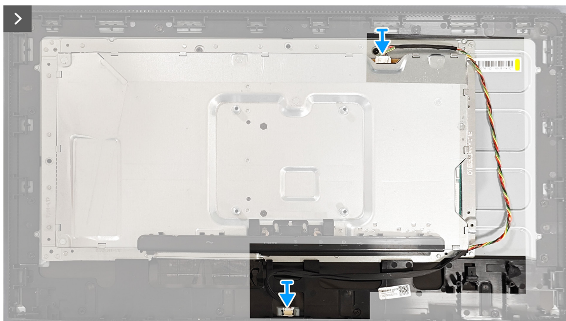
Rysunek 20. Instalacja metalowej ramy
