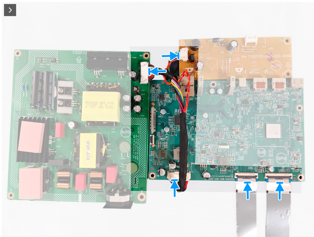
Rysunek 25. Instalacja płyty systemowej i płyty zasilania
