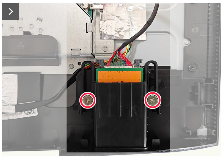
Rysunek 11. Zdejmowanie koncentratora USB
