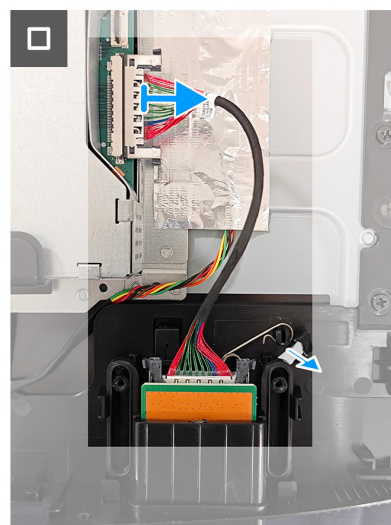
Rysunek 11. Zdejmowanie koncentratora USB
