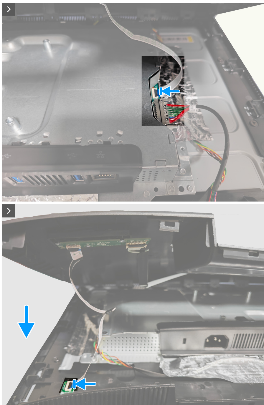
Rysunek 5. Instalacja pokrywy tylnej
