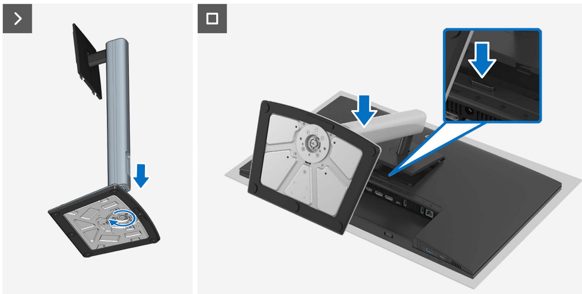
Rysunek 2. Instalacja wspornika
