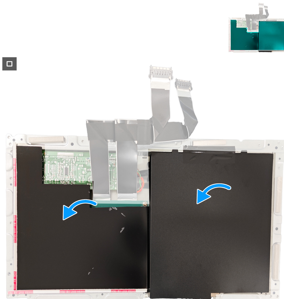
Rysunek 22. Zdejmowanie płyty systemowej i płyty zasilania
