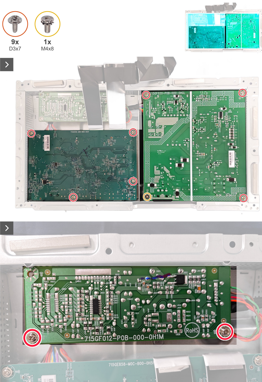
Rysunek 26. Instalacja płyty systemowej i płyty zasilania
