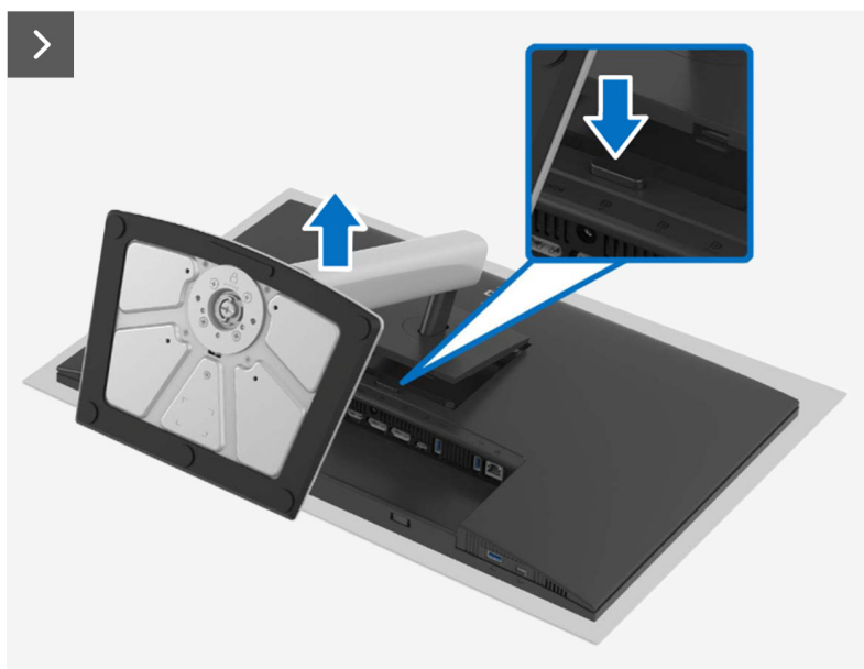
Rysunek 1. Zdejmowanie wspornika
