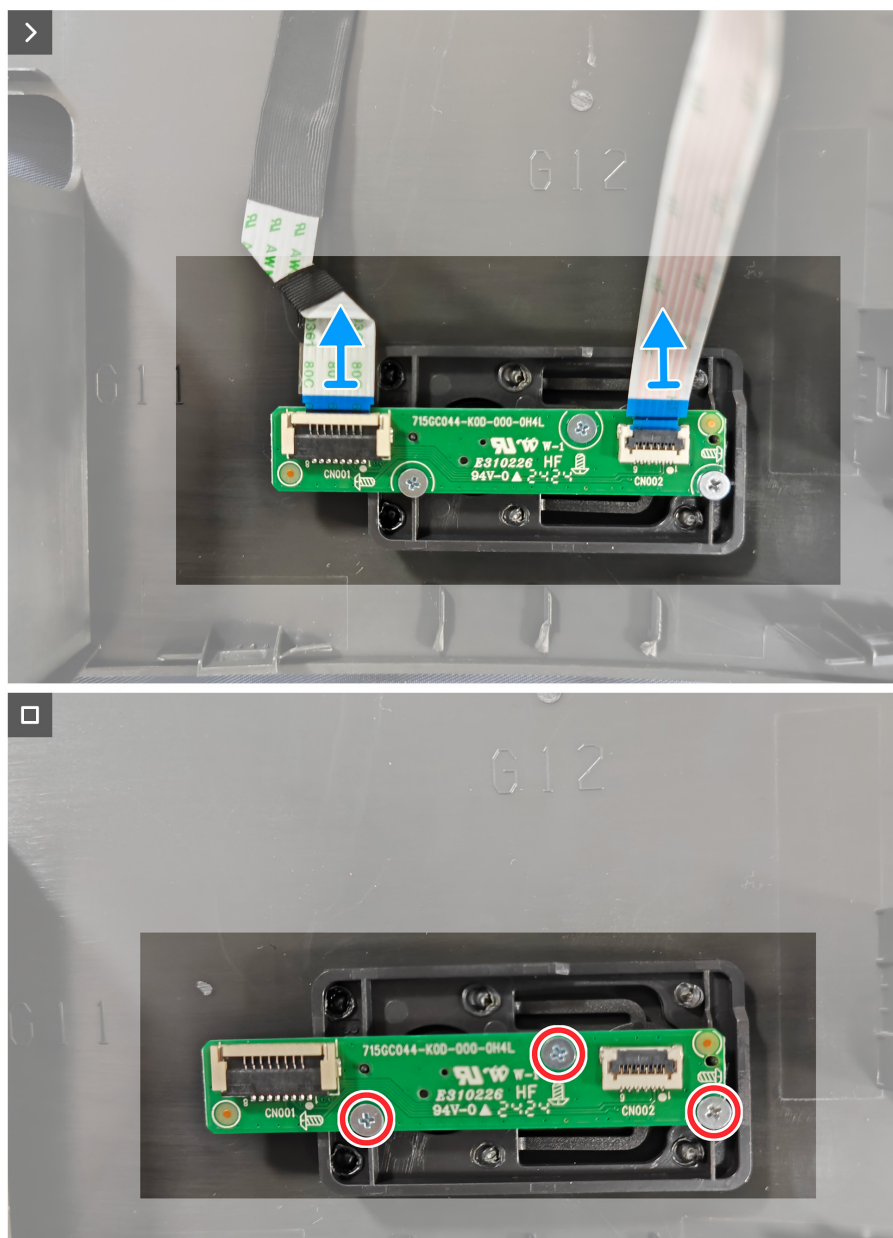
Rysunek 7. Zdejmowanie płyty klawiatury
