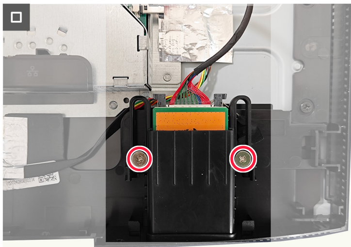
Rysunek 12. Instalacja koncentratora USB
