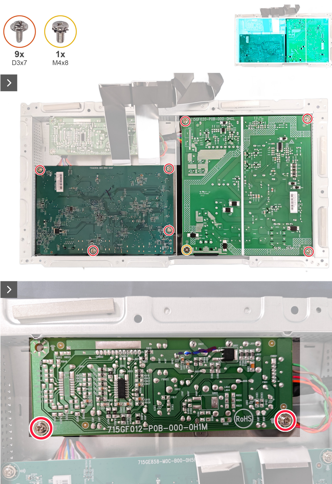
Rysunek 23. Zdejmowanie płyty systemowej i płyty zasilania
