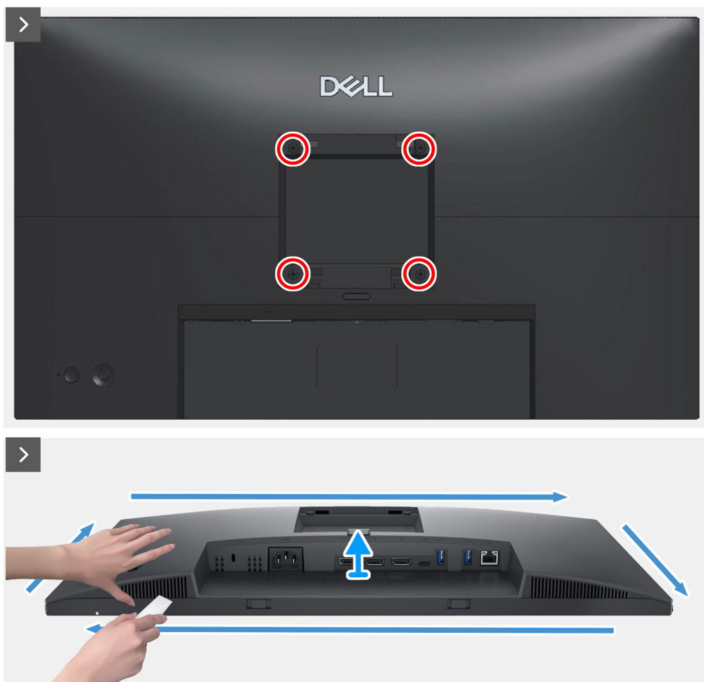
Rysunek 3. Zdejmowanie pokrywy tylnej
