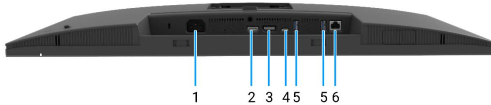
Figure 5. Vue de dessous du moniteur
