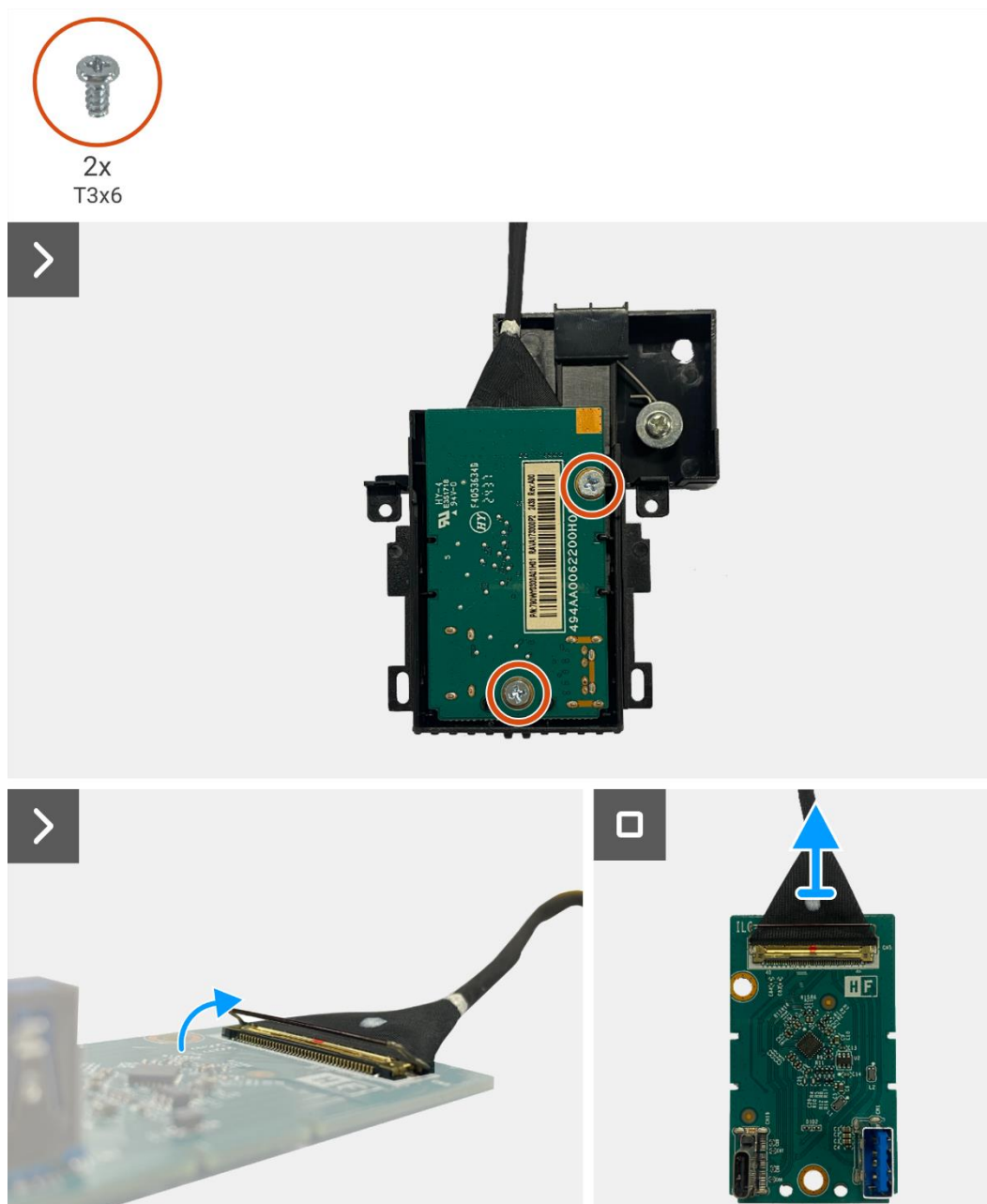
Figure 42. Retrait de la carte QAP
