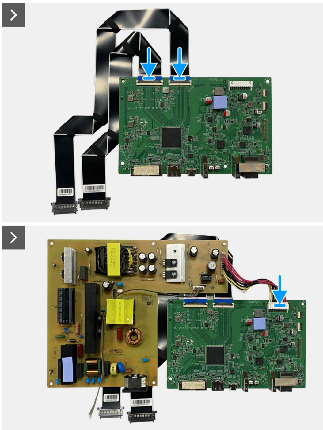
Figure 52. Installation de la carte interface
