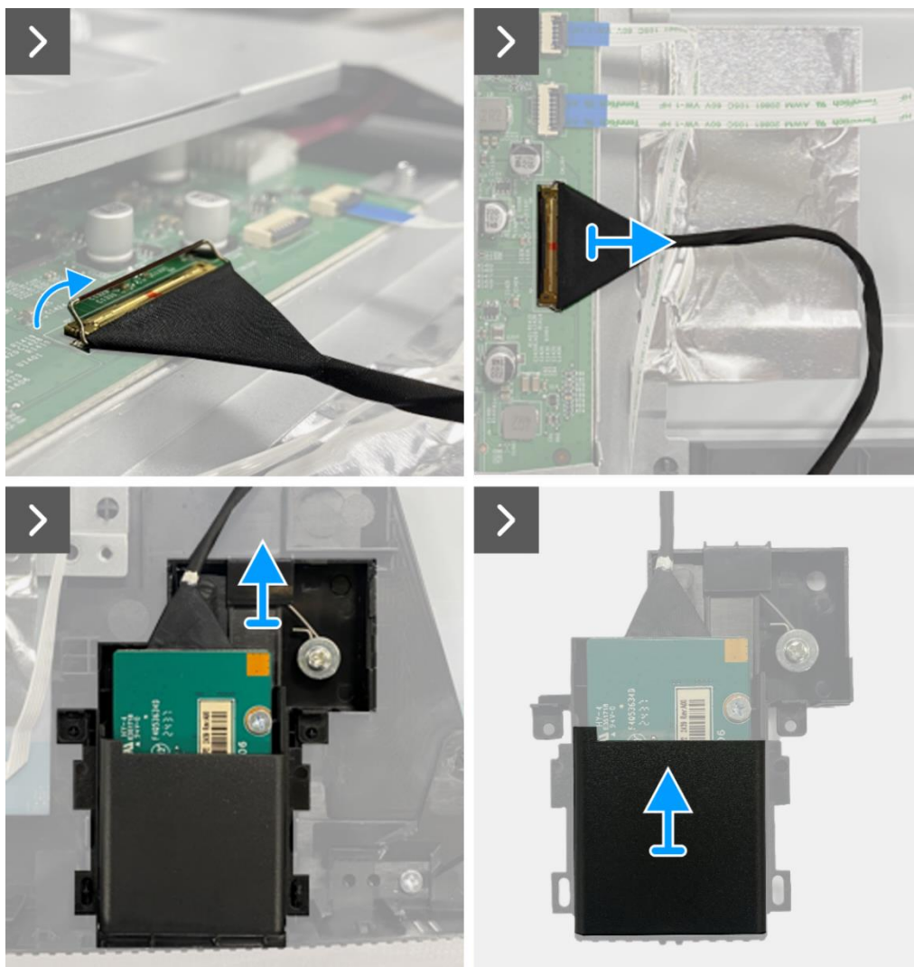
Figure 71. Retrait de la carte QAP
