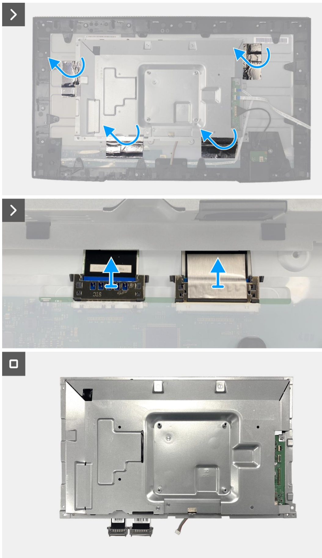
Figure 46. Retrait de l'assemblage du châssis
