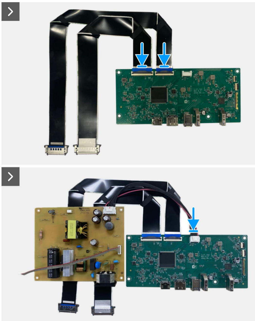
Figure 22. Installation de la carte interface
