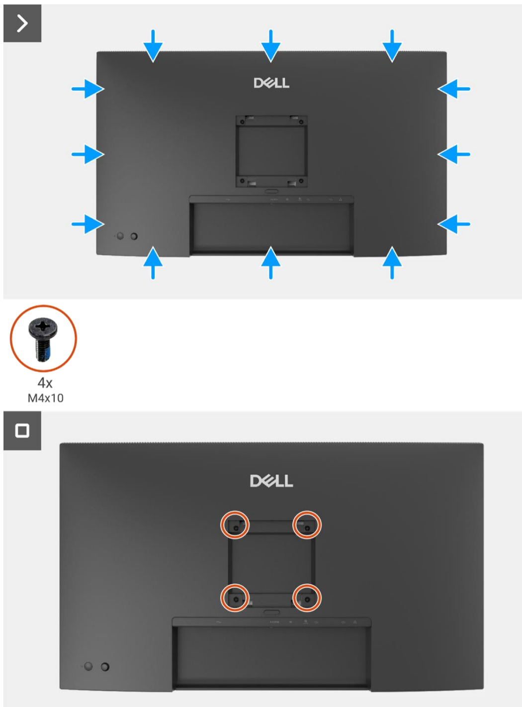
Figure 68. Installation du couvercle arrière
