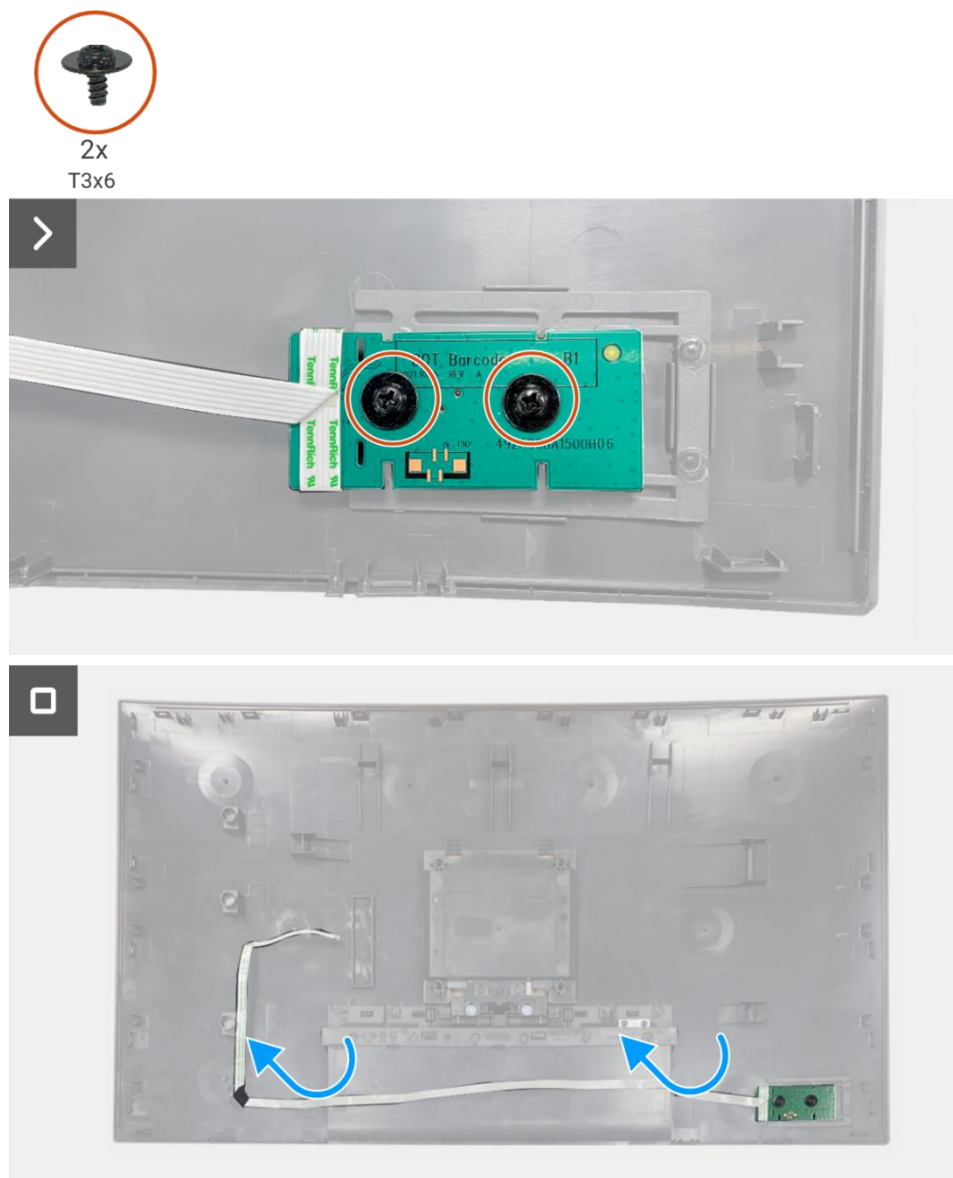
Figure 9. Retrait de la carte clavier
