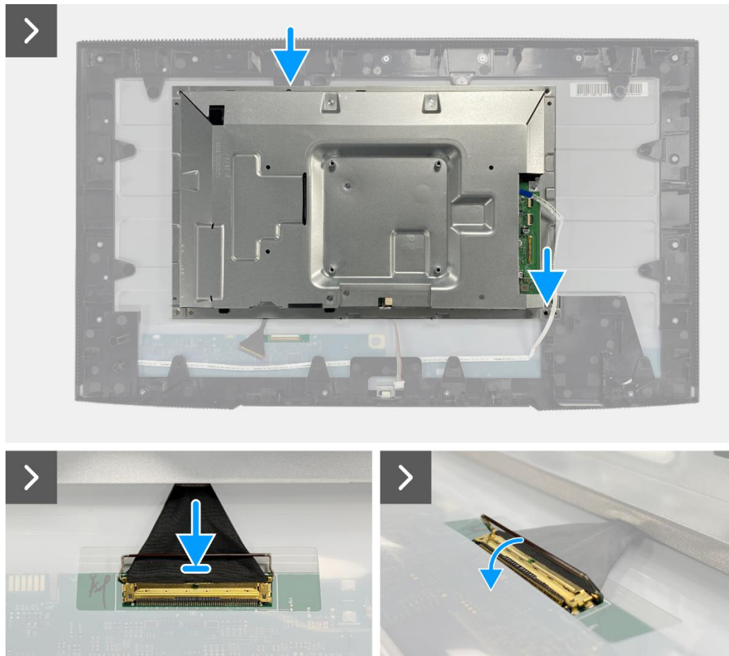
Figure 77. Installation de l'assemblage du châssis
