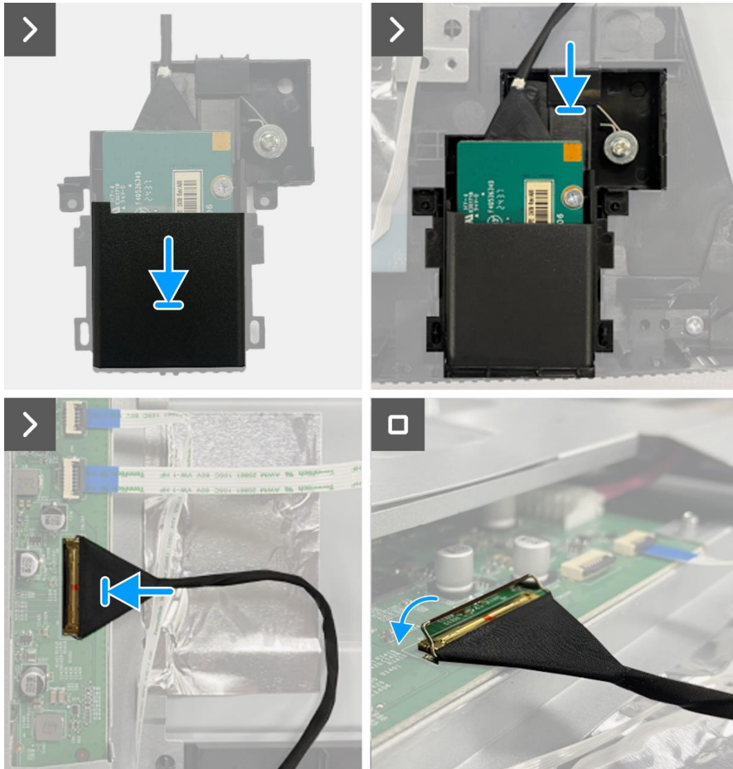
Figure 74. Installation de la carte QAP
