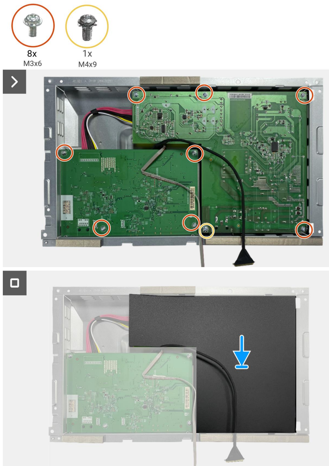
Figure 84. Installation de la carte interface
