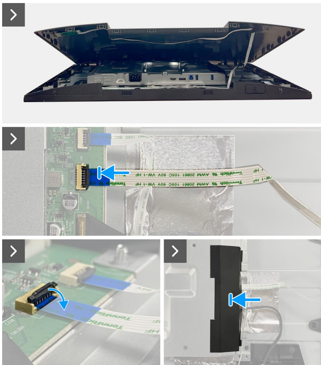
Figure 37. Installation du couvercle arrière
