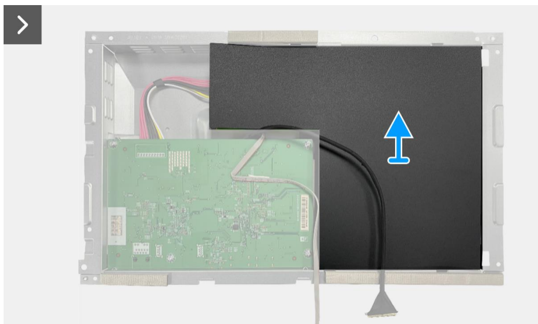
Figure 79. Retrait de la carte interface
