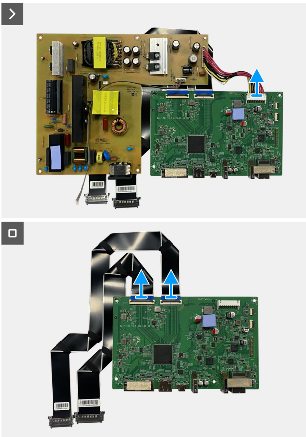
Figure 51. Retrait de la carte interface
