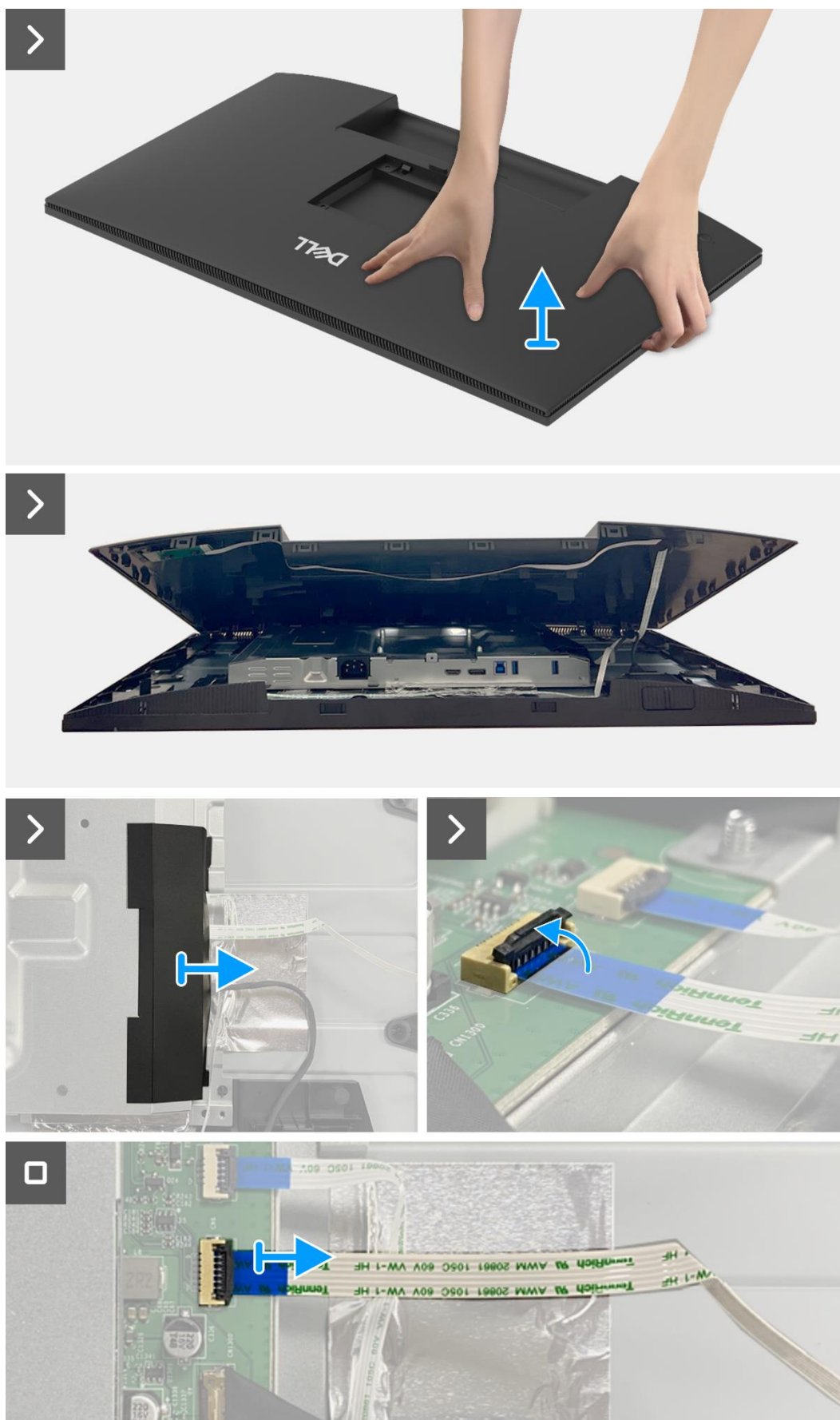
Figure 36. Retrait du couvercle arrière
