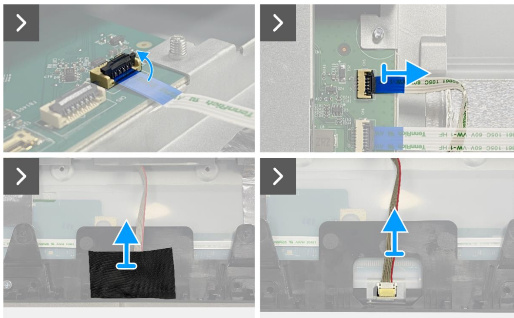
Figure 15. Retrait de l'assemblage du châssis
