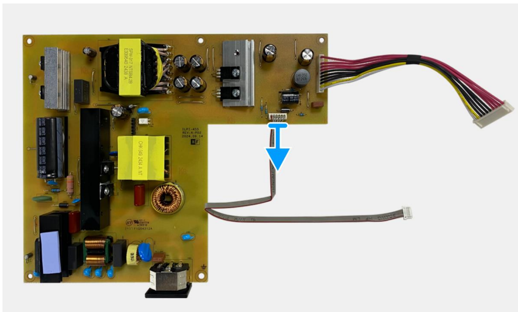
Figure 85. Retrait de la carte d'alimentation
