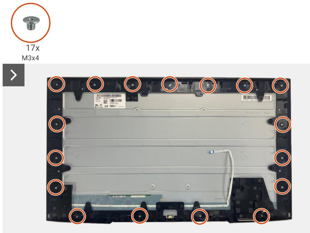
Figure 27. Retrait de la carte LED
