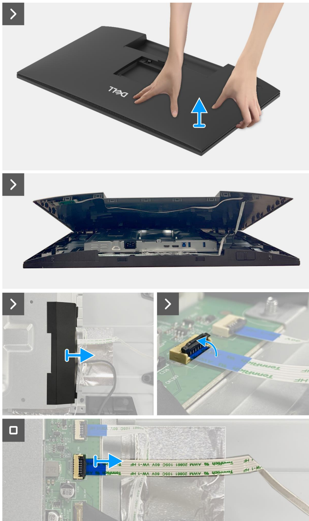
Figure 6. Retrait du couvercle arrière
