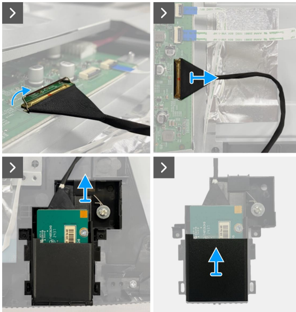
Figure 41. Retrait de la carte QAP
