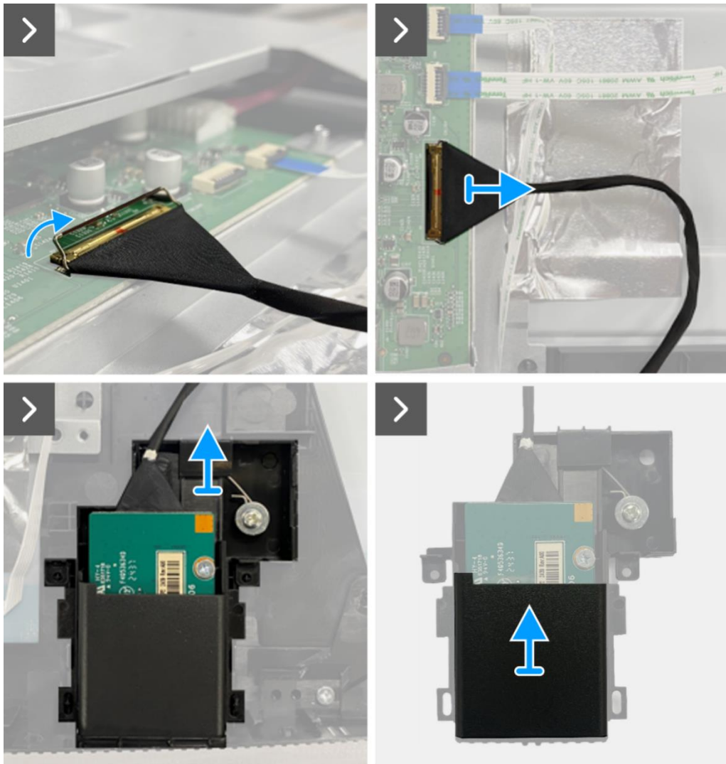
Figure 11. Retrait de la carte QAP
