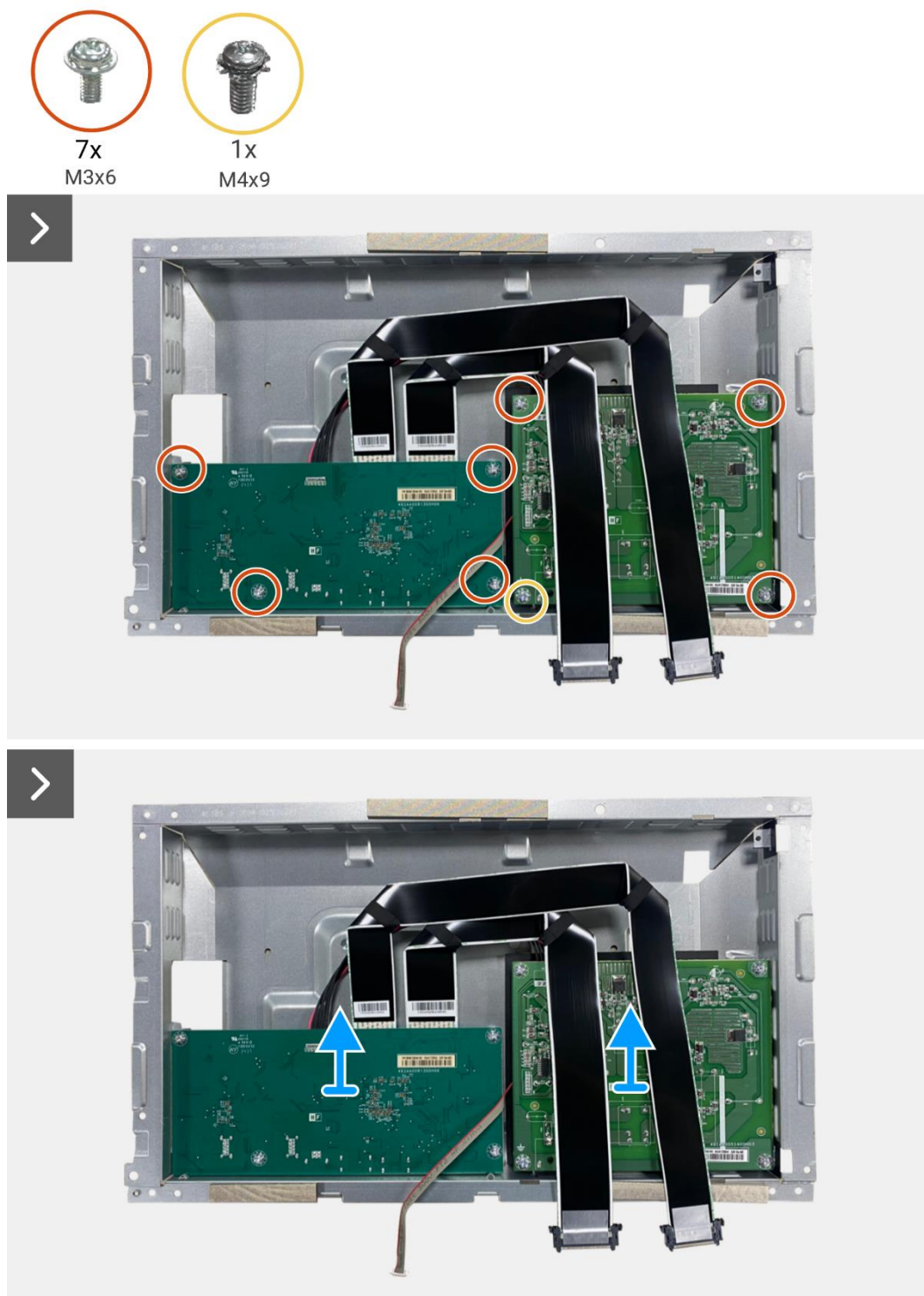
Figure 20. Retrait de la carte interface
