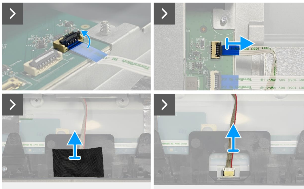
Figure 45. Retrait de l'assemblage du châssis
