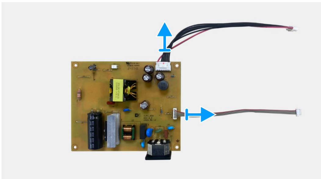
Figure 25. Retrait de la carte d'alimentation
