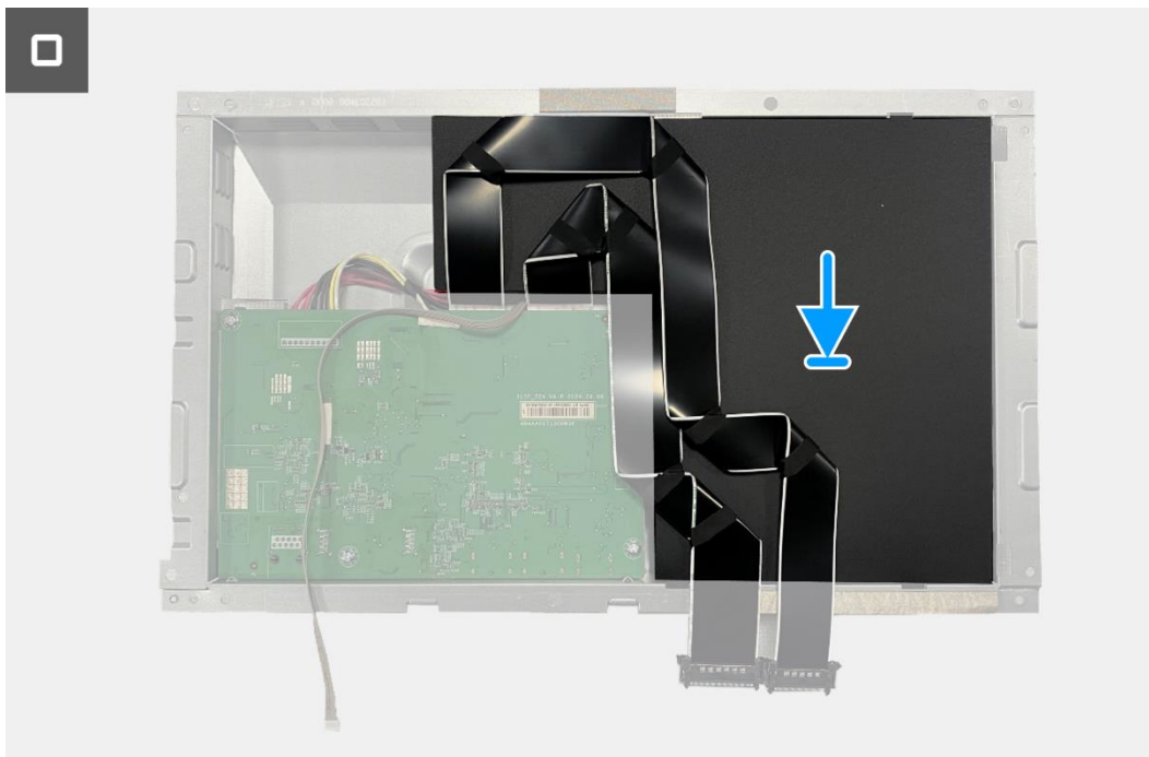
Figure 54. Installation de la carte interface
