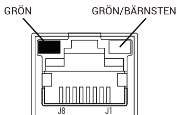
Bild 13. RJ45-portkontakt
