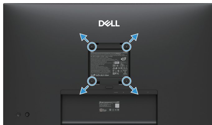
Bild 55. VESA väggmontering
